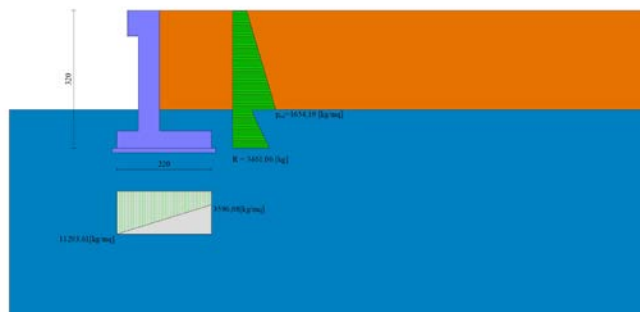
Fig. 4 - Diagramma delle pressioni (combinazione statica) (Combinazione n° 10)
