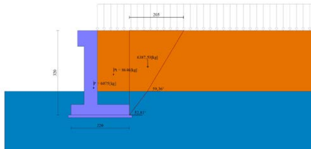
Fig. 3 - Cuneo di spinta (combinazione statica) (Combinazione n° 10)
