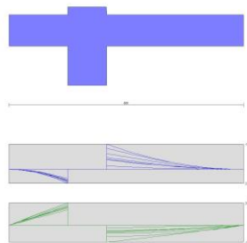
Fig. 7 - Fondazione (Inviluppo)
