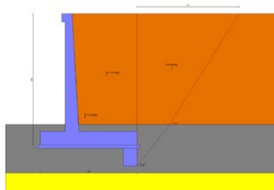
Fig. 3 - Cuneo di spinta (combinazione statica) (Combinazione n° 1)
