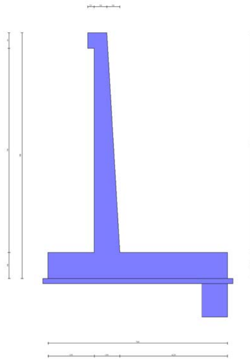
Fig. 1 - Sezione quotata del muro
