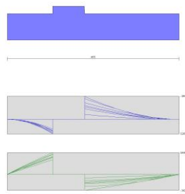
Fig. 7 - Fondazione (Inviluppo)
