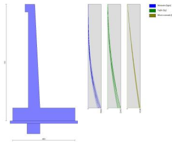
Fig. 5 - Paramento (Inviluppo)
