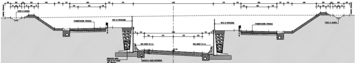
Fig. 3.2.21 - Svincolo Cà Brusà- Sezione
