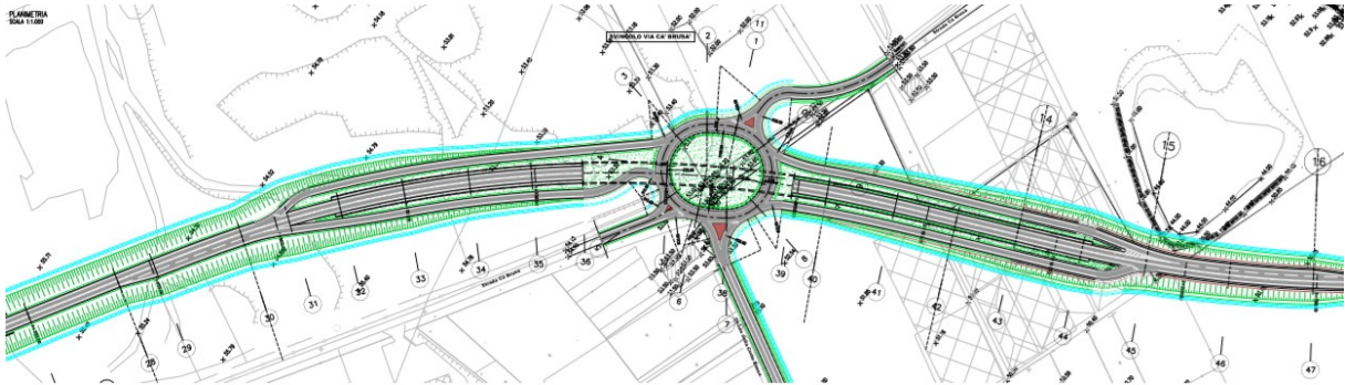
Fig. 3.2.20 - Svincolo Cà Brusà - Planimetria
