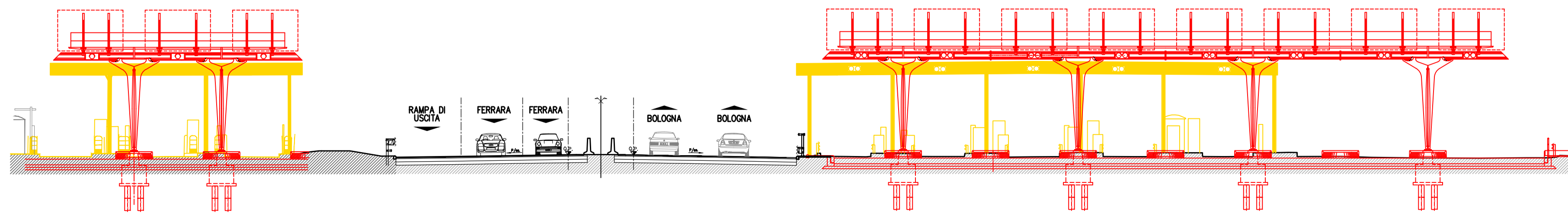
PROSPETTO BARRIERA - CONFRONTO DEMOLIZIONI E COSTRUZIONI SCALA 1:200
