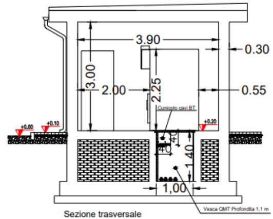
Sezione trasversale
