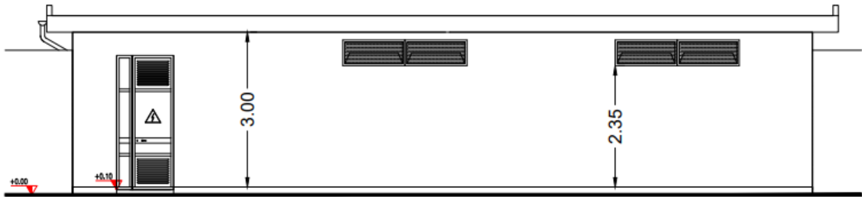
Prospetto esterno
