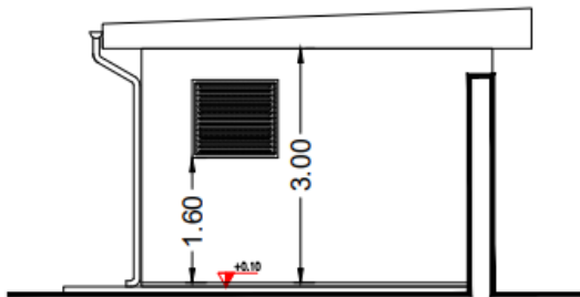
Prospetto laterale
