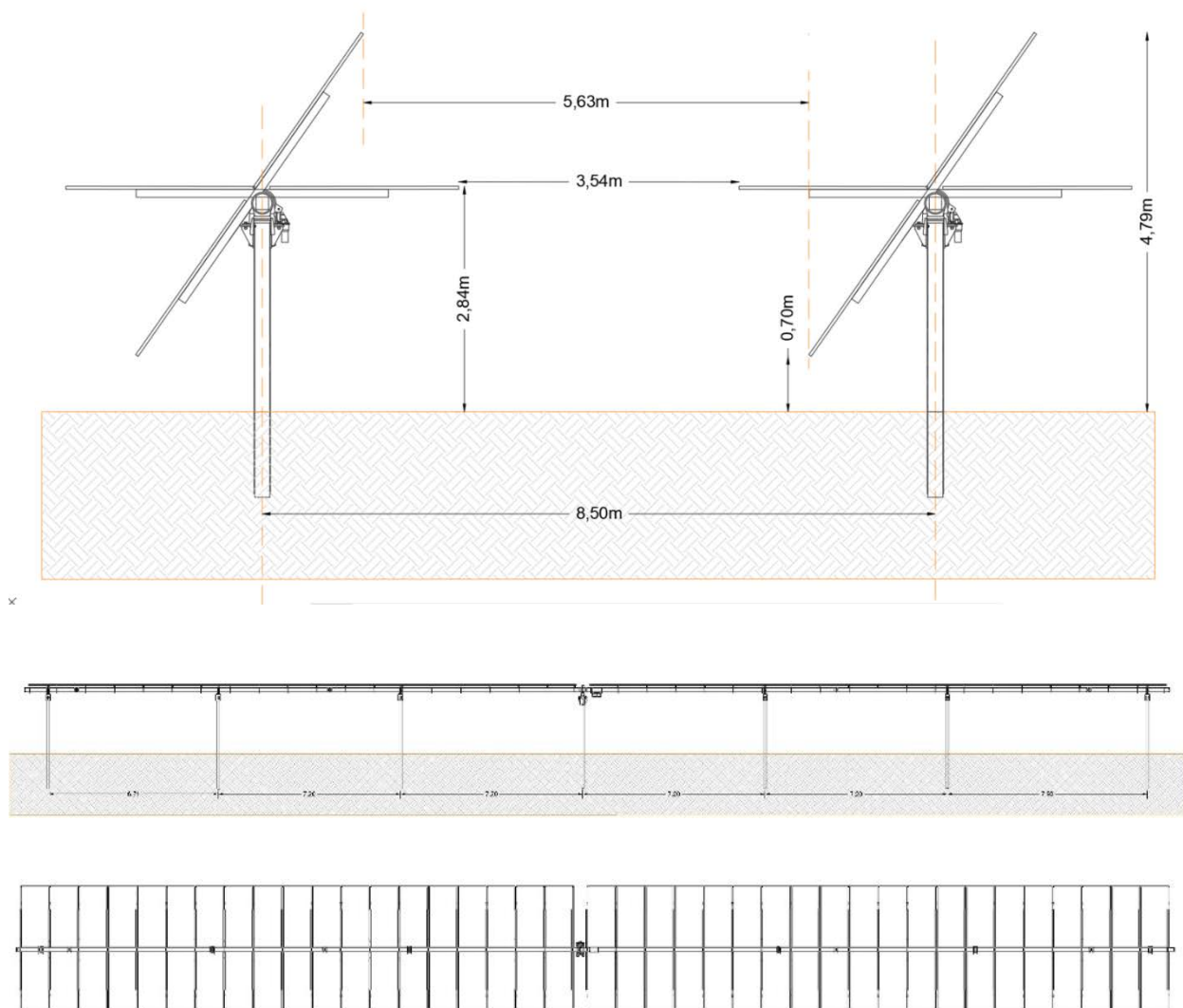
Viste del tracker: laterali, frontale e dall'alto
