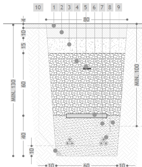
Figura 2: Sezione tipo cavidotto MT composta da due terne da 630 mm 2
