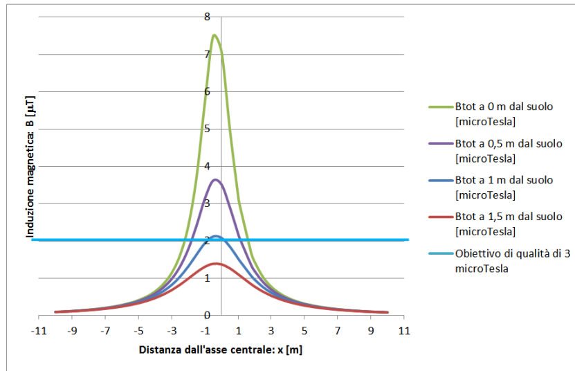
Figura 3: Andamento del campo magnetico generato dal cavidotto MT, composto da due terne da 630 mm 2
