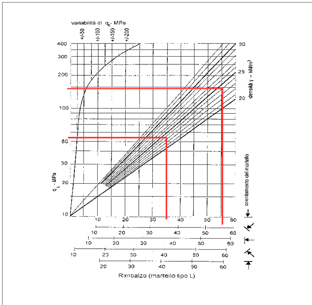
Fig. 78: Grafico di Miller.
