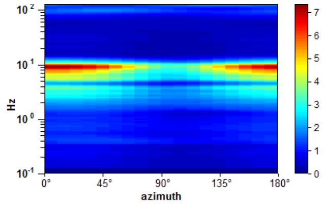
DIREZIONALITA' H/V
