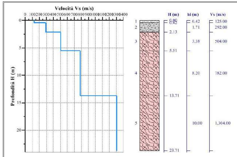
Fig. 30: Sismo-stratigrafia.
