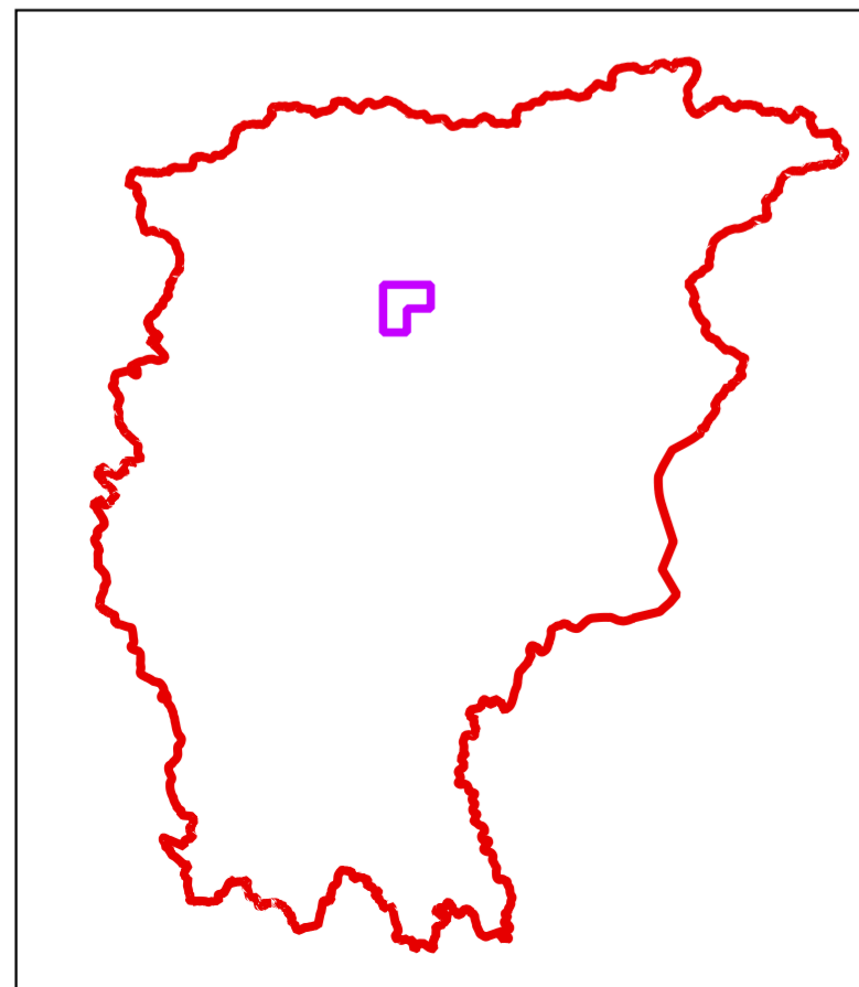
Ubicazione permesso di ricerca "Cime" nella Provincia di Bergamo
