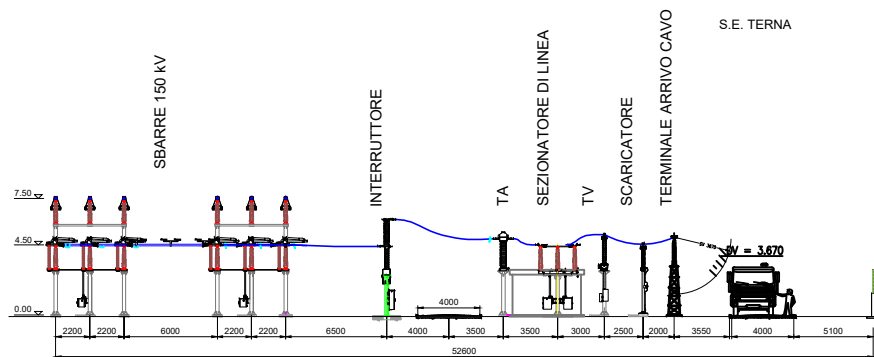
SEZIONE STALLO ARRIVO CAVO PRODUTTORE 150 KV
