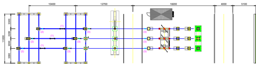
PIANTA STALLO ARRIVO CAVO PRODUTTORE 150 KV
