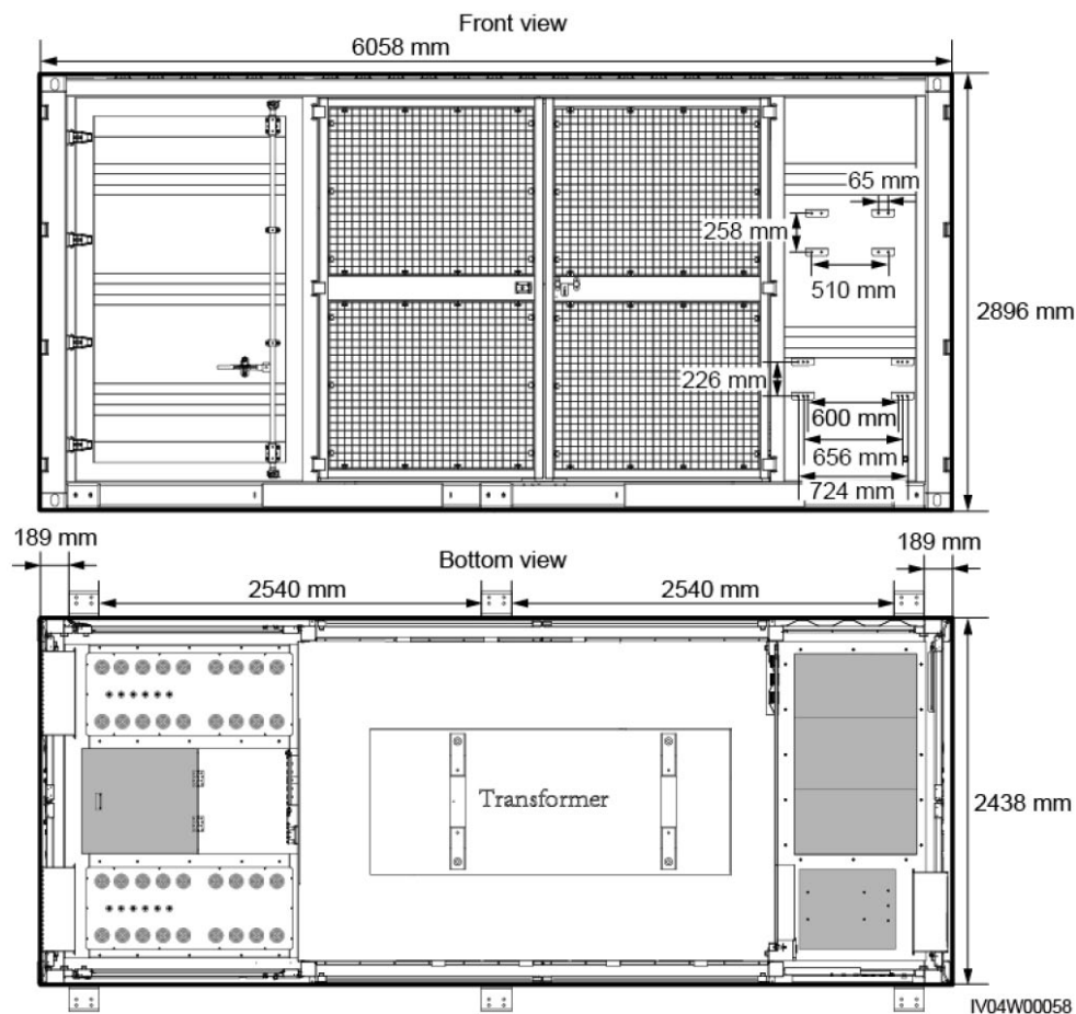
Figura 5 – dimensioni container
