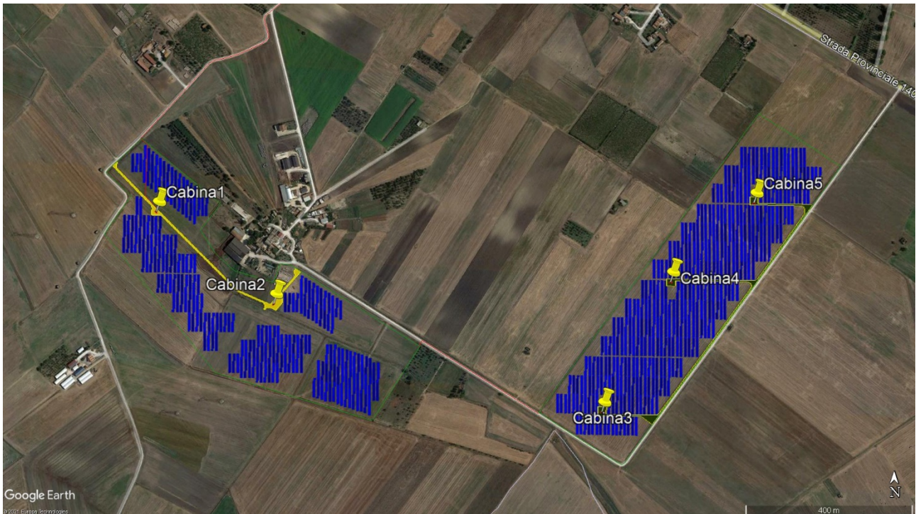
Figura 6 – Posizione cabine
