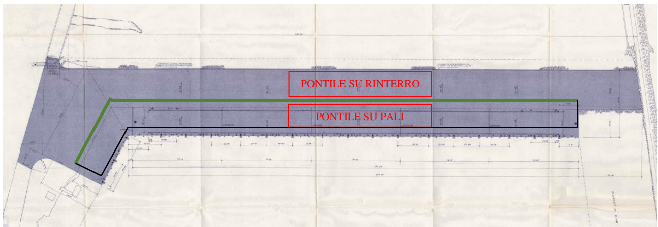
Figura 3-4: Pianta generale banchina – Giunto di dilatazione longitudinale
