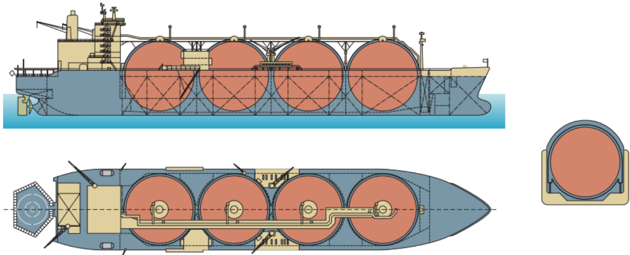
Figura 3-2: Metaniera con Serbatoi Autoportanti di Concezione Moss Rosenberg (Rojey et al.; 1994) 6
