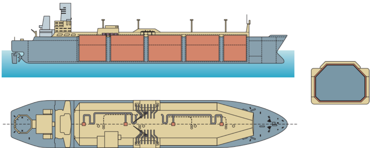
Figura 3-1: Metaniera con Serbatoio integrato con Sistema a Membrana (Rojey et al.; 1994)
