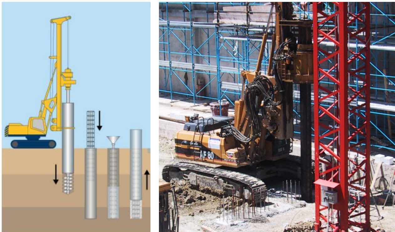
Figura 4-5: Realizzazione di pali trivellati: (a) schema esecutivo; (b) foto macchina
