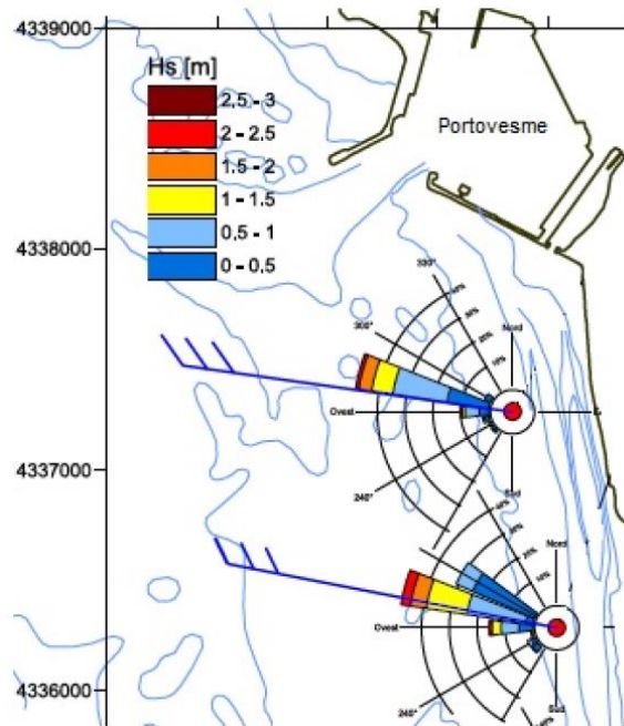
Figura 4-6: Clima Ondoso nei pressi dell'Imboccatura del Porto; Hs = Altezza d'Onda
