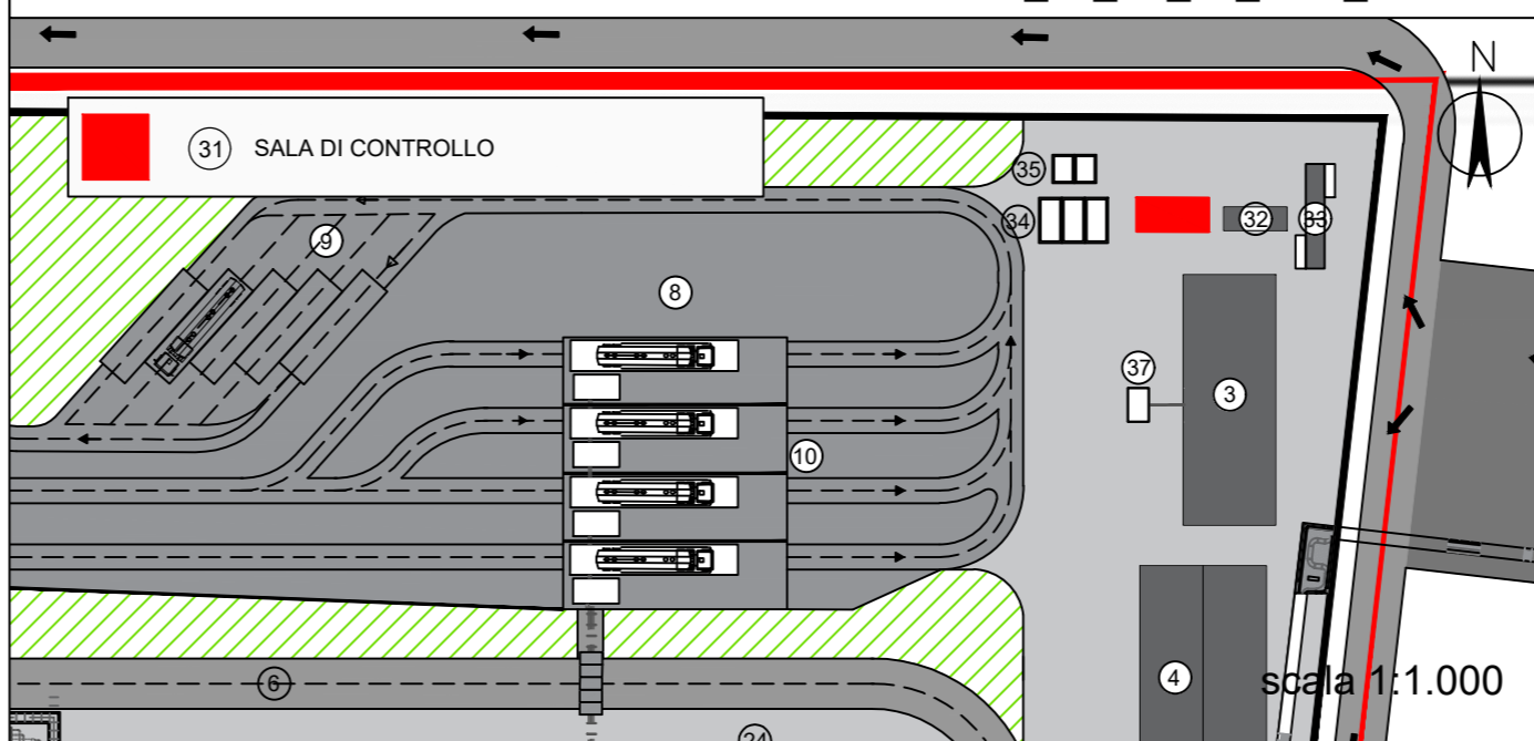
RIFERIMENTO LAYOUT: ELABORATO TECNICO P_03_PL_05_STO_R01
