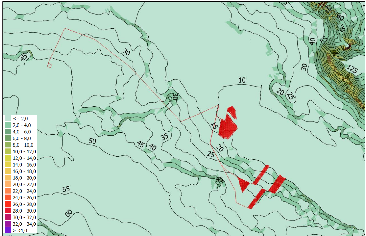
Figura 4: Carta delle pendenze (esprese in gradi) tratte dal modello di elevazione precedente.
