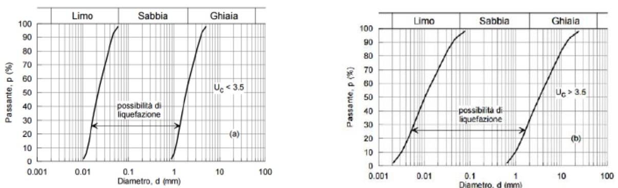
Figura 5 - Fusi granulometrici di terreni suscettibili di liquefazione ai sensi delle NTC
