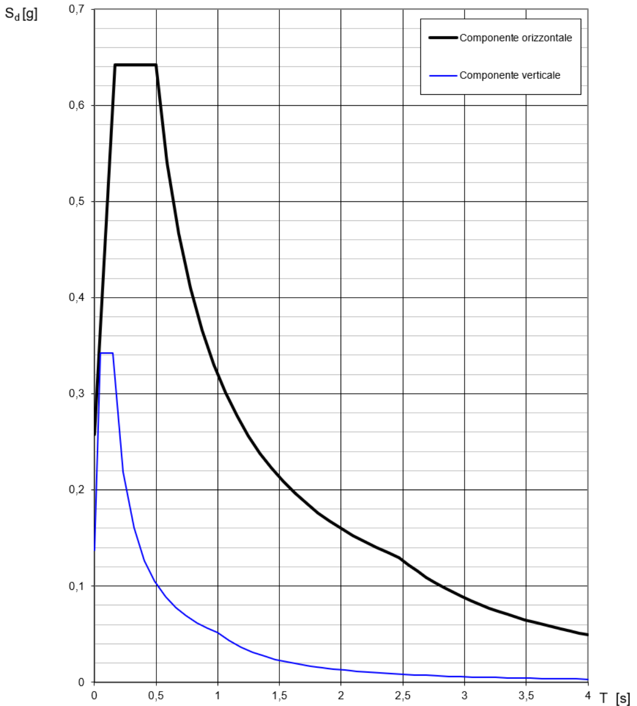
Figura 9: Spettro di risposta Stato limite SLV in forma grafica
