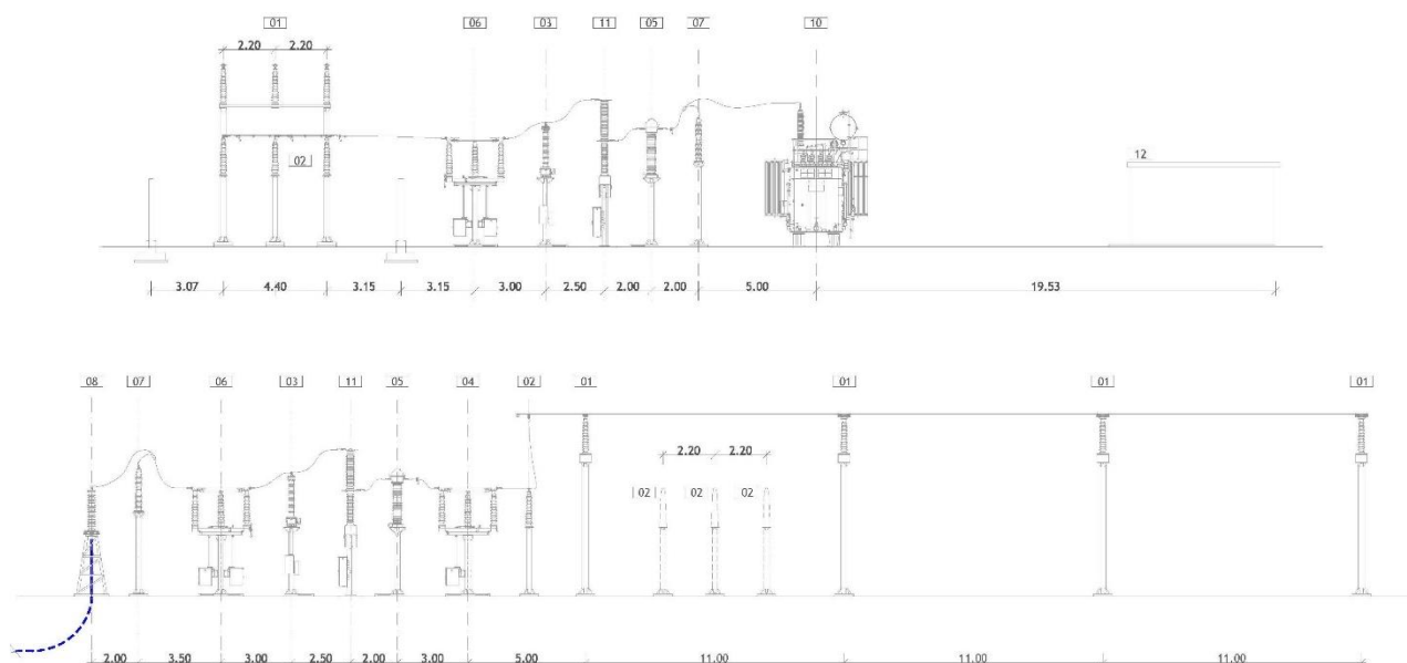
Sezioni Elettromeccaniche
