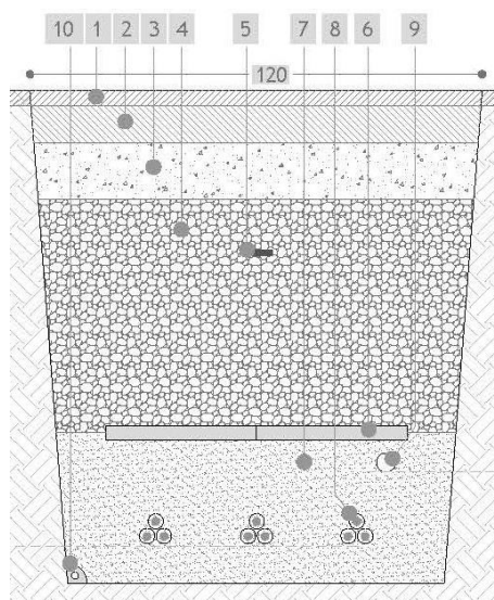
Figura 2: Sezione tipo cavidotto composta da tre terne da 630 mm 2
