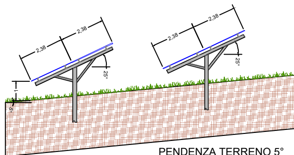
PENDENZA TERRENO 5°
