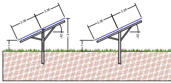
PENDENZA TERRENO 0°
