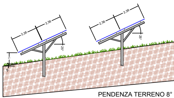
PENDENZA TERRENO 8°
