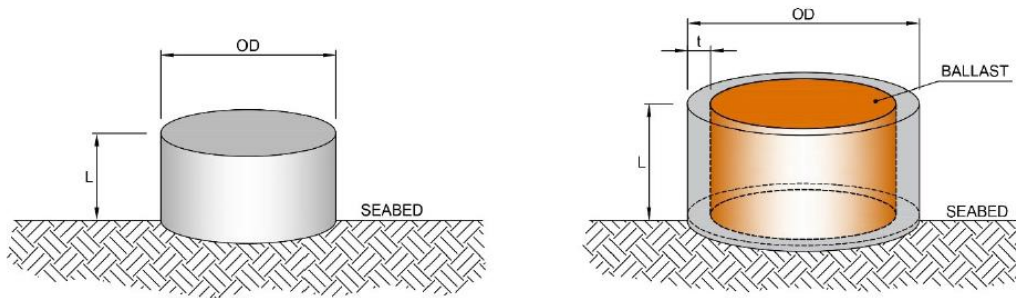
Figura 6 Schema Semplificato di Ancore a Gravità Piene (Sinistra) o Cave con Zavorra (Destra)
