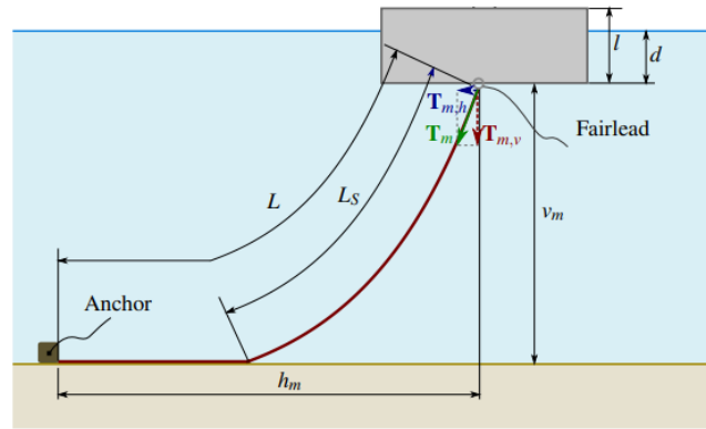
Figura 4 Catenaria
