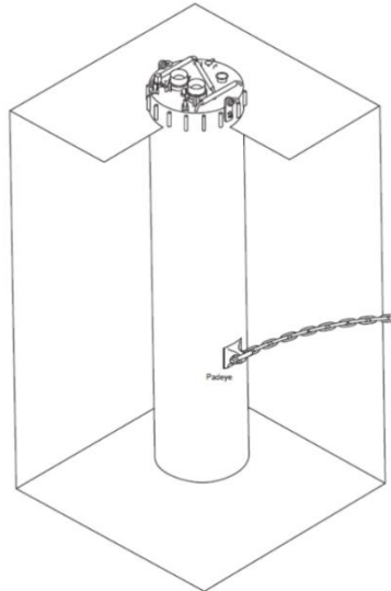
Figura 7 Tipica Connessione tra 'Suction Pile' e Linea di Ormeggio a Catenaria [8]
