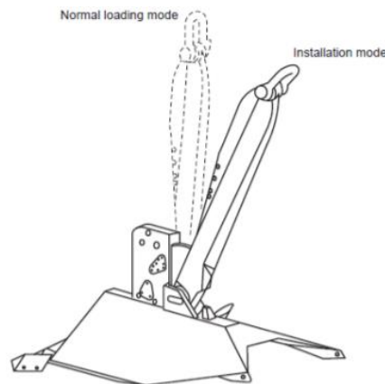
Figura 12 Variazione Angolo 'Shank-Fluke' Installazione/Esercizio per Ancora Bruce Dennla VLA [5]
