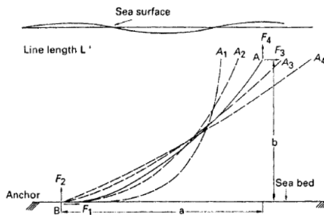
Figura 3 Sistema di Ormeggio con Catenaria [1]
