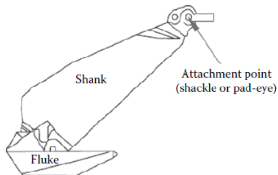
Figura 9 Geometria Tipica di una DEA [24]
