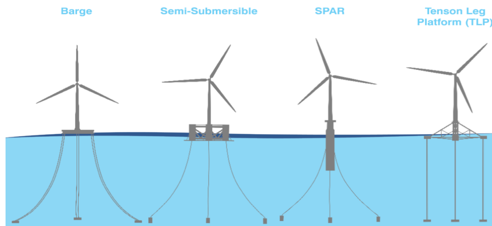
Figura 2 Esempi di Strutture Galleggianti per Parchi Eolici
