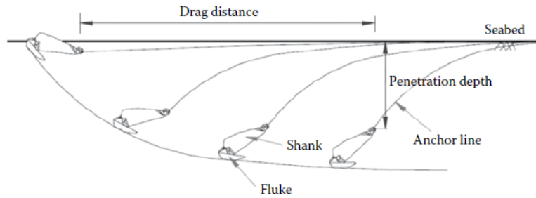
Figura 10 Schema di Installazione di Ancore a Trascinamento DEA [24]
