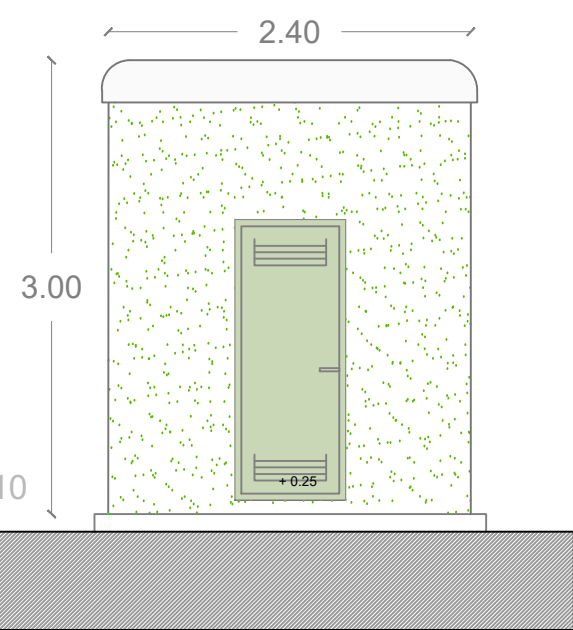
VISTA FRONTALE
