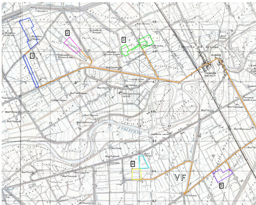
Figura 1: Lay-out impianto su CTR
