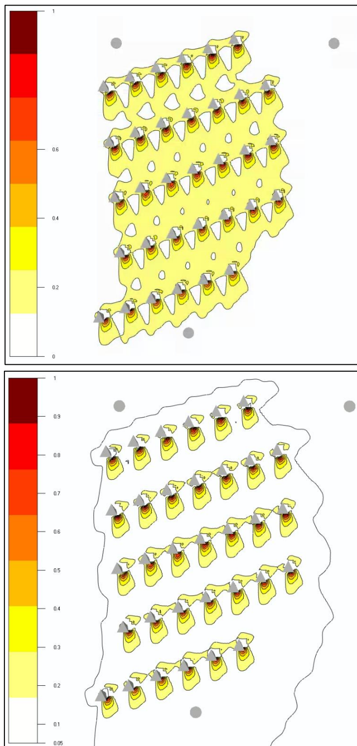
Figura 9.3 – Perdite di scia (wake model 2)
