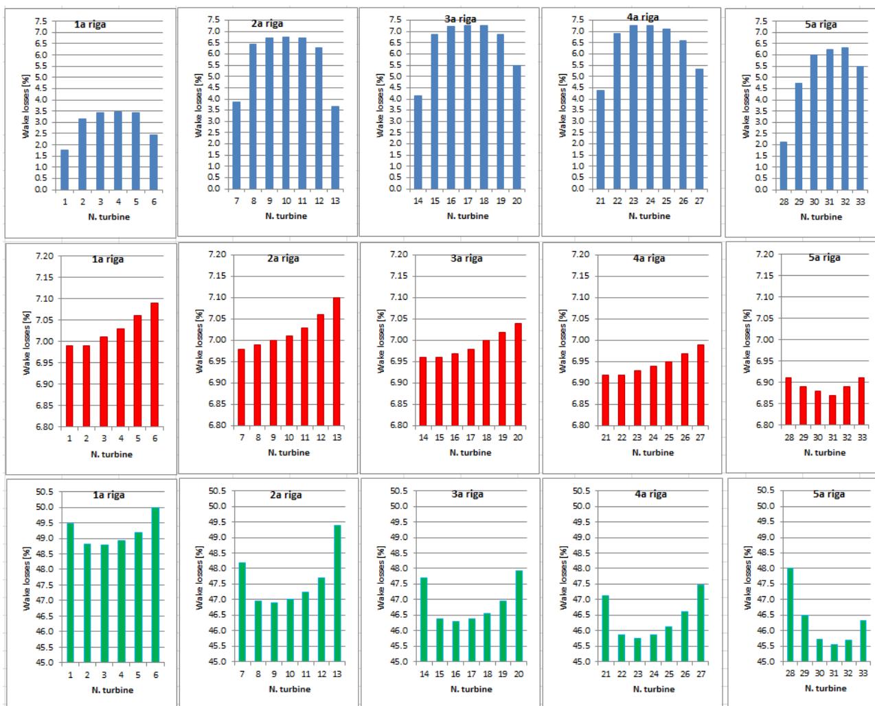
Figura 10.1 – Riassunto delle perdite, velocità media al mozzo e AEP per ogni fila del layout
