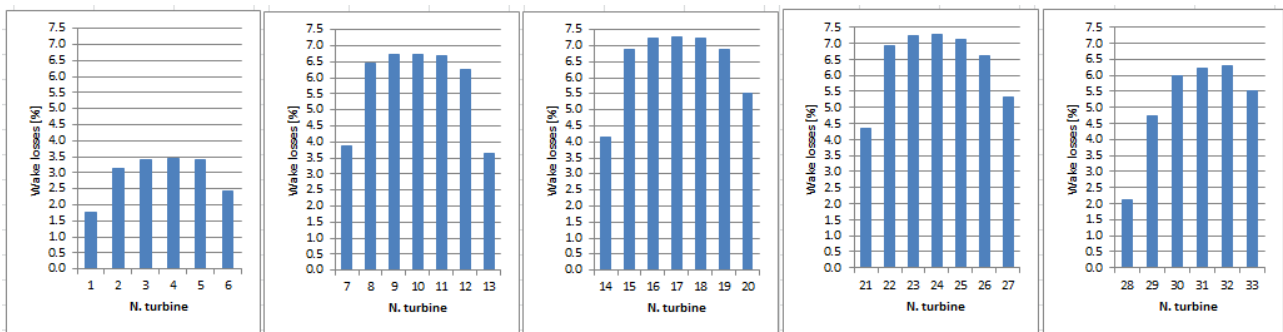
Figura 9.2 – Perdite di scia delle turbine divise in file in base al layout
