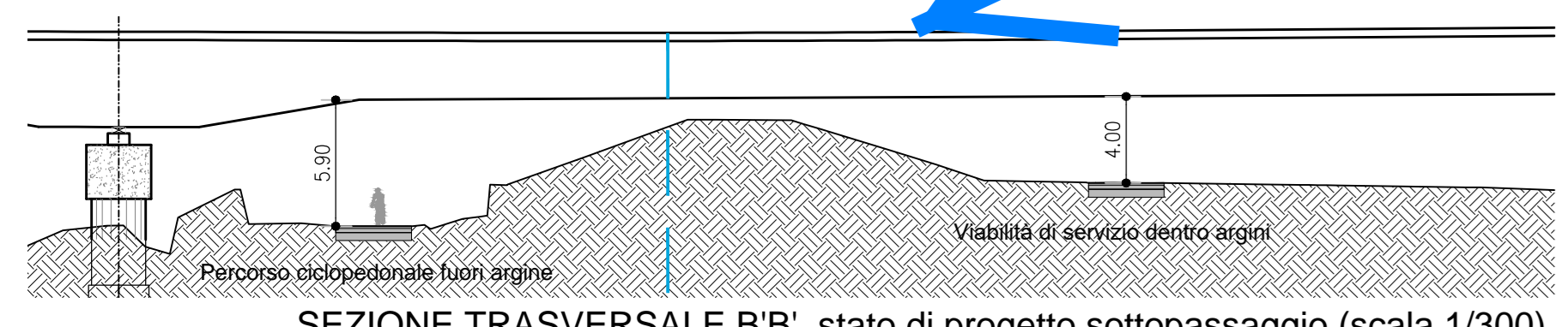
SEZIONE TRASVERSALE BB', stato di progetto sottopassaggio (scala 1/300)
