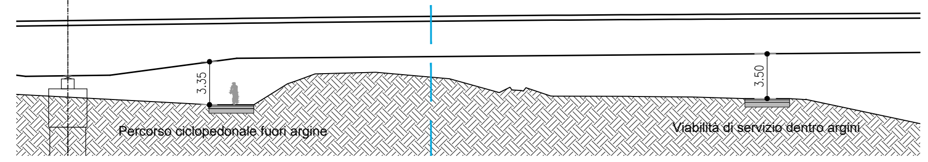
SEZIONE TRASVERSALE AA', stato di progetto sottopassaggio (scala 1/300)
