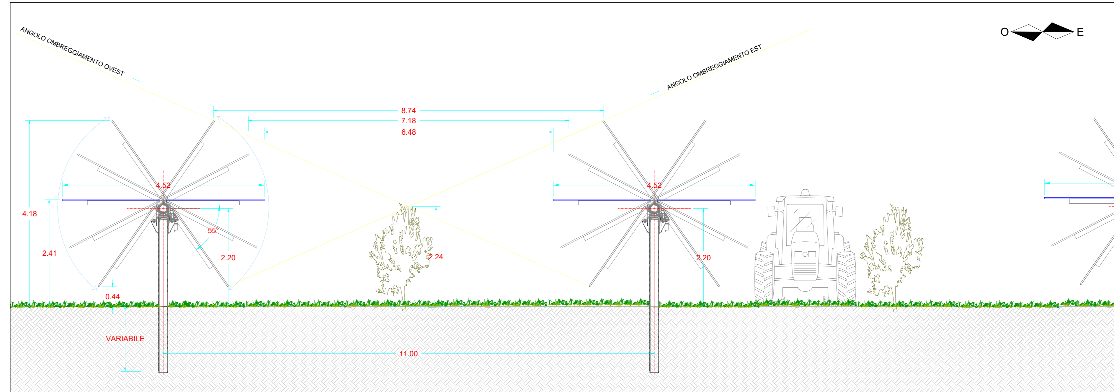
DETTAGLIO SEZIONE TRASVERSALE STRUTTURA - SCALA 1:50
