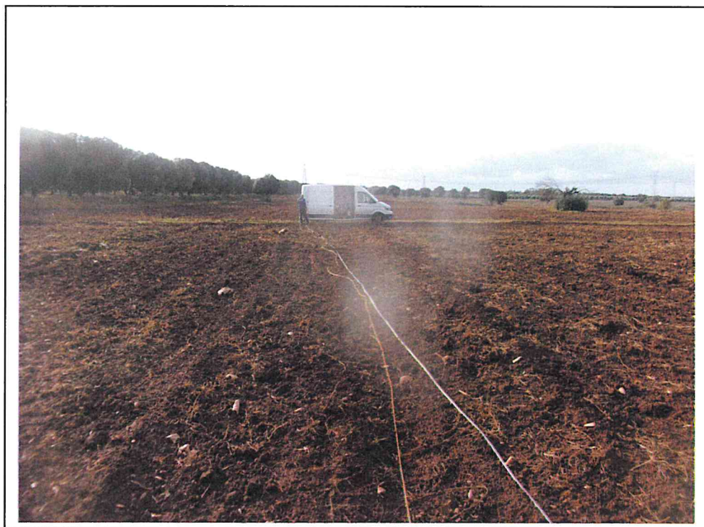
Esecuzione profilo sismico a rifrazione n. 1
