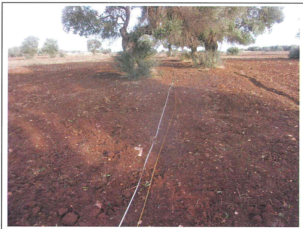
Esecuzione profilo sismico a rifrazione n. 2 e ReMi sullo stesso stendimento
