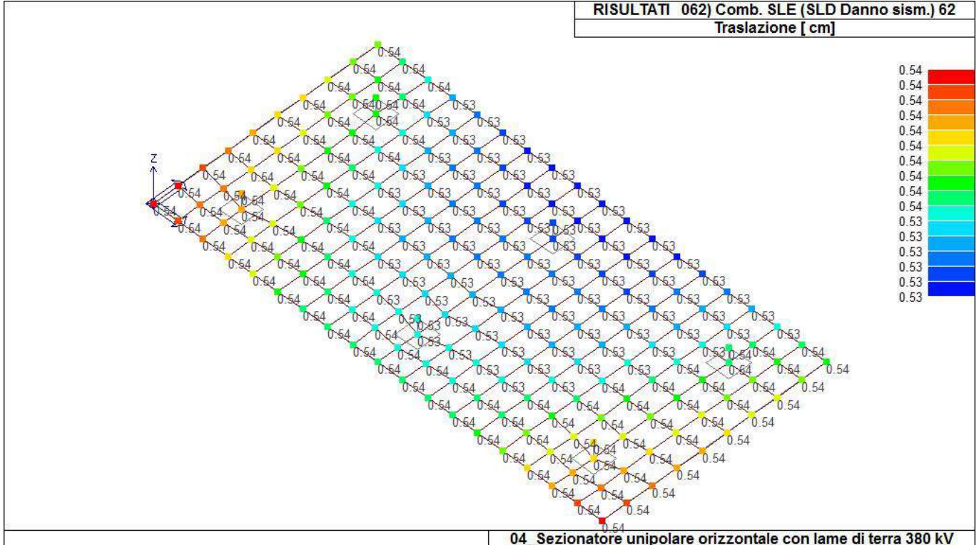
41_RIS_SPOSTAMENTI_062_Comb. SLE (SLD Danno sism.) 62
