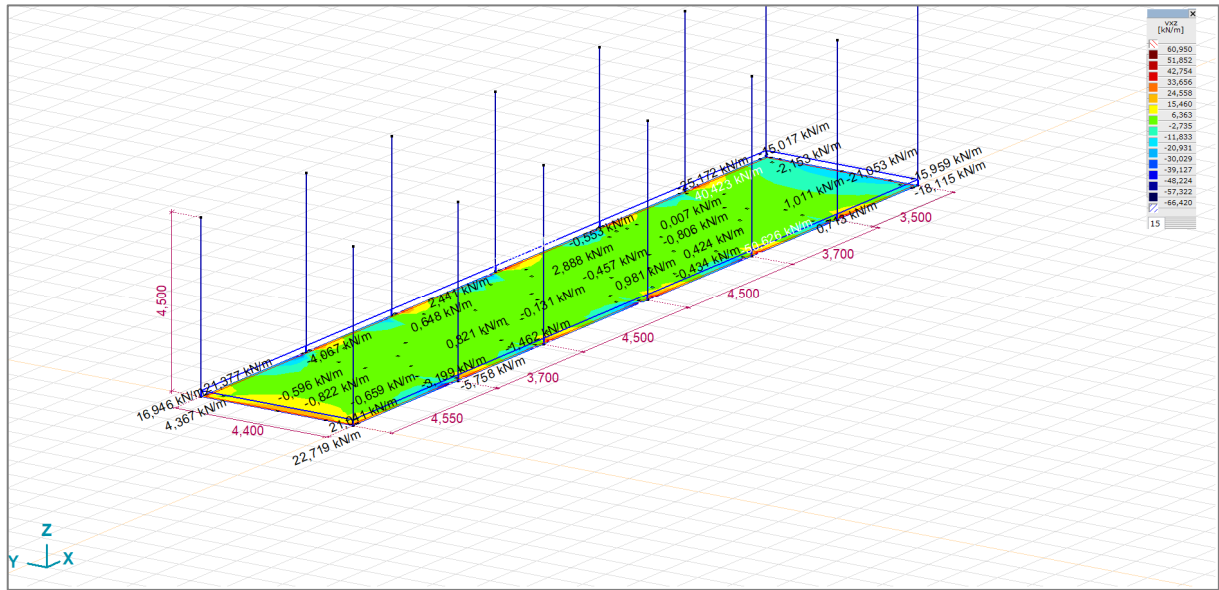
FIGURA 14 v_{xz} , SOLLECITAZIONI TAGLIANTI ISOSUPERFICI 2D
