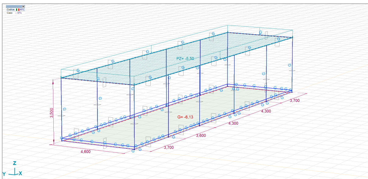
FIGURA 23_VISUALIZZAZIONE CARICHI STATICI SU STRUTTURA
