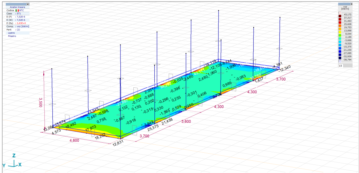
FIGURA 33 vxz, SOLLECITAZIONI TAGLIANTI ISOSUPERFICI 2D
