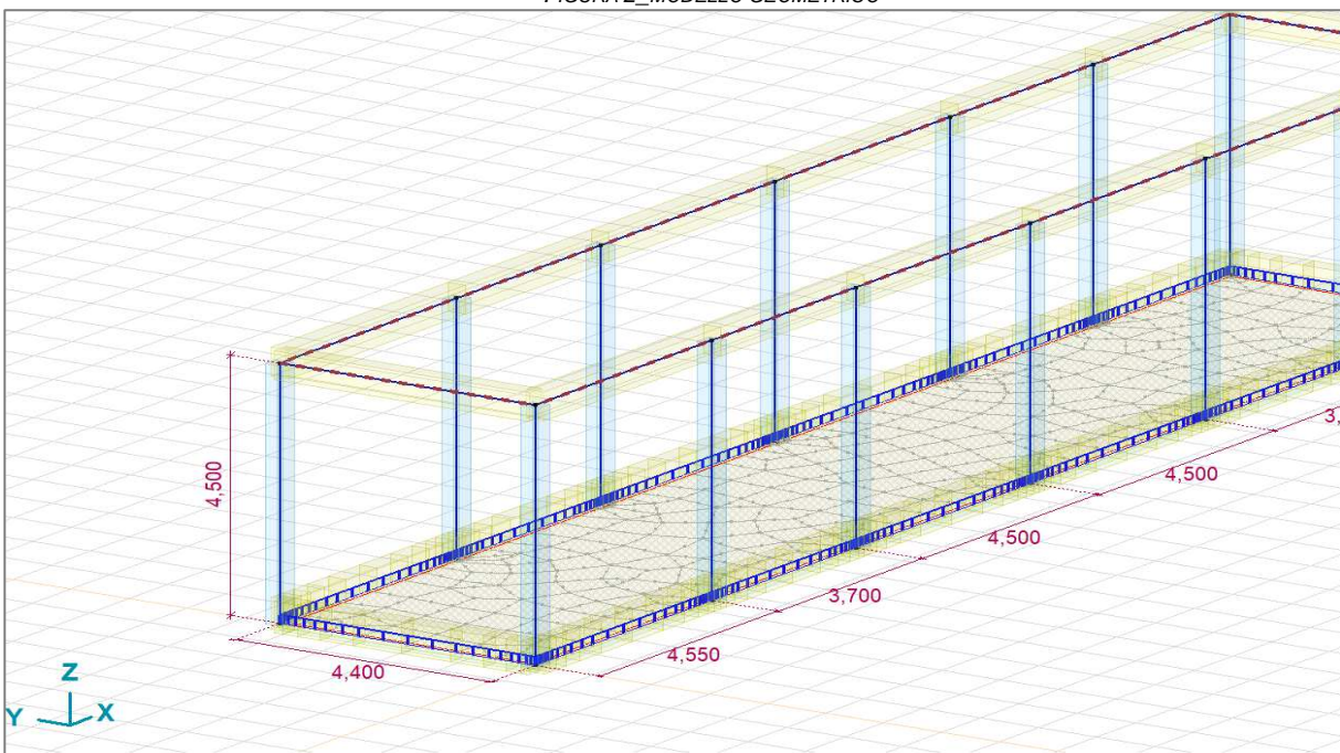
FIGURA 3_MODELLO CON MESHATURA PIASTRA
