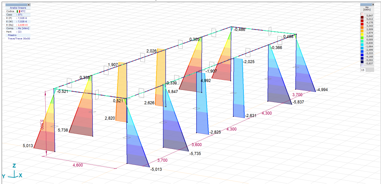
FIGURA 26 Mz, DIAGRAMMA DEI MOMENTI FLETTENTI
