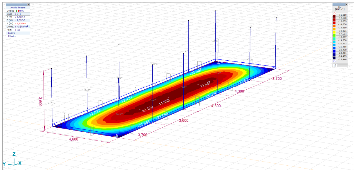
FIGURA 39 EZ, ISOLINEE CEDIMENTI – MAX 3MM
