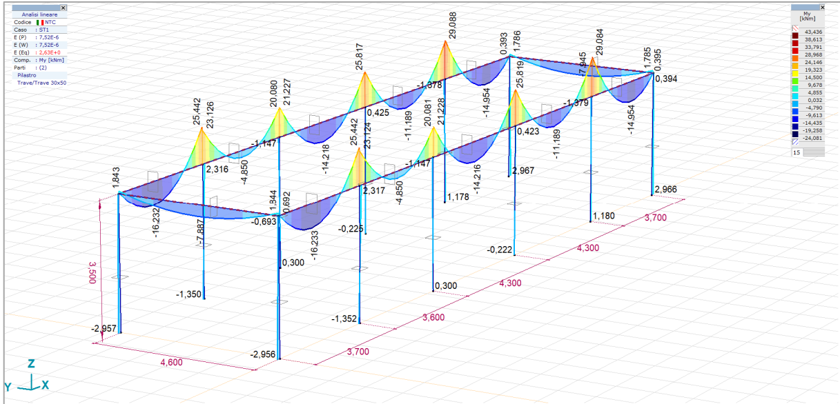
FIGURA 25 My, DIAGRAMMA DEI MOMENTI FLETTENTI
