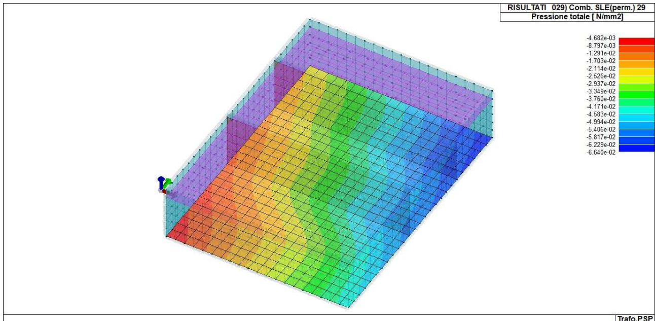
FIGURA 40_ANDAMENTO DEI CARICHI AL SUOLO
