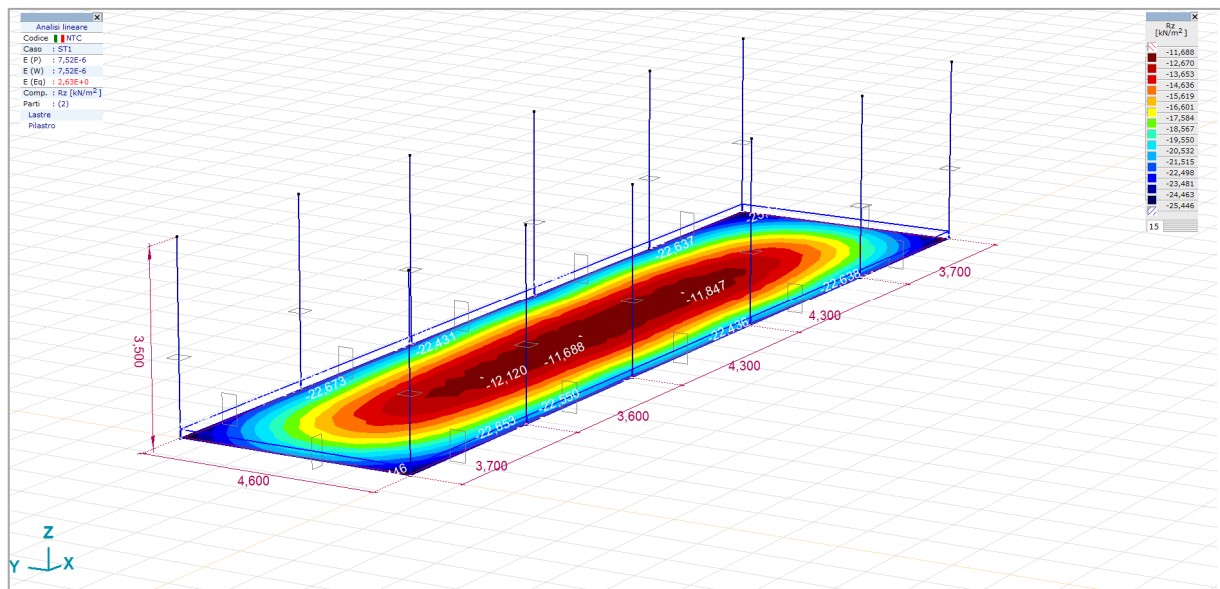
FIGURA 37_ANDAMENTO DEI CARICHI AL SUOLO
