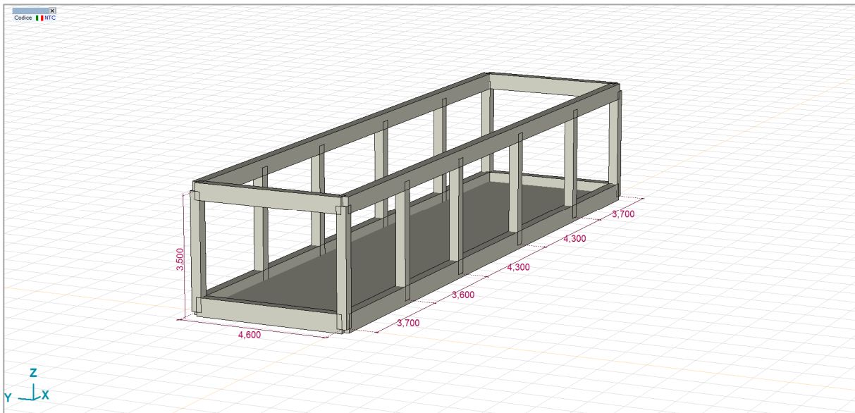
FIGURA 21_MODELLO GEOMETRICO – VISTA SOLIDA
