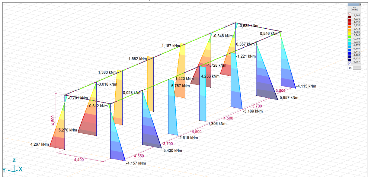
FIGURA 6 My, DIAGRAMMA DEI MOMENTI FLETTENTI
