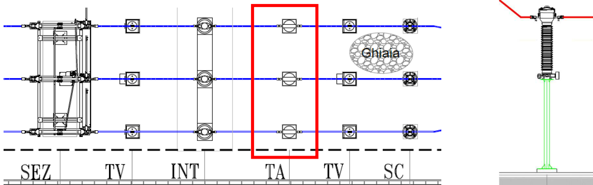
Figura 46_Tipico trasformatore di corrente – vista prospettica e planimetrica
