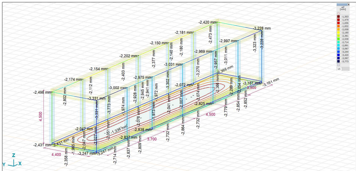
FIGURA 20 eZ, ISOLINEE CEDIMENTI – MAX 3-4MM
