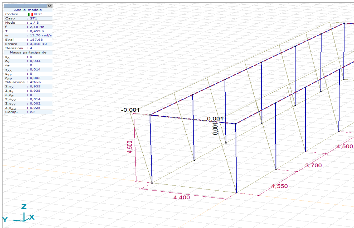
FIGURA 5_FORMA MODALE 1°MODO DI VIBRARE
