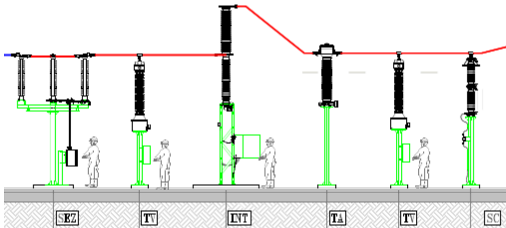
Figura 41_vista sezione elettromeccanica Apparecchiature AT
