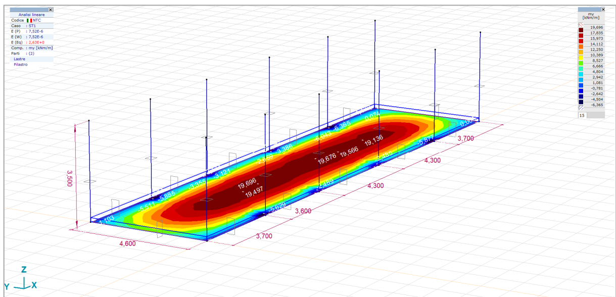
FIGURA 32 m_y , sollecitazioni flessionali Isosuperfici 2D
