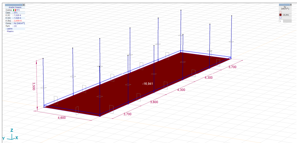
FIGURA 38_ANDAMENTO DEI CARICHI AL SUOLO_VALORE MEDIO
