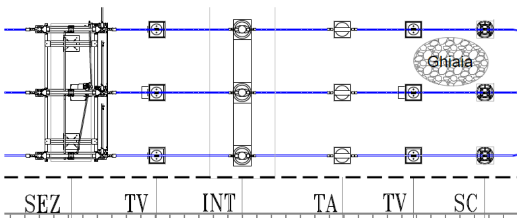
Figura 42_planimetria elettromeccanica apparecchiature AT
