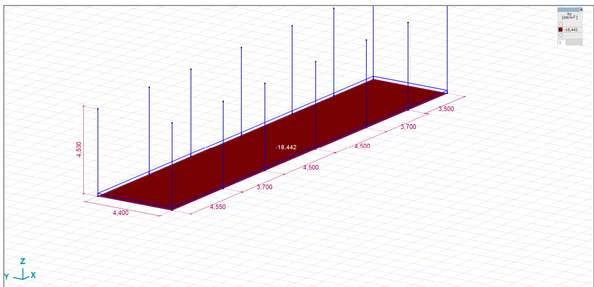
FIGURA 19_ANDAMENTO DEI CARICHI AL SUOLO_VALORE MEDIO
