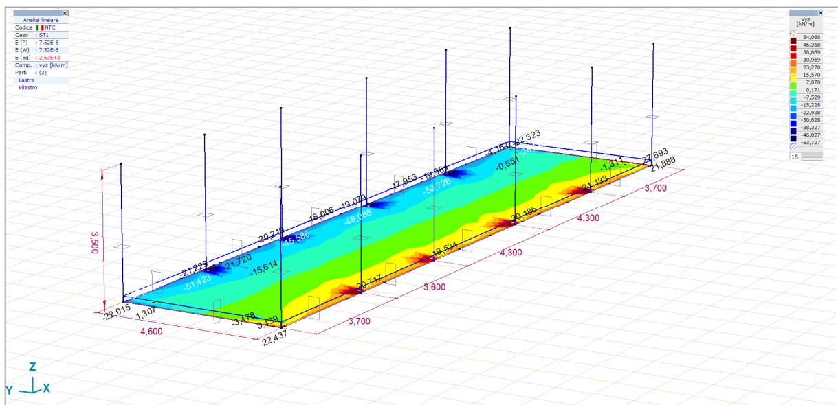
FIGURA 34 vyz, SOLLECITAZIONI TAGLIANTI ISOSUPERFICI 2D
