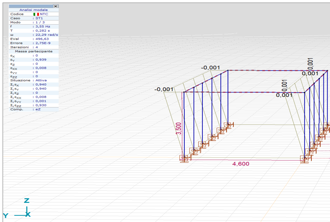
FIGURA 24_FORMA MODALE 1°MODO DI VIBRARE
