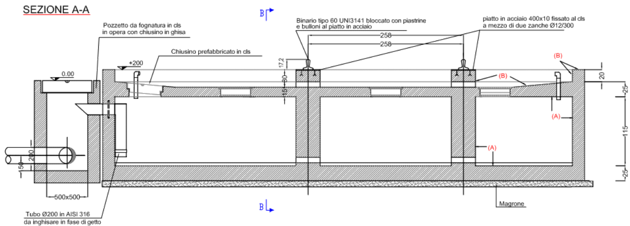
Sezione fondazione
