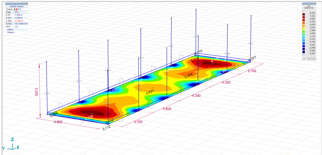
FIGURA 31 m_x , sollecitazioni flessionali Isosuperfici 2D
