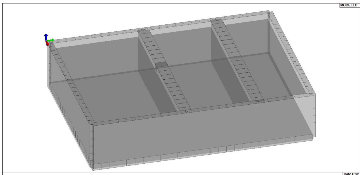
Modello FEM (senza soletta di copertura) – Vista 3D
