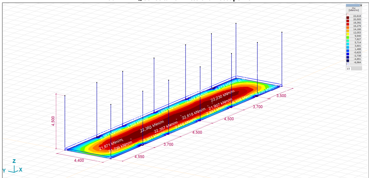
FIGURA 13 m_y , sollecitazioni flessionali Isosuperfici 2D
