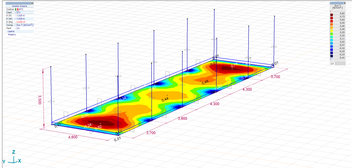
FIGURA 29 Sxx TENSIONI ELEMENTI BIDIMENSIONALI ISOSUPERFICI 2D
