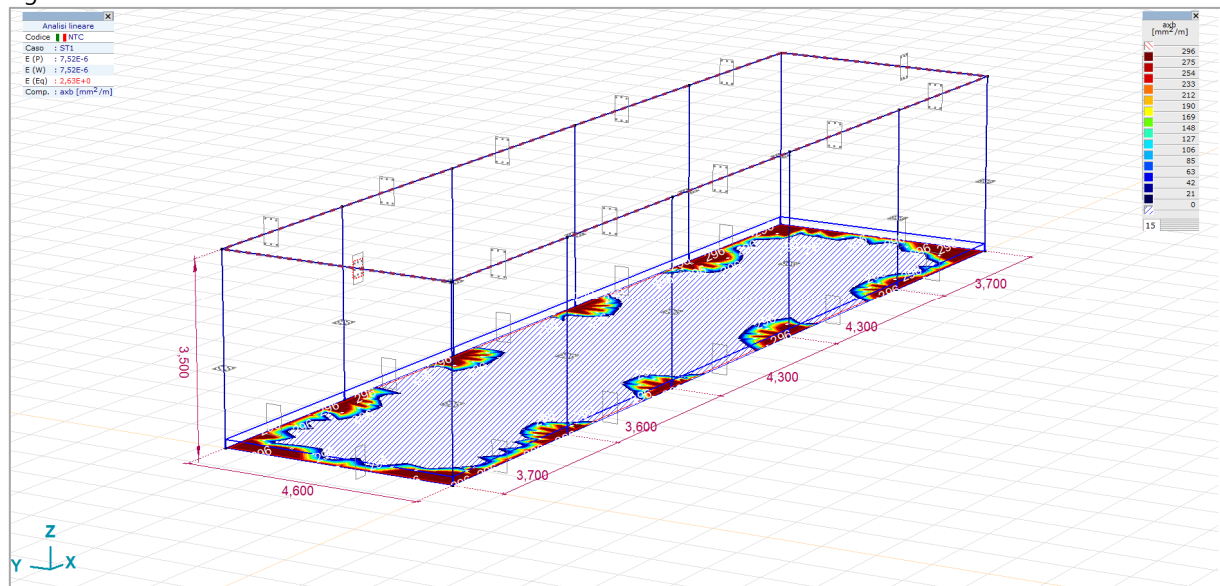
FIGURA 35 ARMATURA MINIMA X
