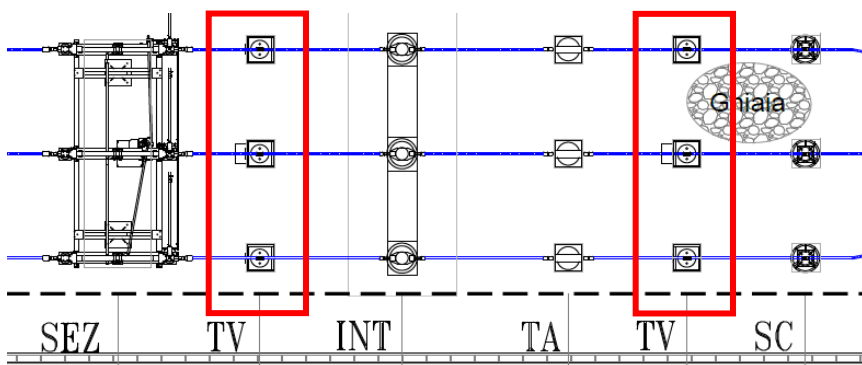
Figura 45_Tipico Trasformatore di tensione – vista prospettica e planimetrica
