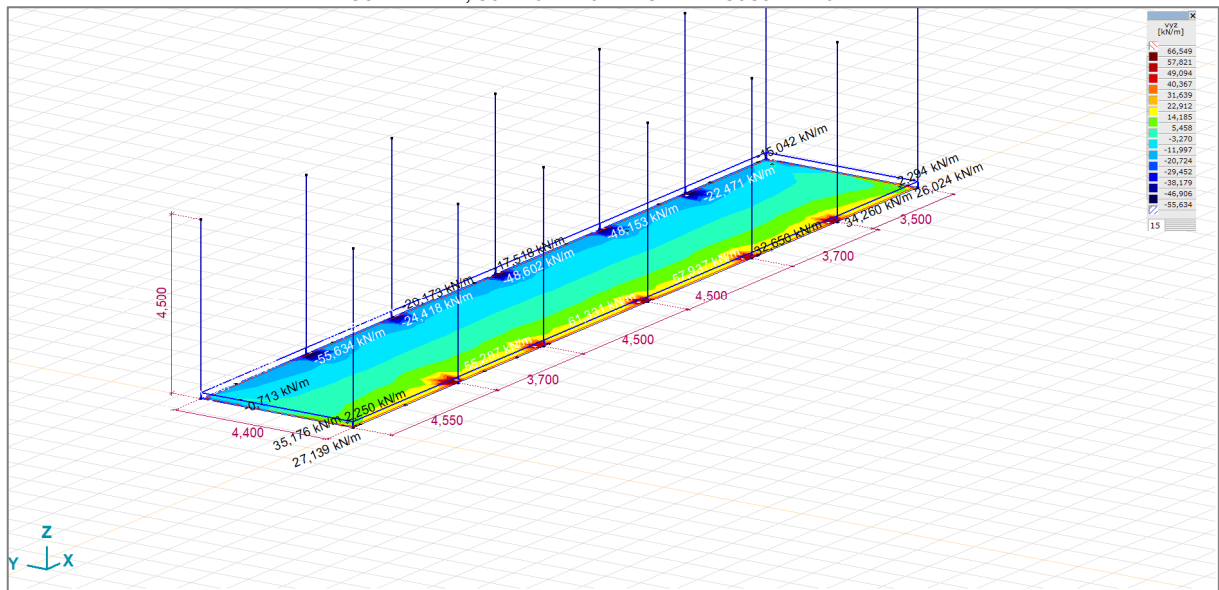
FIGURA 15 v_{yz} , SOLLECITAZIONI TAGLIANTI ISOSUPERFICI 2D
