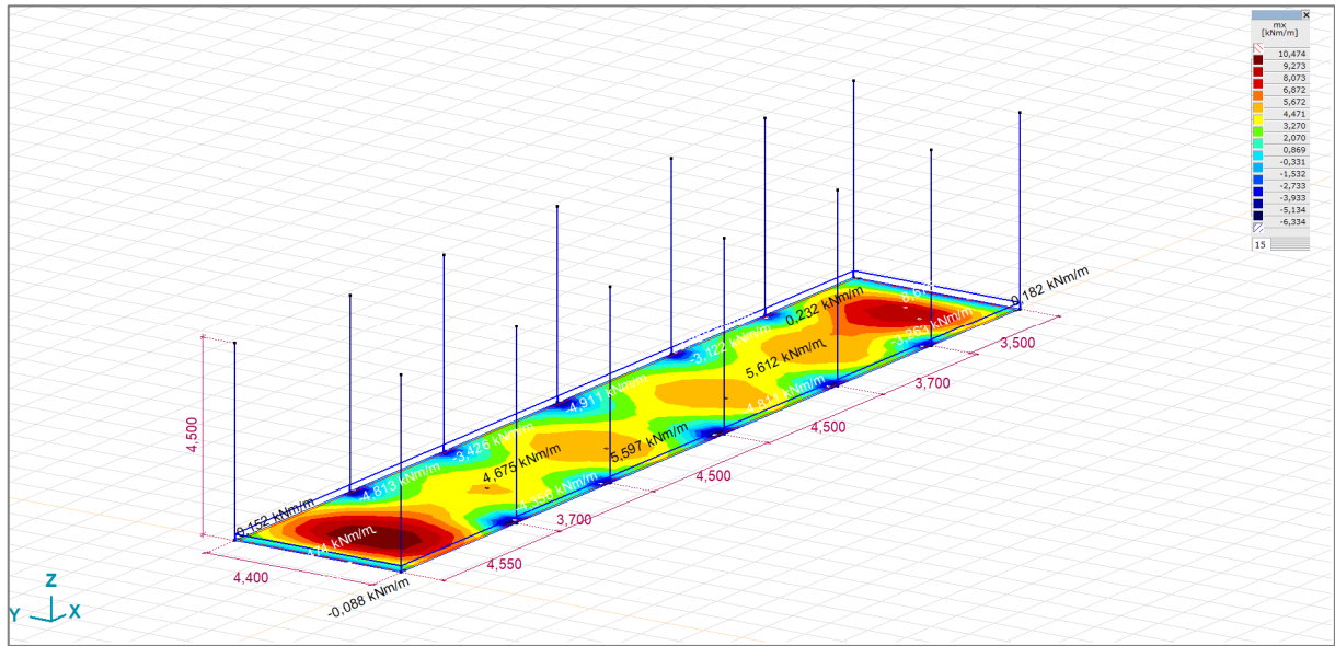
FIGURA 12 m_x , sollecitazioni flessionali Isosuperfici 2D
