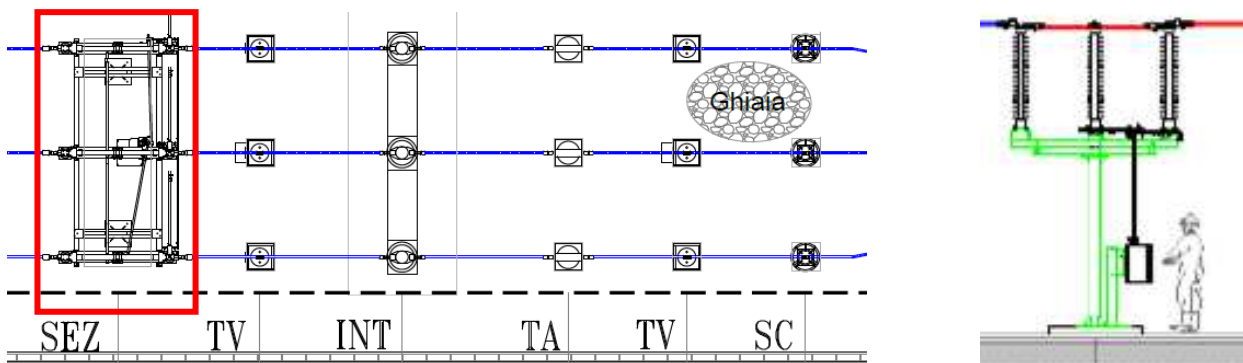
Figura 43_Tipico sezionatore tripolare – vista prospettica e planimetrica
