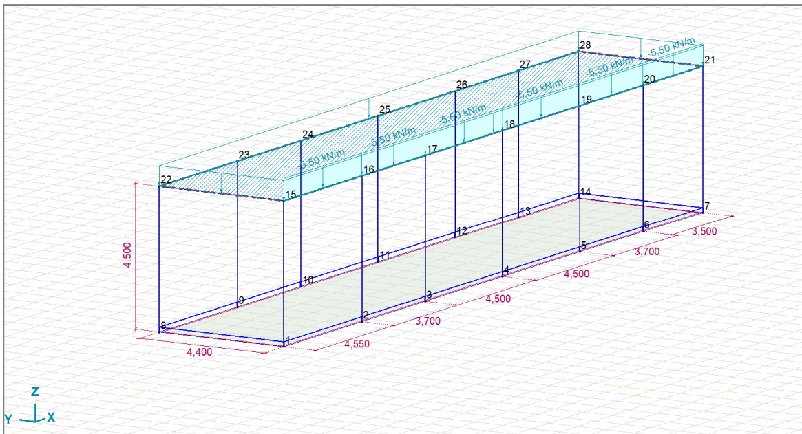
FIGURA 4 _VISUALIZZAZIONE CARICHI STATICI SU STRUTTURA
