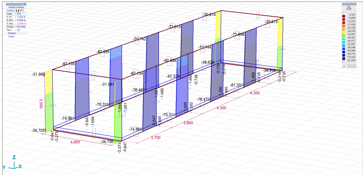
FIGURA 27 N, DIAGRAMMA SFORZI NORMALI
