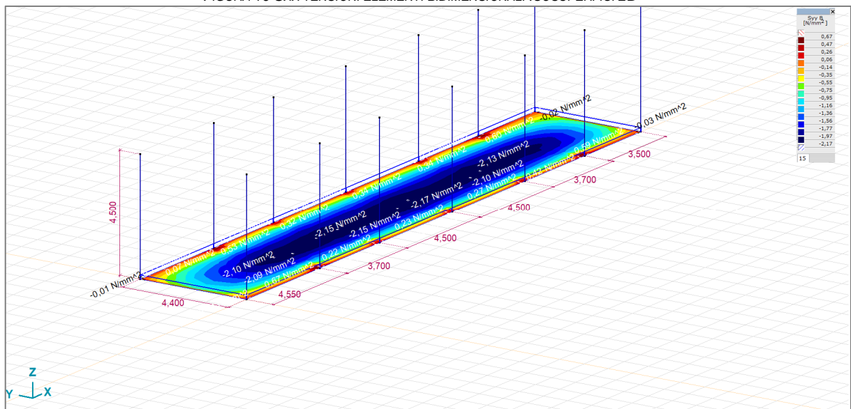
FIGURA 10 S_{xx} TENSIONI ELEMENTI BIDIMENSIONALI ISOSUPERFICI 2D
