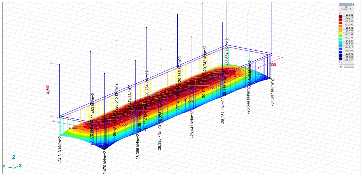
FIGURA 18_ANDAMENTO DEI CARICHI AL SUOLO
