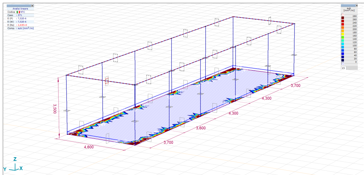
FIGURA 36 ARMATURA MINIMA Y
