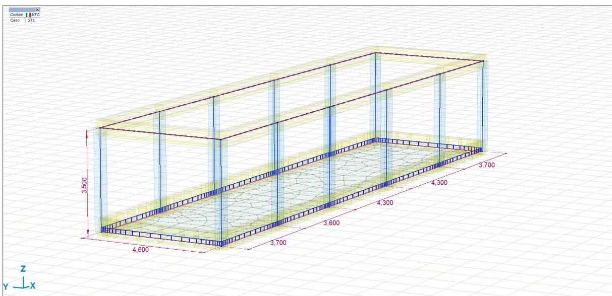
FIGURA 22_MODELLO CON MESHATURA PIASTRA
