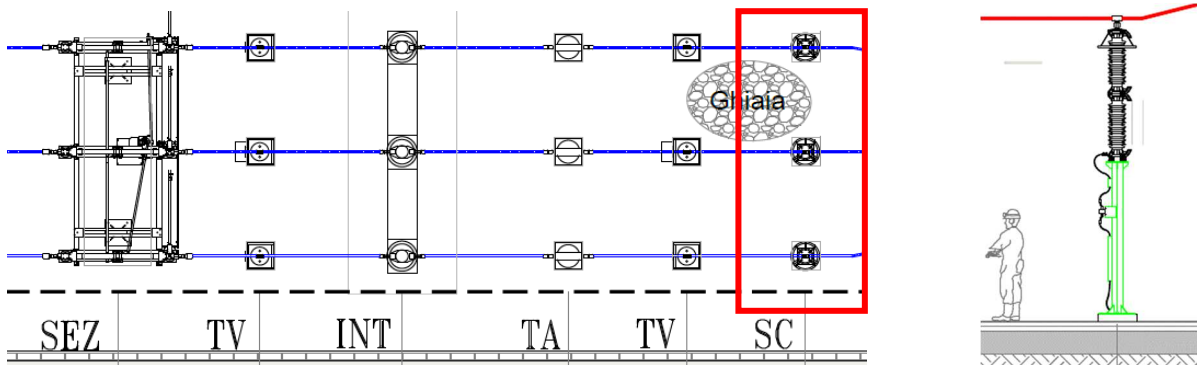
Figura 47_Tipico scaricatore di sovratensione – vista prospettica e planimetrica
