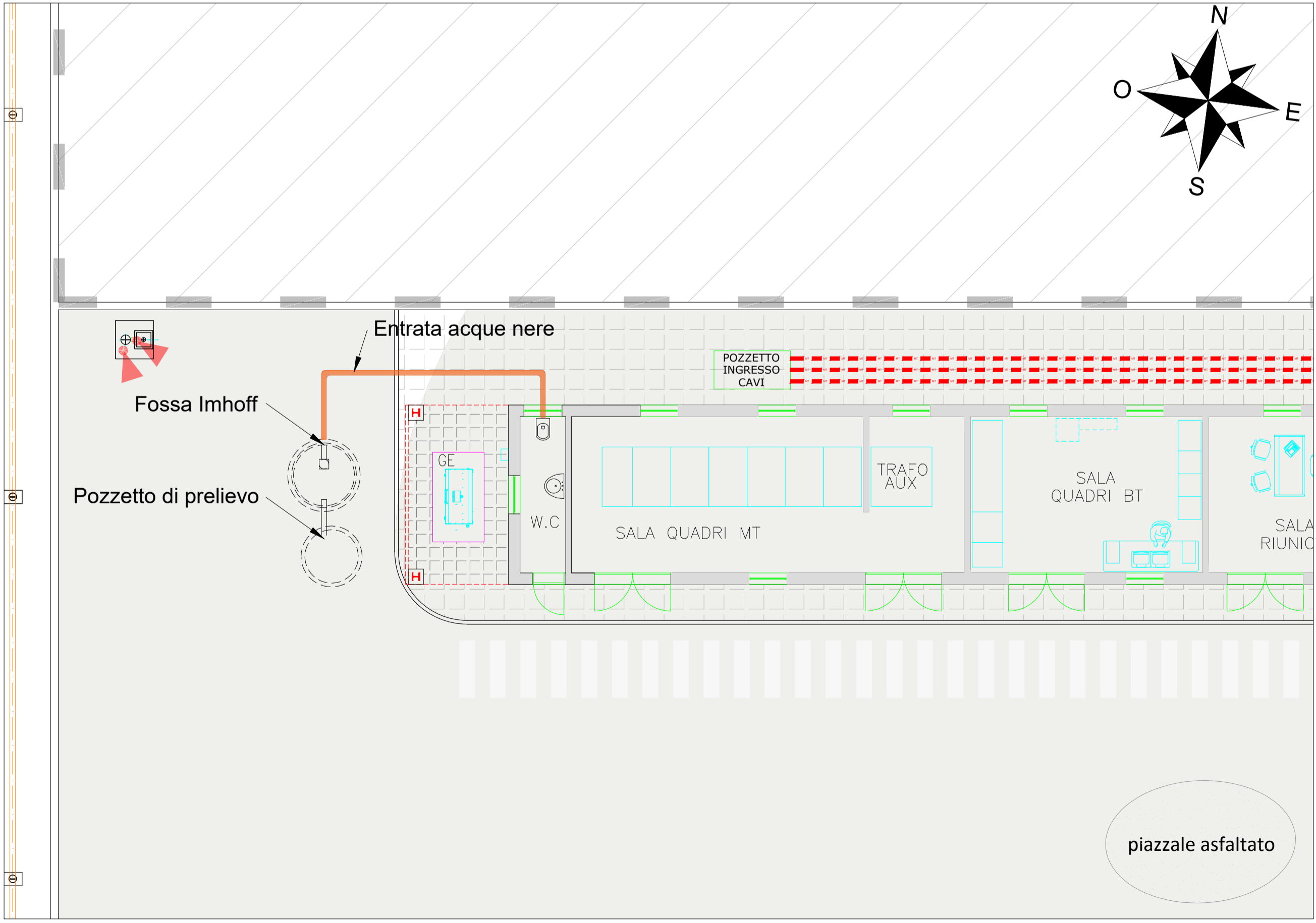
LAYOUT STAZIONE UTENTE DETTAGLIO POZZO IMHOFF - SCALA 1:100
