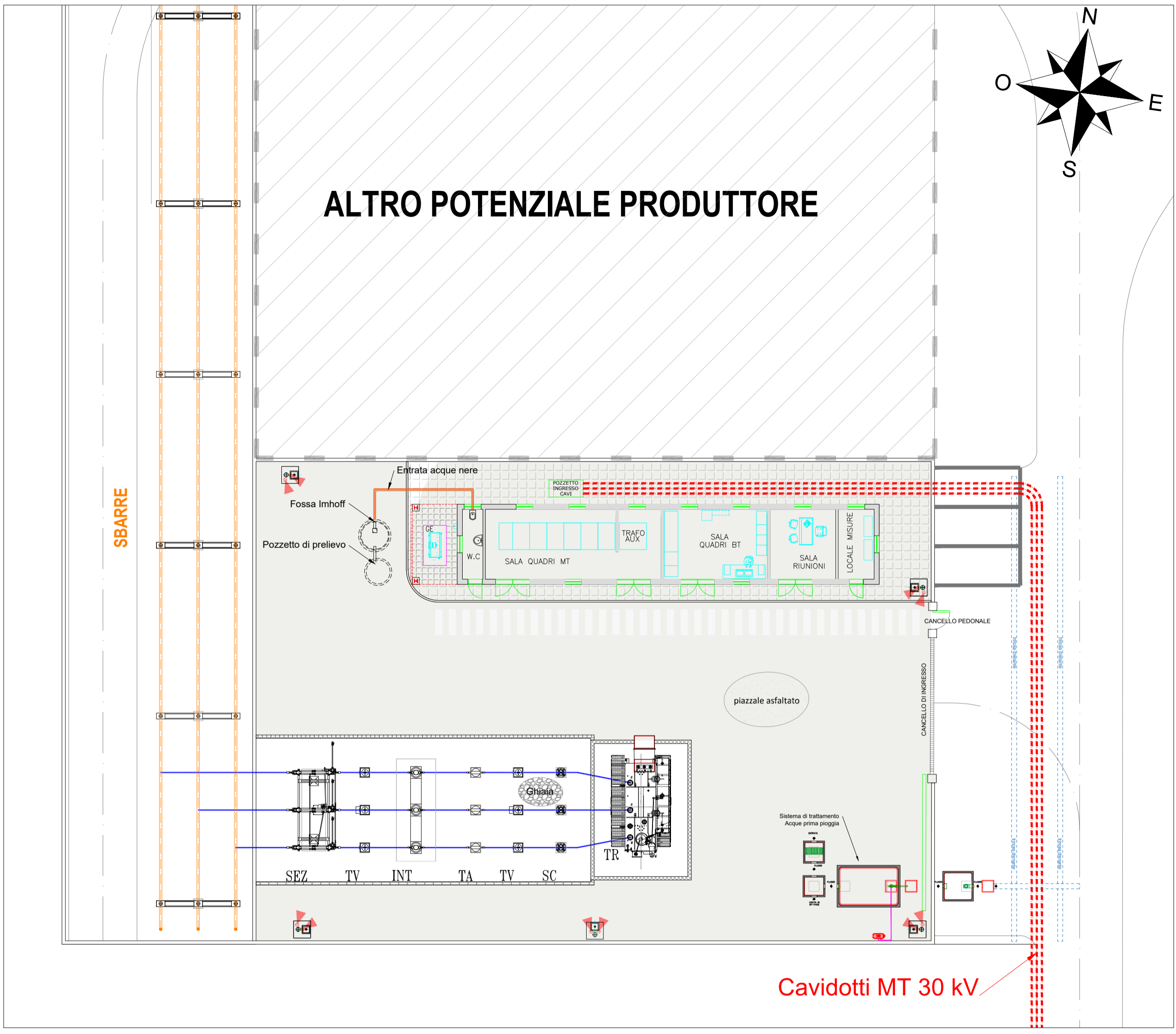
LAYOUT STAZIONE UTENTE DETTAGLIO POZZO IMHOFF - SCALA 1:100
