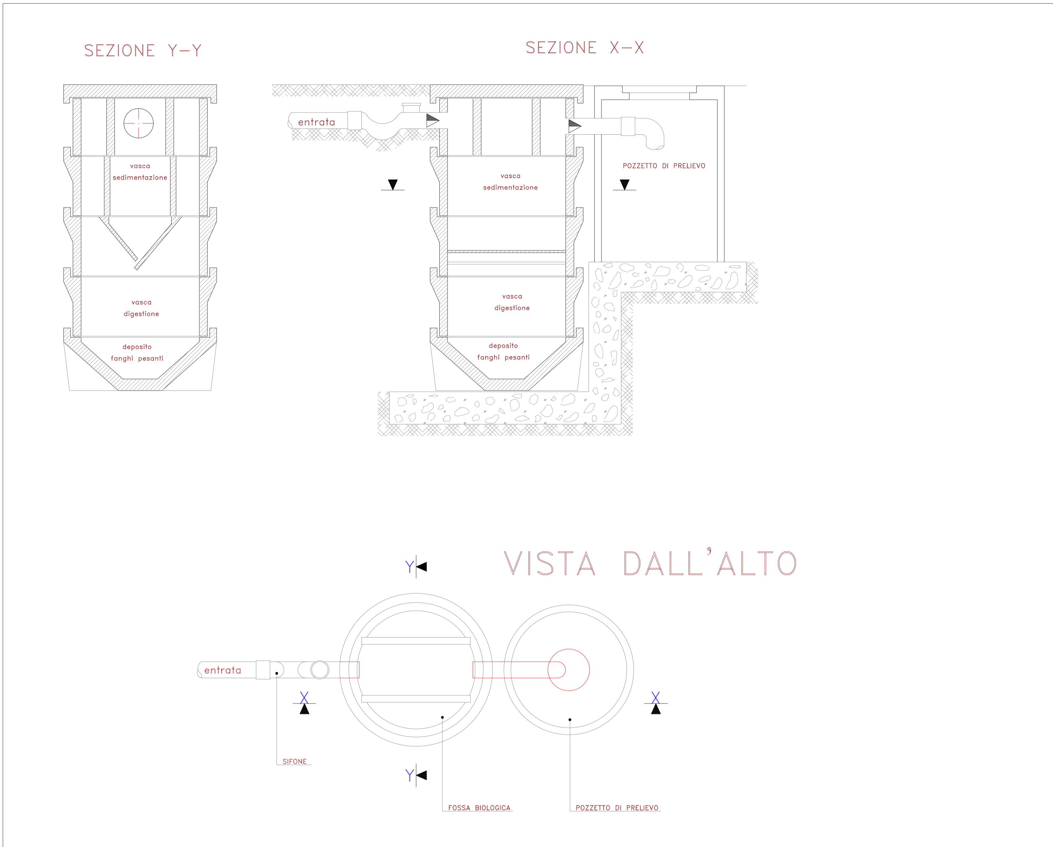
LAYOUT STAZIONE UTENTE DETTAGLIO POZZO IMHOFF - SCALA 1:100
