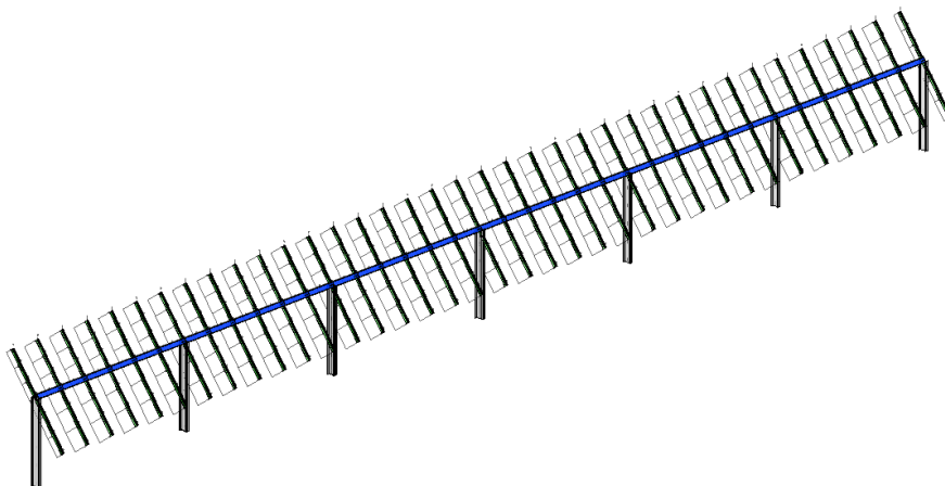
Vista assonometrica modello strutturale
