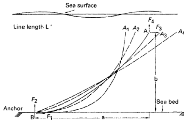
Figura 3 Sistema di Ormeggio con Catenaria [1]
