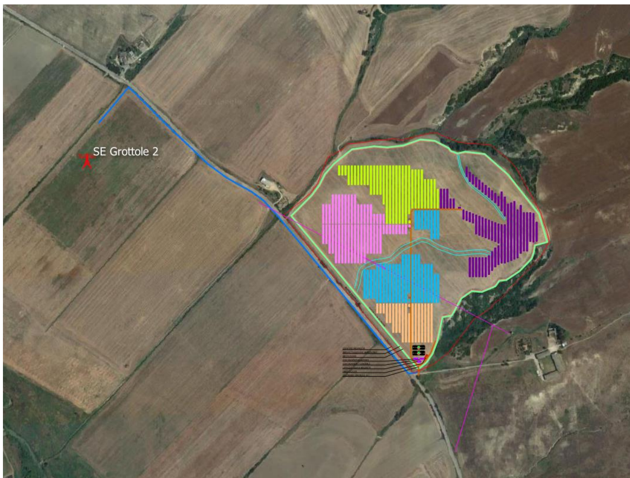
Figura 1 – Inquadramento dell'impianto FV ed opere di connessione su ortofoto
