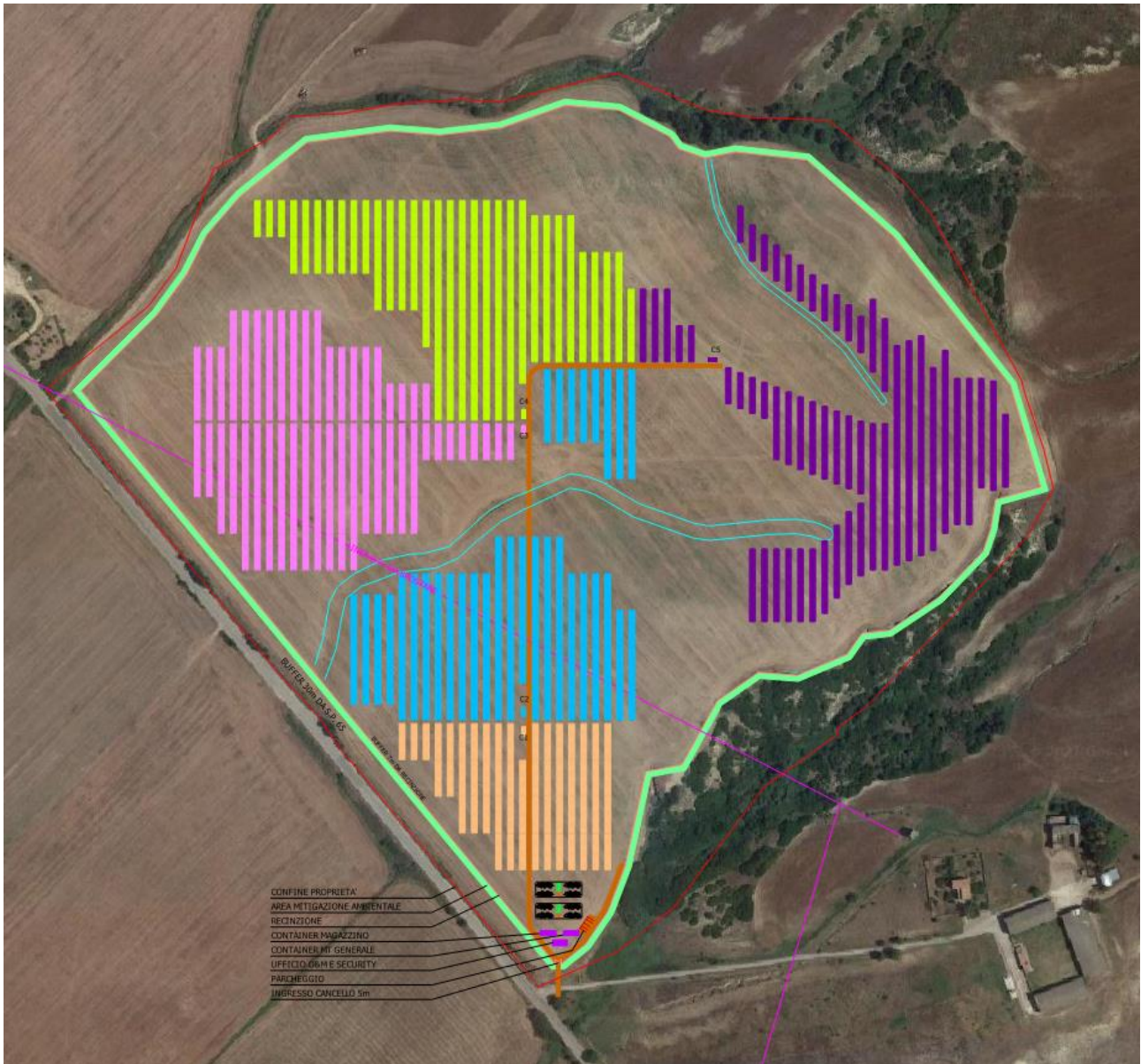
Figura 2 - Layout d'impianto su ortofoto
