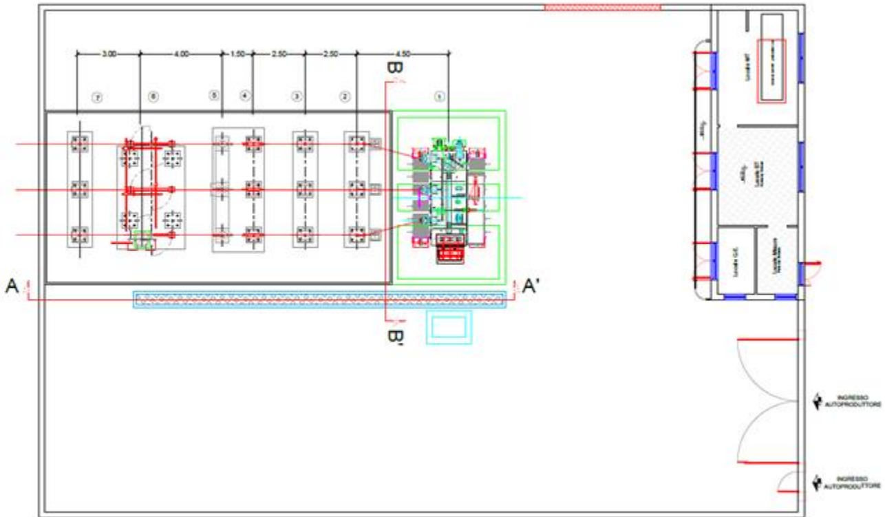
Figura 10 - Layout della sottostazione utente
