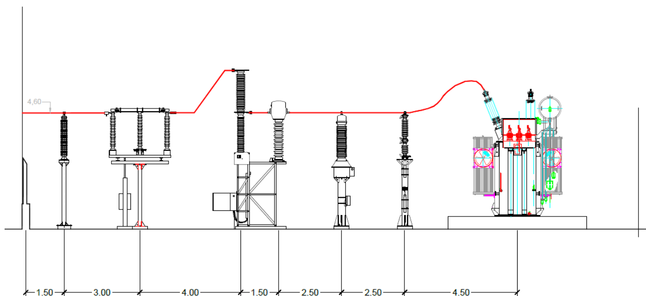
Figura 11 - Vista laterale delle apparecchiature elettromeccaniche in AT
