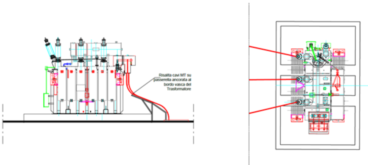
Figura 12 - Viste in sezione e in piante del trasformatore AT/MT
