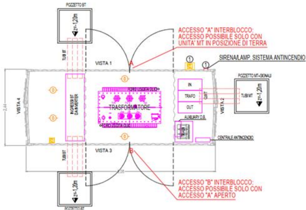
Figura 6 - Layout preliminare cabina di trasformazione BT/MT
