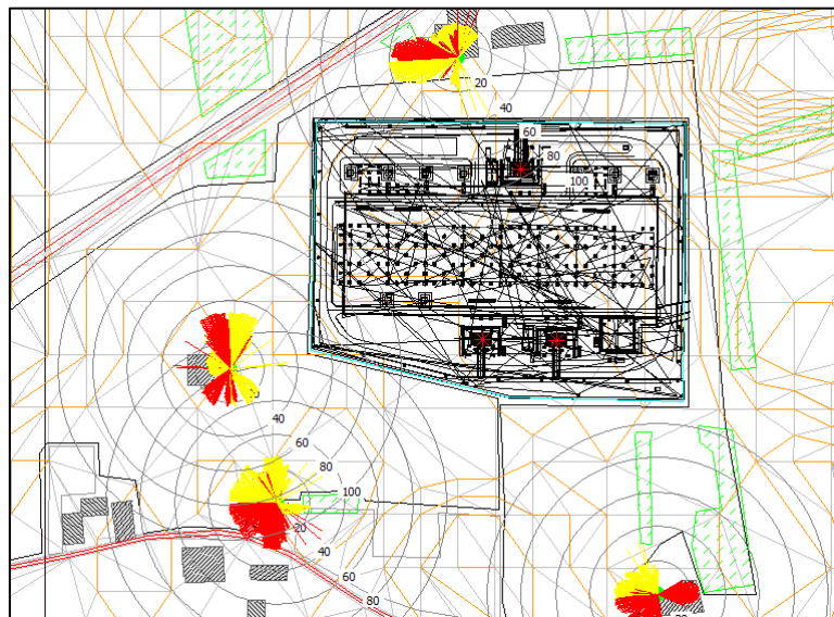
Figura 4: Specifica dell'applicazione della tecnica di calcolo a tracciamento di raggi (ray-tracing).
