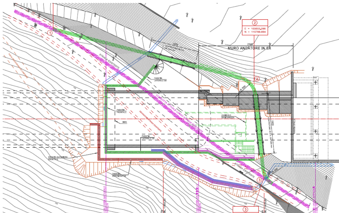
Planimetria interventi risoluzione condotta forzata Iscla
