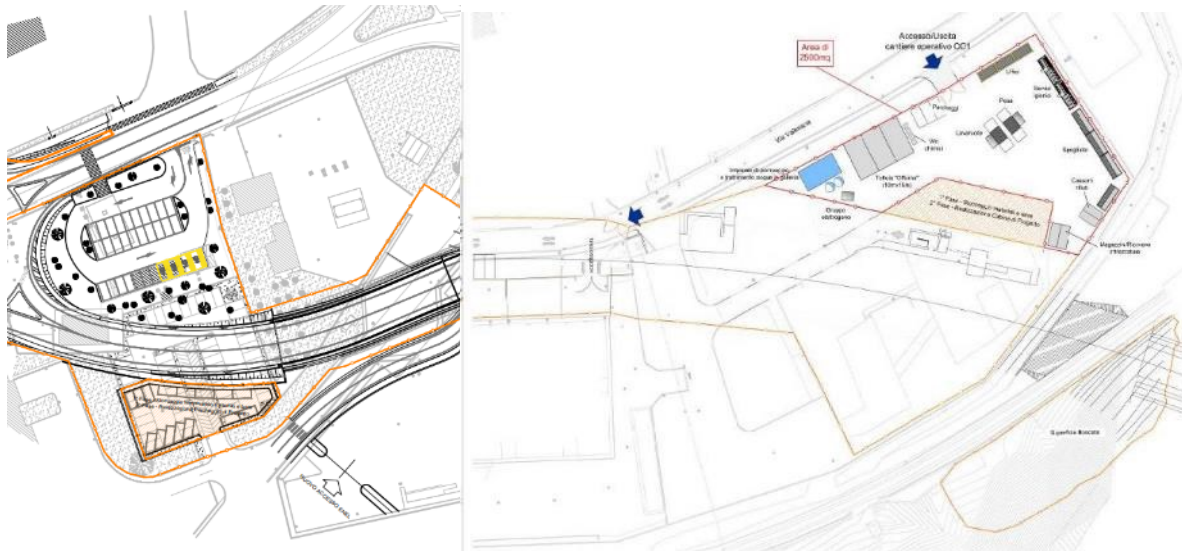
Figura 4.1.5 –Layout del Cantiere Operativo Sud – inquadramenti di dettaglio (fonte: V02CA00CANSC01_C)
