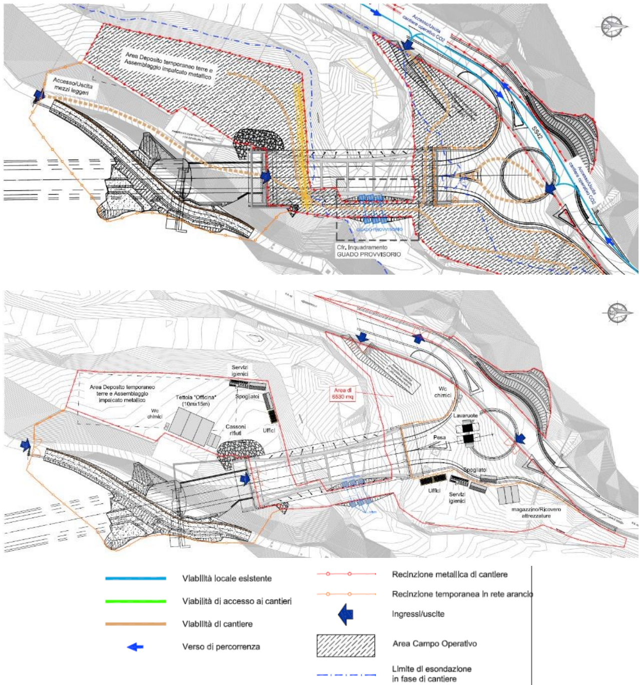
Figura 4.1.6 – Localizzazione e layout del Cantiere Operativo Nord (fonte: V01CA00CANPL01_C e V01CA00CANSC01_C)
