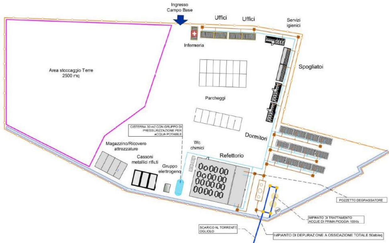
Figura 4.1.3 – Dettaglio del layout del cantiere base
