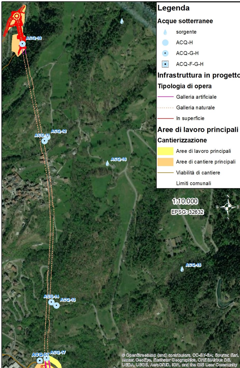
Figura 6.2.3 – Localizzazione delle postazioni di monitoraggio – galleria naturale
