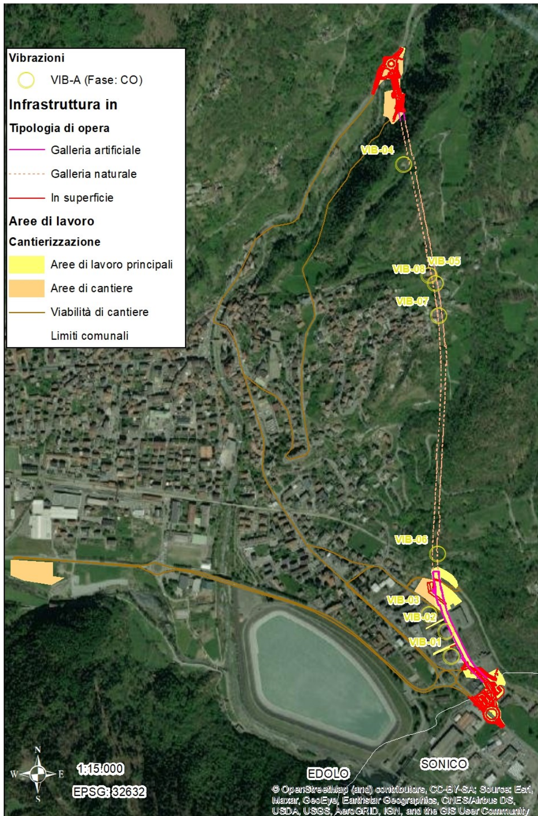
Figura 6.6.1 - Planimetria localizzazione dei monitoraggi – inquadramento componente Vibrazione
