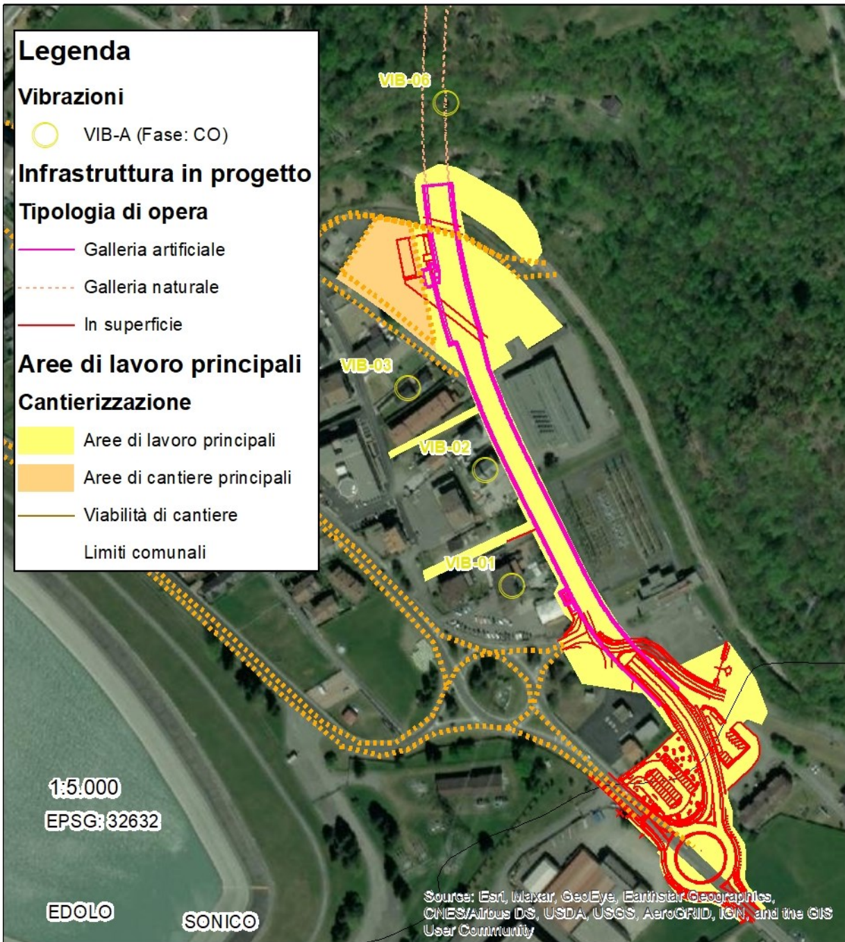
Figura 6.6.2 - Planimetria localizzazione indicativa postazioni di monitoraggio della componente Vibrazioni – Cantiere Operativo Sud
