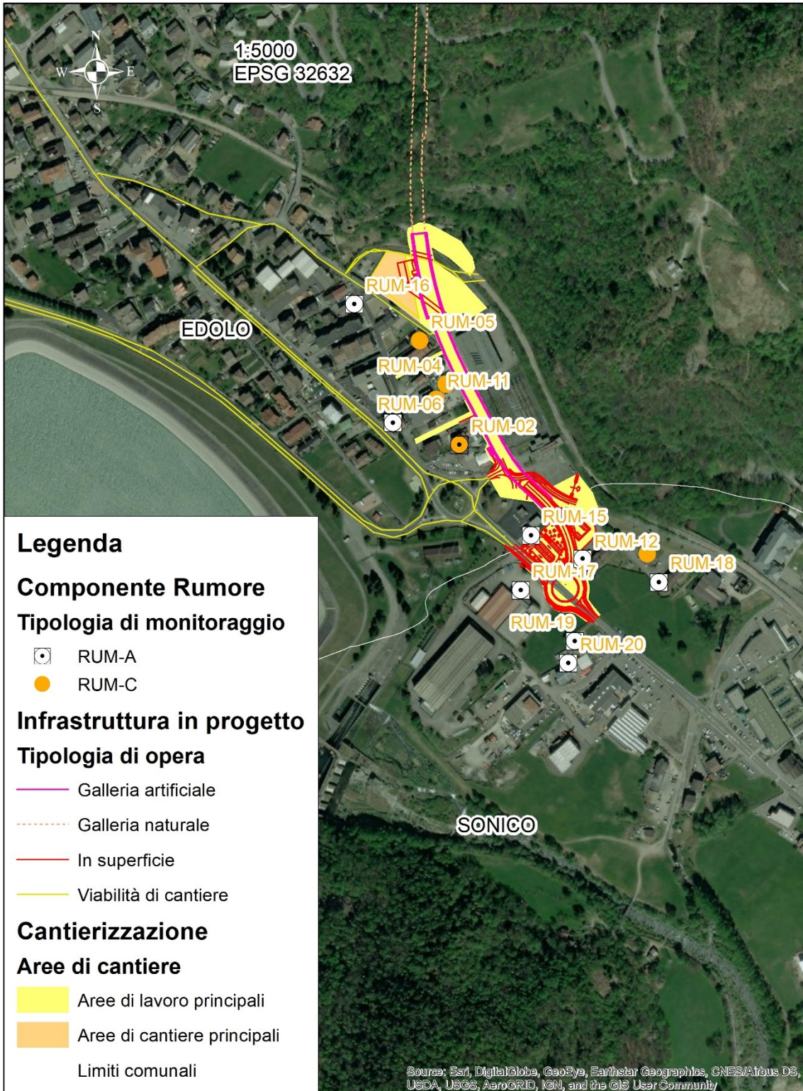
Figura 6.5.2 - Planimetria localizzazione indicativa postazioni di monitoraggio della componente Rumore – Cantiere Operativo Sud
