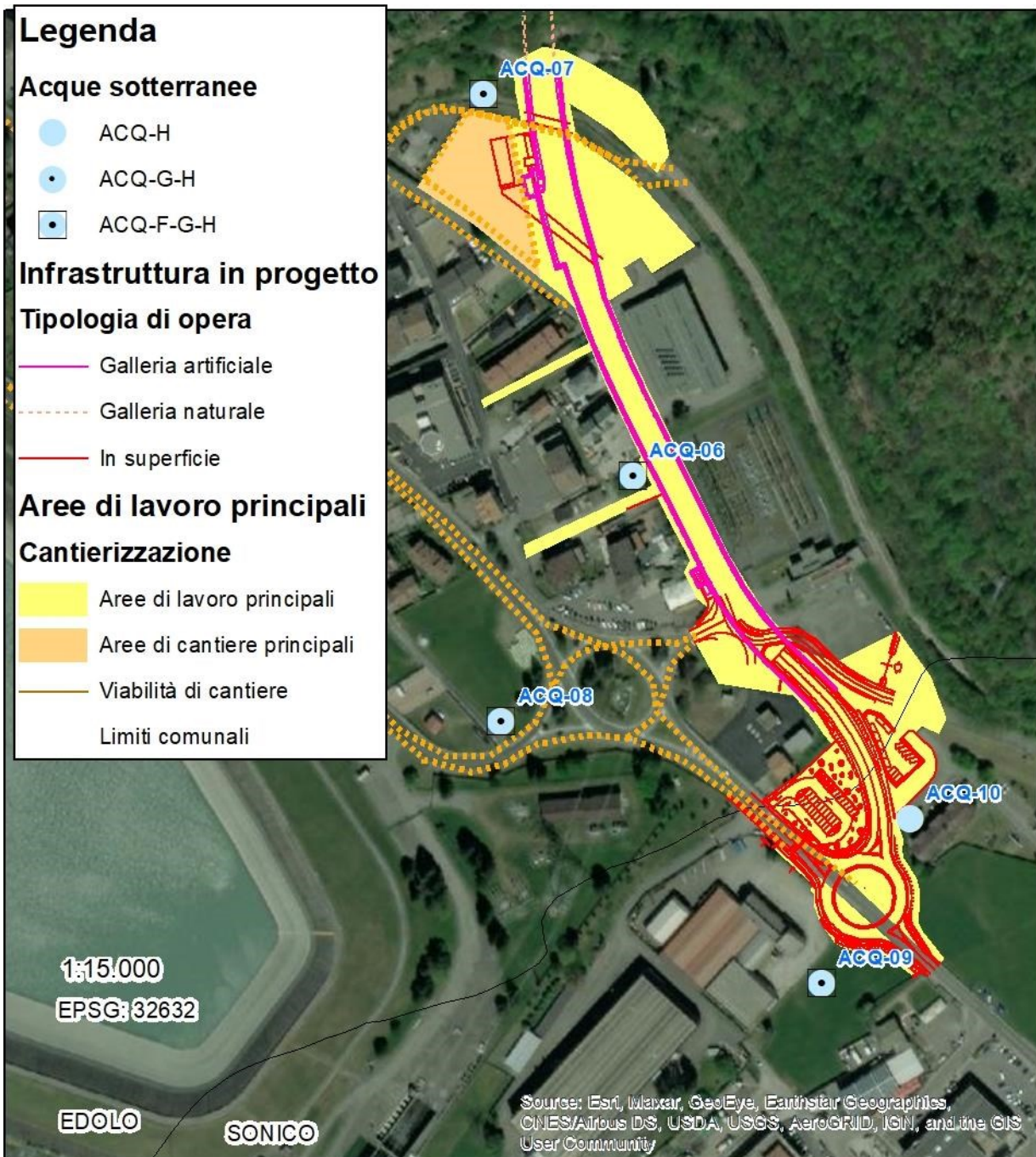
Figura 6.2.4 – Localizzazione delle postazioni di monitoraggio presso il Cantiere Operativo Sud
