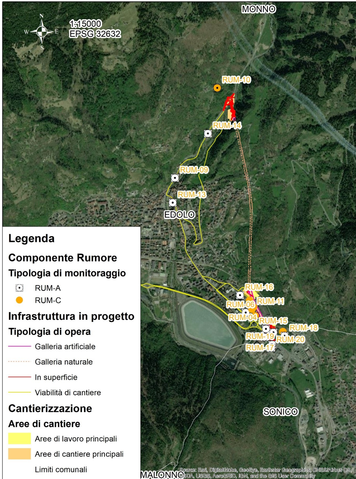
Figura 6.5.1 - Planimetria localizzazione dei monitoraggi – inquadramento componente Rumore
