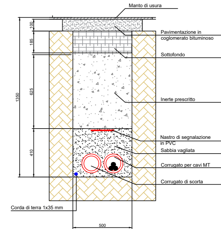
Posa n. 5 1 CORRUGATO+SCORTA PER 1 CAVO MT SU STRADA ASFALTATA
