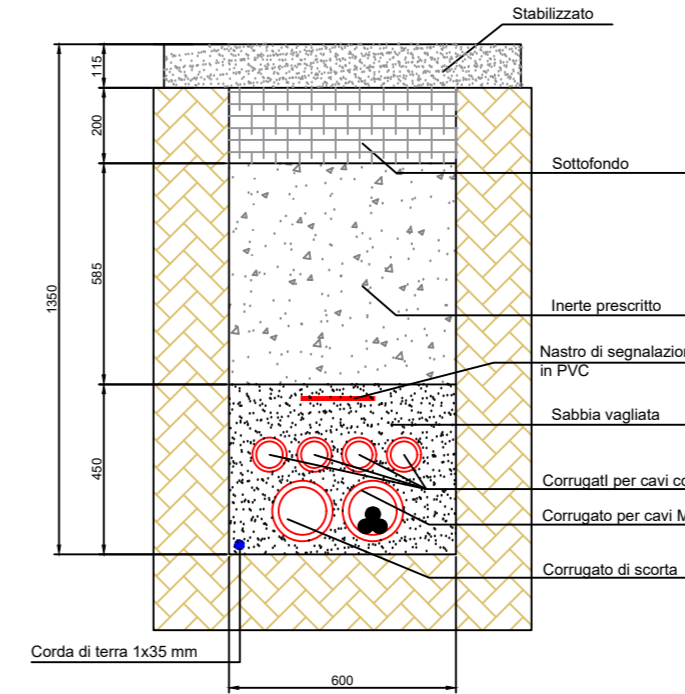
Posa n. 5 1 CORRUGATO+SCORTA PER 1 CAVO MT SU STRADA ASFALTATA
