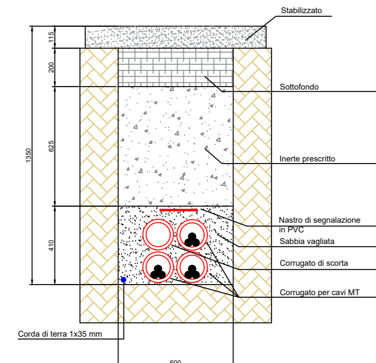
Posa n. 7 3 CORRUGATI+SCORTA PER 3 CAVI MT SU STRADA INTERNA
