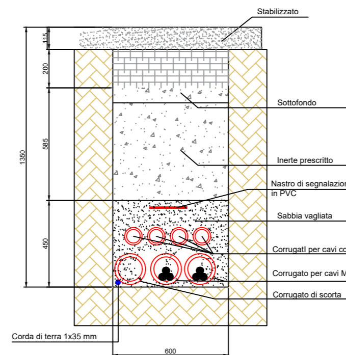
Posa n. 6 1 CORRUGATO+SCORTA PER 2 CAVI MT+DA 1 A 4 CORRUGATI PER CAVI CA SU STRADA INTERNA
