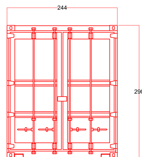
Fronte
