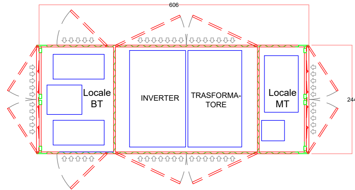
SEZIONE LONGITUDINALE
