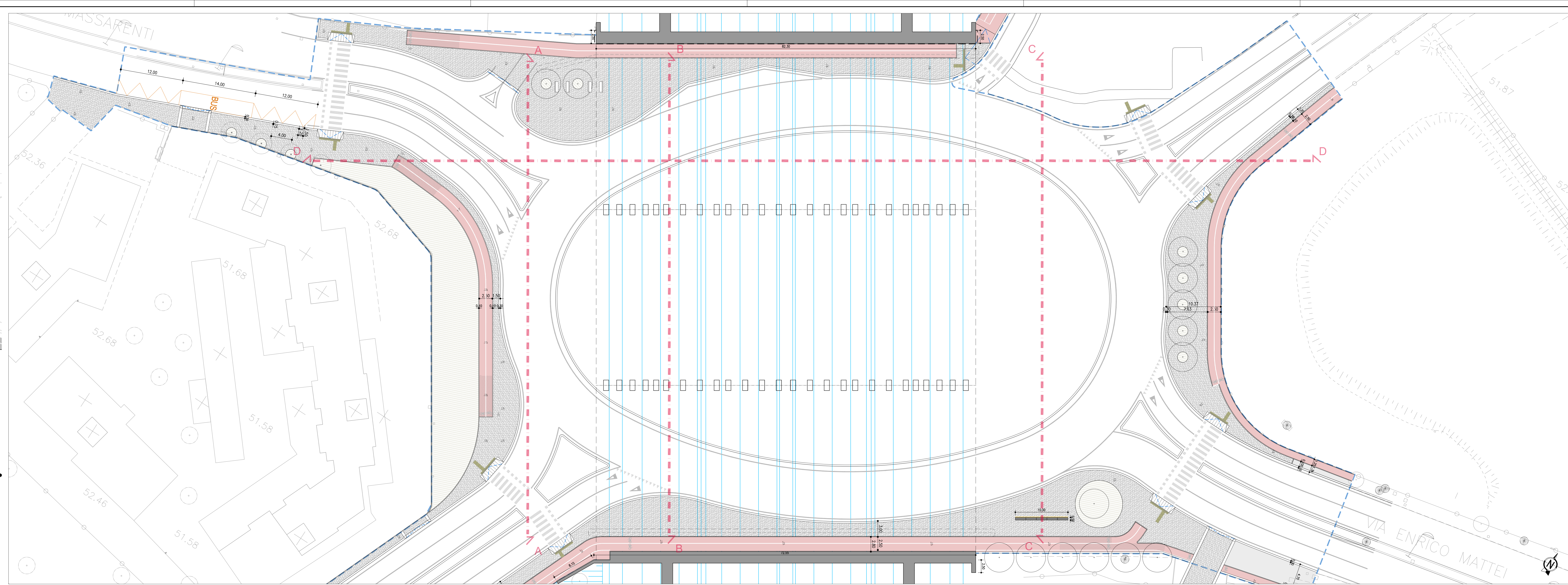
PROGETTO, planimetria (scala 1:250)
