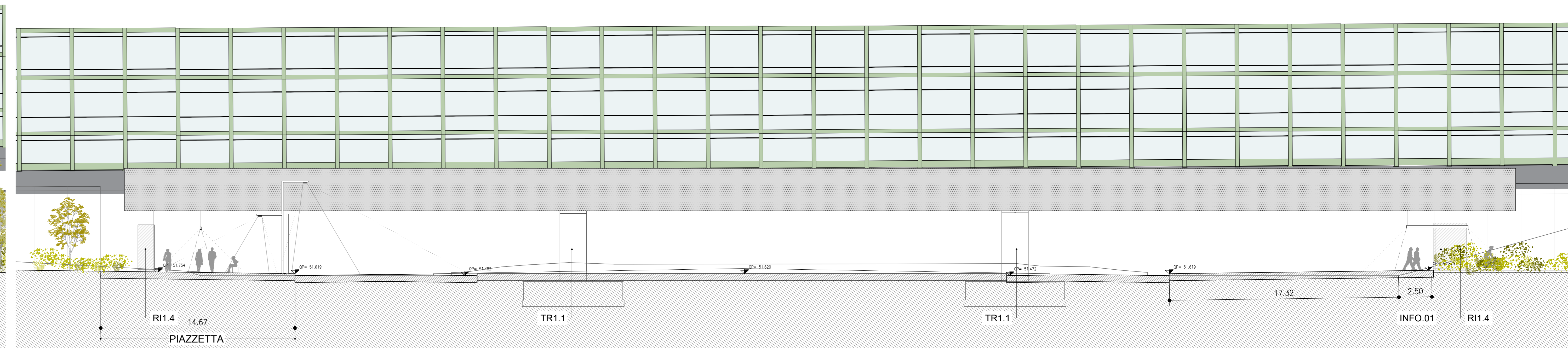
SEZIONE BB (scala 1:150)
