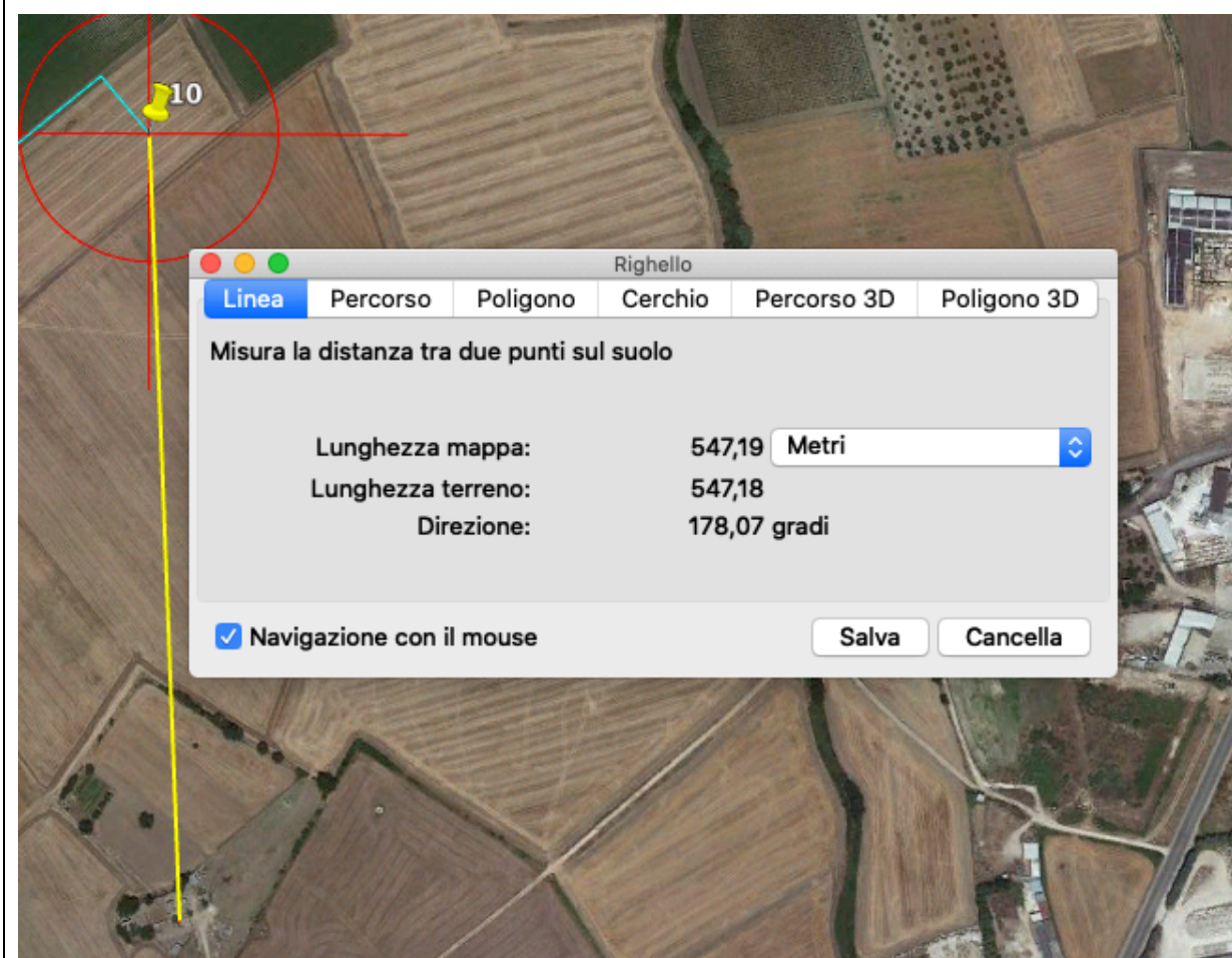
WTG 10 distanza da R4 m.547
