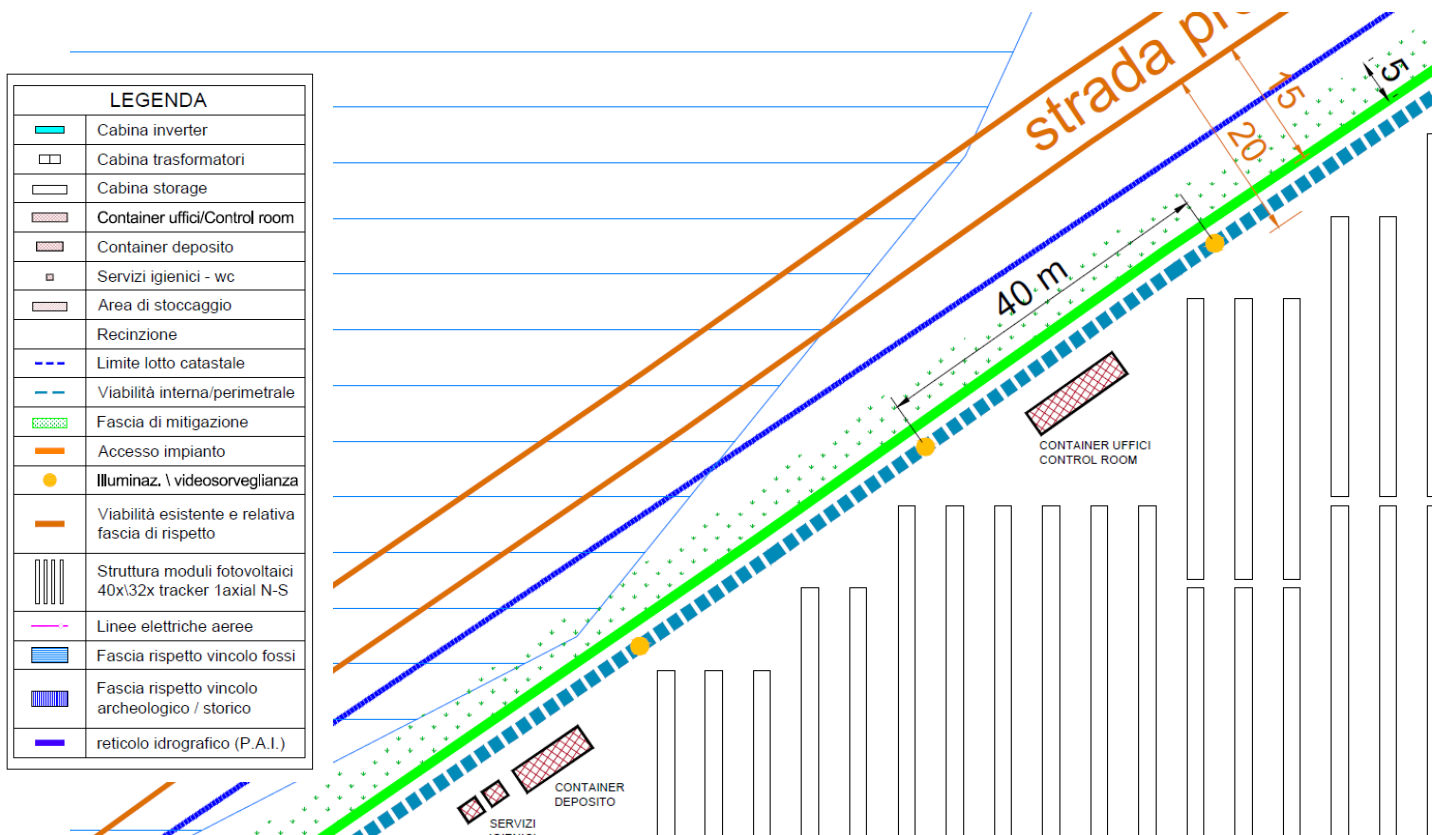
Posizionamento corpi illuminanti, tavola esemplificativa.
