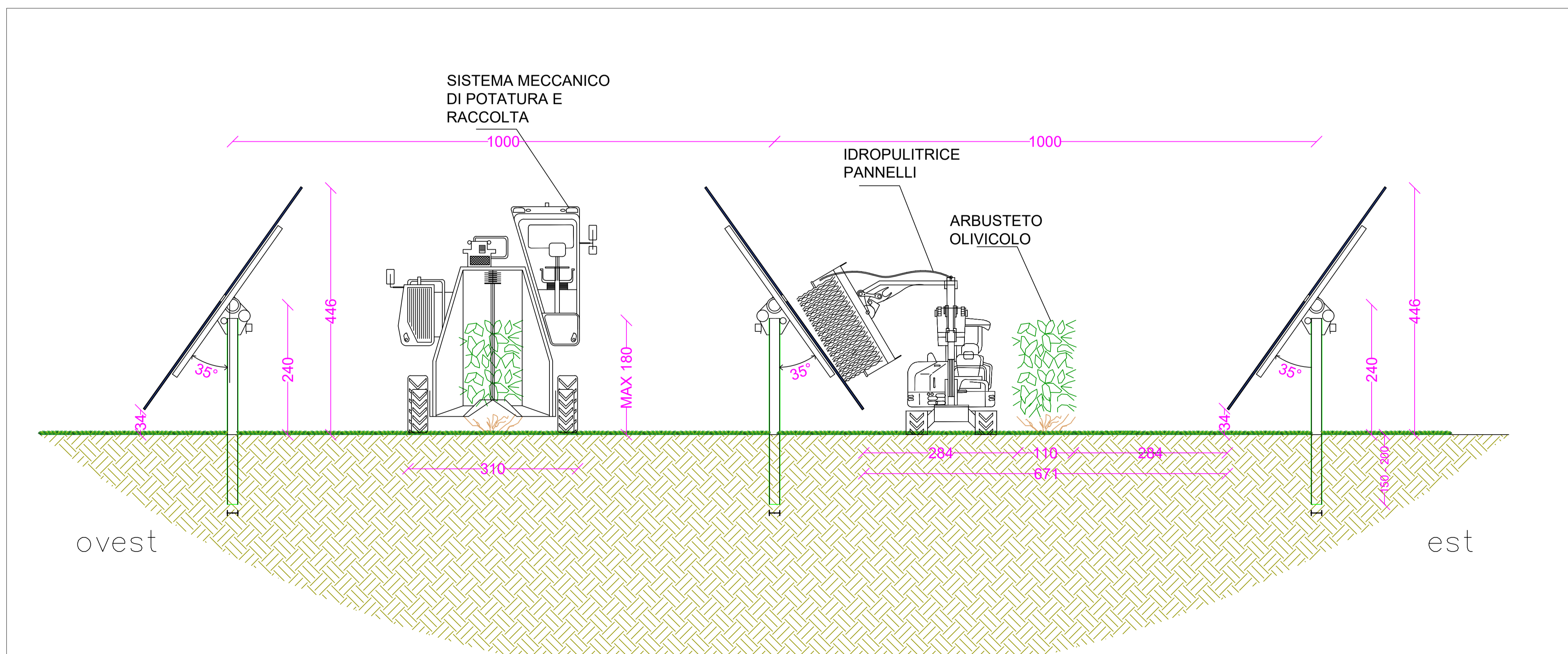
SCHEMA DI SEZIONE TIPO DISPOSIZIONE FILARI NELLA CONFIGURAZIONE DI MANUTENZIONE - SCALA 1:50
