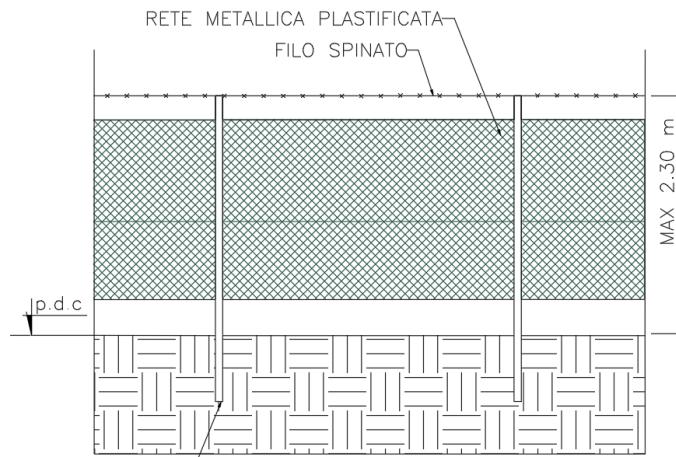
Figura 11 - Tipico recinzione perimetrale area impianto di generazione
