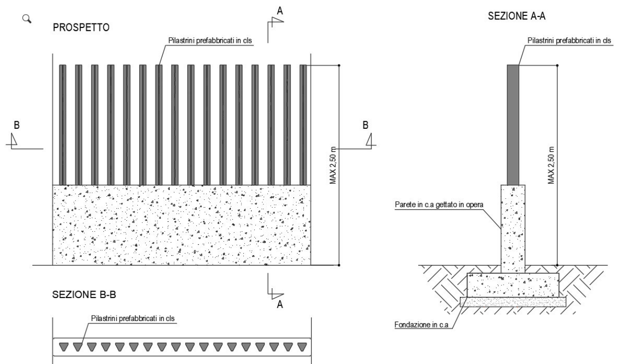
Figura 12 - Tipico recinzione perimetrale SE utente ed impianto di generazione
