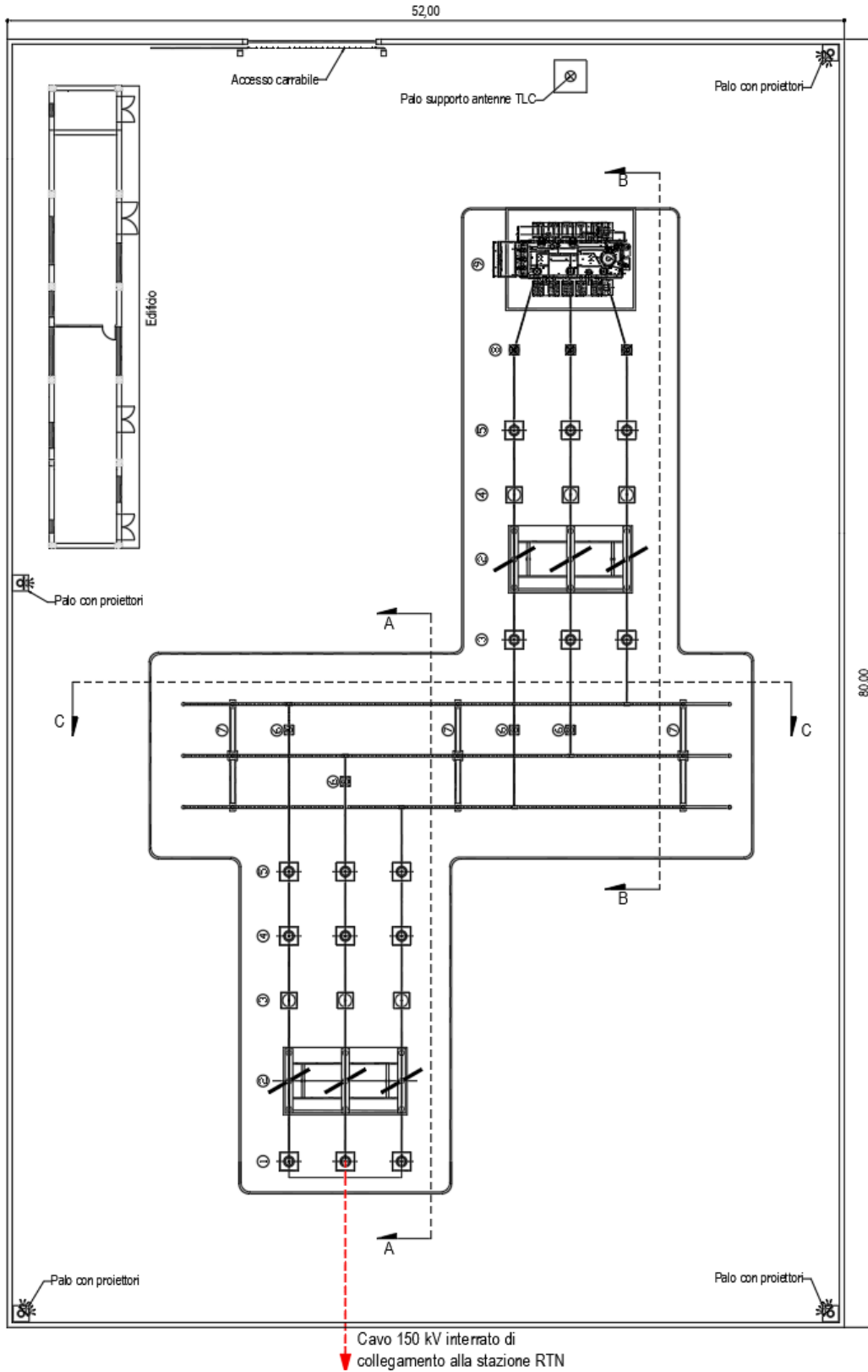
Figura 15 – Planimetria SE utente
