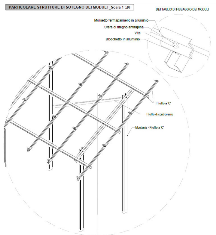
Figura 8 - Stralcio Particolare costruttivo supporto
