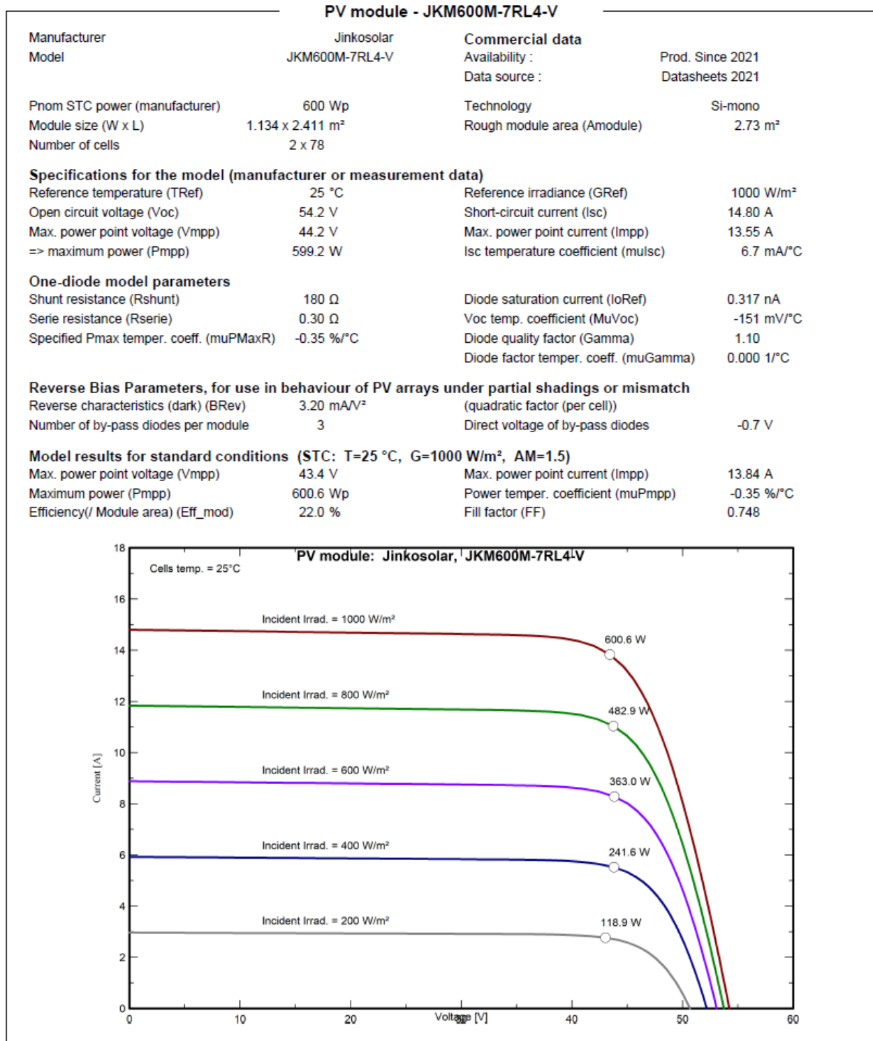
Figura 13 – Stralcio Scheda tecnica Pannello FV da 600 Wp
