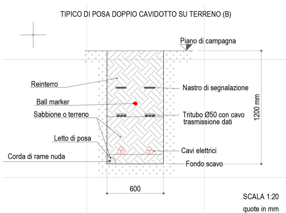
Figura 5 - Tipico posa cavidotto su terreno
