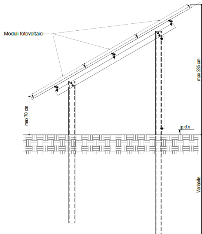
Figura 7 - Sezione pannello fotovoltaico su supporto
