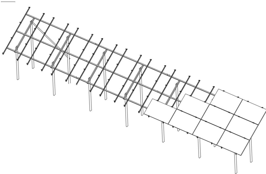
Figura 6 - Schema strutture di sostegno di tipo fisso
