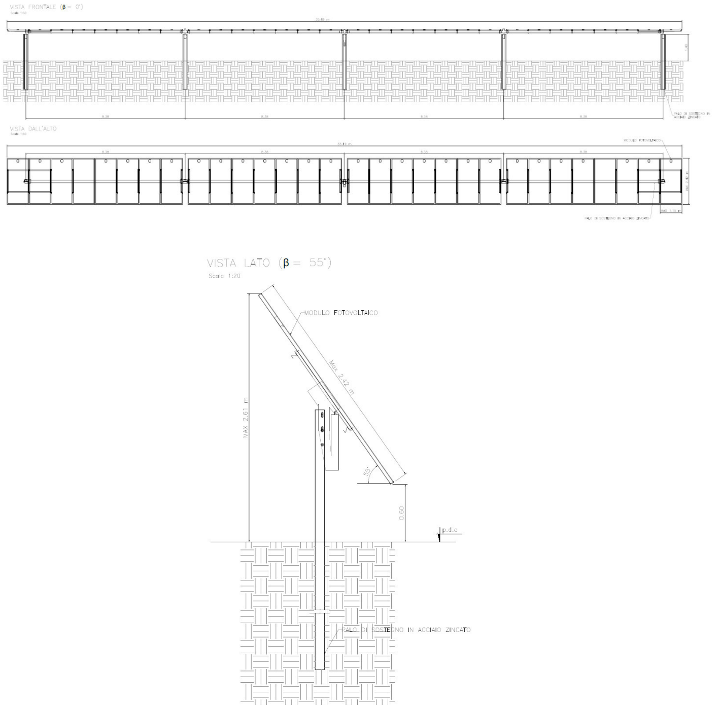
Figura 9 - Stralcio Particolare costruttivo tracker
