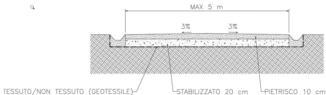
Figura 10 - Sezione tipo -viabilità interna
