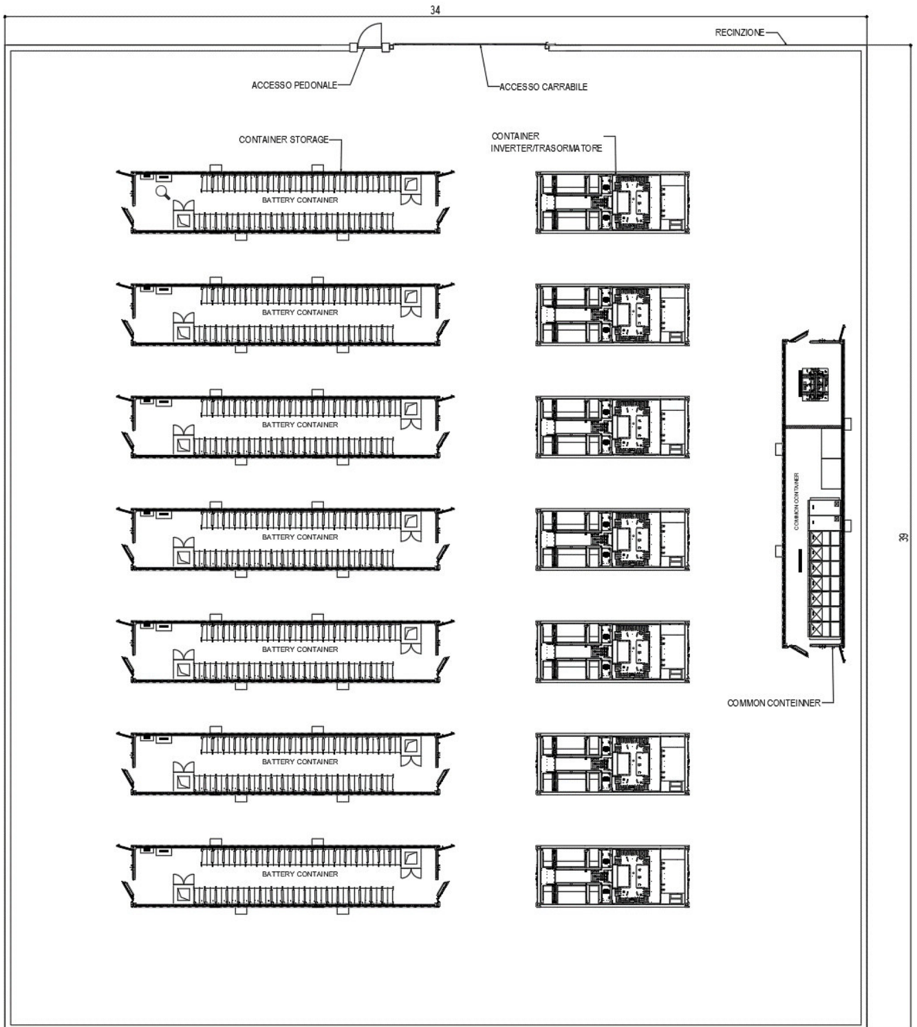
Figura 19 - Planimetria impianto di accumulo elettrochimico
