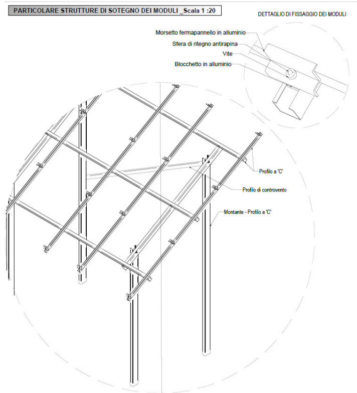
Figura 5 – Stralcio Particolare costruttivo supporto fisso
