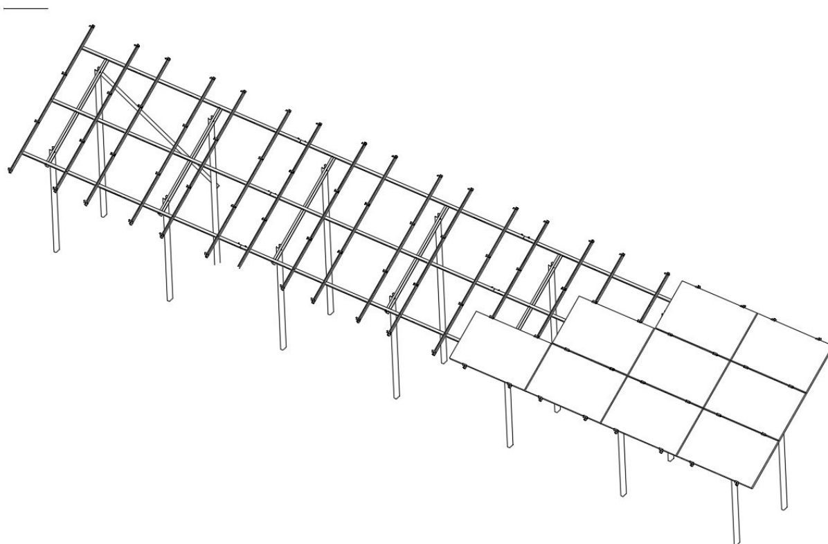
Figura 3 - Schema strutture di sostegno tipo fisso
