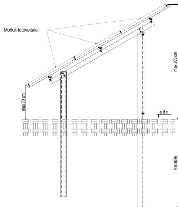
Figura 4 - Sezione pannello fotovoltaico su supporto fisso
