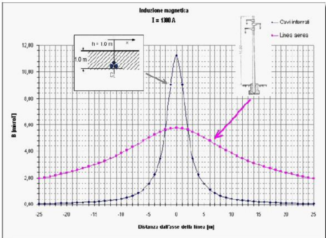
Figura 1: Attenuazione dell'induzione magnetica dovuta all'interramento dei cavi
