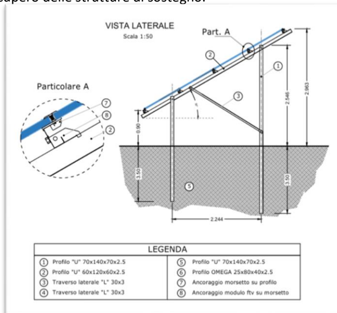
Figura 3 sezione strutture di sostegno
