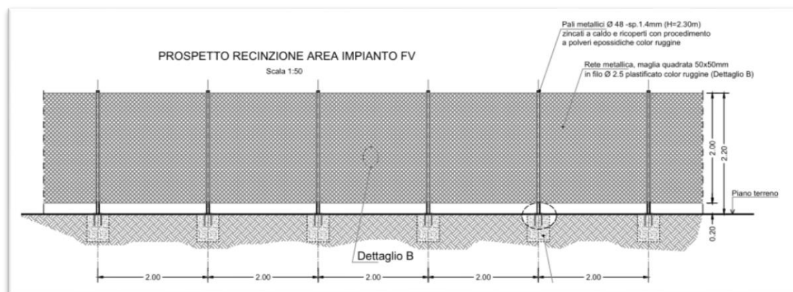
Figura 4 recinzione
