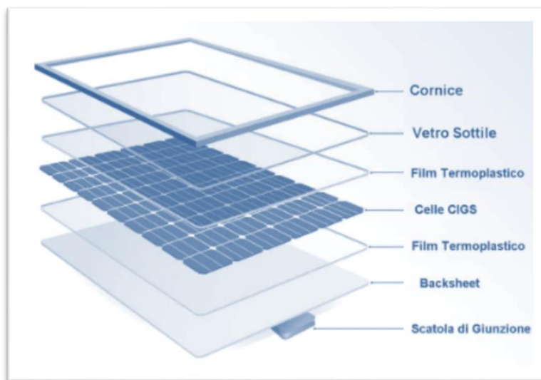
Figura 2 Spaccato modulo fv
