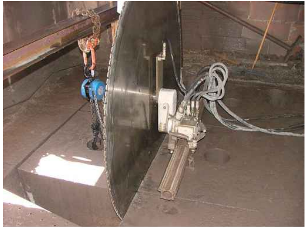
Esempi di esecuzione dei tagli su solai cementizi
