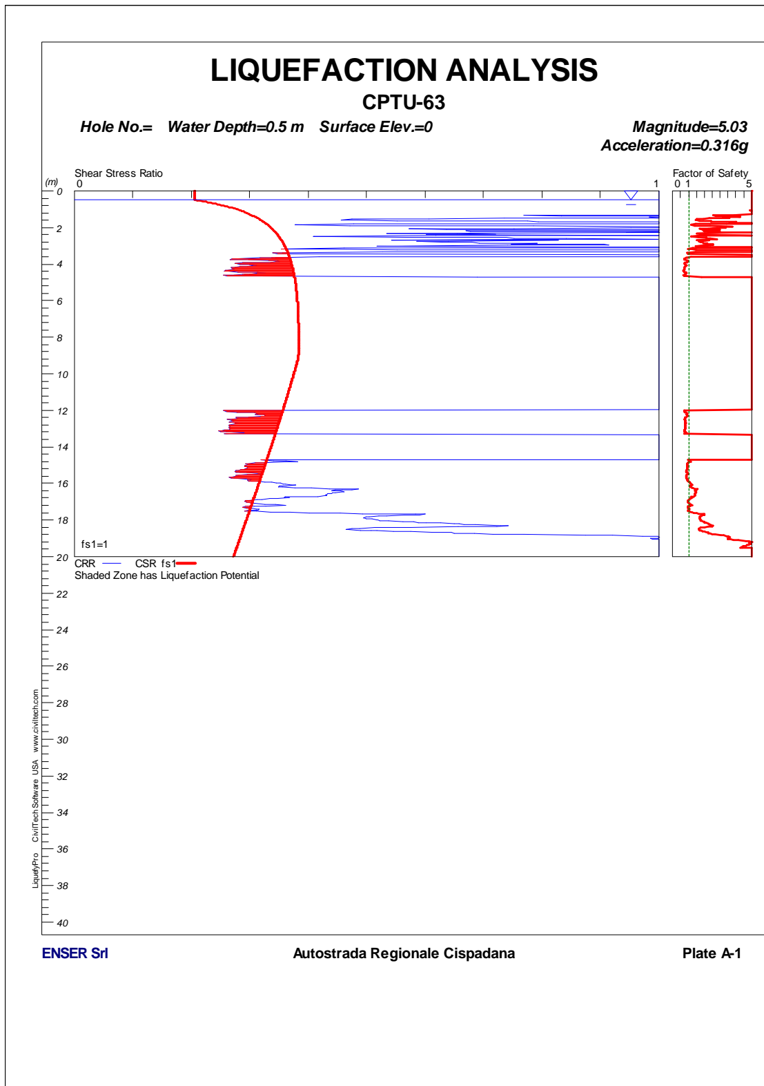
FIGURA 1-38: CPTU63 – VERIFICA A LIQUEFAZIONE.
