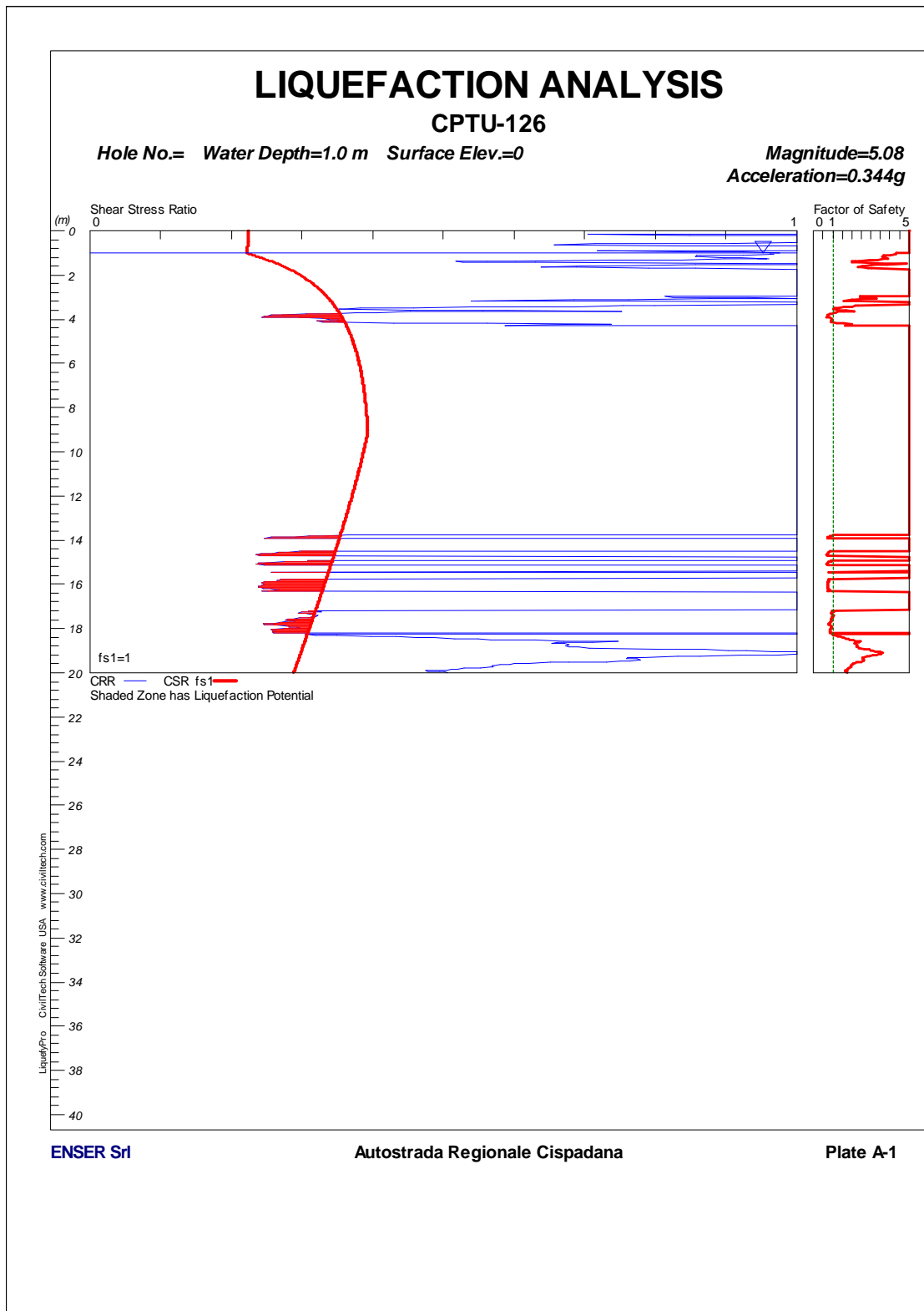
FIGURA 1-86: CPTU126 – VERIFICA A LIQUEFAZIONE.
