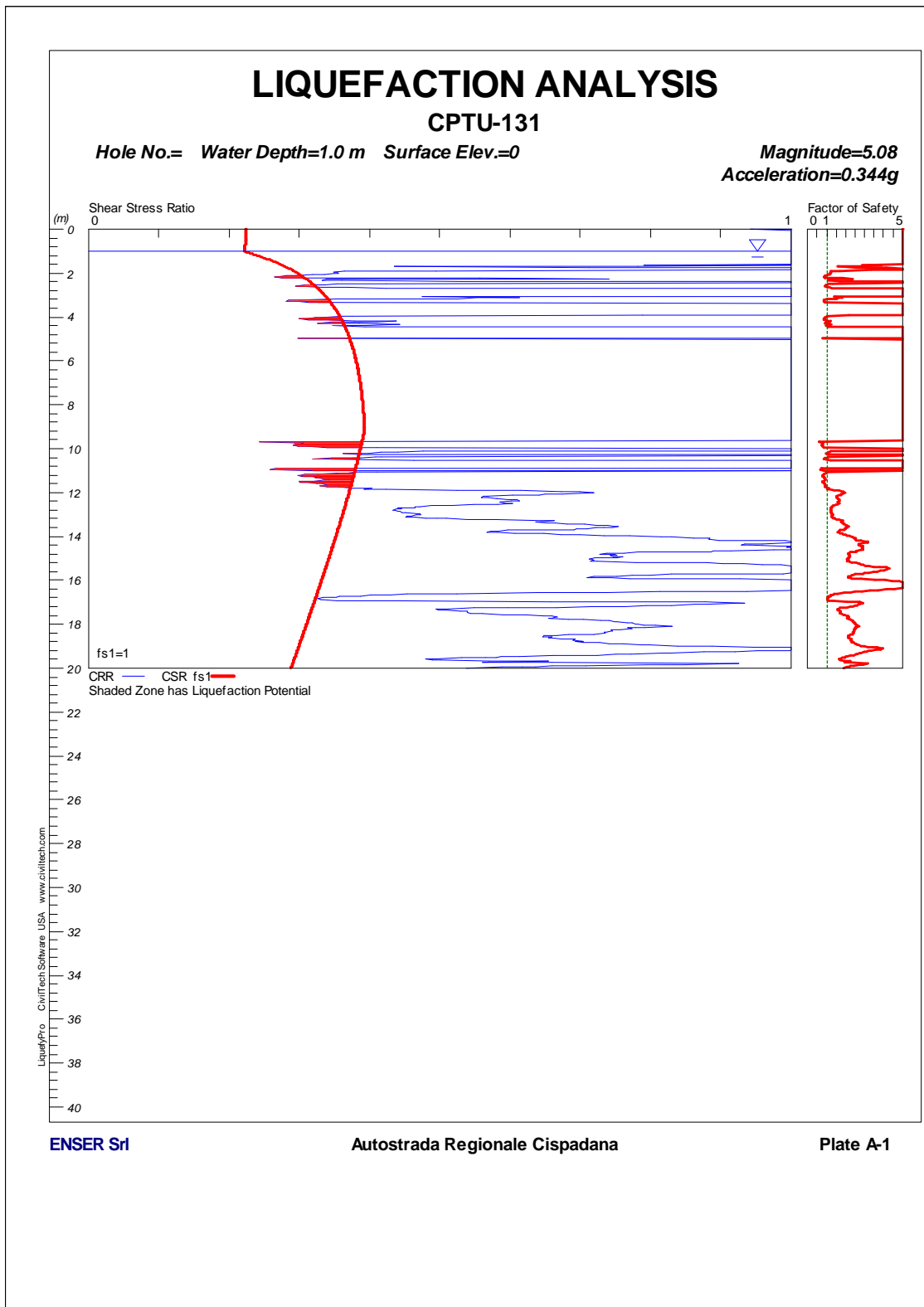
FIGURA 1-89: CPTU131 – VERIFICA A LIQUEFAZIONE.
