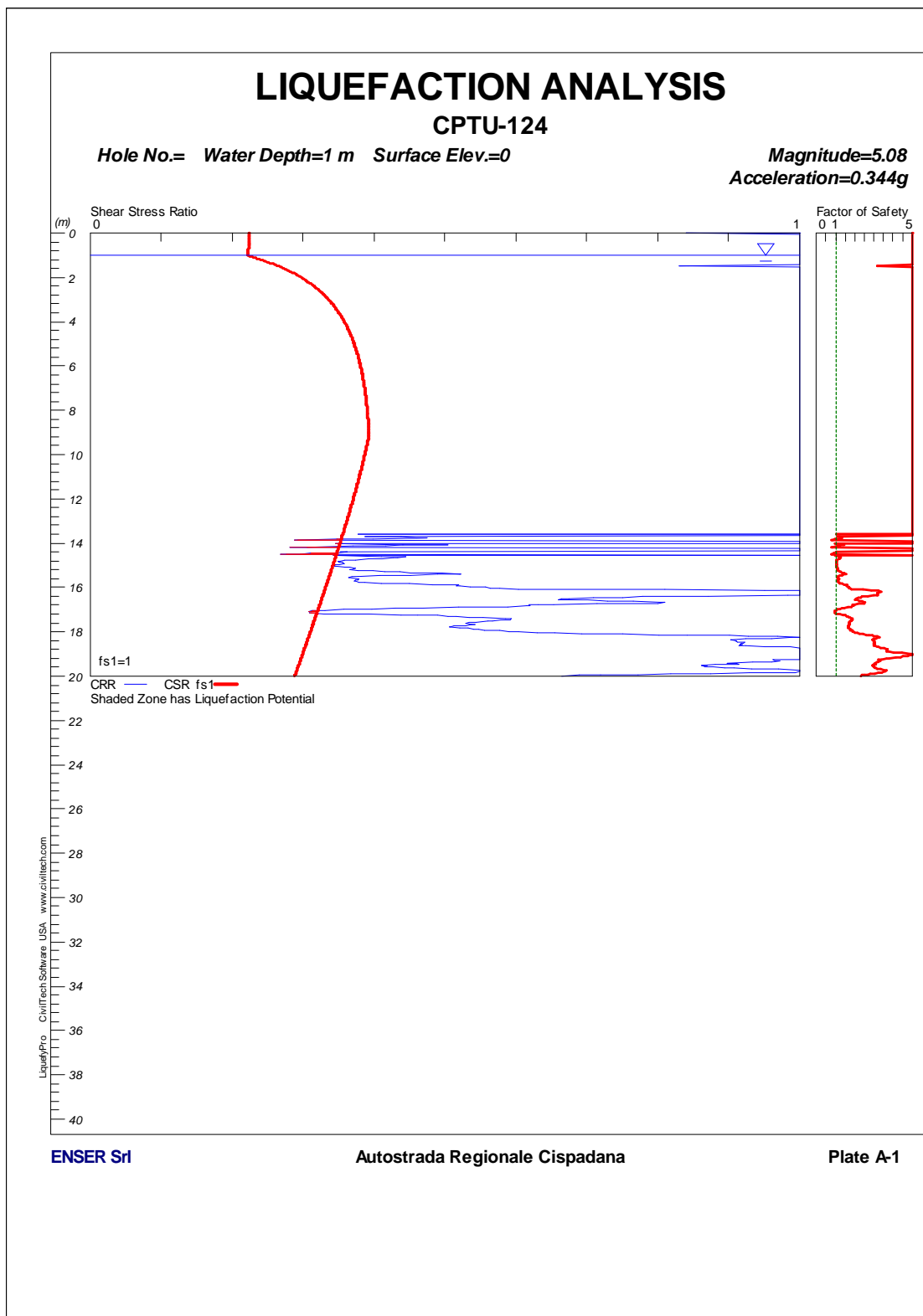
FIGURA 1-84: CPTU124 – VERIFICA A LIQUEFAZIONE.
