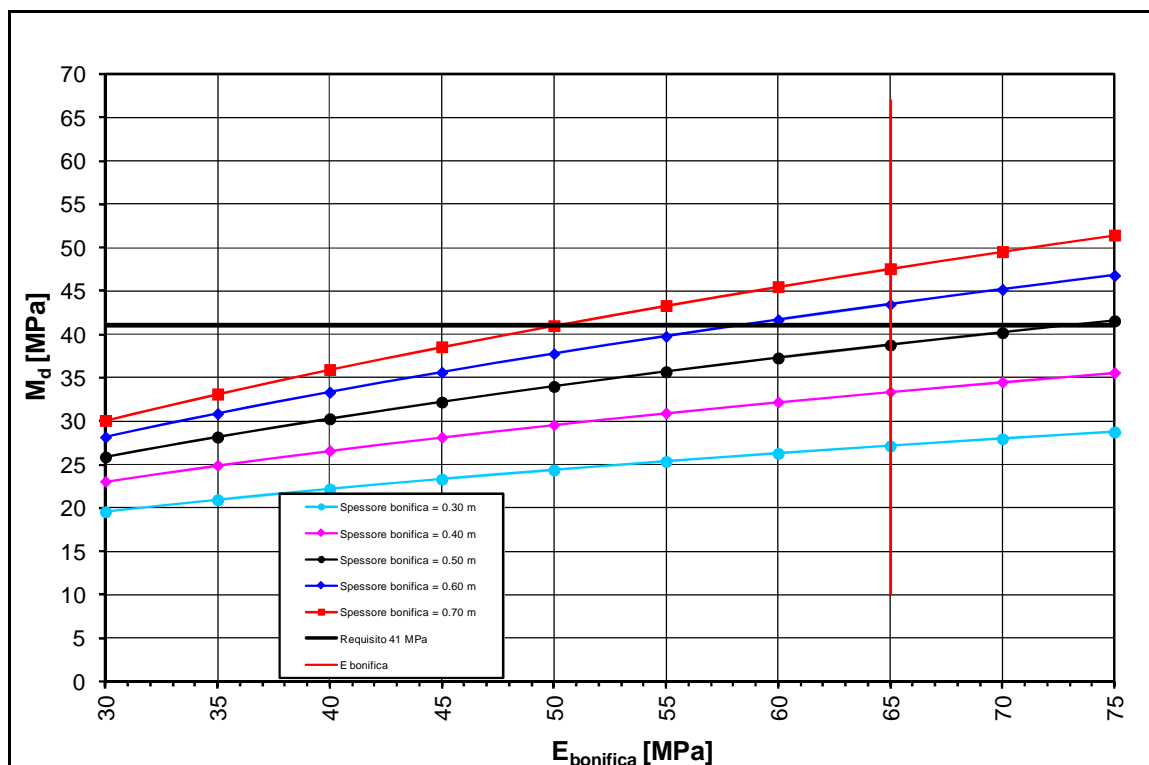
FIGURA 2-24: TRATTO 25 – DETERMINAZIONE SPESSORE DI BONIFICA.
