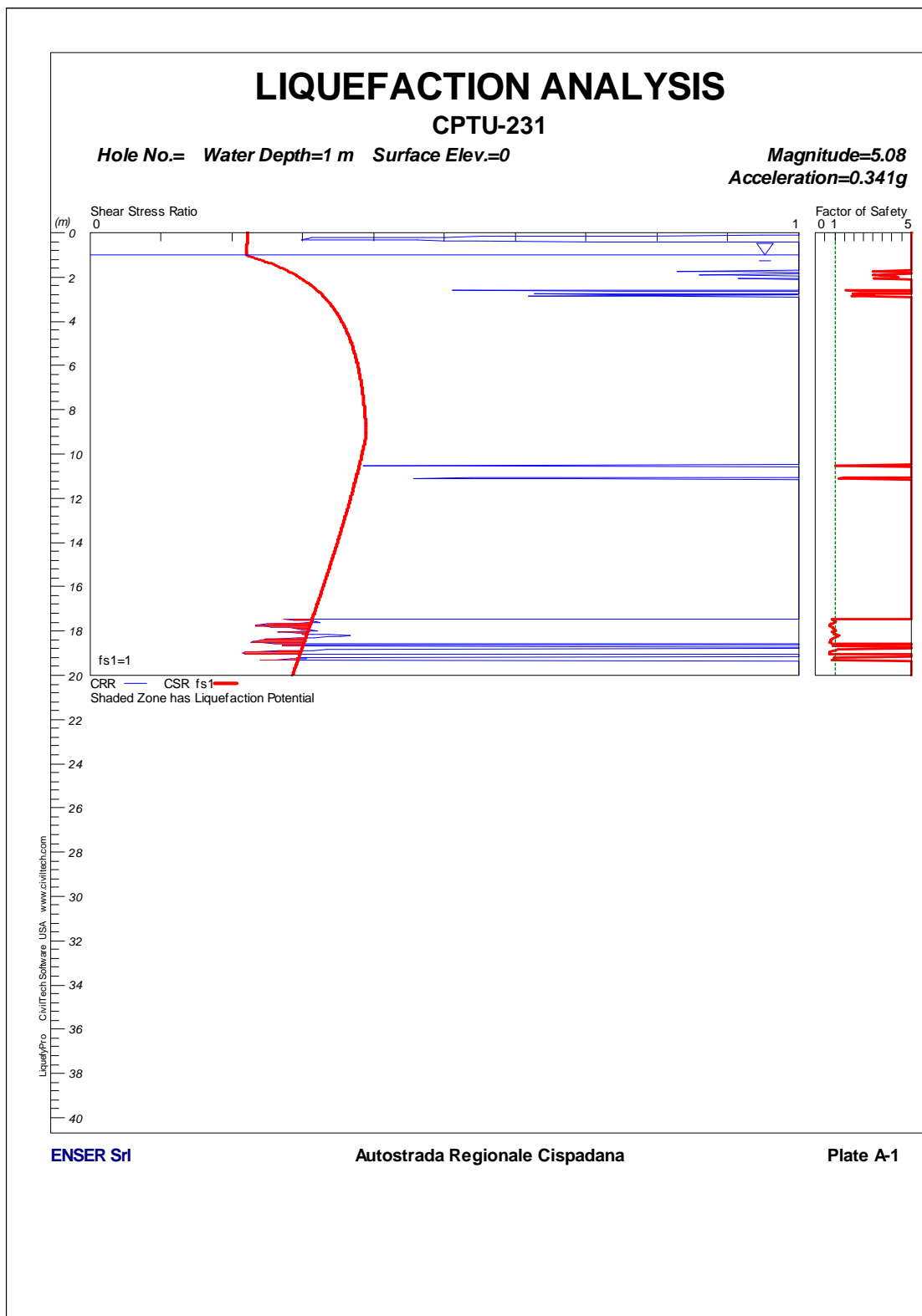
FIGURA 1-107: CPTU231 – VERIFICA A LIQUEFAZIONE.
