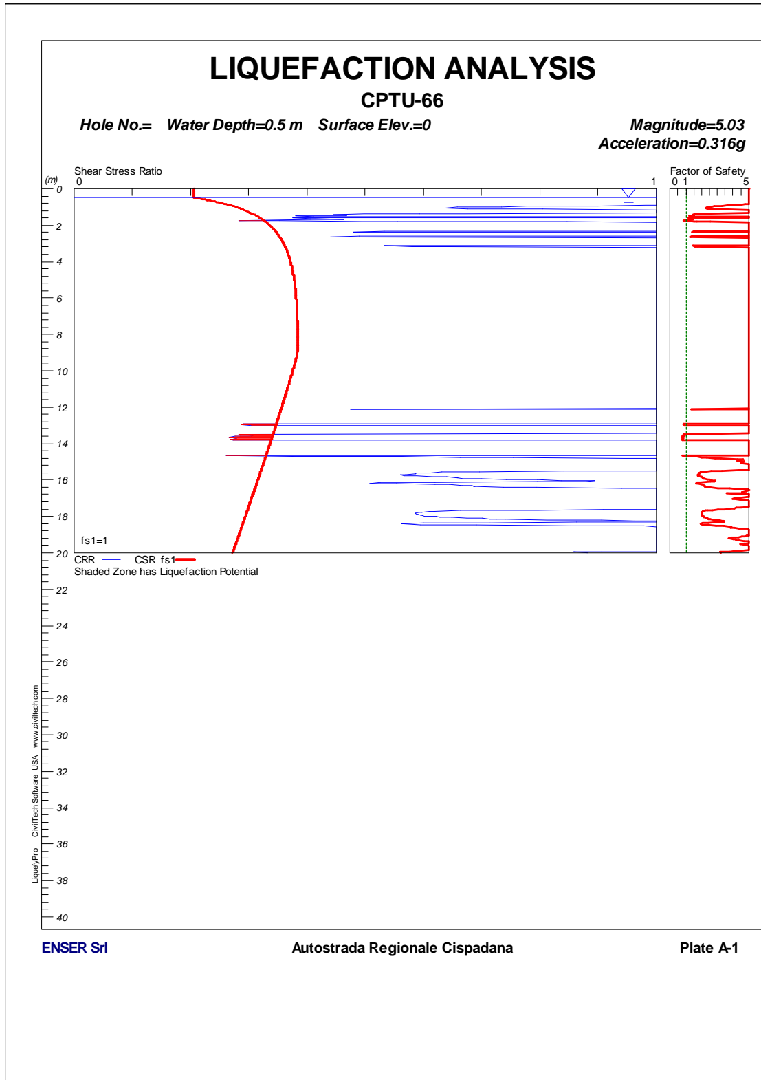
FIGURA 1-41: CPTU66 – VERIFICA A LIQUEFAZIONE.
