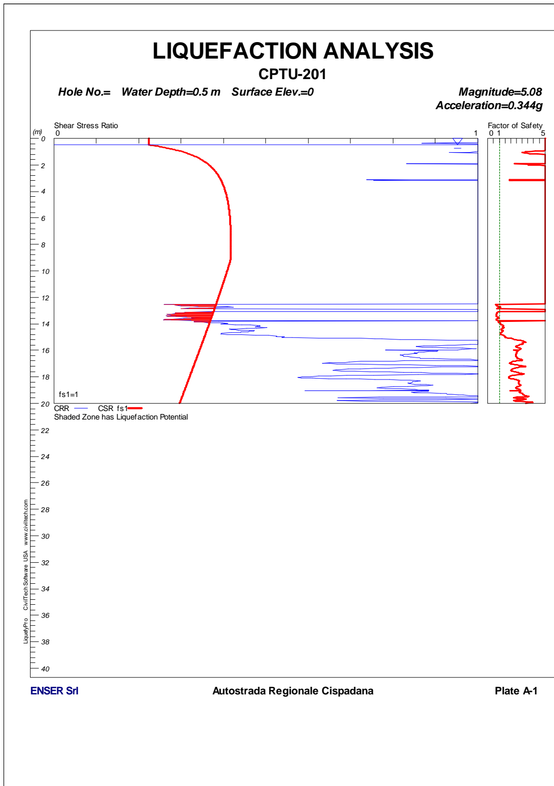
FIGURA 1-91: CPTU201 – VERIFICA A LIQUEFAZIONE.
