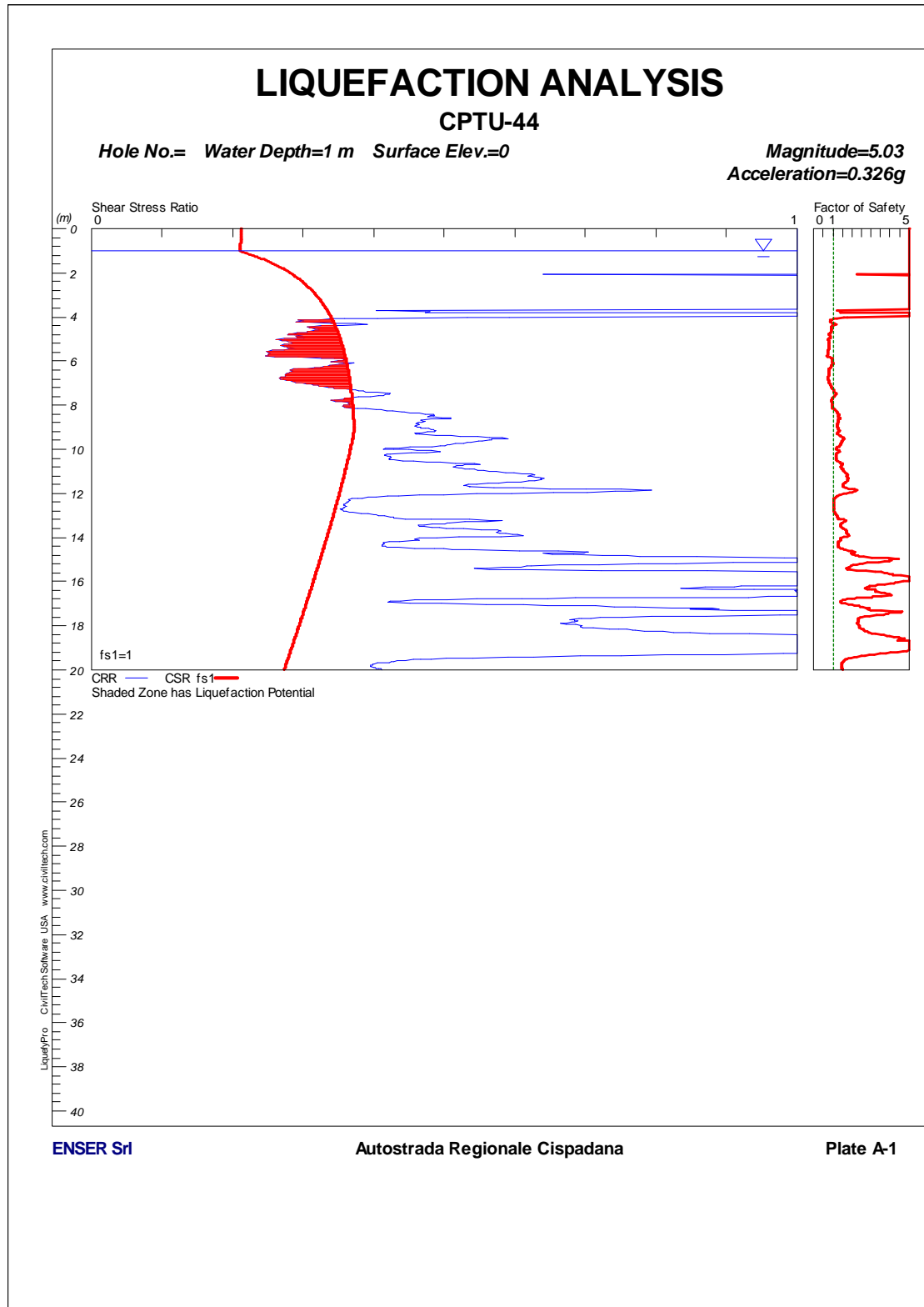
FIGURA 1-19: CPTU44 – VERIFICA A LIQUEFAZIONE.
