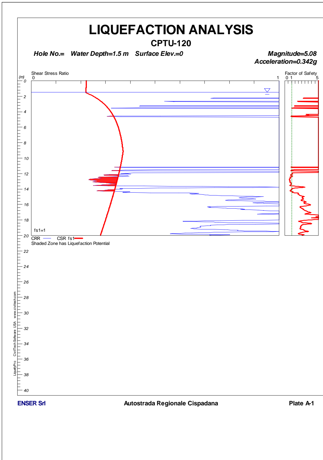
FIGURA 1-80: CPTU120 – VERIFICA A LIQUEFAZIONE.
