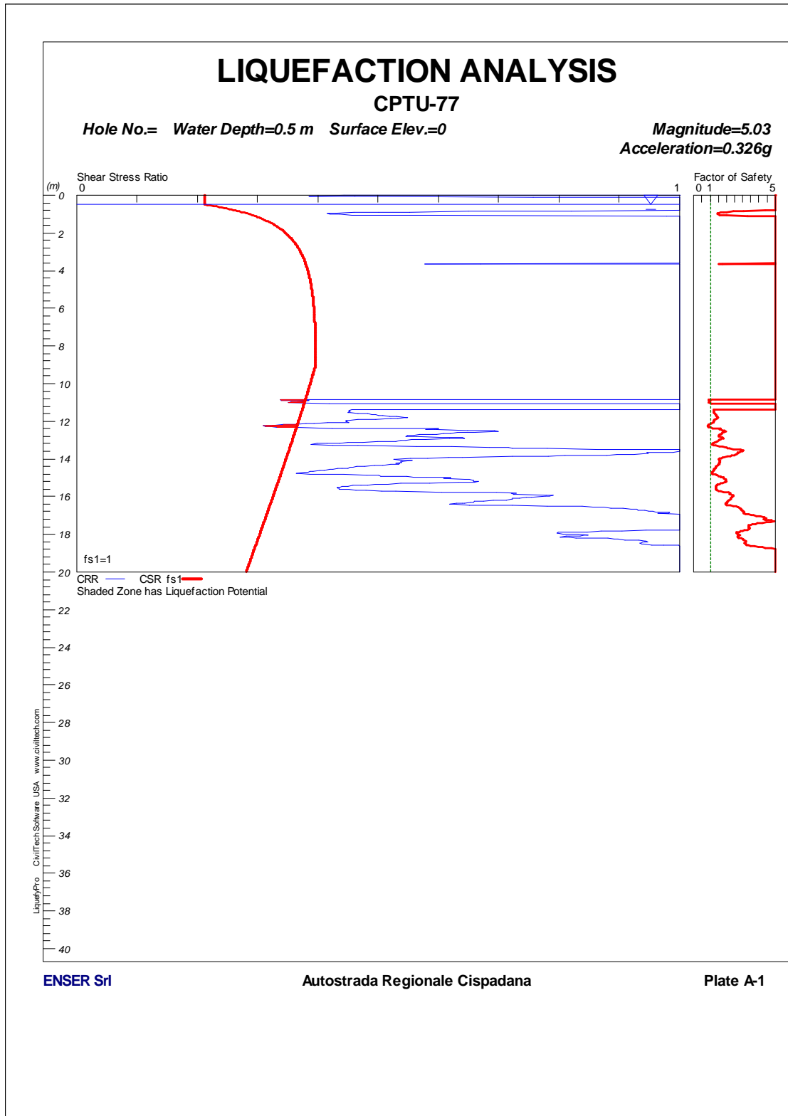
FIGURA 1-47: CPTU77 – VERIFICA A LIQUEFAZIONE.
