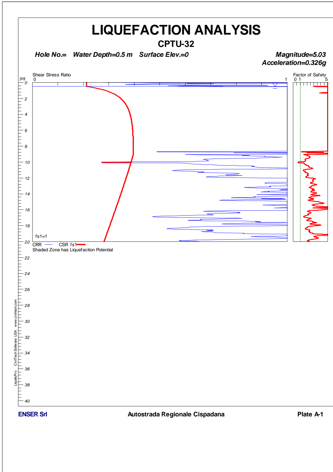
FIGURA 1-10: CPTU32 – VERIFICA A LIQUEFAZIONE.
