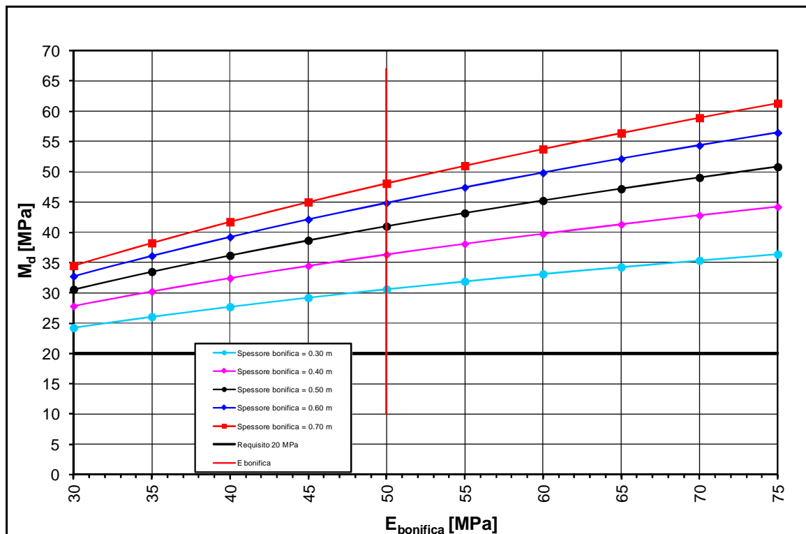
FIGURA 2-3: TRATTO 3 – DETERMINAZIONE SPESSORE DI BONIFICA.
