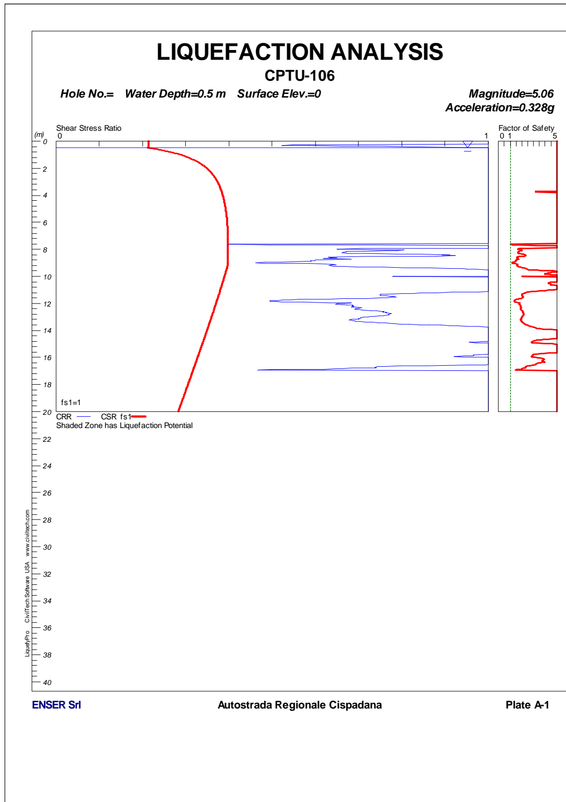
FIGURA 1-67: CPTU106 – VERIFICA A LIQUEFAZIONE.
