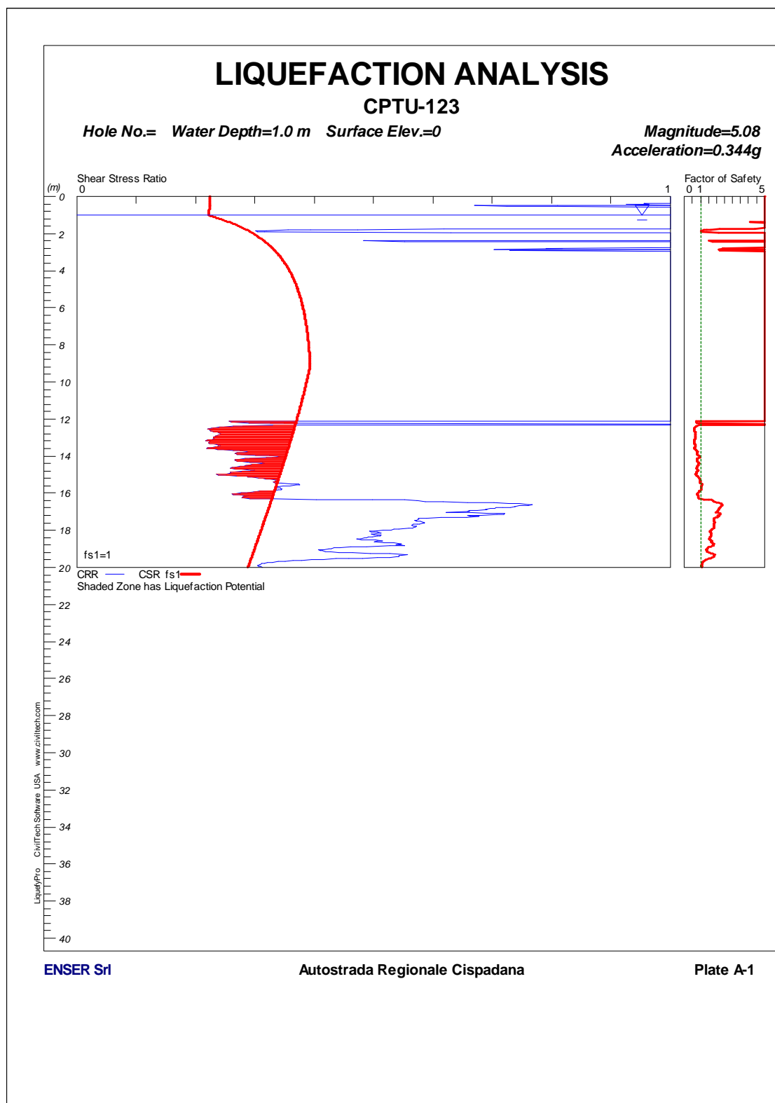
FIGURA 1-83: CPTU123 – VERIFICA A LIQUEFAZIONE.
