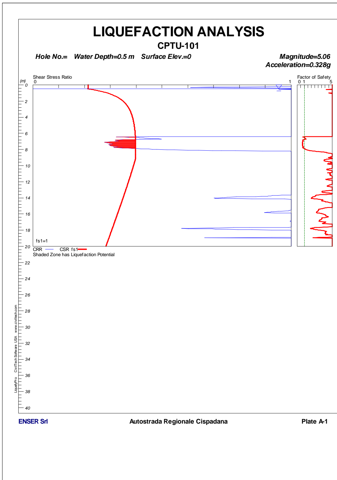
FIGURA 1-62: CPTU101 – VERIFICA A LIQUEFAZIONE.
