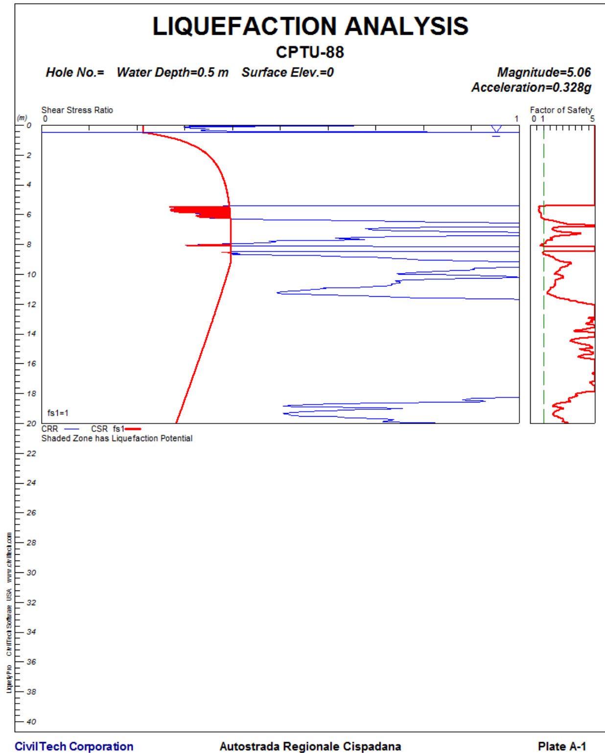
FIGURA 1-53: CPTU88 – VERIFICA A LIQUEFAZIONE.
