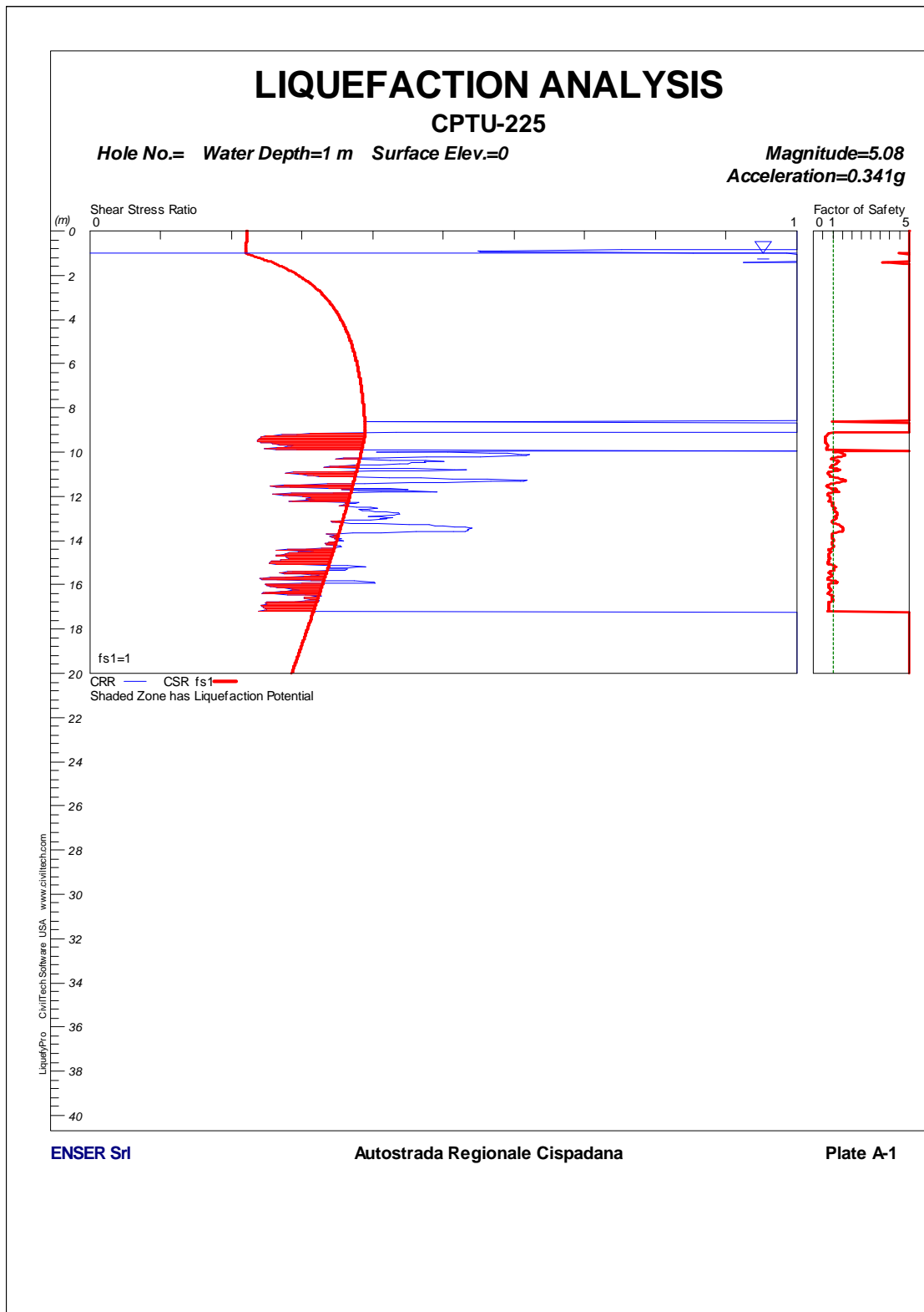
FIGURA 1-105: CPTU225 – VERIFICA A LIQUEFAZIONE.
