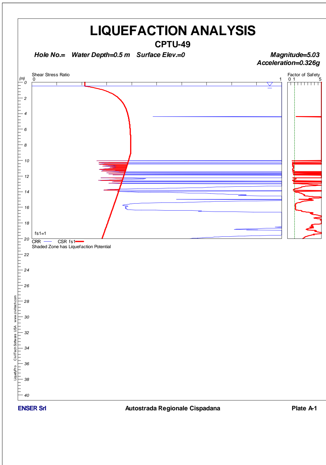
FIGURA 1-24: CPTU49 – VERIFICA A LIQUEFAZIONE.
