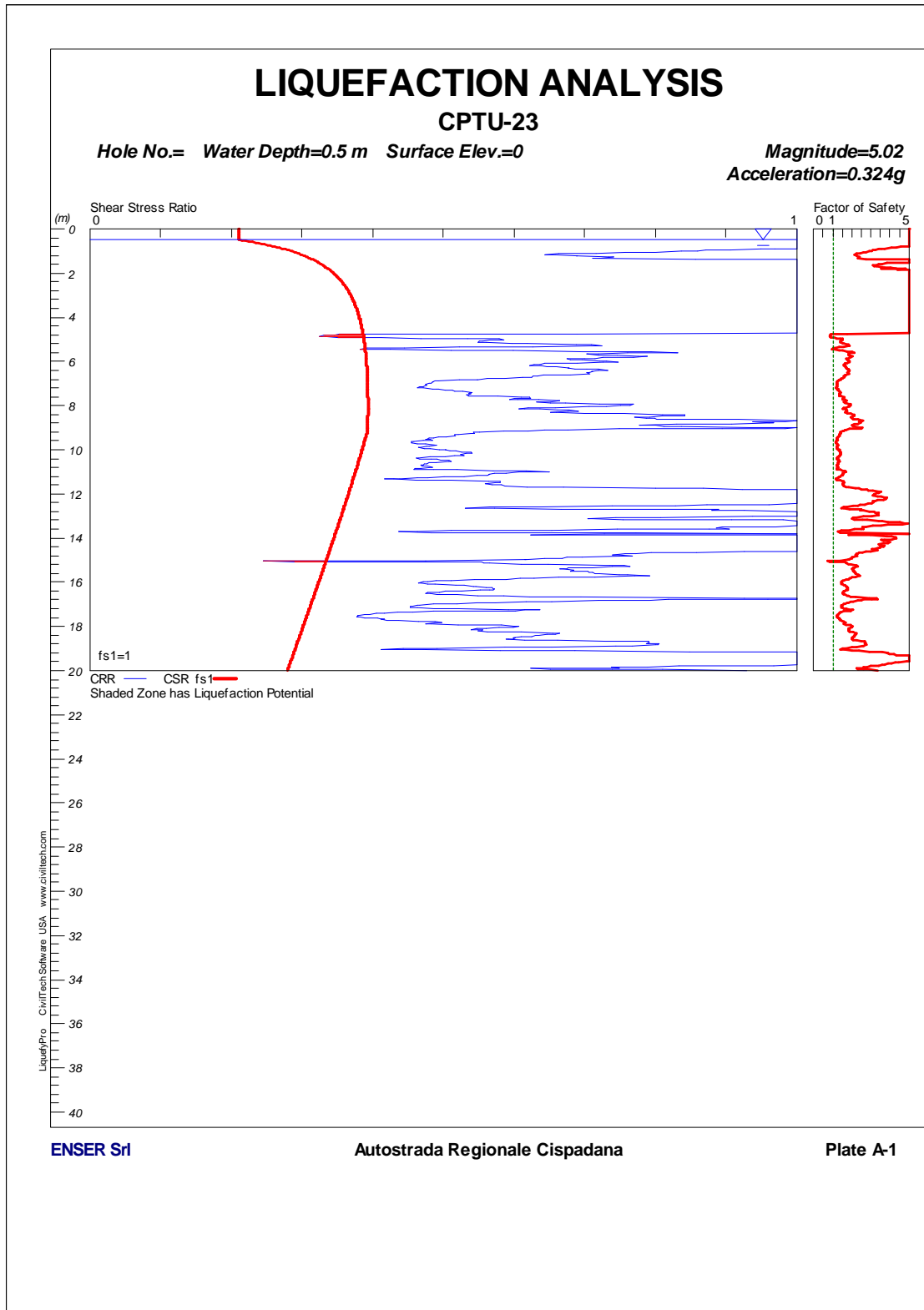
FIGURA 1-4: CPTU23 – VERIFICA A LIQUEFAZIONE.
