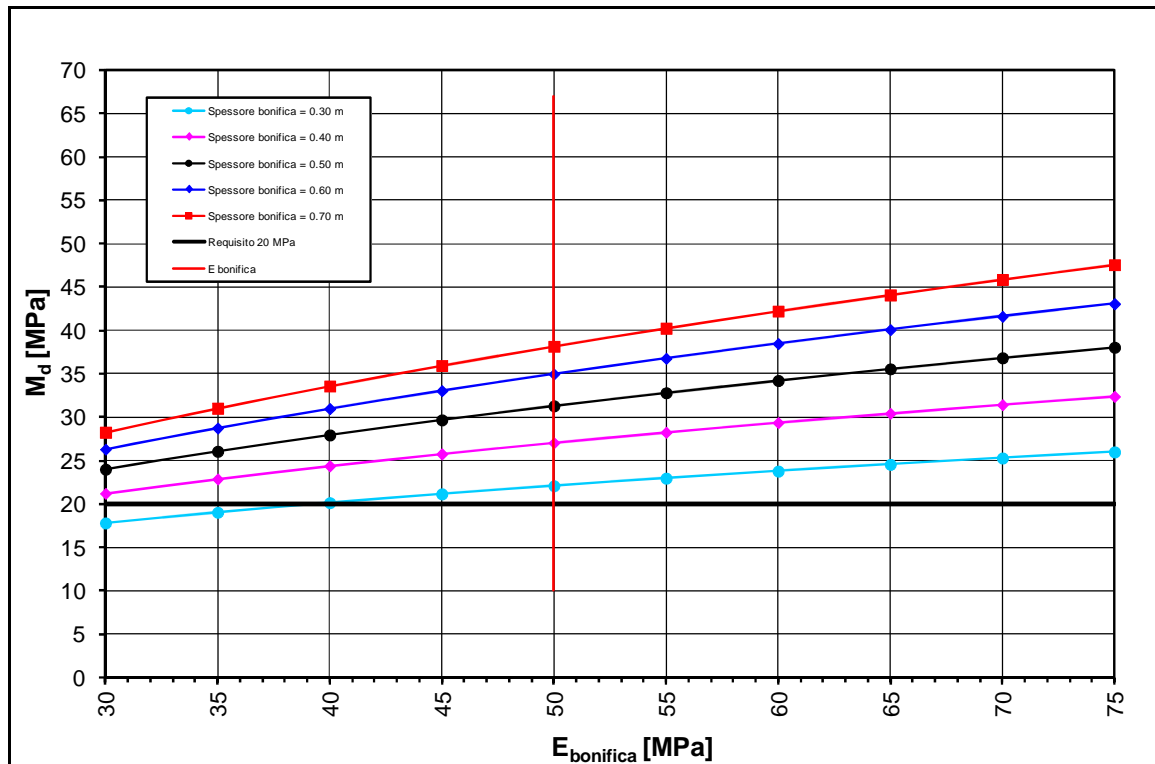
FIGURA 2-38: TRATTO 39 – DETERMINAZIONE SPESSORE DI BONIFICA.
