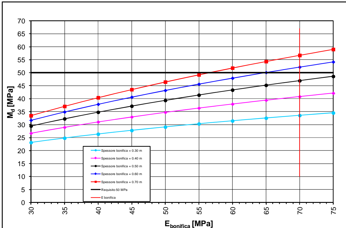
FIGURA 2-19: TRATTO 19 – DETERMINAZIONE SPESSORE DI BONIFICA.
