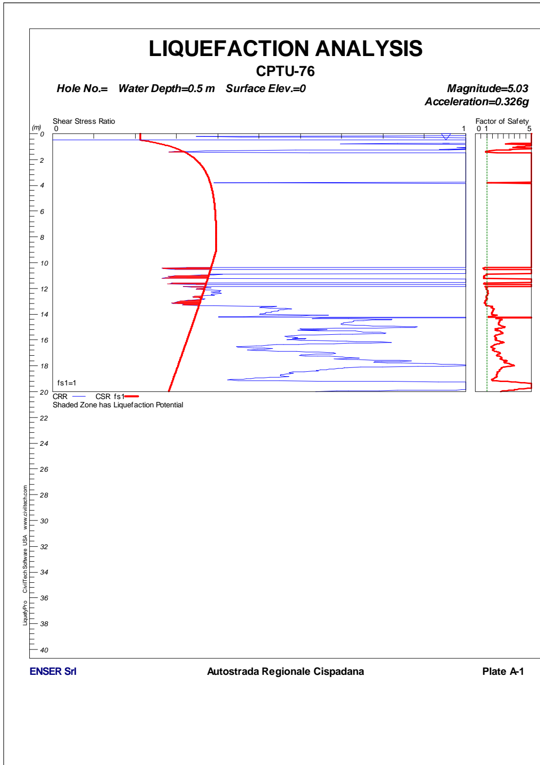
FIGURA 1-46: CPTU76 – VERIFICA A LIQUEFAZIONE.
