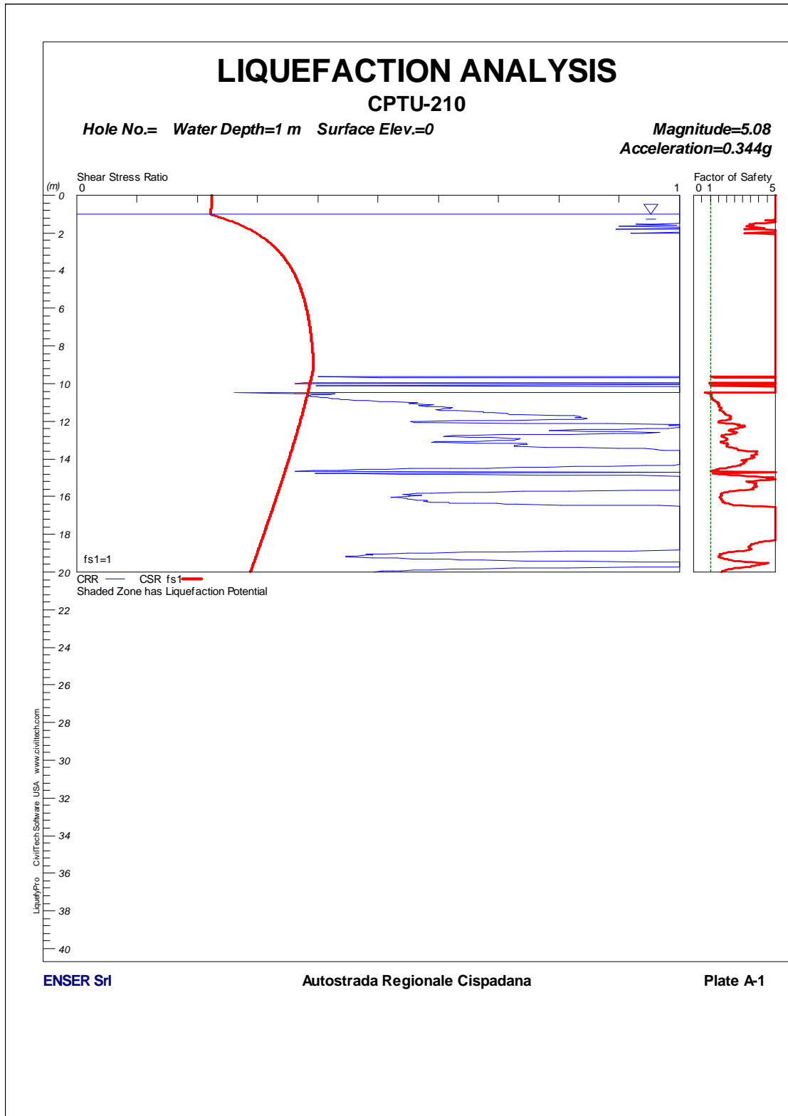
FIGURA 1-95: CPTU210 – VERIFICA A LIQUEFAZIONE.
