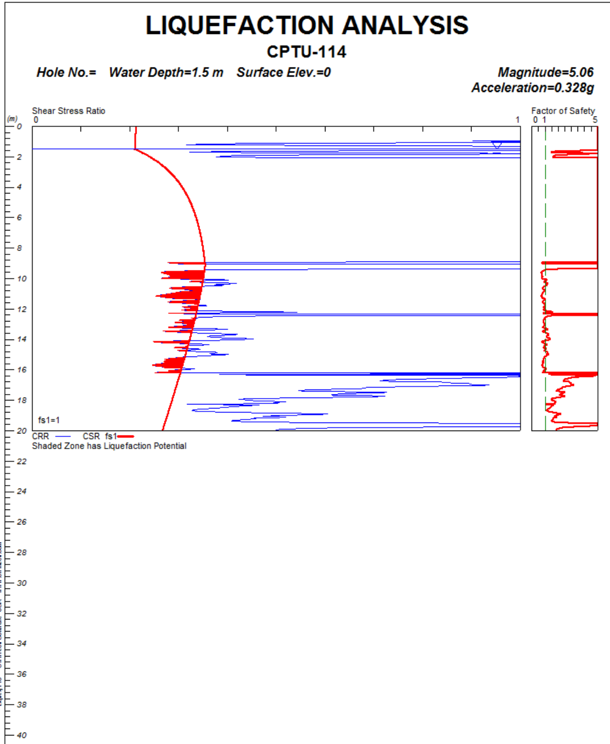
FIGURA 1-74: CPTU114 – VERIFICA A LIQUEFAZIONE.
