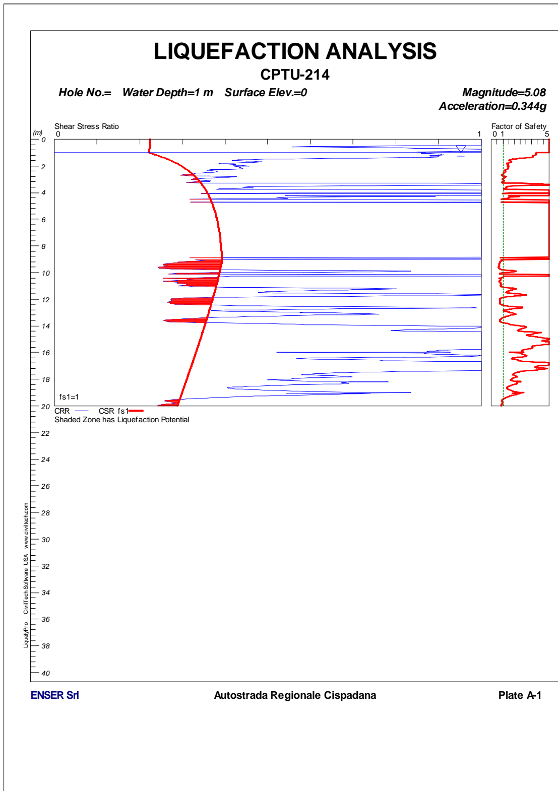
FIGURA 1-98: CPTU214 – Verifica a Liquefazione.
