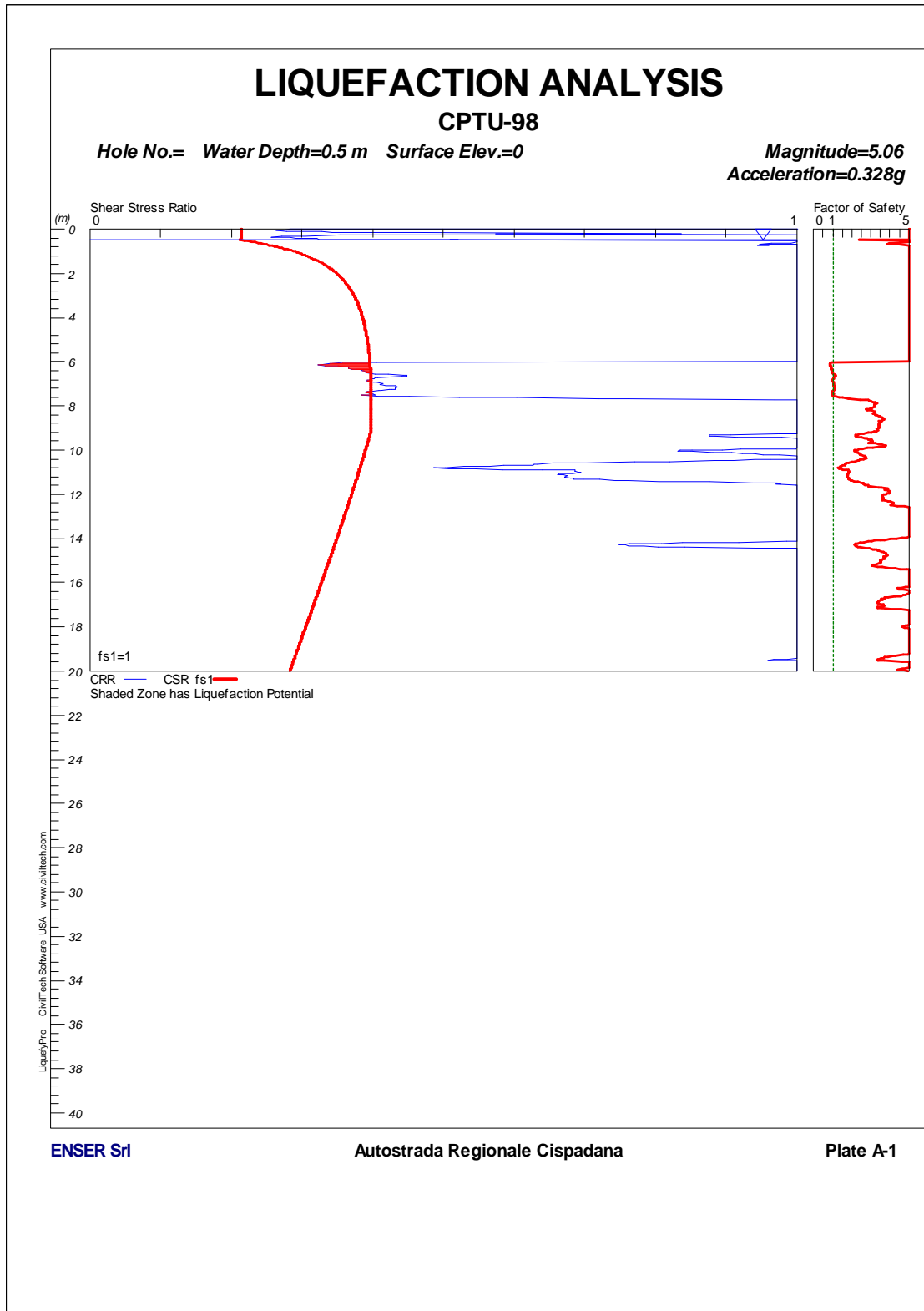
FIGURA 1-59: CPTU98 – VERIFICA A LIQUEFAZIONE.
