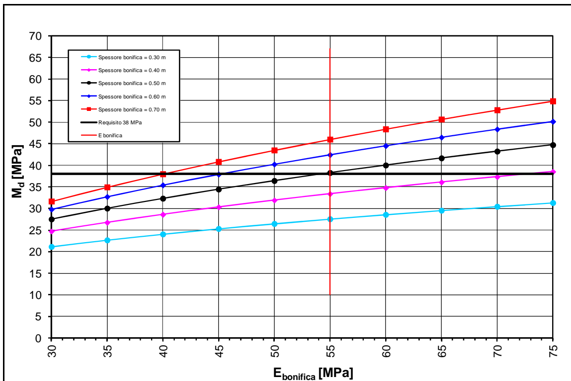
FIGURA 2-44: TRATTO 47 – DETERMINAZIONE SPESSORE DI BONIFICA.
