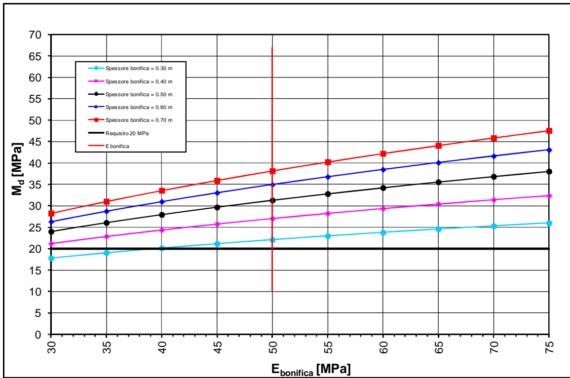
FIGURA 2-28: TRATTO 29 – DETERMINAZIONE SPESSORE DI BONIFICA.
