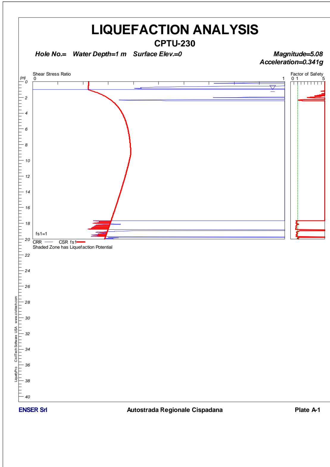
FIGURA 1-106: CPTU230 – VERIFICA A LIQUEFAZIONE.
