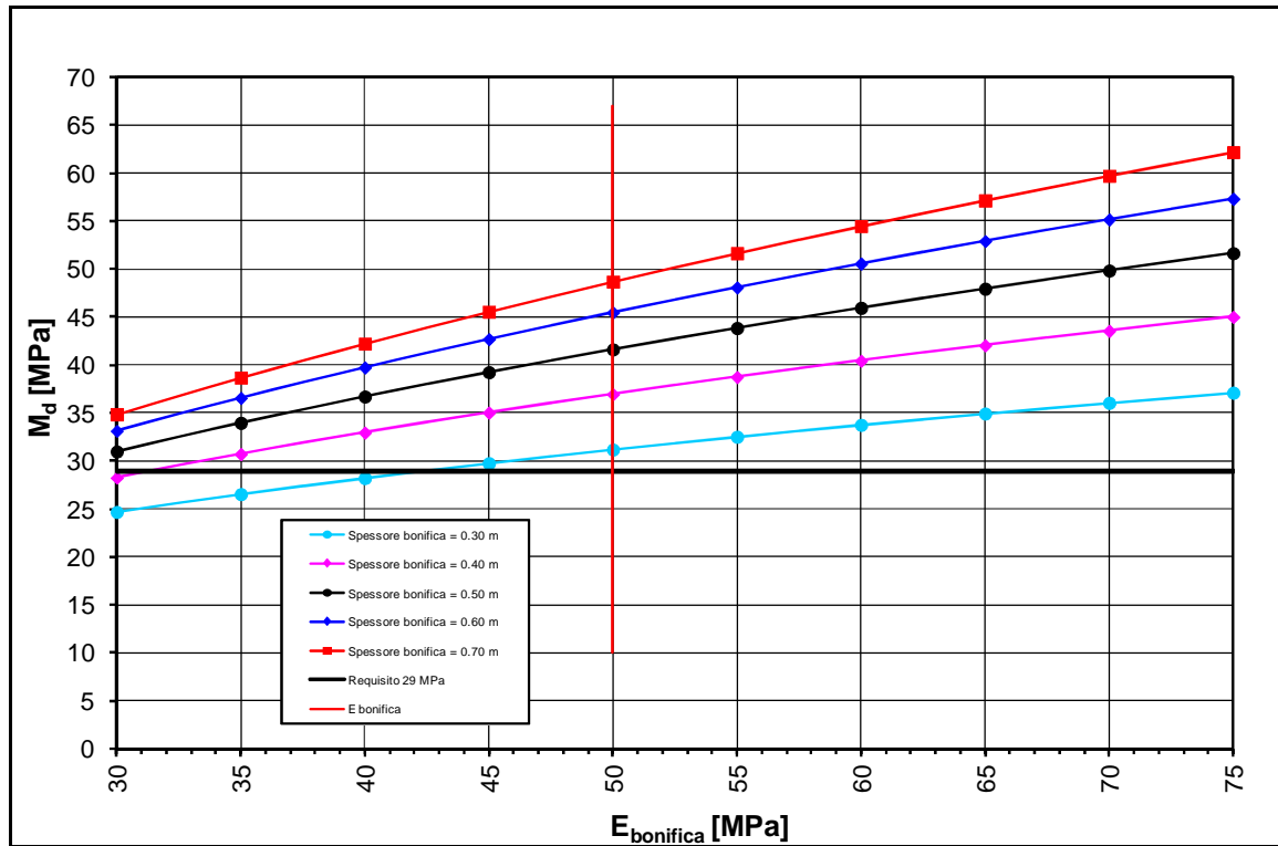
FIGURA 2-1: TRATTO 1 – DETERMINAZIONE SPESSORE DI BONIFICA.
