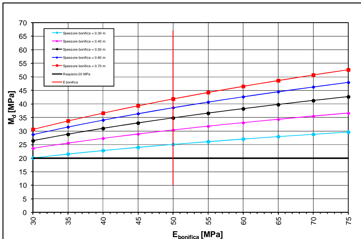
FIGURA 2-31: TRATTO 32 – DETERMINAZIONE SPESSORE DI BONIFICA.
