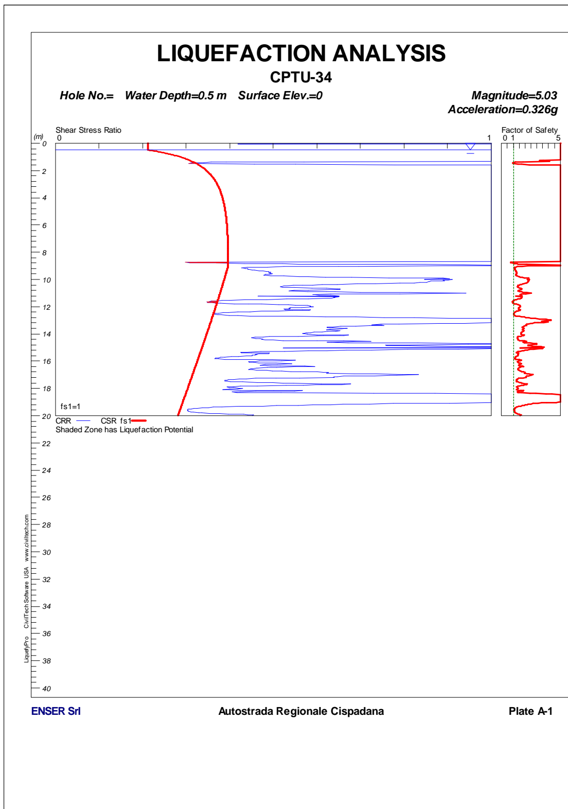
FIGURA 1-12: CPTU34 – VERIFICA A LIQUEFAZIONE.
