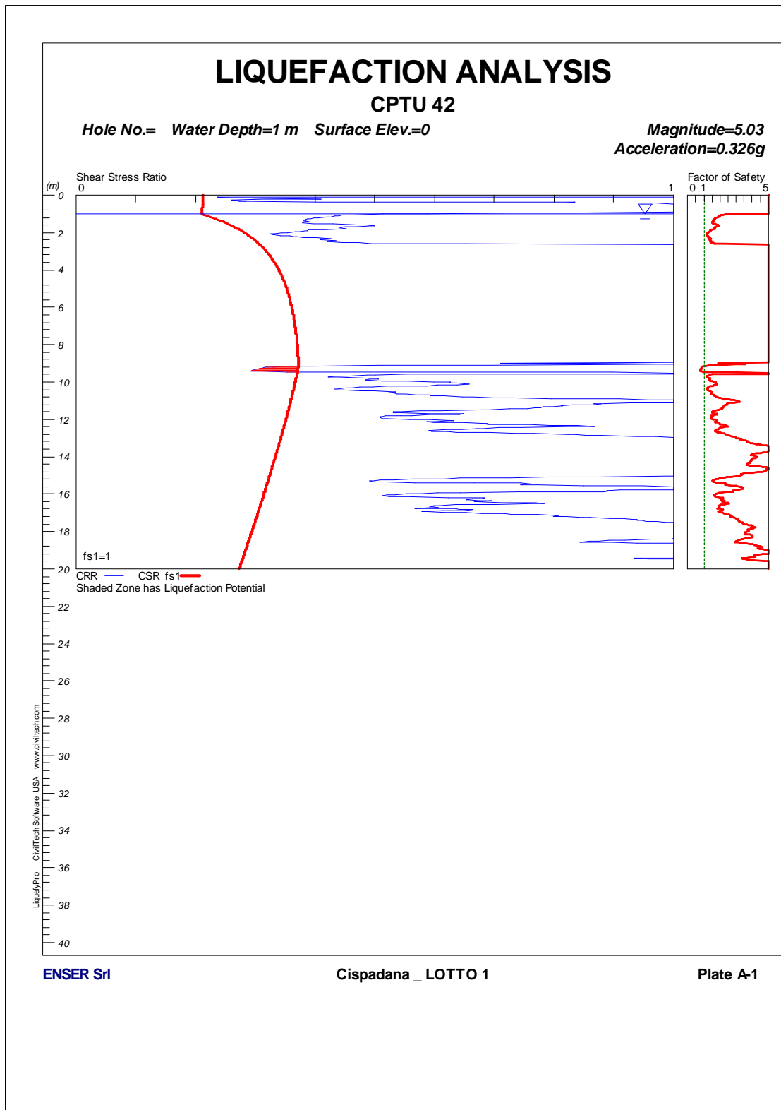
FIGURA 1-17: CPTU42 – VERIFICA A LIQUEFAZIONE.
