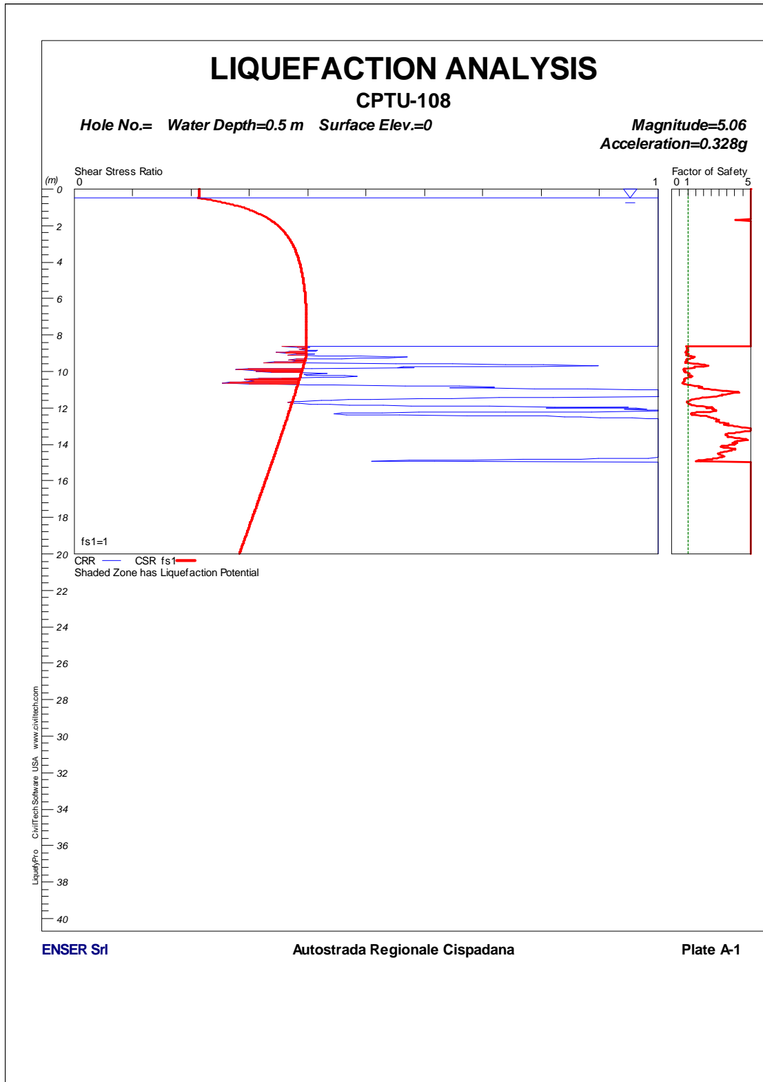
FIGURA 1-69: CPTU108 – VERIFICA A LIQUEFAZIONE.
