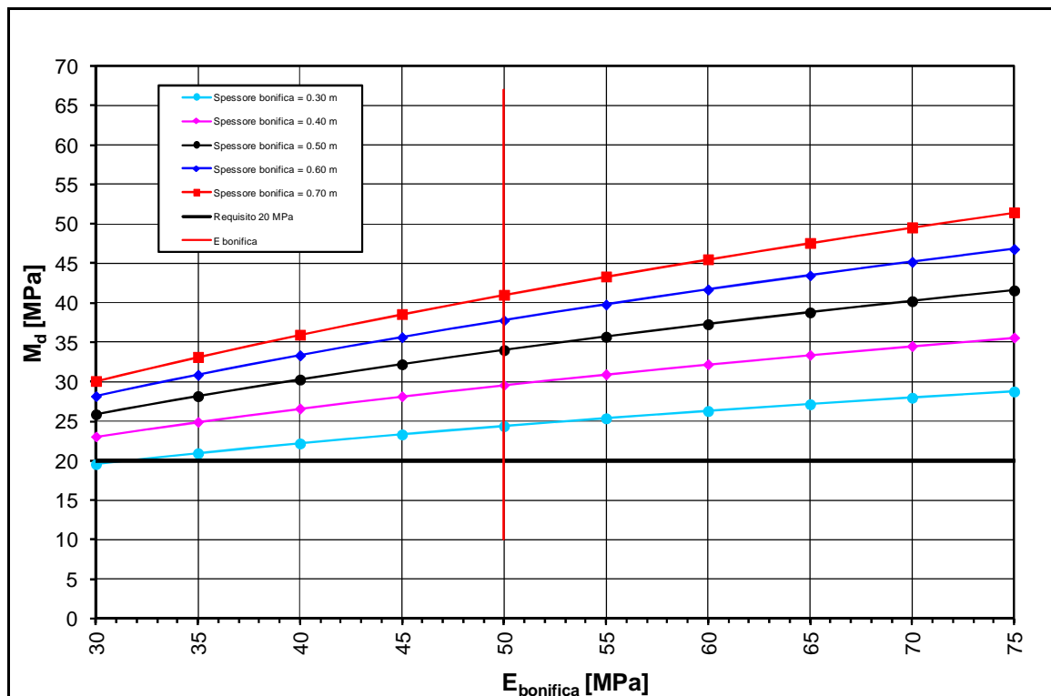
FIGURA 2-47: TRATTO 50 – DETERMINAZIONE SPESSORE DI BONIFICA.
