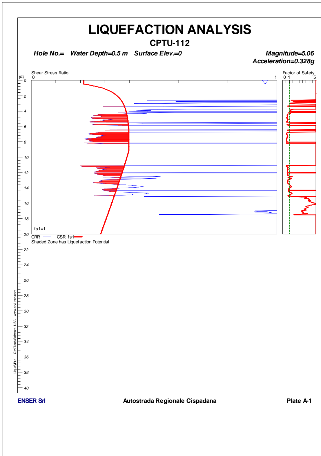
FIGURA 1-72: CPTU112 – VERIFICA A LIQUEFAZIONE.
