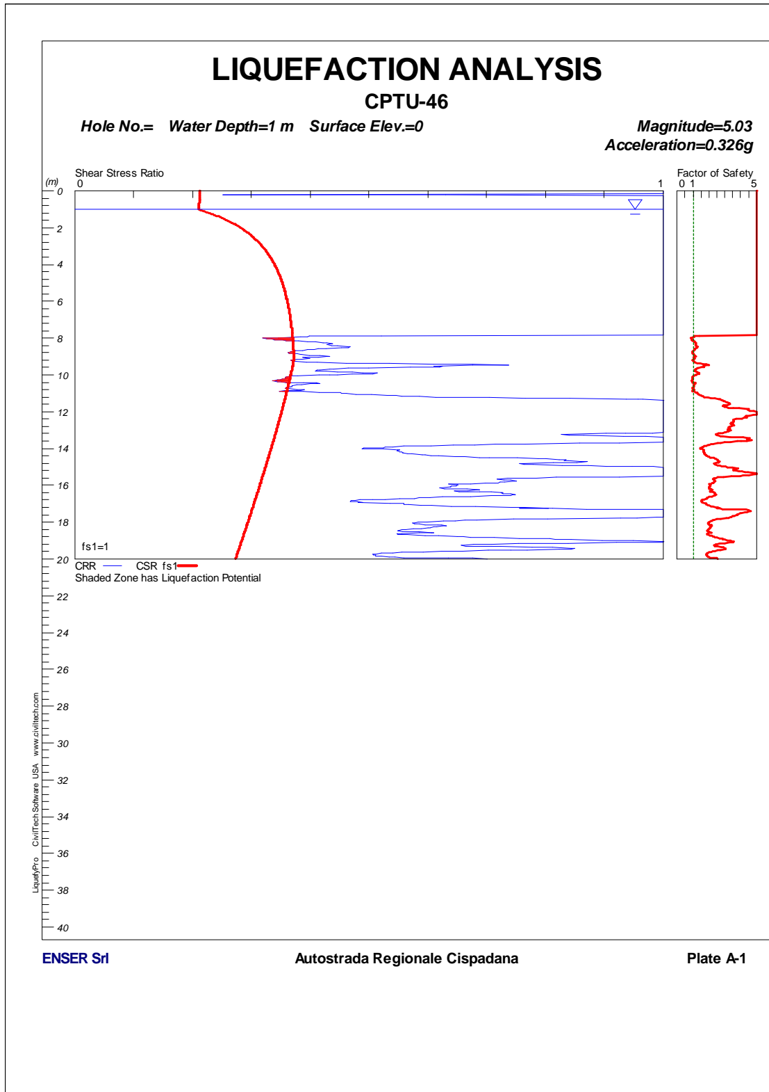
FIGURA 1-21: CPTU46 – VERIFICA A LIQUEFAZIONE.
