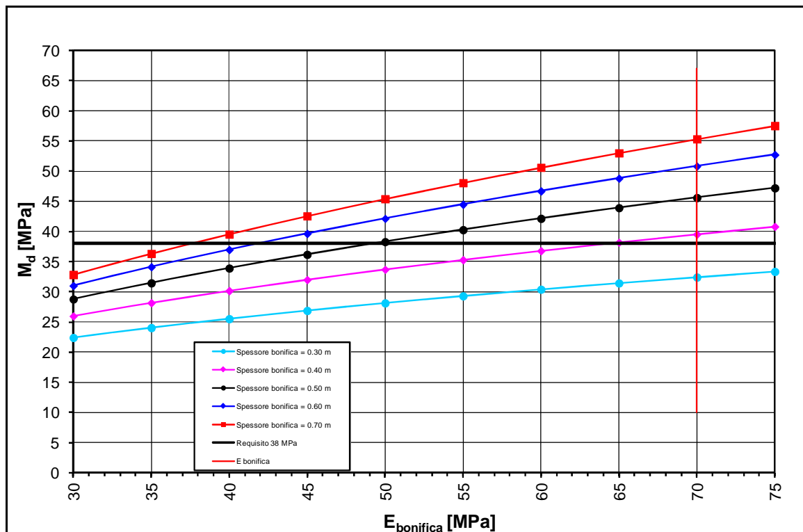
FIGURA 2-53: TRATTO 56 – DETERMINAZIONE SPESSORE DI BONIFICA.
