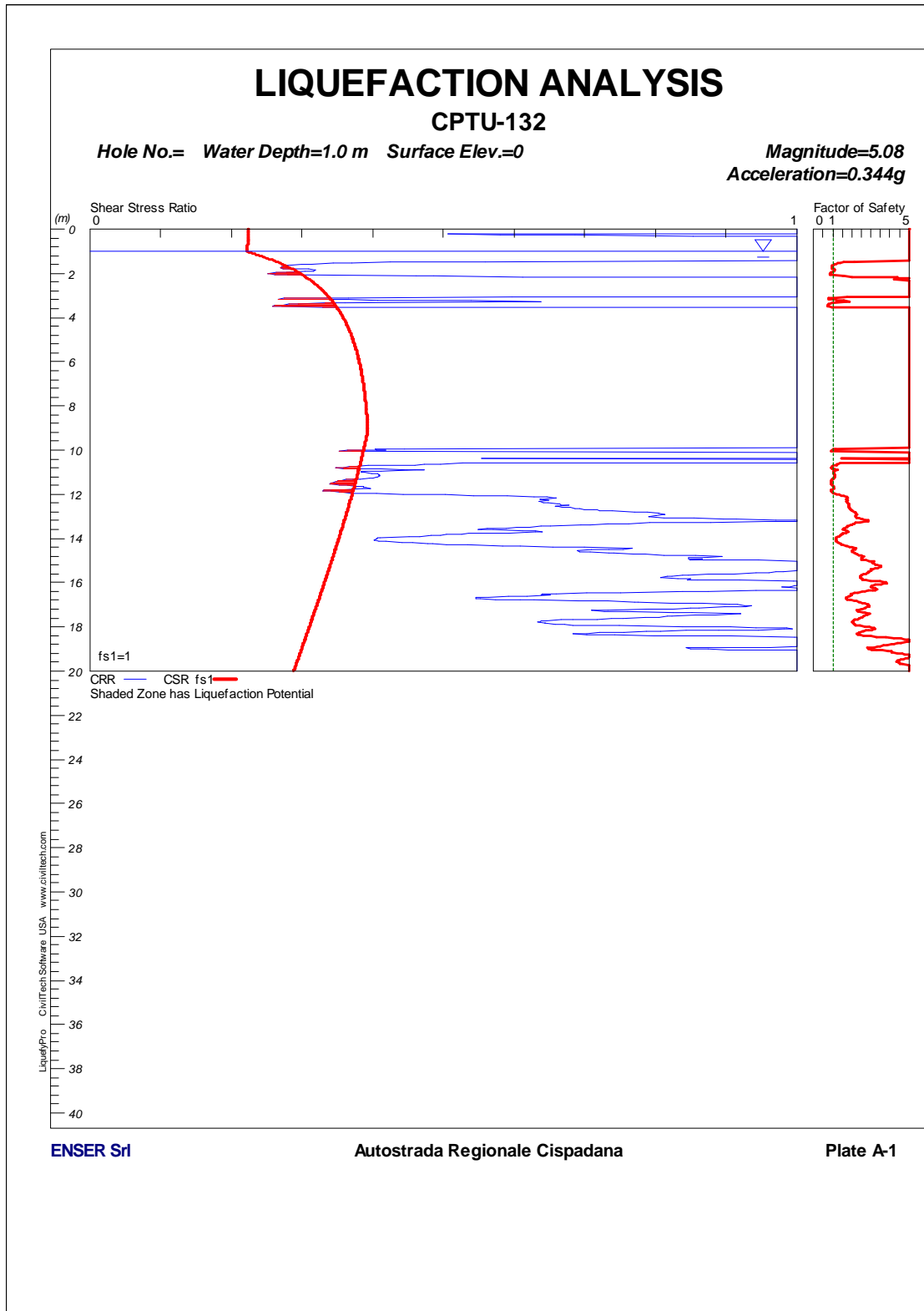
FIGURA 1-90: CPTU132 – VERIFICA A LIQUEFAZIONE.
