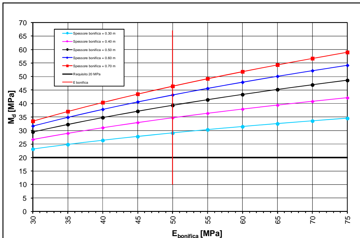
FIGURA 2-9: TRATTO 9 – DETERMINAZIONE SPESSORE DI BONIFICA.
