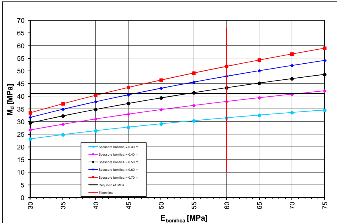
FIGURA 2-57: TRATTO 60 – DETERMINAZIONE SPESSORE DI BONIFICA.
