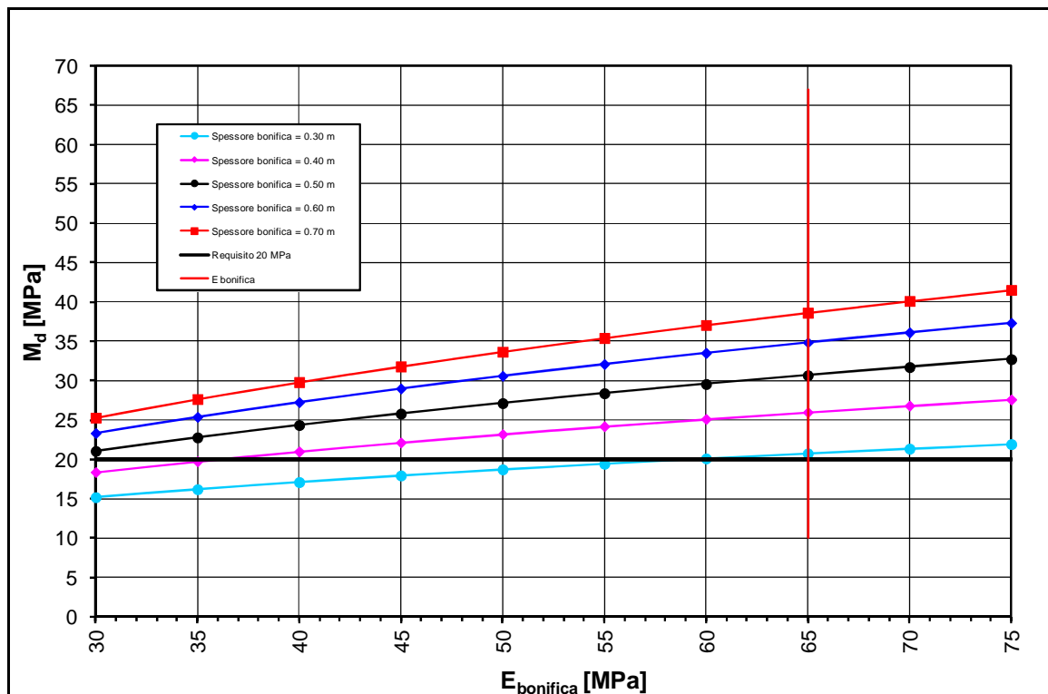
FIGURA 2-35: TRATTO 36 – DETERMINAZIONE SPESSORE DI BONIFICA.
