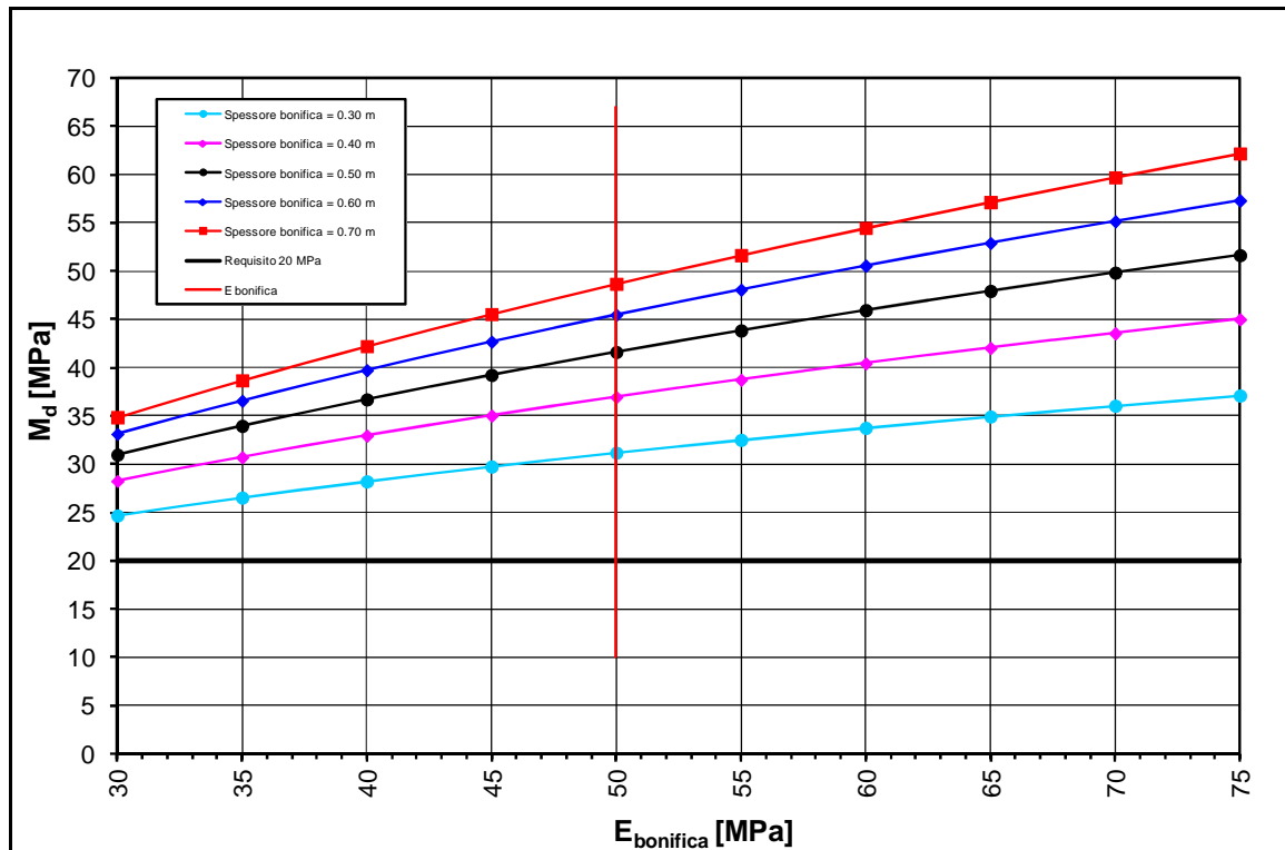
FIGURA 2-16: TRATTO 16 – DETERMINAZIONE SPESSORE DI BONIFICA.
