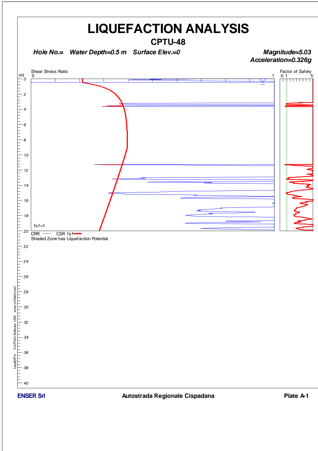
FIGURA 1-23: CPTU48 – VERIFICA A LIQUEFAZIONE.
