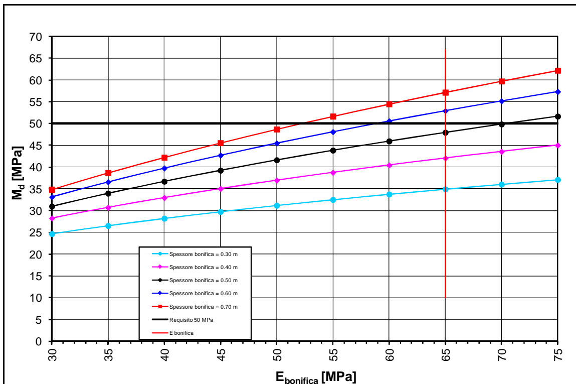
FIGURA 2-45: TRATTO 48 – DETERMINAZIONE SPESSORE DI BONIFICA.
