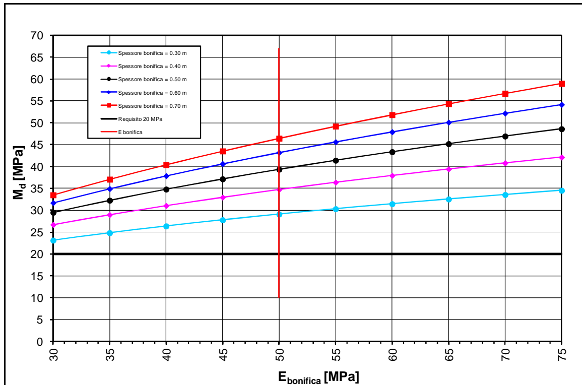
FIGURA 2-58: TRATTO 61 – DETERMINAZIONE SPESSORE DI BONIFICA.
