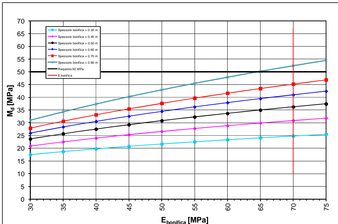
FIGURA 2-11: TRATTO 10A – DETERMINAZIONE SPESSORE DI BONIFICA.
