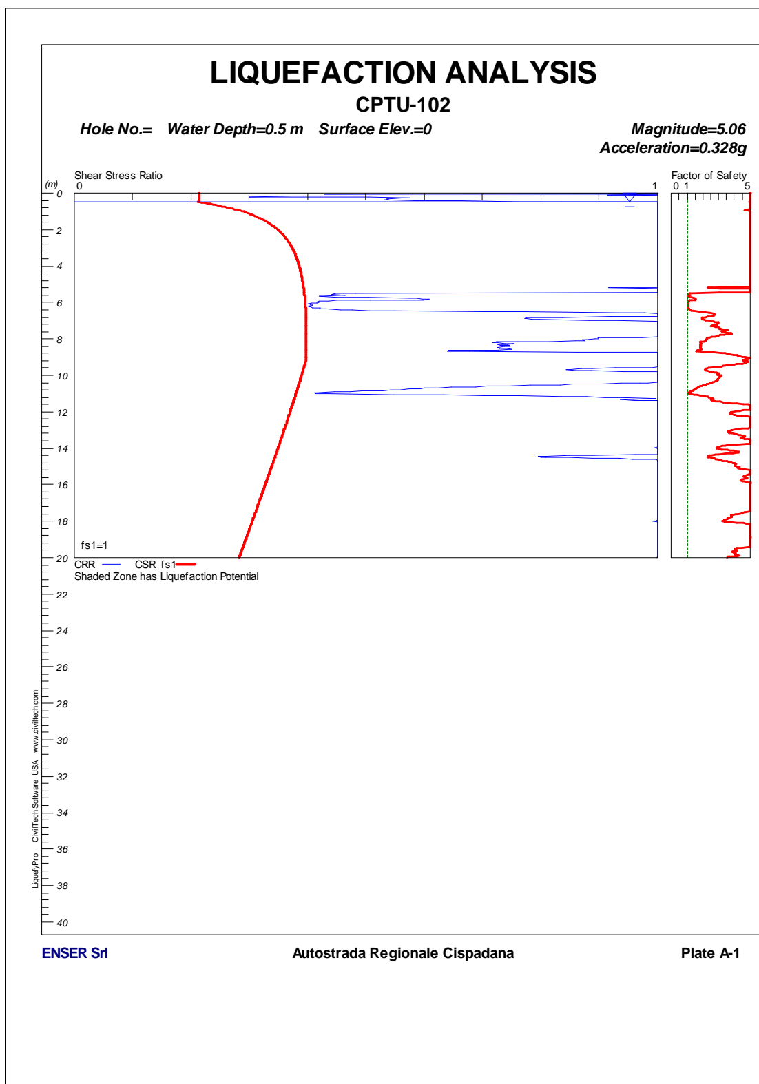
FIGURA 1-63: CPTU102 – VERIFICA A LIQUEFAZIONE.
