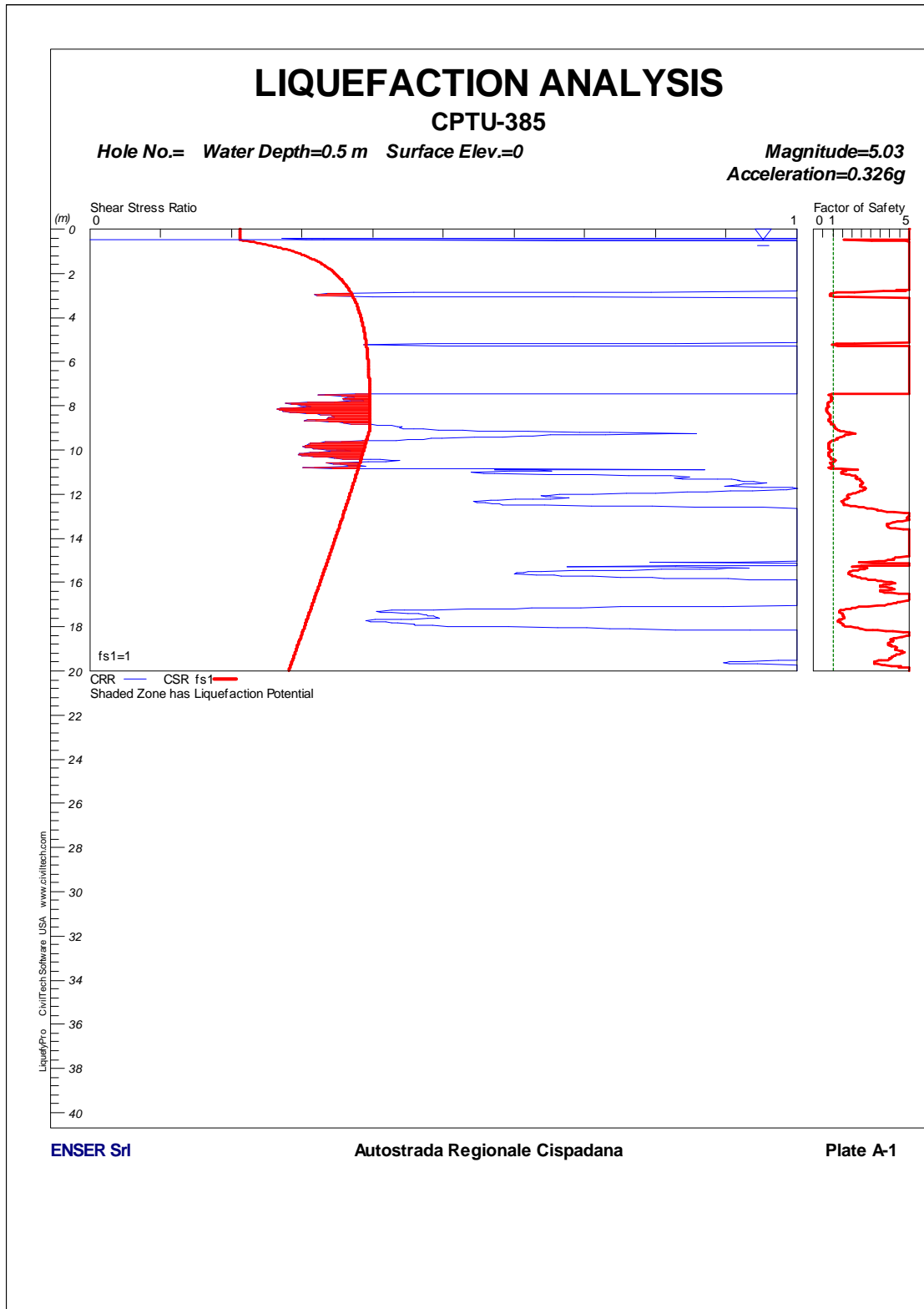
FIGURA 1-109: CPTU385 – VERIFICA A LIQUEFAZIONE.
