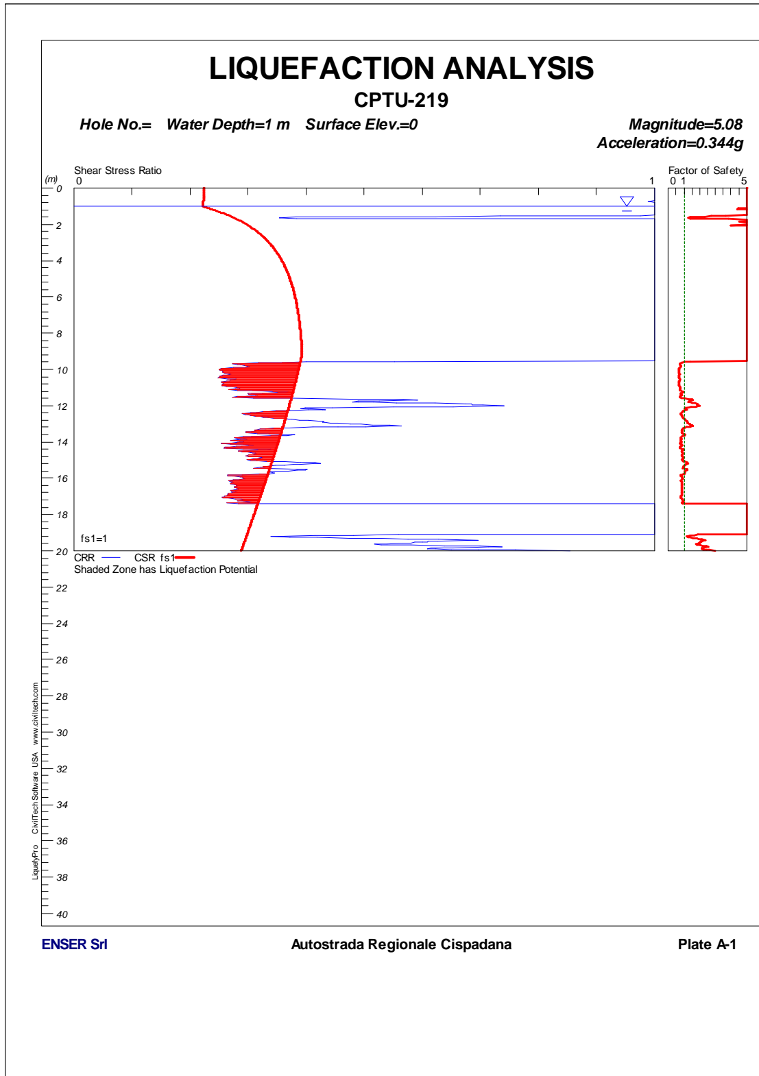
FIGURA 1-102: CPTU219 – VERIFICA A LIQUEFAZIONE.
