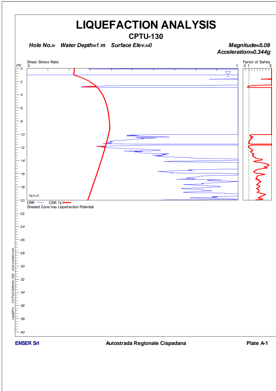
FIGURA 1-88: CPTU130 – VERIFICA A LIQUEFAZIONE.
