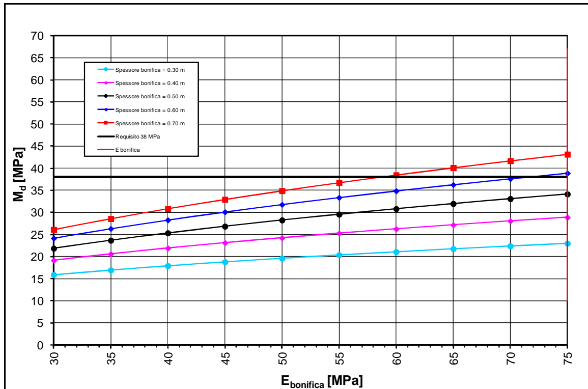
FIGURA 2-26: TRATTO 27 – DETERMINAZIONE SPESSORE DI BONIFICA.
