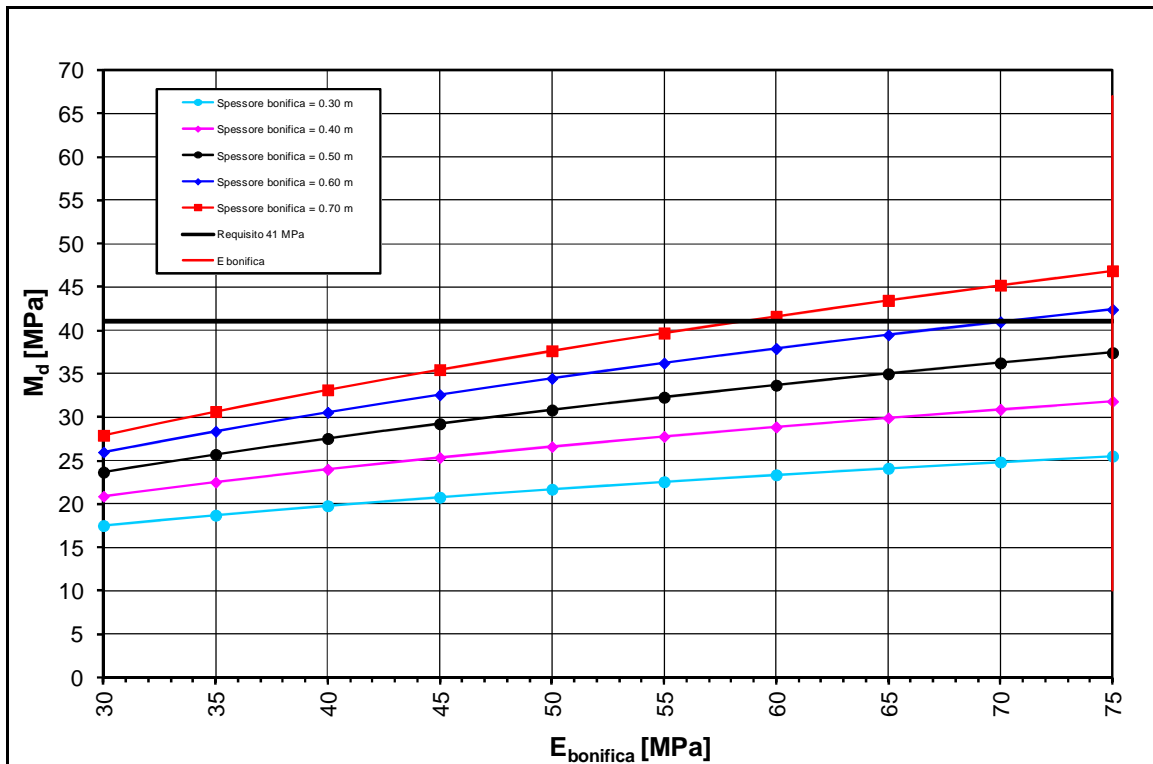
FIGURA 2-10: TRATTO 10 – DETERMINAZIONE SPESSORE DI BONIFICA.
