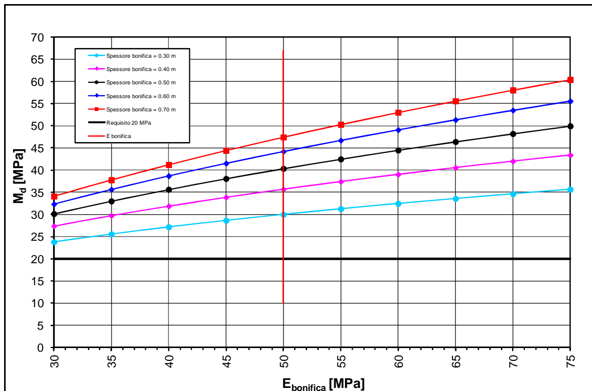
FIGURA 2-21: TRATTO 22 – DETERMINAZIONE SPESSORE DI BONIFICA.
