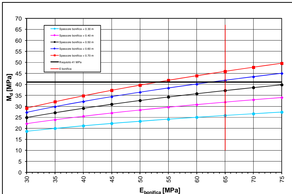
FIGURA 2-33: TRATTO 34 – DETERMINAZIONE SPESSORE DI BONIFICA.
