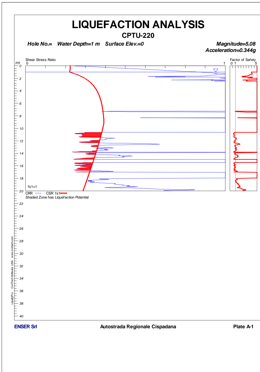
FIGURA 1-103: CPTU220 – VERIFICA A LIQUEFAZIONE.
