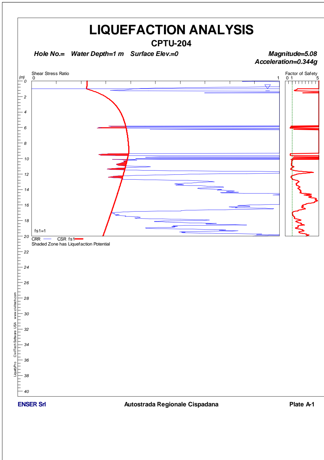
FIGURA 1-93: CPTU204 – VERIFICA A LIQUEFAZIONE.
