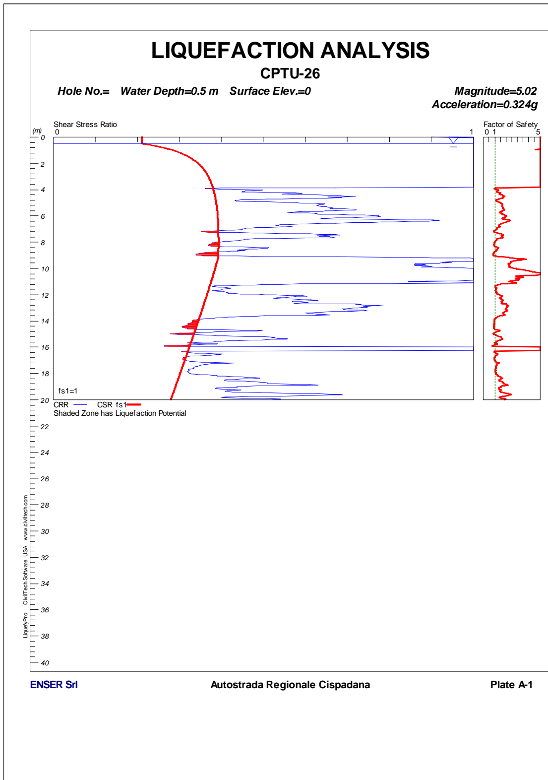
FIGURA 1-6: CPTU26 – VERIFICA A LIQUEFAZIONE.
