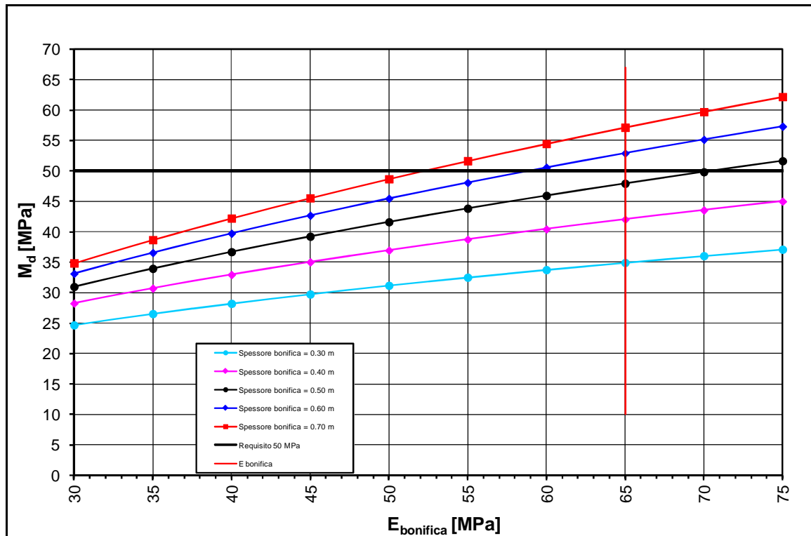
FIGURA 2-2: TRATTO 2 – DETERMINAZIONE SPESSORE DI BONIFICA.
