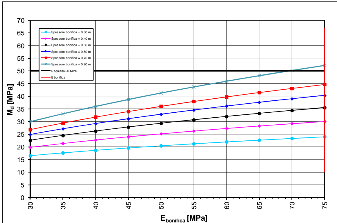
FIGURA 2-29: TRATTO 30 – DETERMINAZIONE SPESSORE DI BONIFICA.
