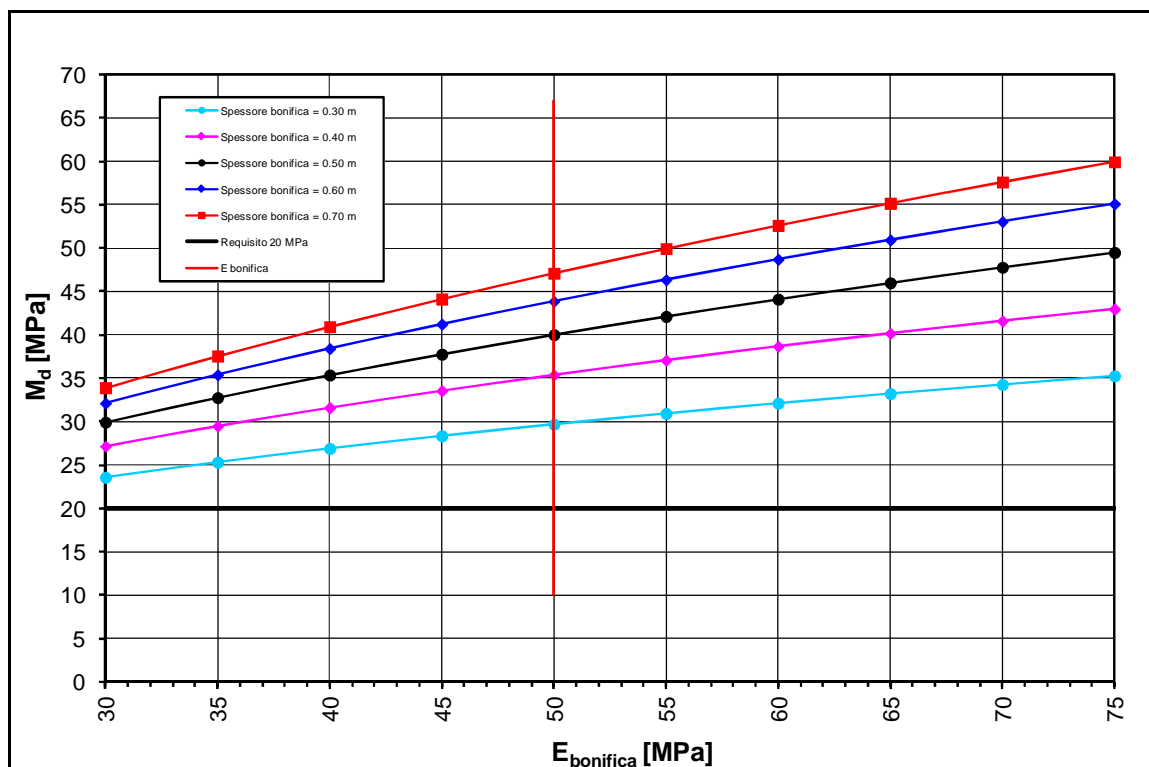
FIGURA 2-25: TRATTO 26 – DETERMINAZIONE SPESSORE DI BONIFICA.
