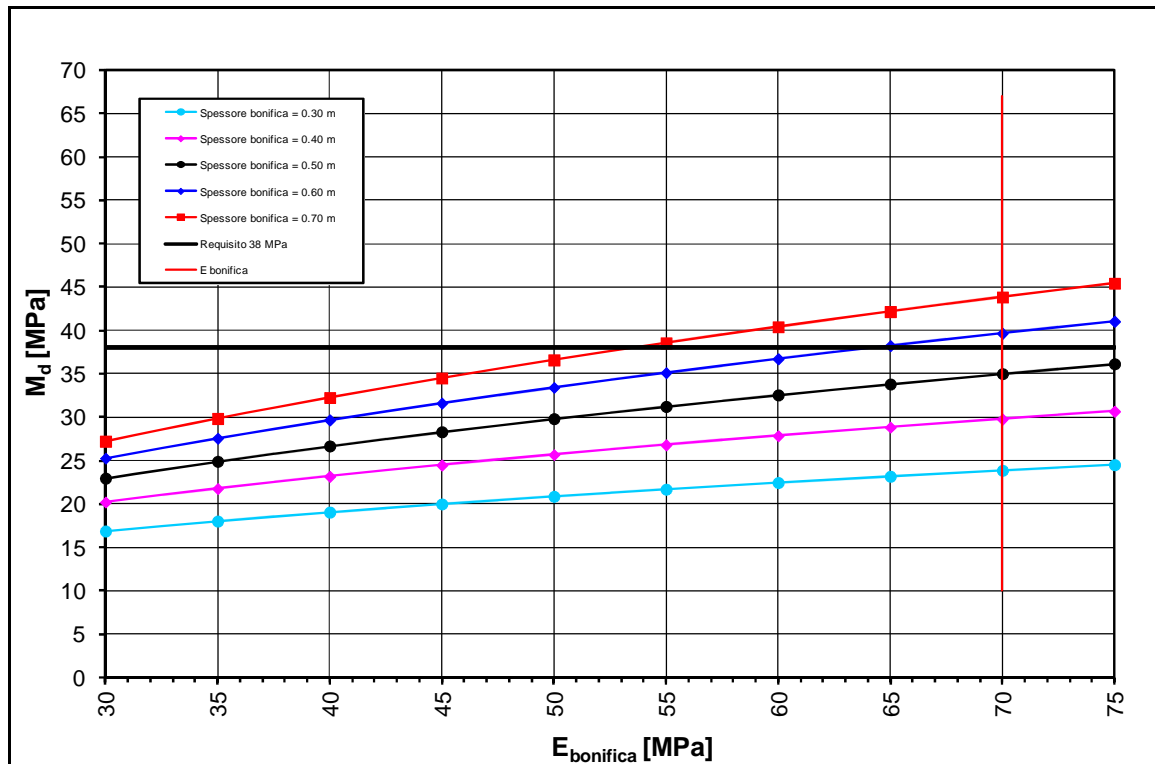
FIGURA 2-46: TRATTO 49 – DETERMINAZIONE SPESSORE DI BONIFICA.
