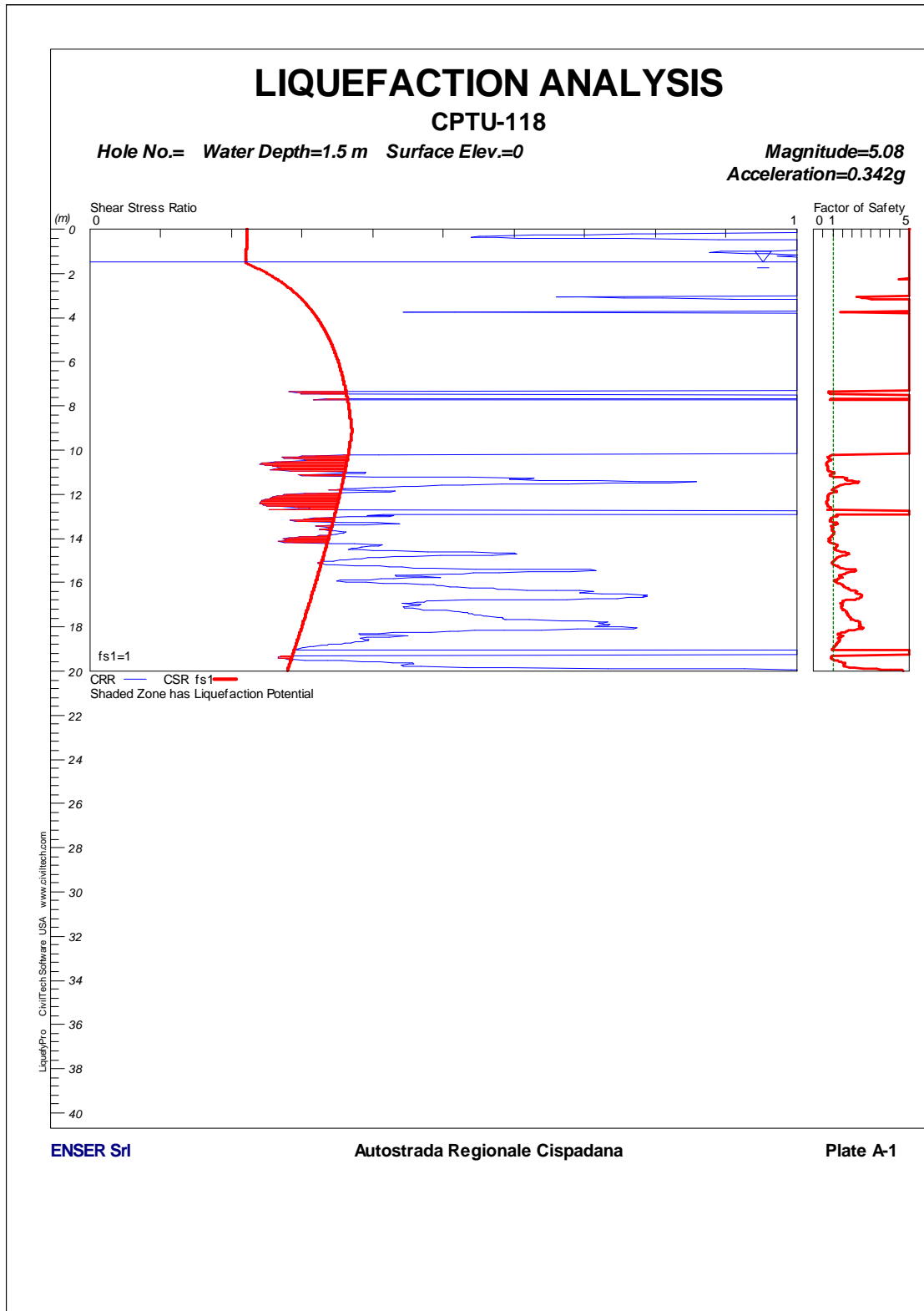
FIGURA 1-78: CPTU118 – VERIFICA A LIQUEFAZIONE.
