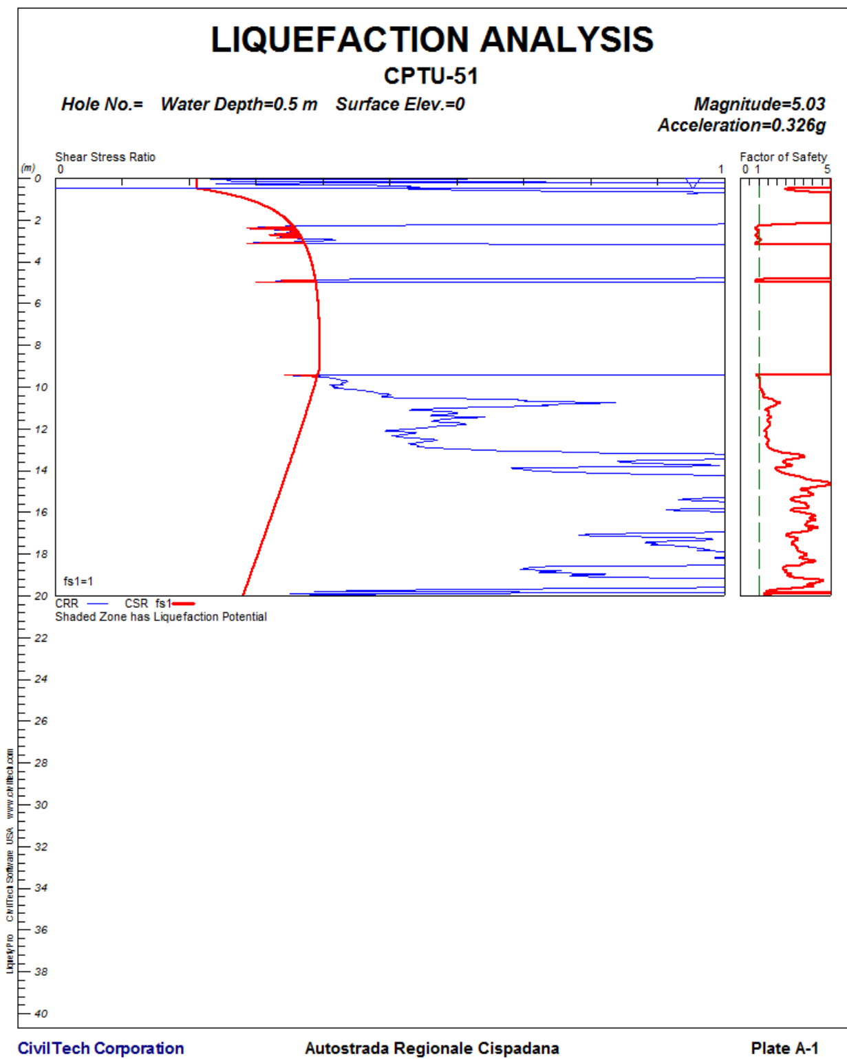
FIGURA 1-26: CPTU51 – VERIFICA A LIQUEFAZIONE.
