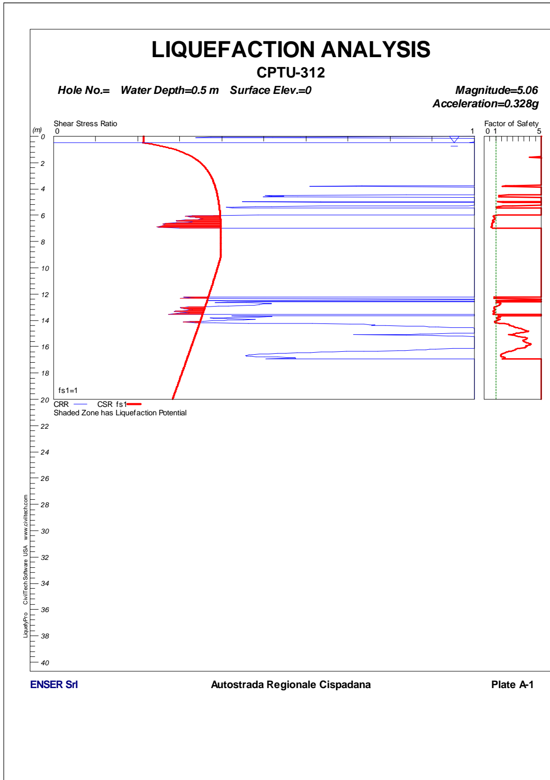
FIGURA 1-108: CPTU312 – VERIFICA A LIQUEFAZIONE.
