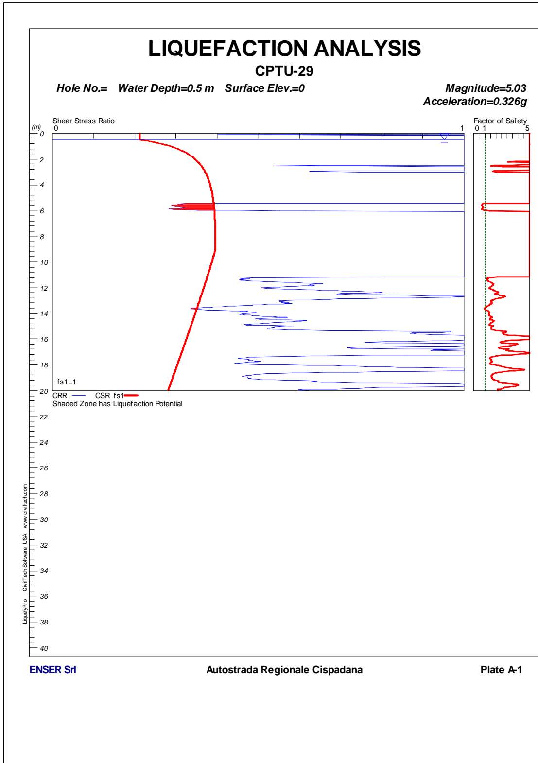
FIGURA 1-7: CPTU29 – VERIFICA A LIQUEFAZIONE.
