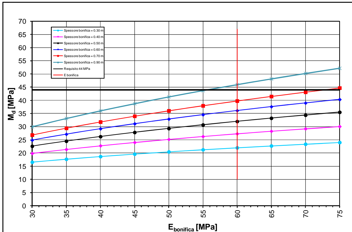
FIGURA 2-48: TRATTO 51 – DETERMINAZIONE SPESSORE DI BONIFICA.
