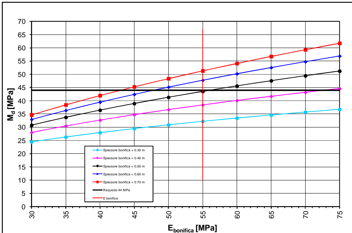
FIGURA 2-22: TRATTO 23 – DETERMINAZIONE SPESSORE DI BONIFICA.
