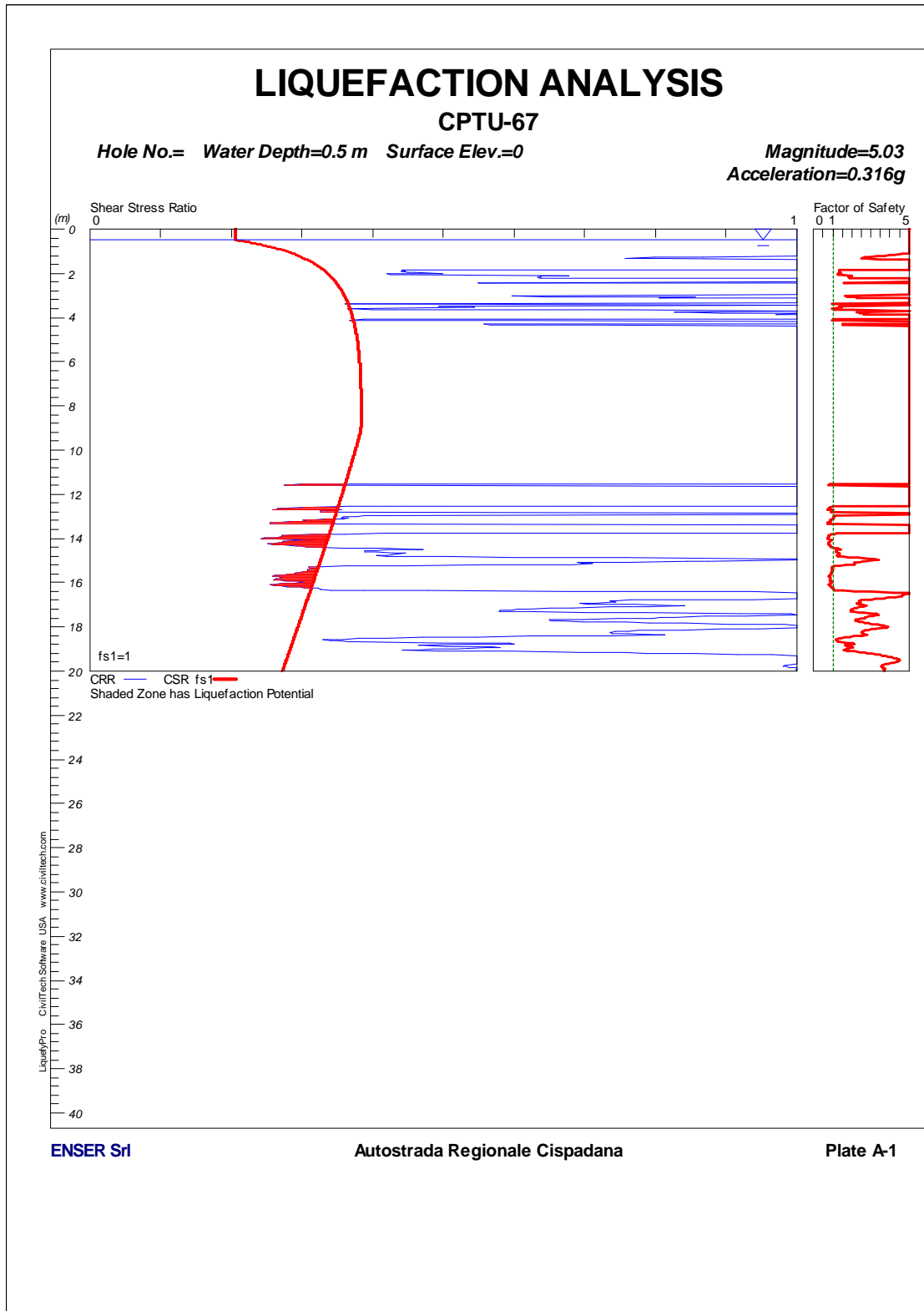
FIGURA 1-42: CPTU67 – VERIFICA A LIQUEFAZIONE.
