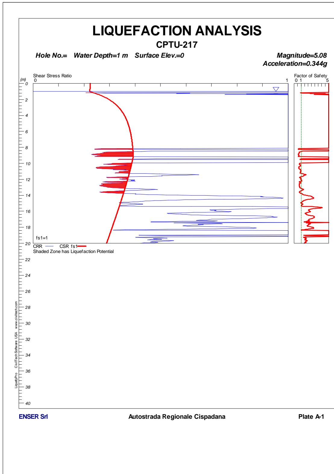
FIGURA 1-101: CPTU217 – VERIFICA A LIQUEFAZIONE.
