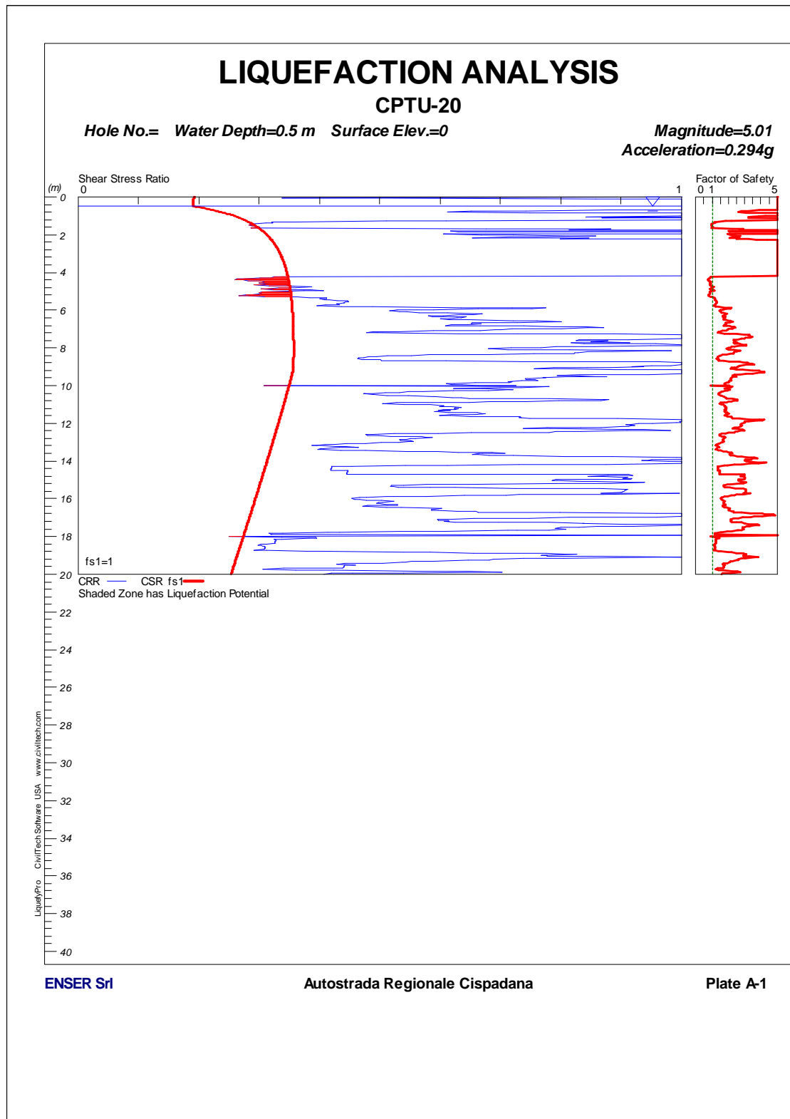
FIGURA 1-1: CPTU20 – VERIFICA A LIQUEFAZIONE.
