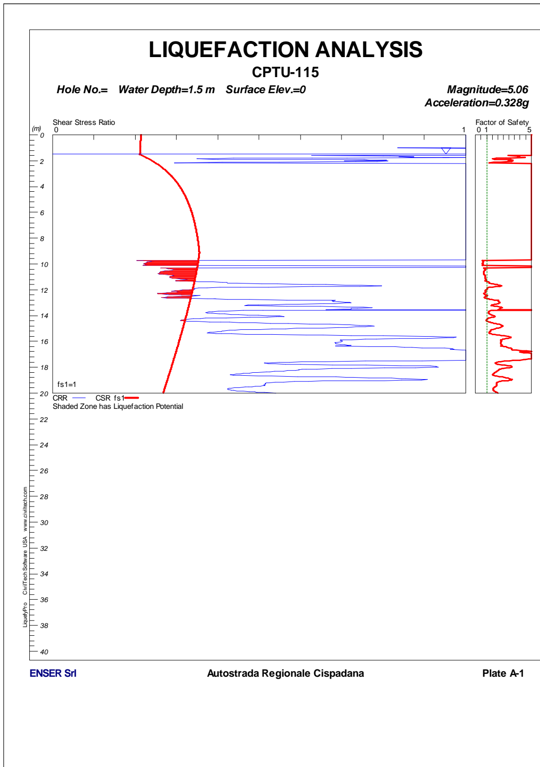
FIGURA 1-75: CPTU115 – VERIFICA A LIQUEFAZIONE.
