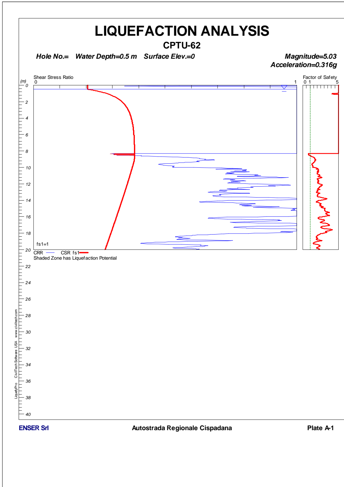
FIGURA 1-37: CPTU62 – VERIFICA A LIQUEFAZIONE.
