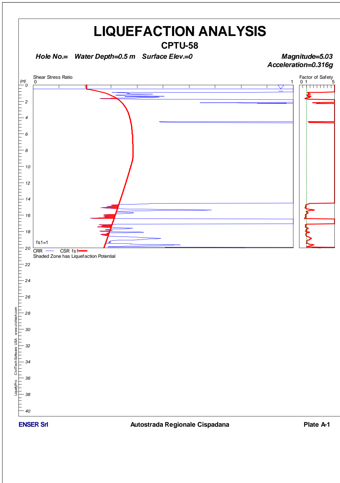
FIGURA 1-33: CPTU58 – VERIFICA A LIQUEFAZIONE.
