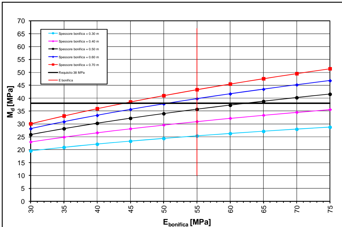
FIGURA 2-40: TRATTO 41 – DETERMINAZIONE SPESSORE DI BONIFICA.
