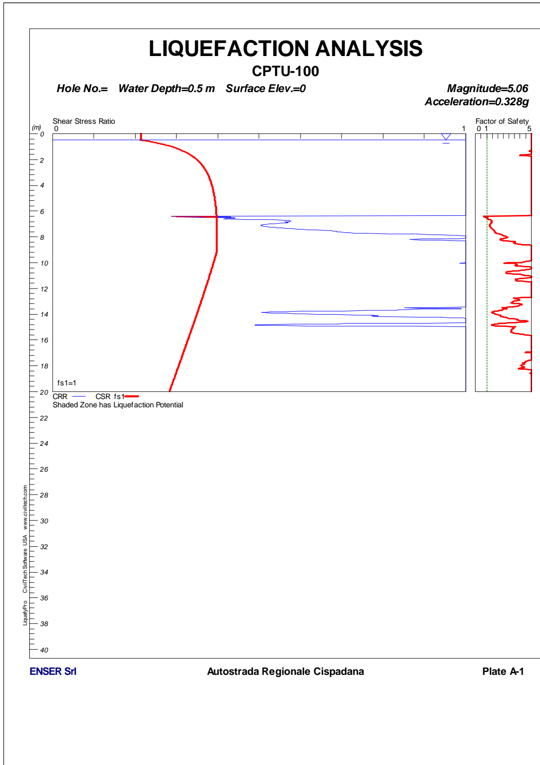
FIGURA 1-61: CPTU100 – VERIFICA A LIQUEFAZIONE.
