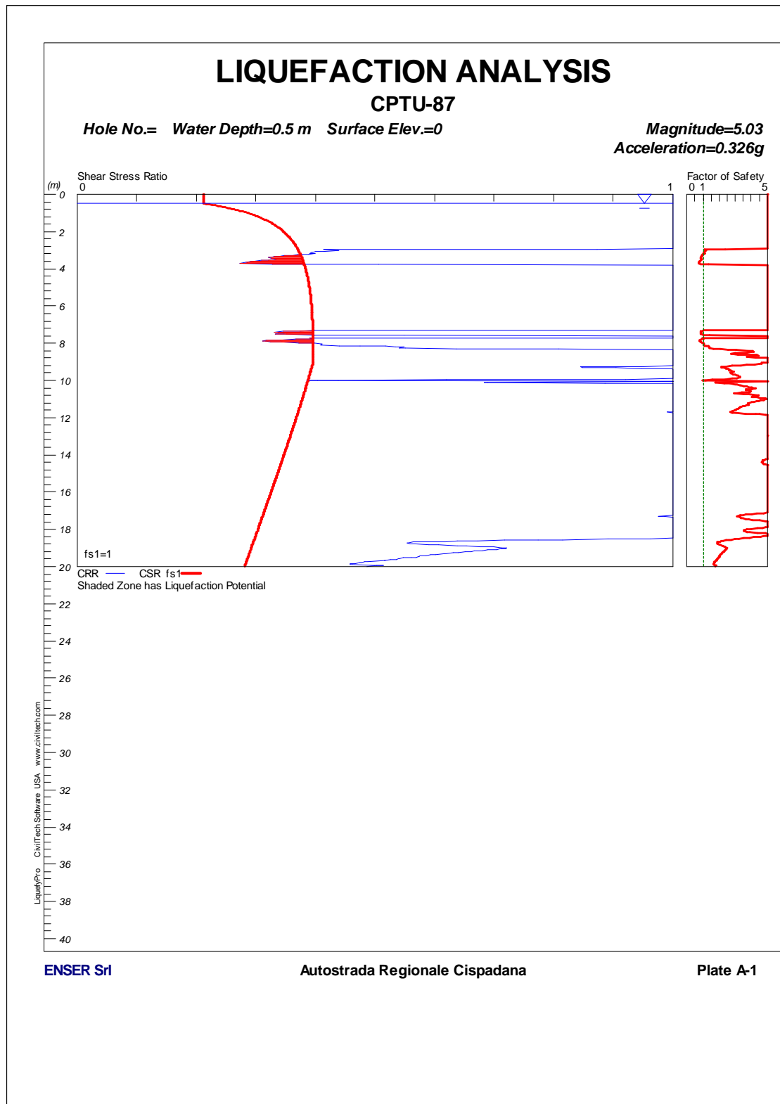
FIGURA 1-52: CPTU87 – VERIFICA A LIQUEFAZIONE.
