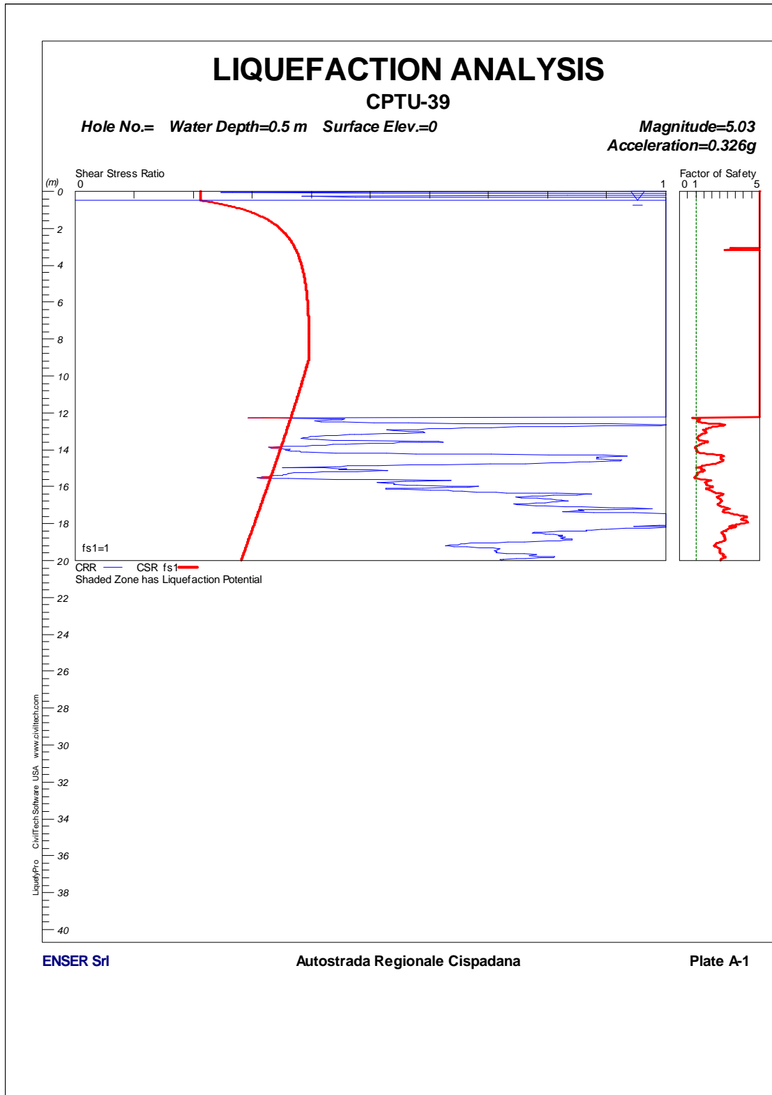
FIGURA 1-14: CPTU39 – VERIFICA A LIQUEFAZIONE.
