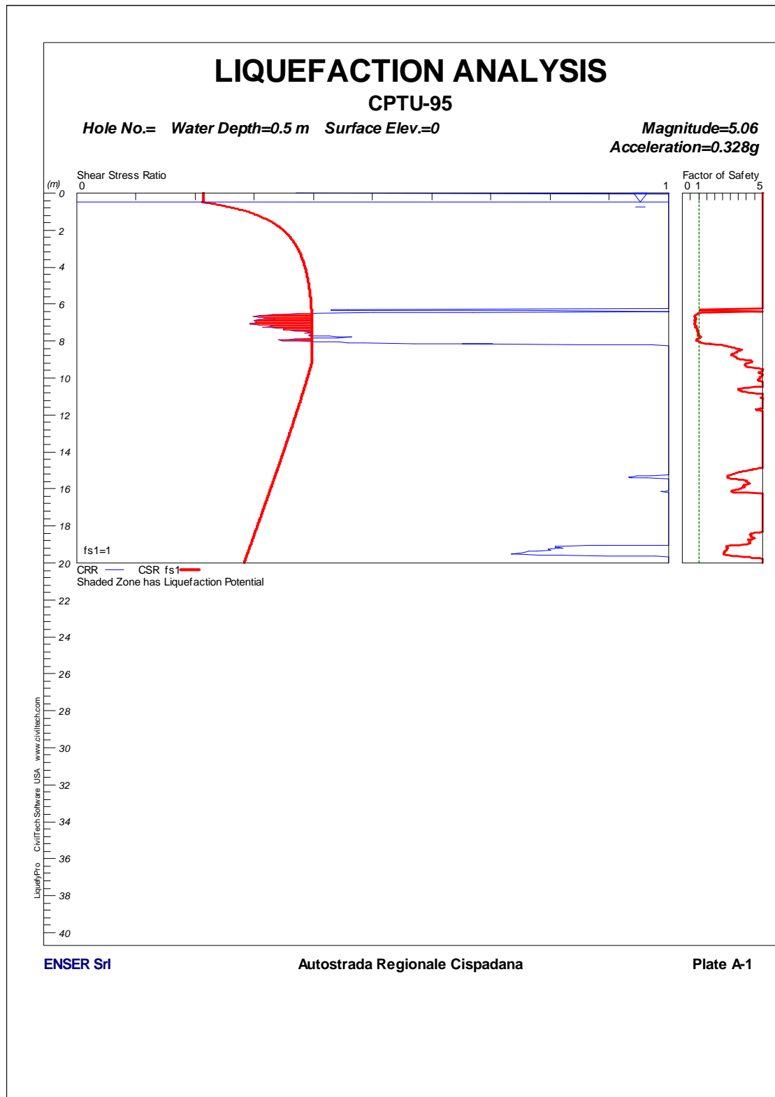
FIGURA 1-57: CPTU95 – VERIFICA A LIQUEFAZIONE.
