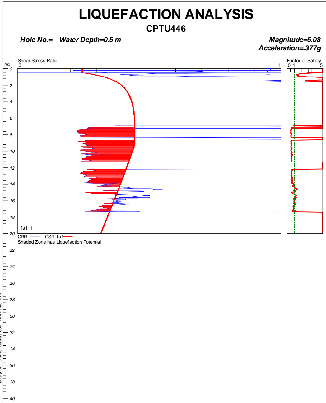
FIGURA 1-110: CPTU446 – VERIFICA A LIQUEFAZIONE.
