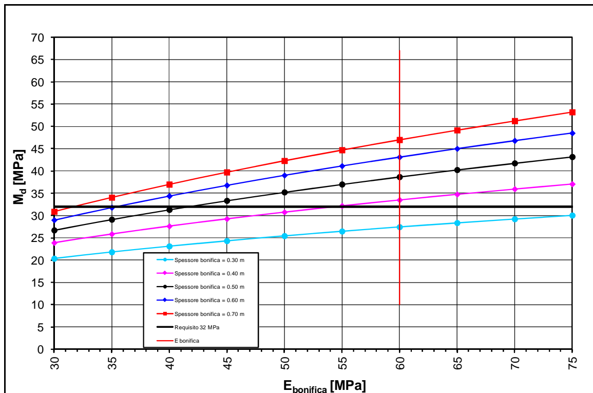
FIGURA 2-55: TRATTO 58 – DETERMINAZIONE SPESSORE DI BONIFICA.
