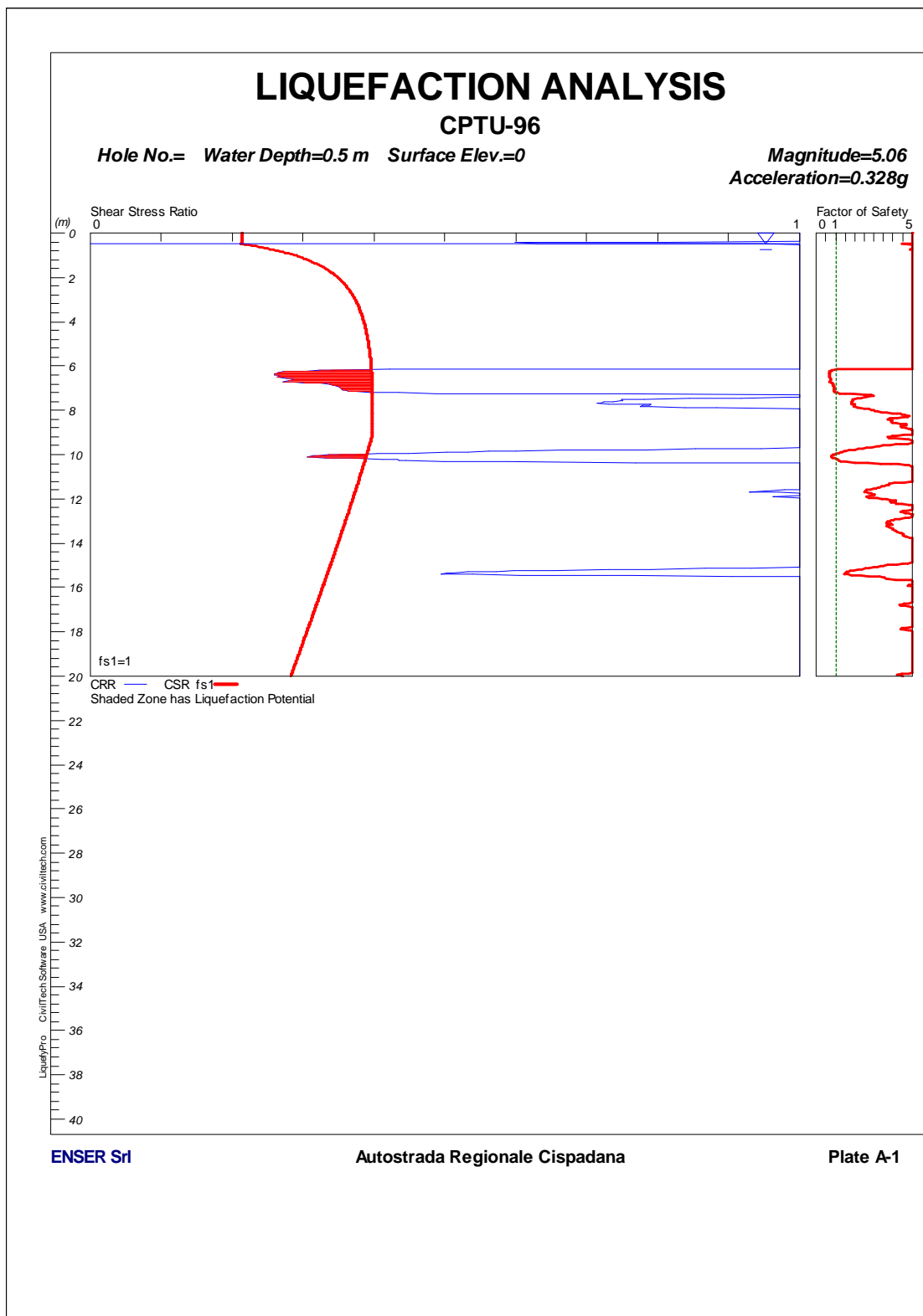
FIGURA 1-58: CPTU96 – VERIFICA A LIQUEFAZIONE.
