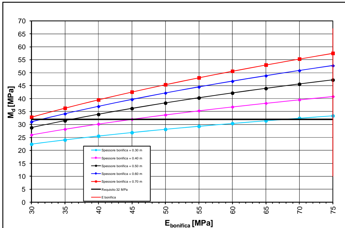
FIGURA 2-50: TRATTO 53 – DETERMINAZIONE SPESSORE DI BONIFICA.
