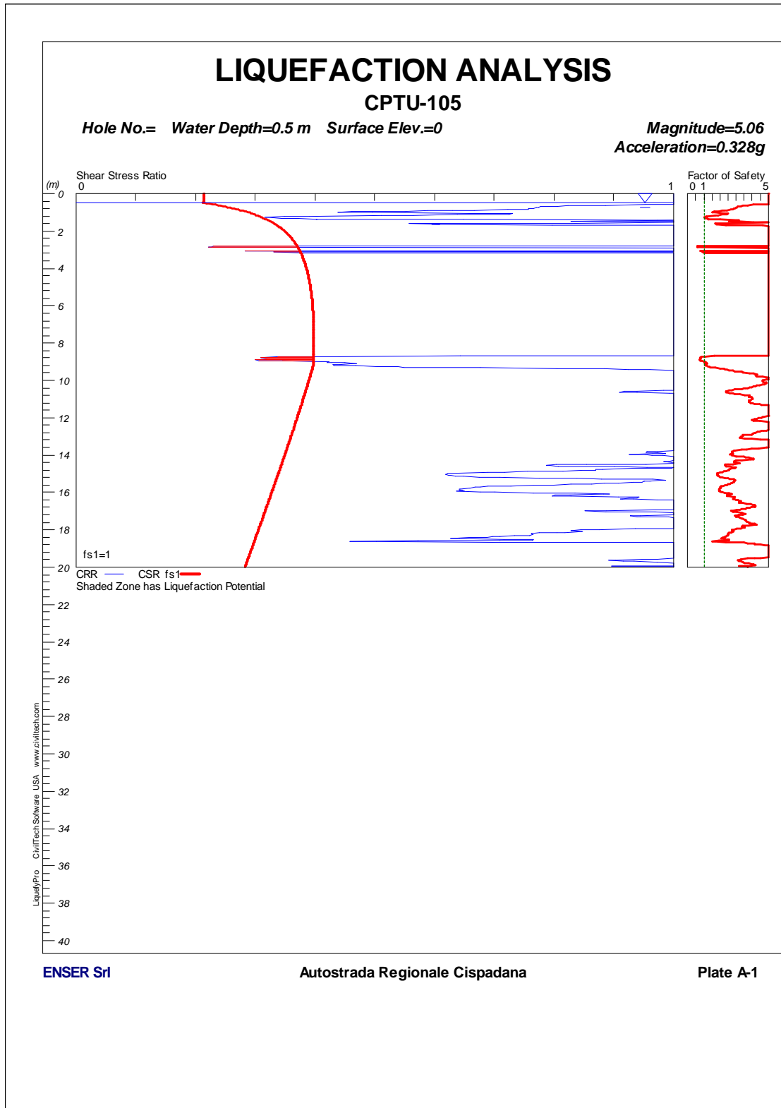
FIGURA 1-66: CPTU105 – VERIFICA A LIQUEFAZIONE.
