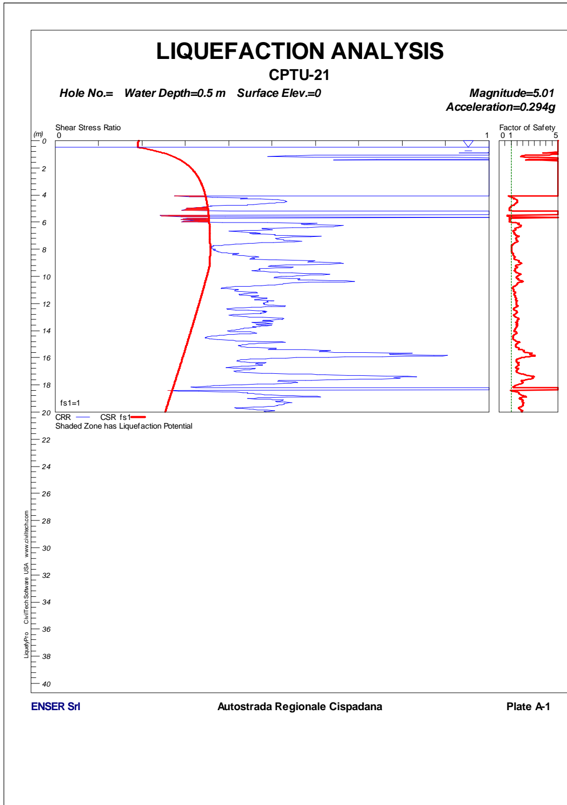
FIGURA 1-2: CPTU21 – VERIFICA A LIQUEFAZIONE.
