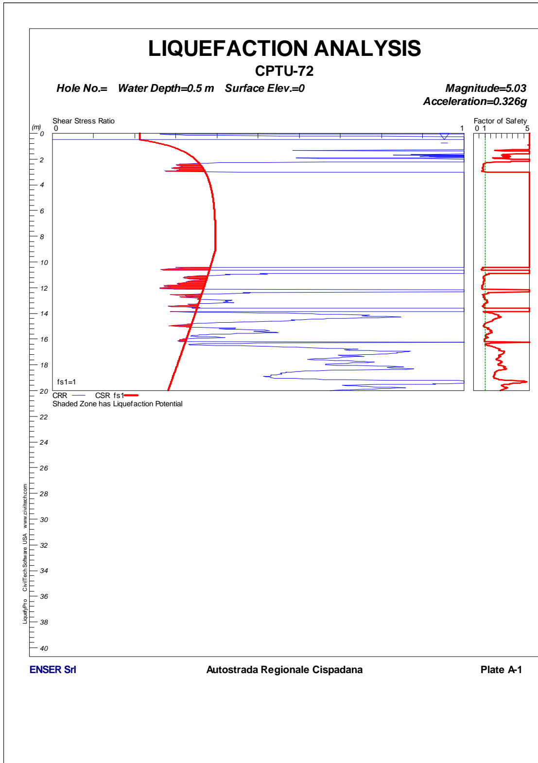
FIGURA 1-44: CPTU72 – VERIFICA A LIQUEFAZIONE.
