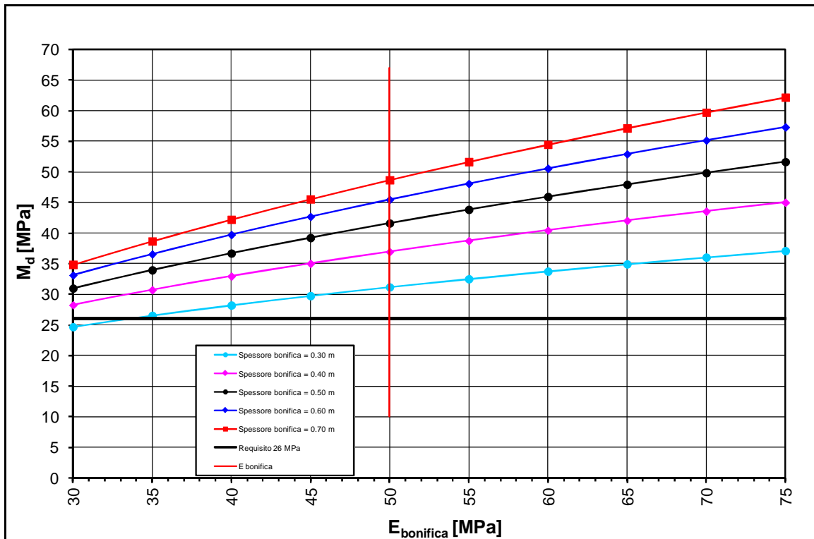
FIGURA 2-4: TRATTO 4 – DETERMINAZIONE SPESSORE DI BONIFICA.
