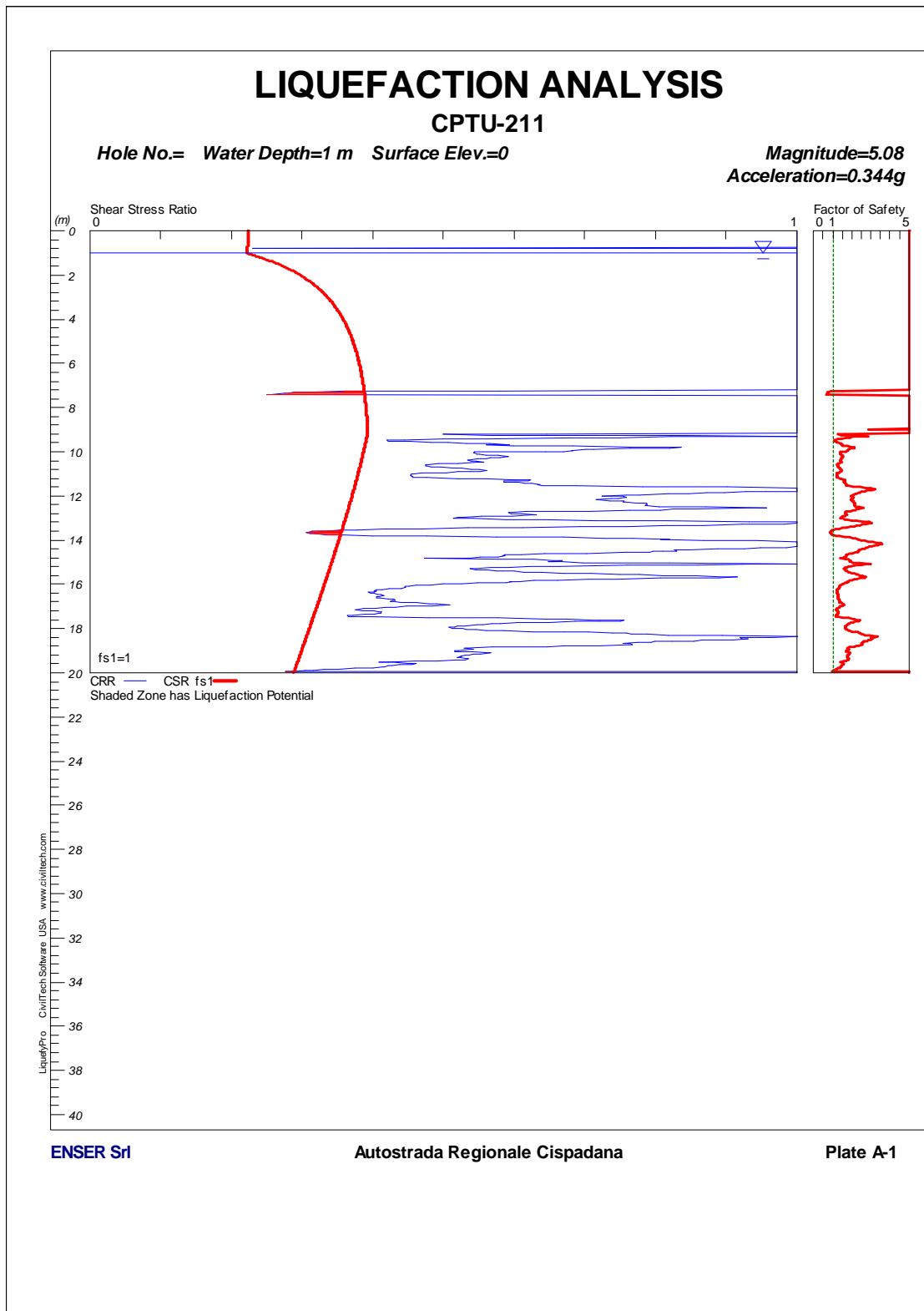
FIGURA 1-96: CPTU211 – Verifica a Liquefazione.
