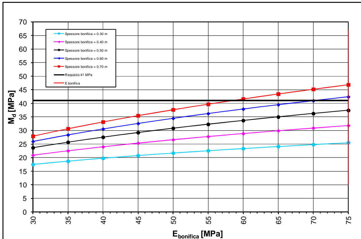
FIGURA 2-6: TRATTO 6 – DETERMINAZIONE SPESSORE DI BONIFICA.
