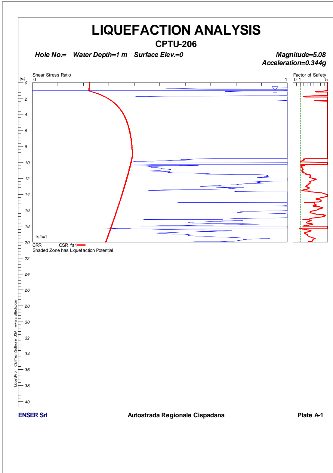
FIGURA 1-94: CPTU206 – VERIFICA A LIQUEFAZIONE.
