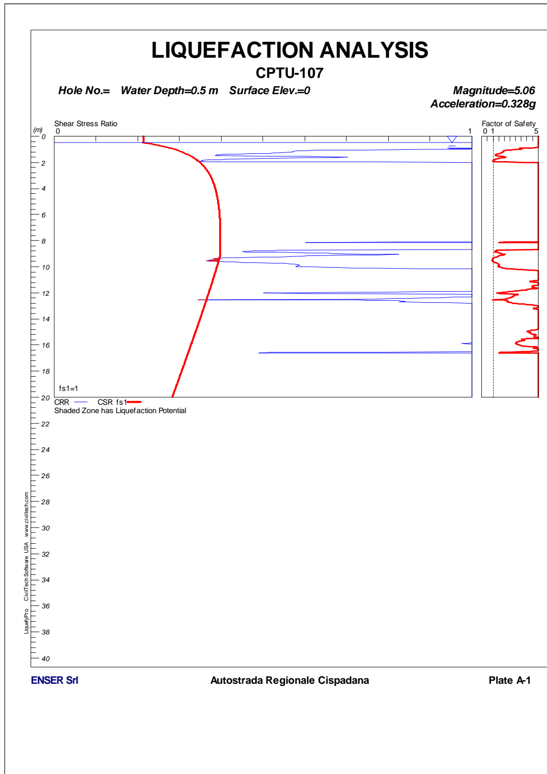
FIGURA 1-68: CPTU107 – VERIFICA A LIQUEFAZIONE.
