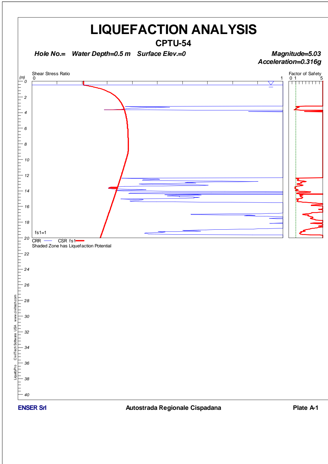
FIGURA 1-29: CPTU54 – VERIFICA A LIQUEFAZIONE.
