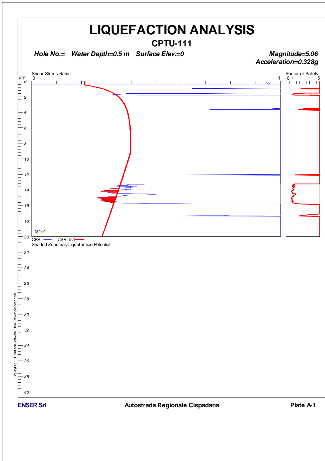
FIGURA 1-71: CPTU111 – VERIFICA A LIQUEFAZIONE.
