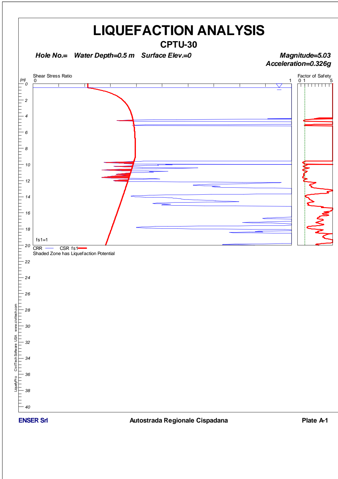
FIGURA 1-8: CPTU30 – VERIFICA A LIQUEFAZIONE.
