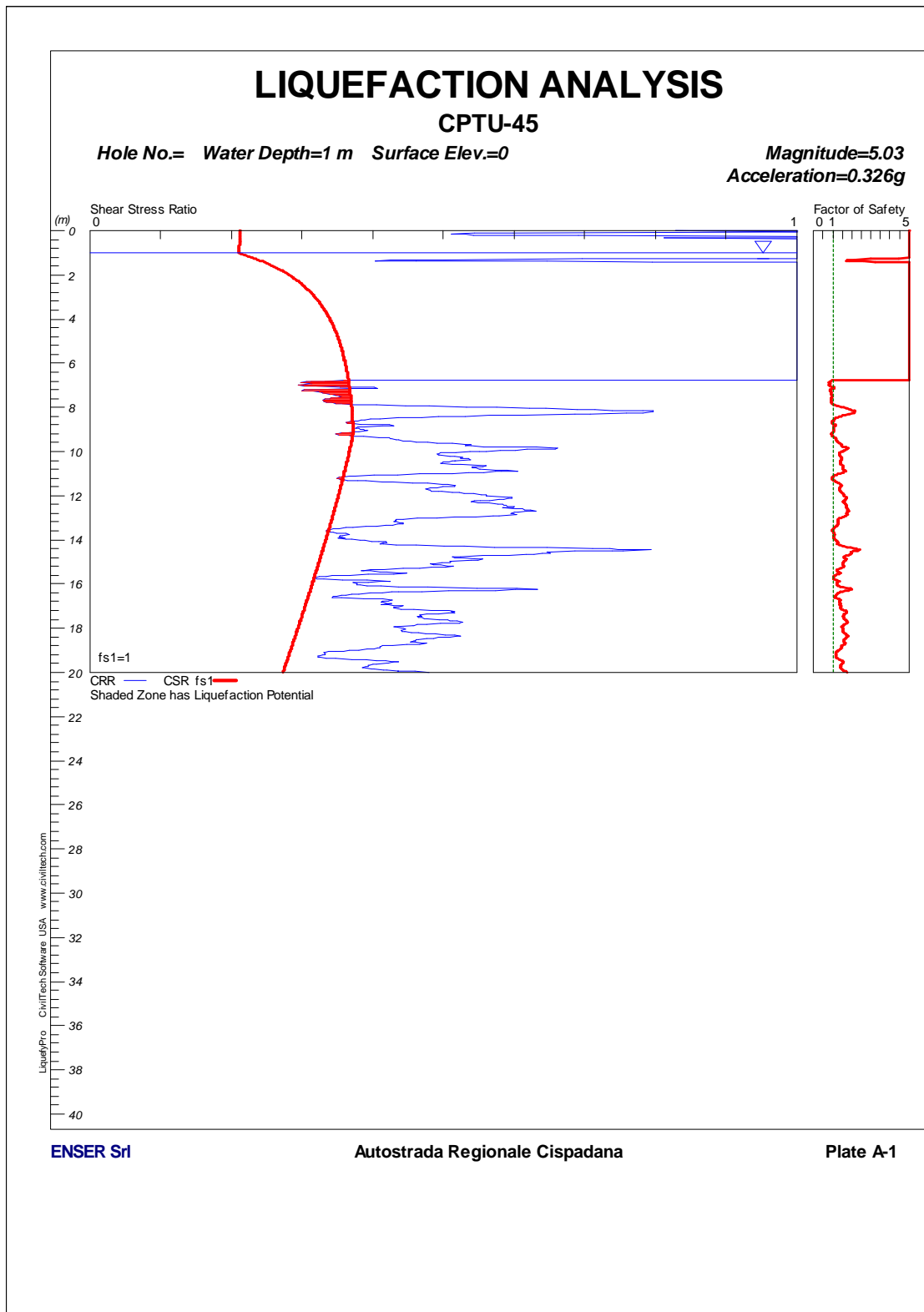
FIGURA 1-20: CPTU45 – VERIFICA A LIQUEFAZIONE.
