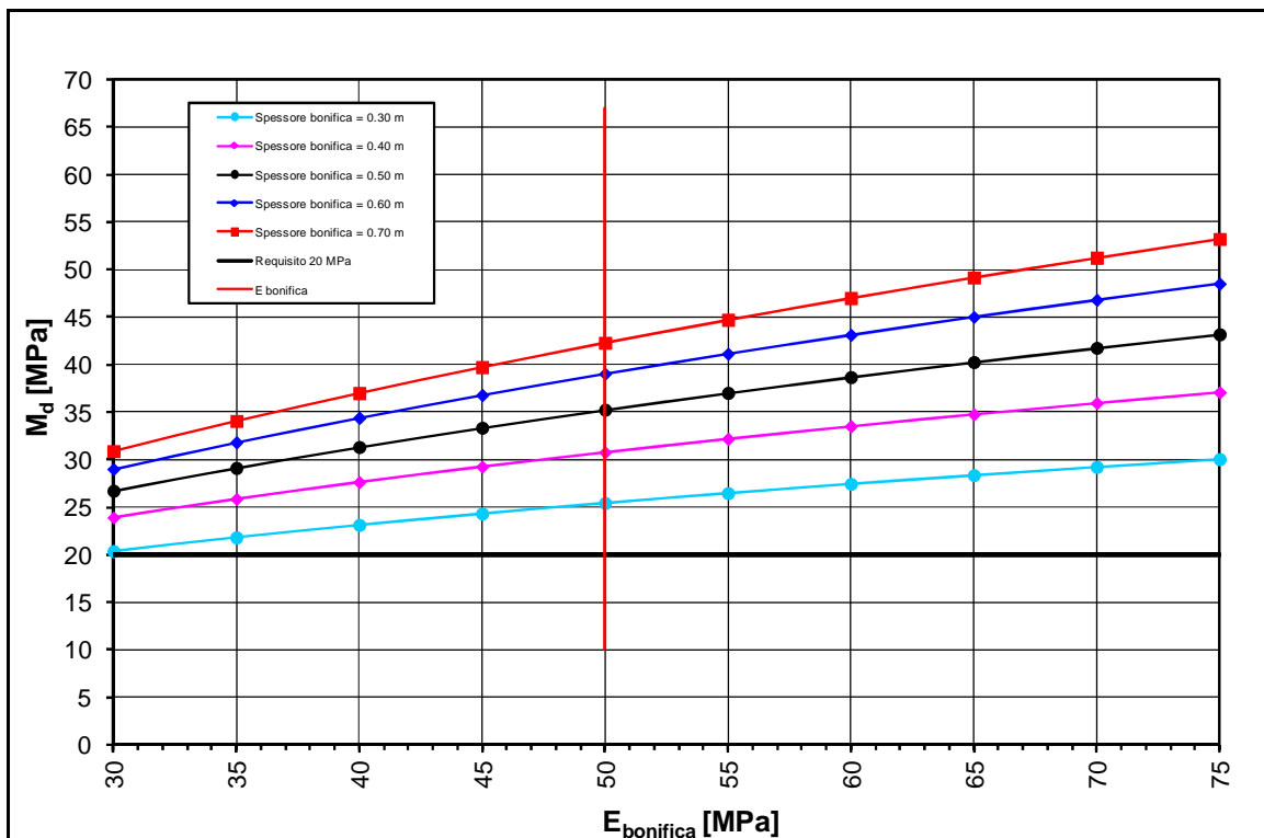
FIGURA 2-5: TRATTO 5 – DETERMINAZIONE SPESSORE DI BONIFICA.
