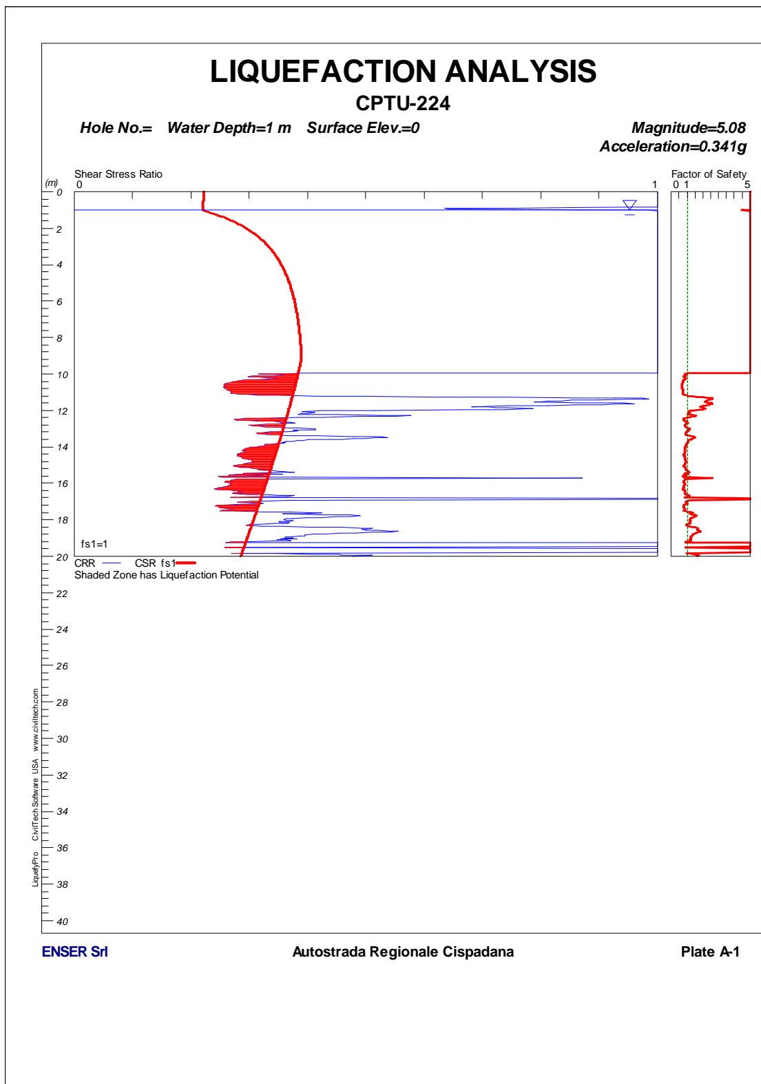
FIGURA 1-104: CPTU224 – VERIFICA A LIQUEFAZIONE.
