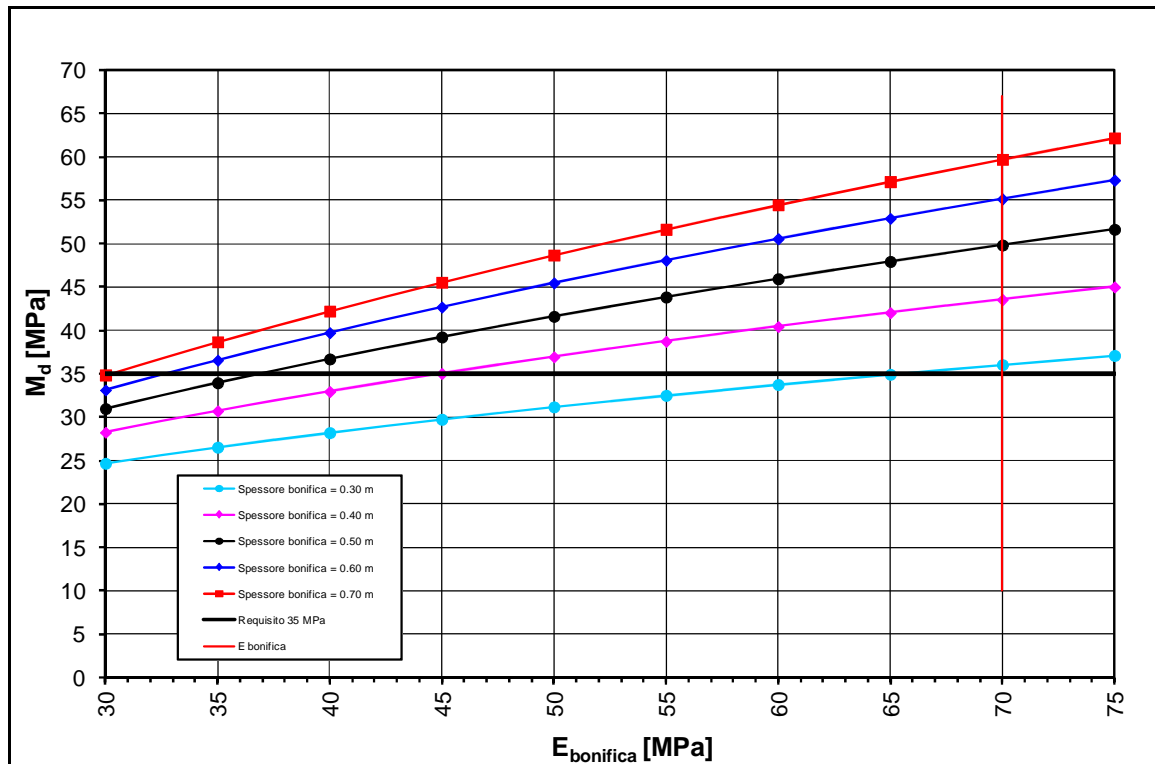
FIGURA 2-14: TRATTO 14 – DETERMINAZIONE SPESSORE DI BONIFICA.
