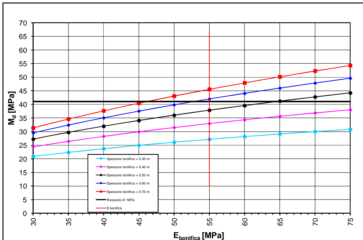
FIGURA 2-59: TRATTO 62 – DETERMINAZIONE SPESSORE DI BONIFICA.
