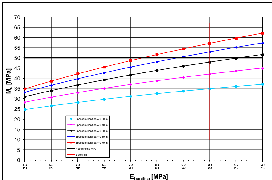
FIGURA 2-37: TRATTO 38 – DETERMINAZIONE SPESSORE DI BONIFICA.
