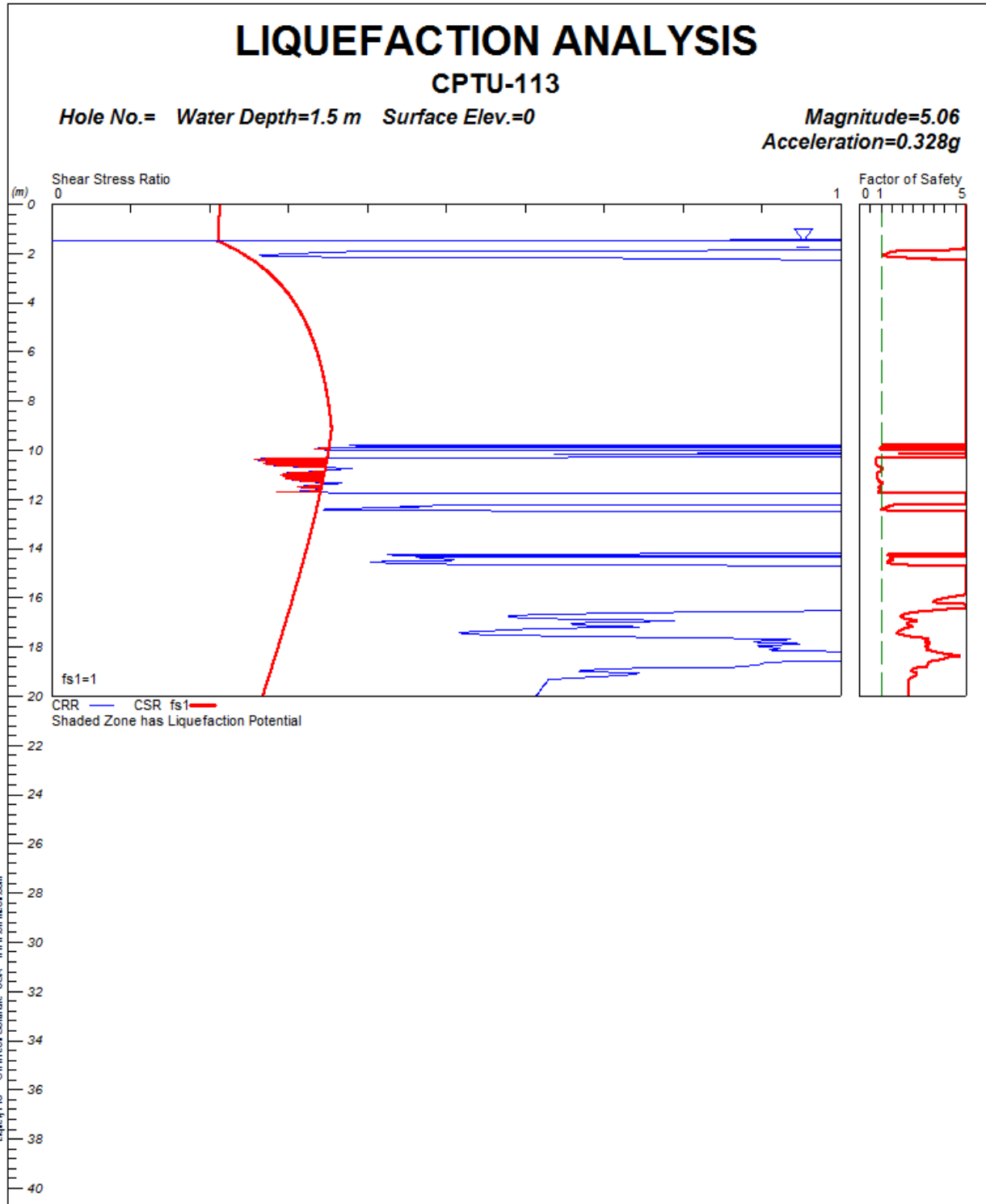
FIGURA 1-73: CPTU113 – VERIFICA A LIQUEFAZIONE.
