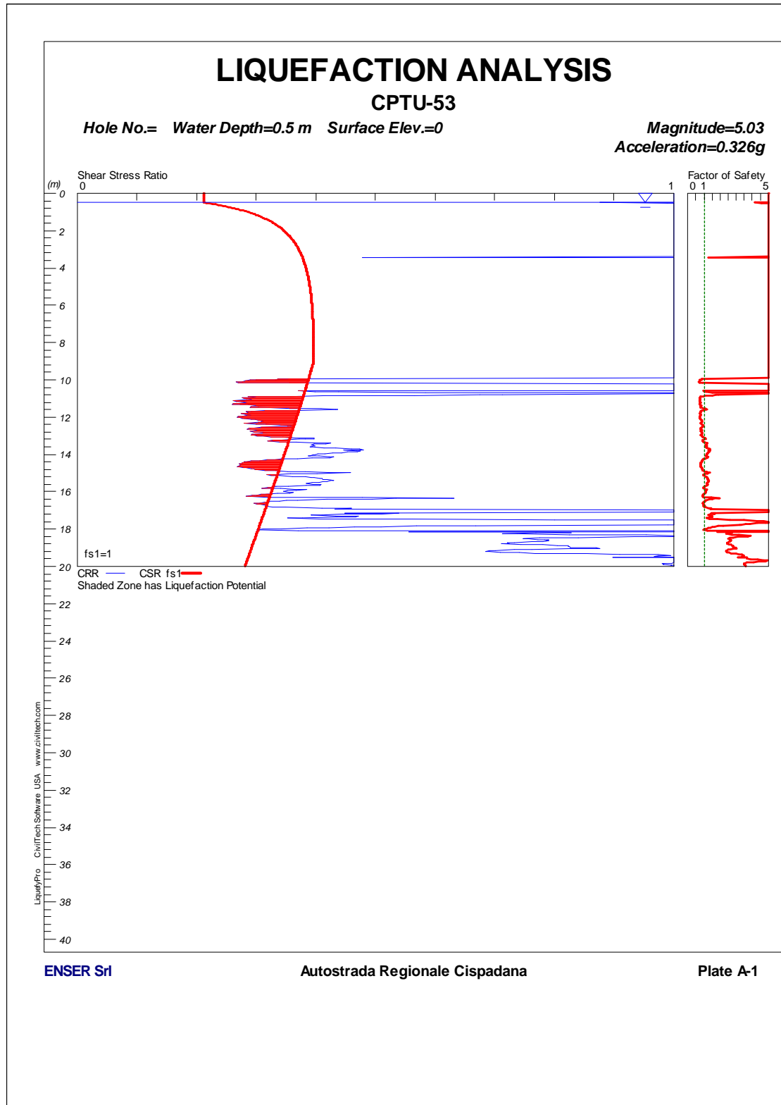
FIGURA 1-28: CPTU53 – VERIFICA A LIQUEFAZIONE.
