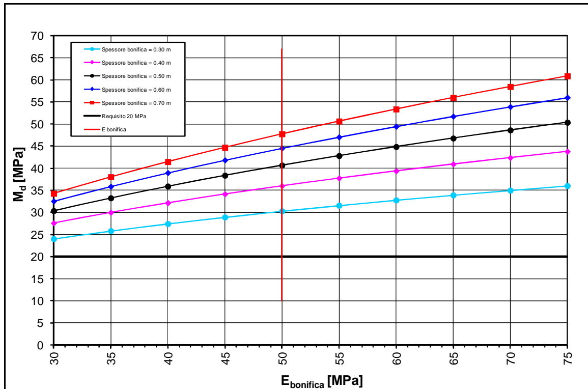
FIGURA 2-36: TRATTO 37 – DETERMINAZIONE SPESSORE DI BONIFICA.
