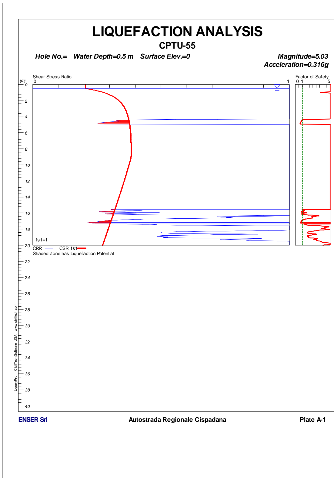
FIGURA 1-30: CPTU55 – VERIFICA A LIQUEFAZIONE.
