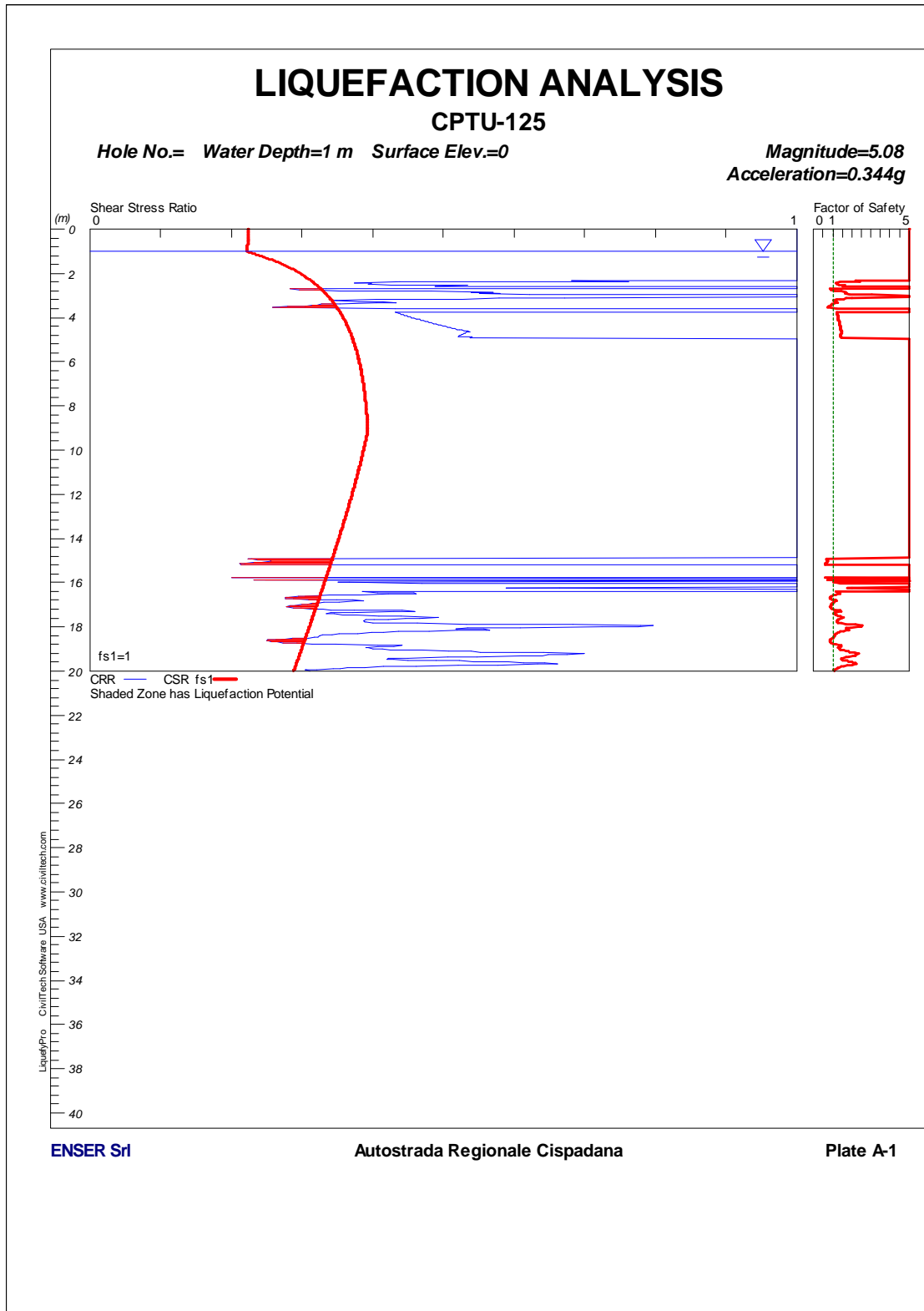
FIGURA 1-85: CPTU125 – VERIFICA A LIQUEFAZIONE.
