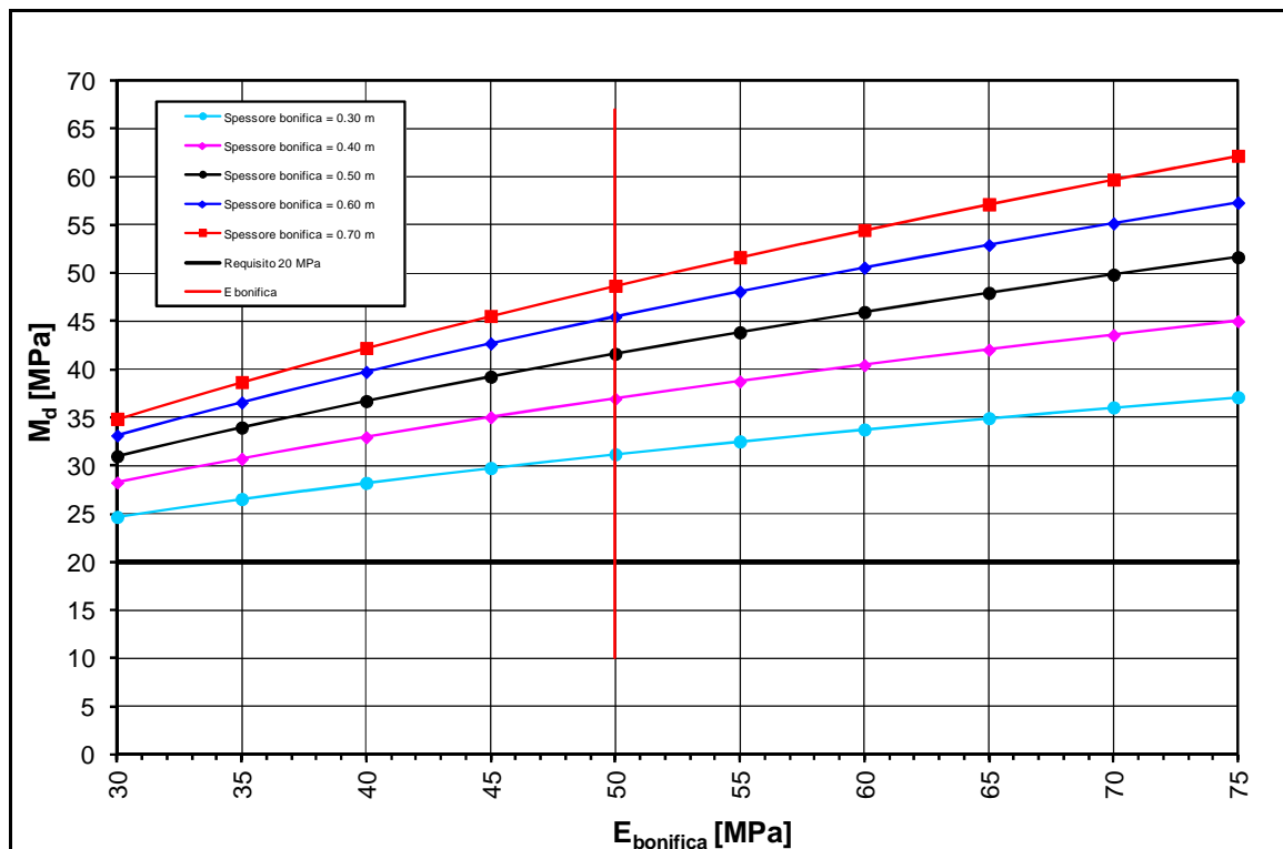
FIGURA 2-15: TRATTO 15 – DETERMINAZIONE SPESSORE DI BONIFICA.
