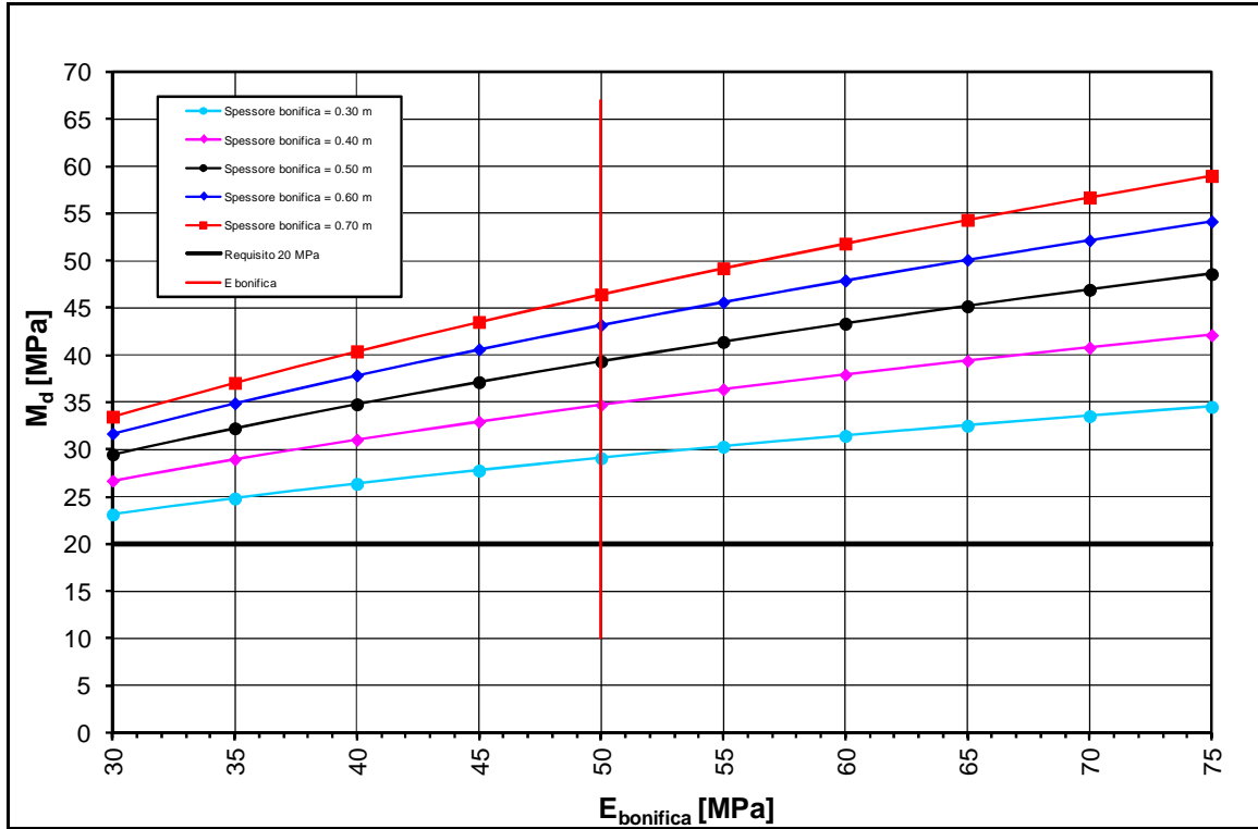
FIGURA 2-18: TRATTO 18 – DETERMINAZIONE SPESSORE DI BONIFICA.
