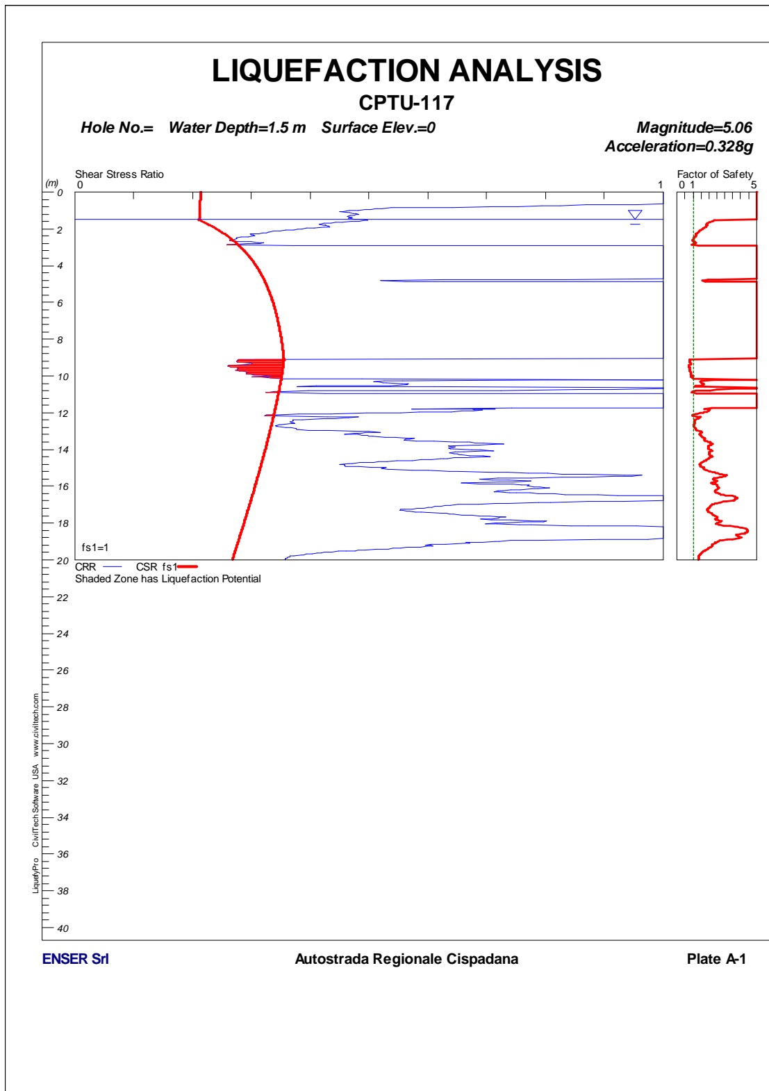
FIGURA 1-77: CPTU117 – VERIFICA A LIQUEFAZIONE.
