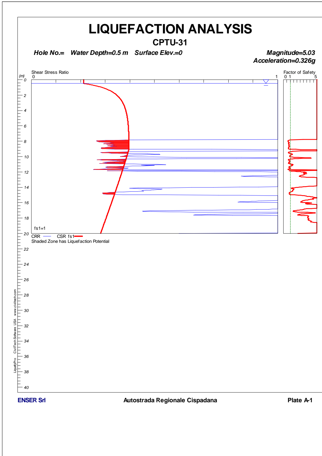
FIGURA 1-9: CPTU31 – VERIFICA A LIQUEFAZIONE.
