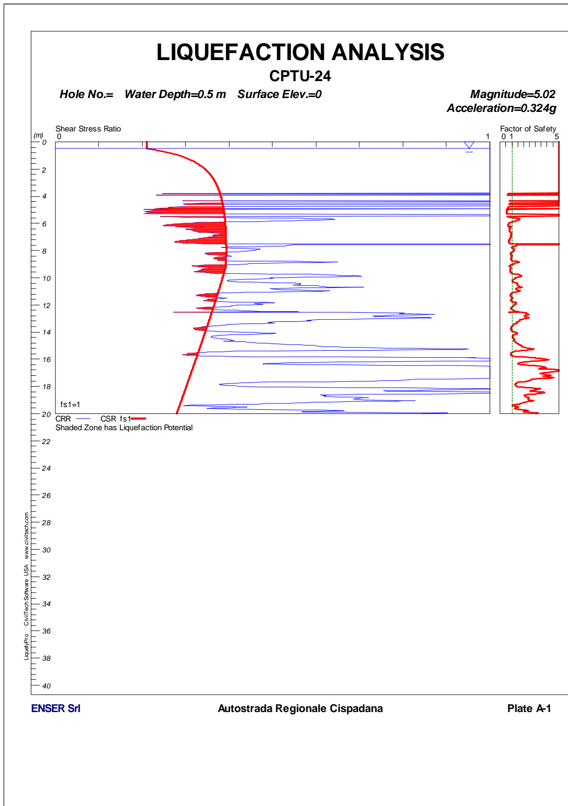
FIGURA 1-5: CPTU24 – VERIFICA A LIQUEFAZIONE.
