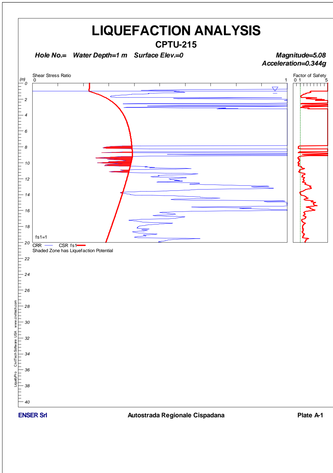
FIGURA 1-99: CPTU215 – Verifica a Liquefazione.
