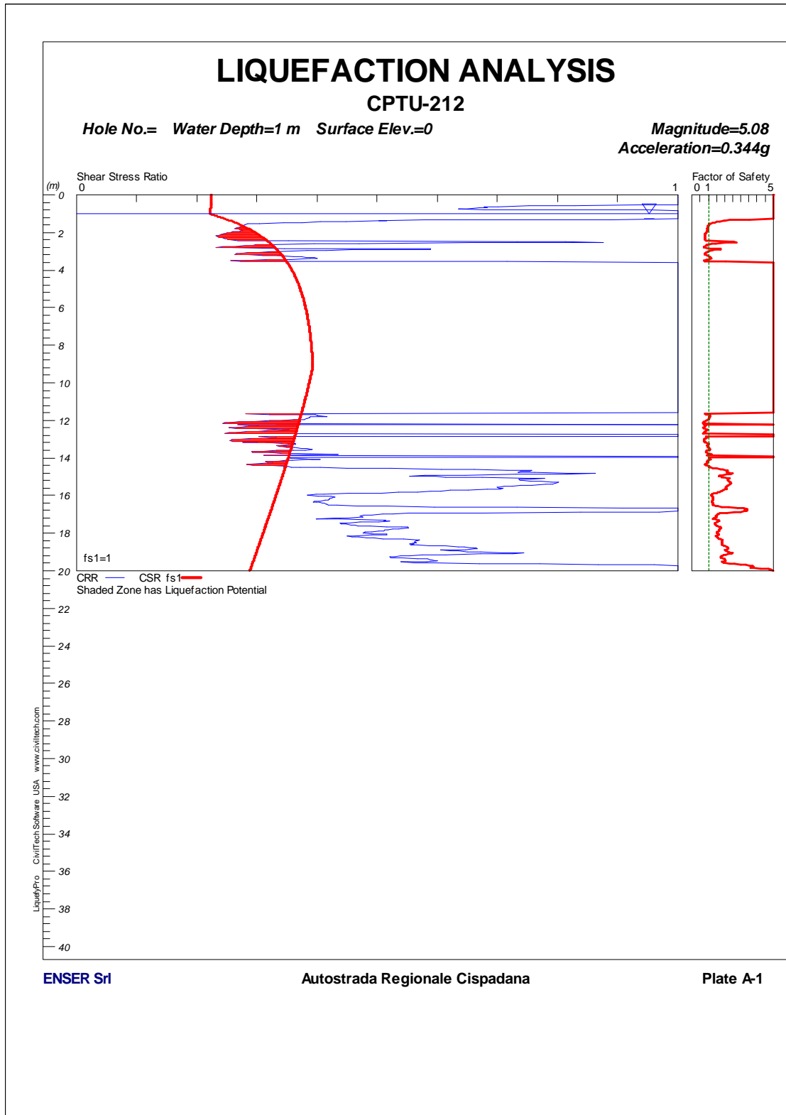
FIGURA 1-97: CPTU212 – Verifica a Liquefazione.
