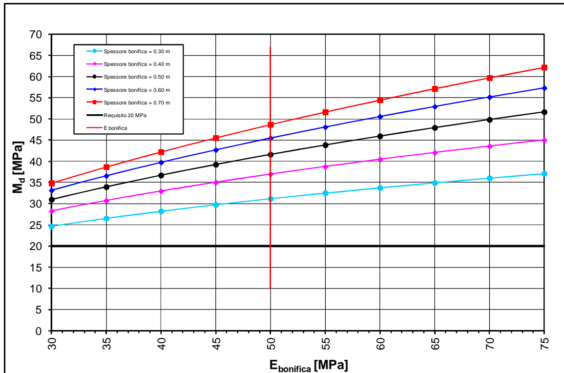
FIGURA 2-34: TRATTO 35 – DETERMINAZIONE SPESSORE DI BONIFICA.
