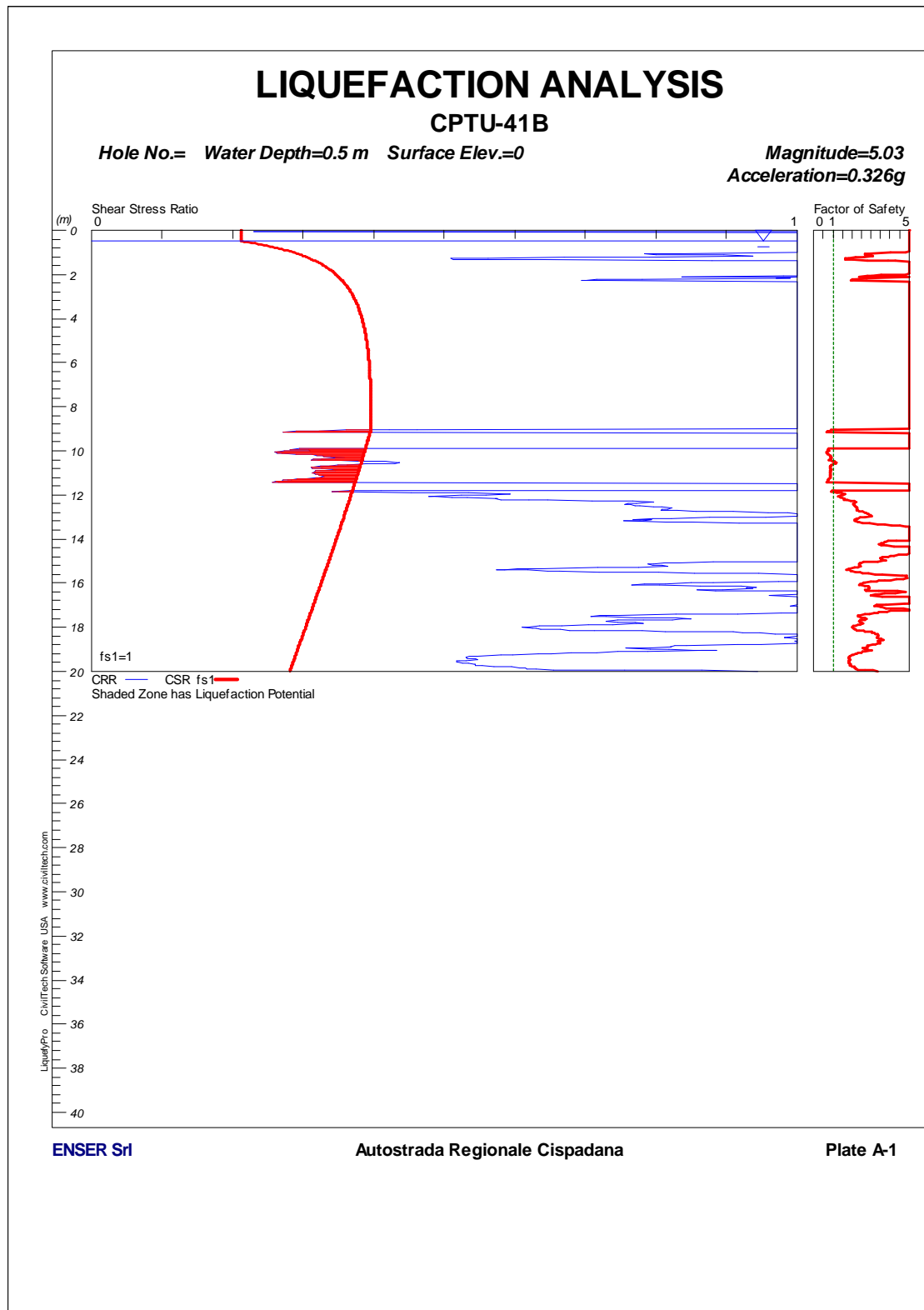
FIGURA 1-16: CPTU41 – VERIFICA A LIQUEFAZIONE.
