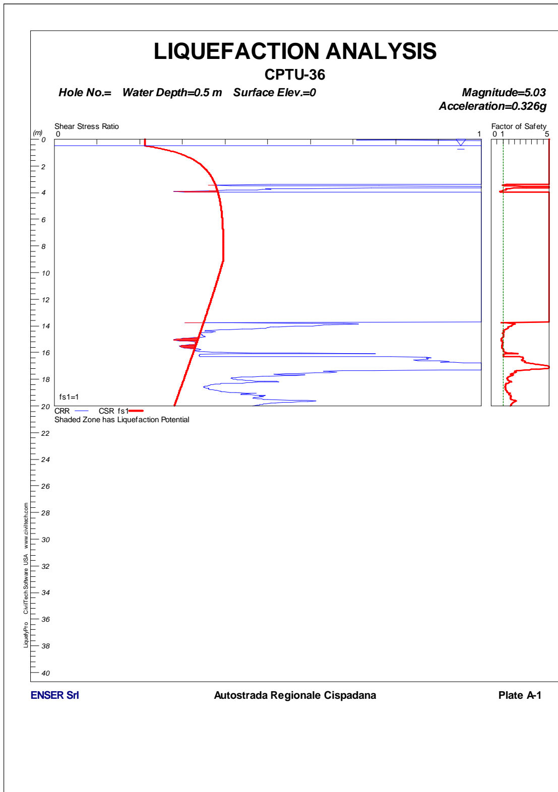
FIGURA 1-13: CPTU36 – VERIFICA A LIQUEFAZIONE.
