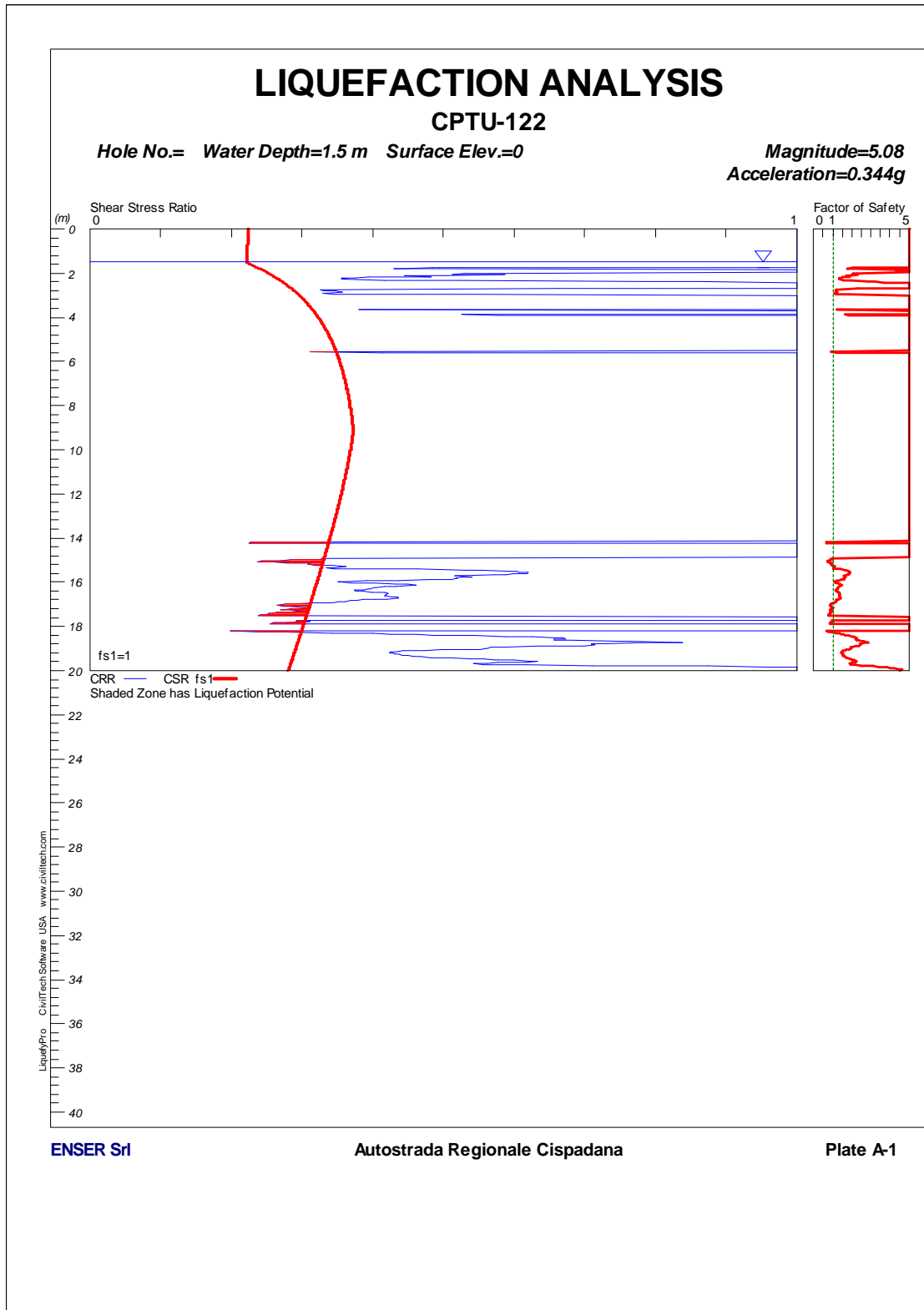
FIGURA 1-82: CPTU122 – VERIFICA A LIQUEFAZIONE.
