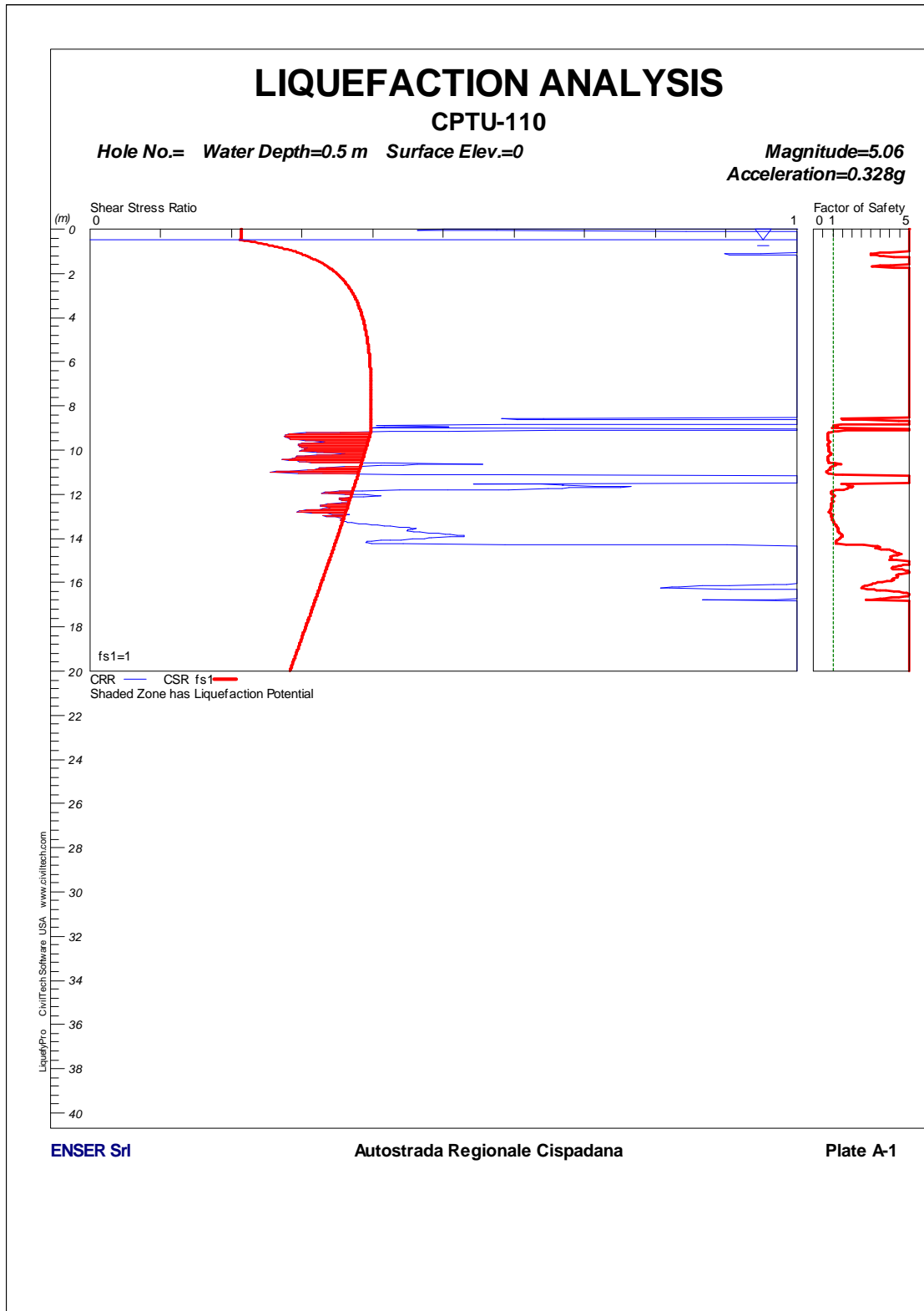
FIGURA 1-70: CPTU110 – VERIFICA A LIQUEFAZIONE.
