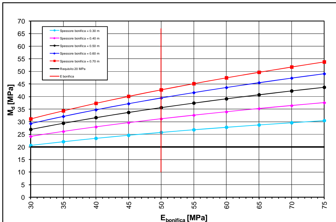
FIGURA 2-51: TRATTO 54 – DETERMINAZIONE SPESSORE DI BONIFICA.
