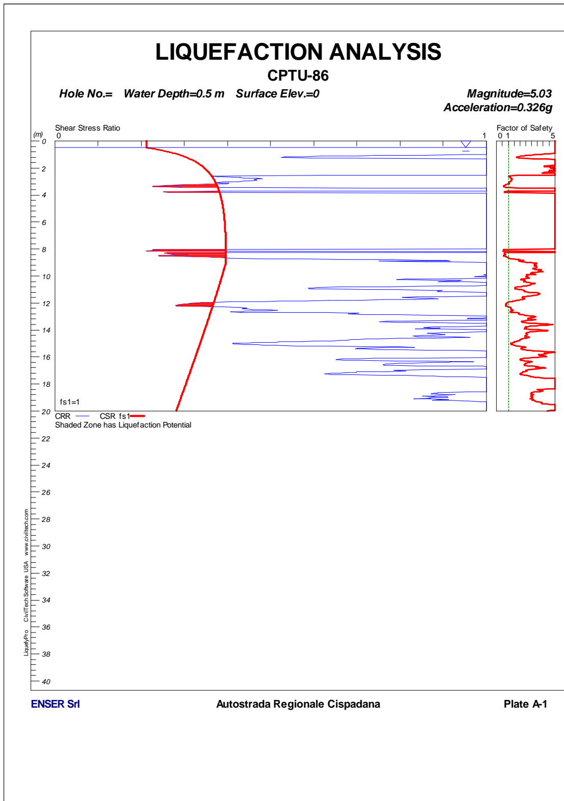
FIGURA 1-51: CPTU86 – VERIFICA A LIQUEFAZIONE.
