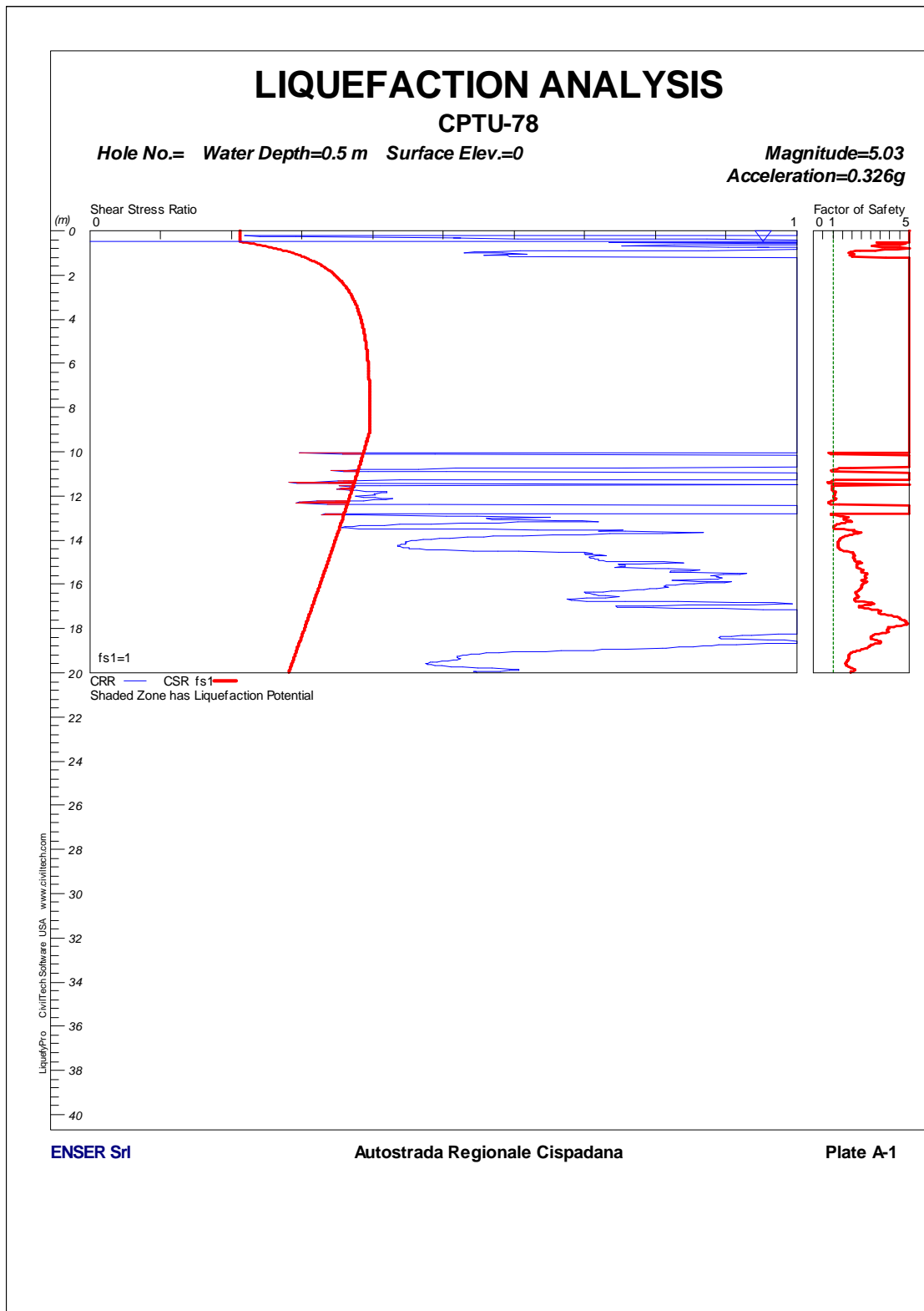
FIGURA 1-48: CPTU78 – VERIFICA A LIQUEFAZIONE.
