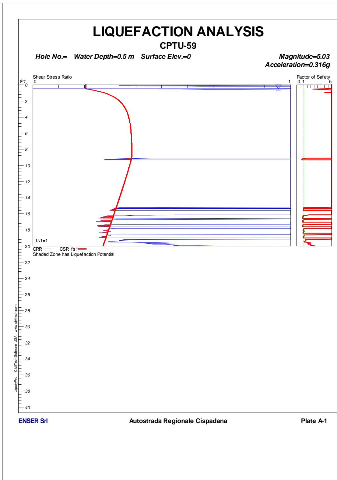
FIGURA 1-34: CPTU59 – VERIFICA A LIQUEFAZIONE.
