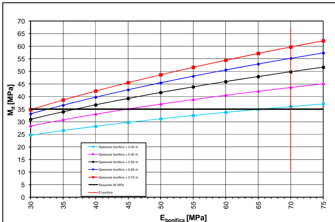
FIGURA 2-17: TRATTO 17 – DETERMINAZIONE SPESSORE DI BONIFICA.
