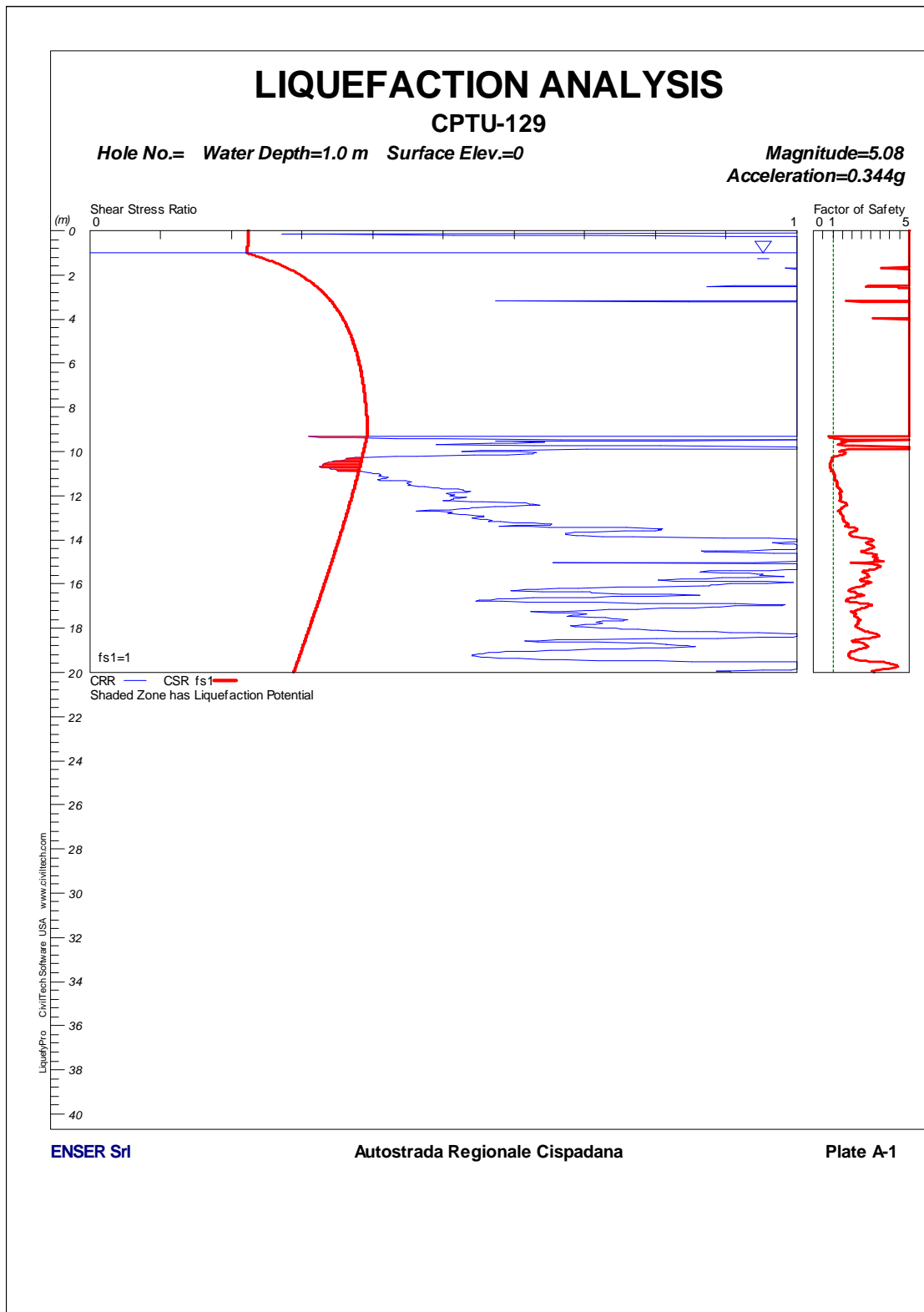
FIGURA 1-87: CPTU129 – VERIFICA A LIQUEFAZIONE.
