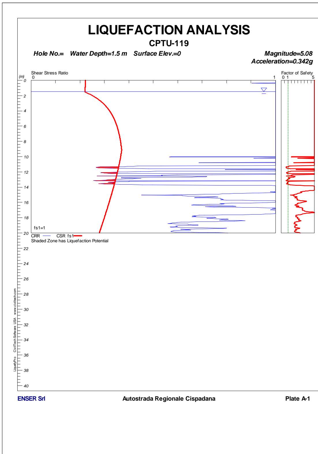
FIGURA 1-79: CPTU119 – VERIFICA A LIQUEFAZIONE.
