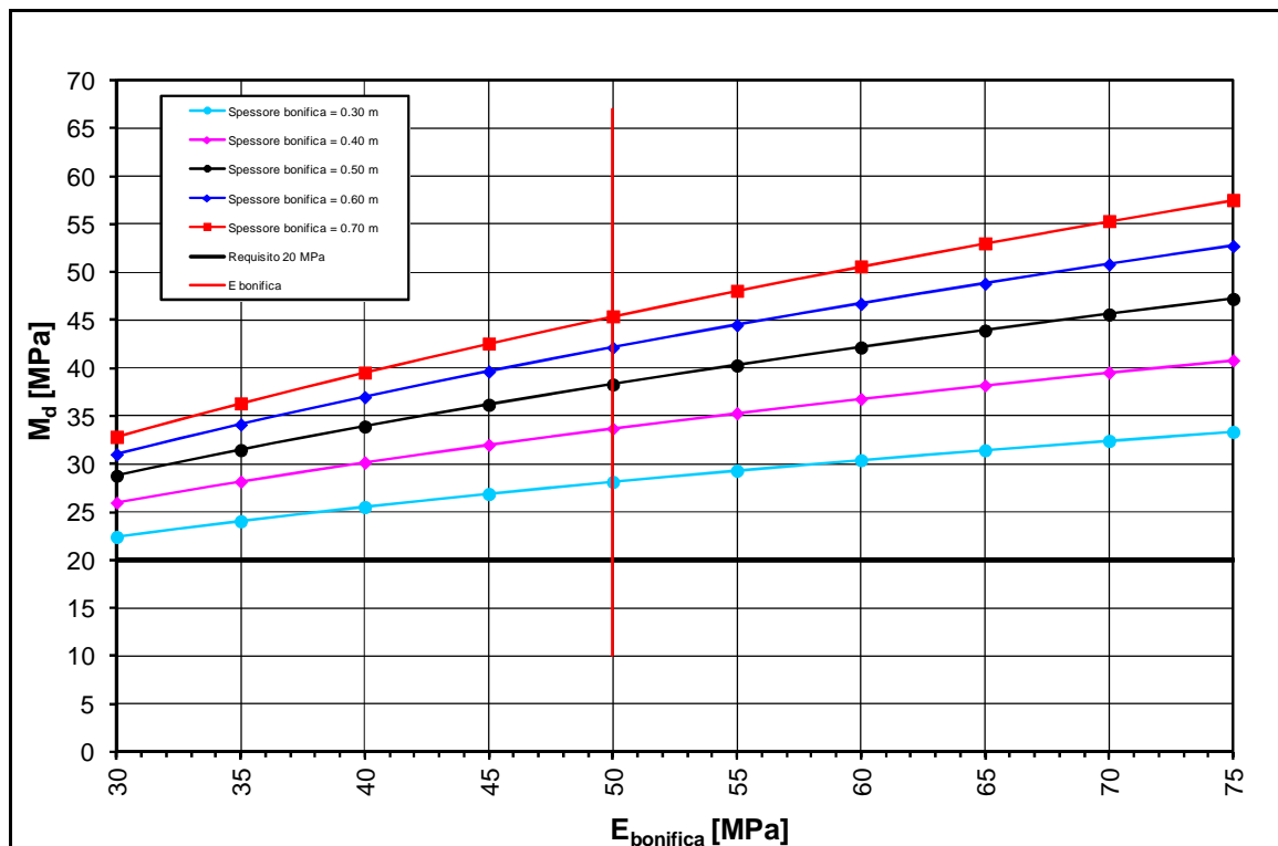
FIGURA 2-43: TRATTO 46 – DETERMINAZIONE SPESSORE DI BONIFICA.
