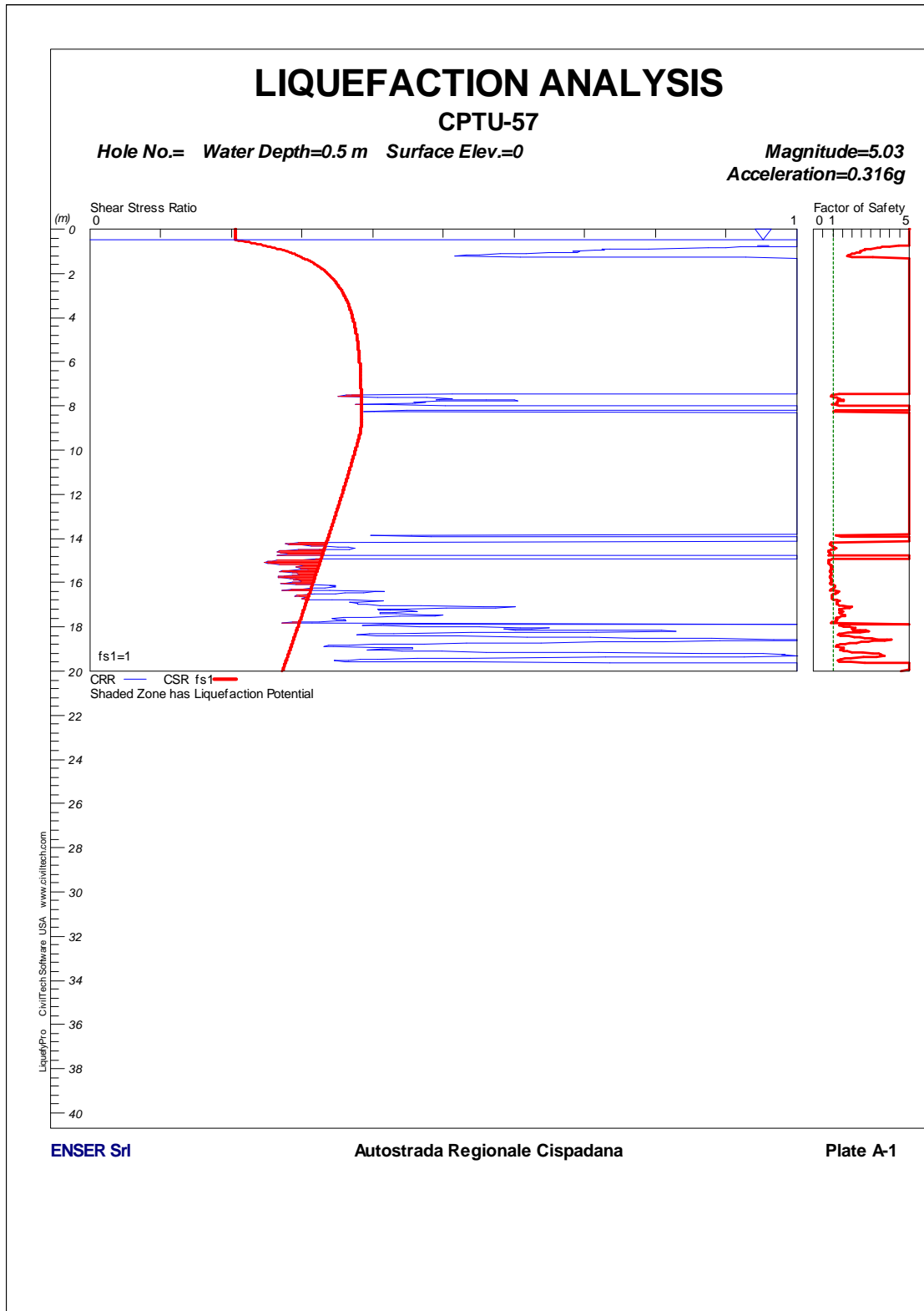
FIGURA 1-32: CPTU57 – VERIFICA A LIQUEFAZIONE.
