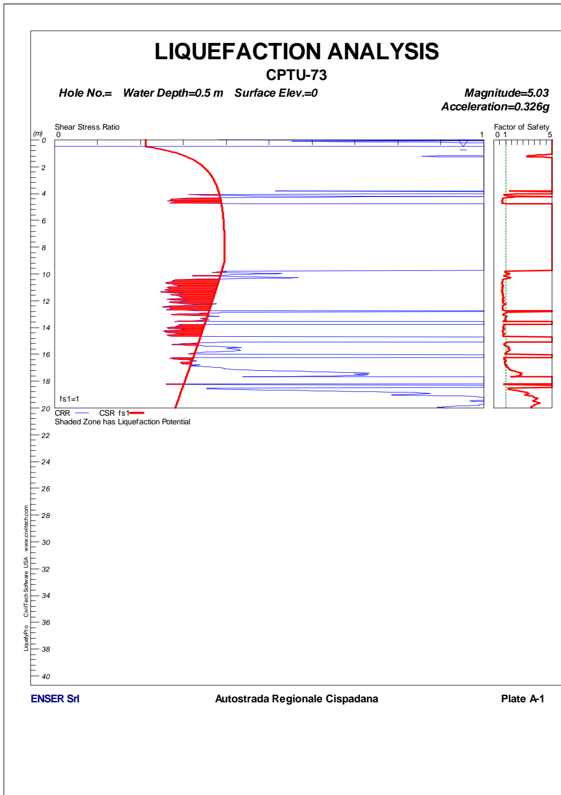
FIGURA 1-45: CPTU73 – VERIFICA A LIQUEFAZIONE.
