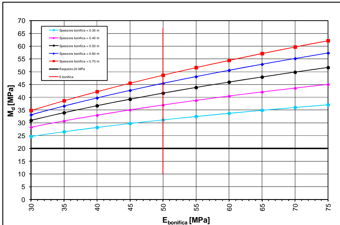
FIGURA 2-60: TRATTO 63 – DETERMINAZIONE SPESSORE DI BONIFICA.
