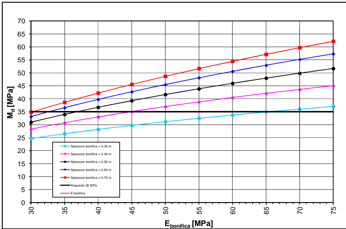
FIGURA 2-12: TRATTO 12 – DETERMINAZIONE SPESSORE DI BONIFICA.
