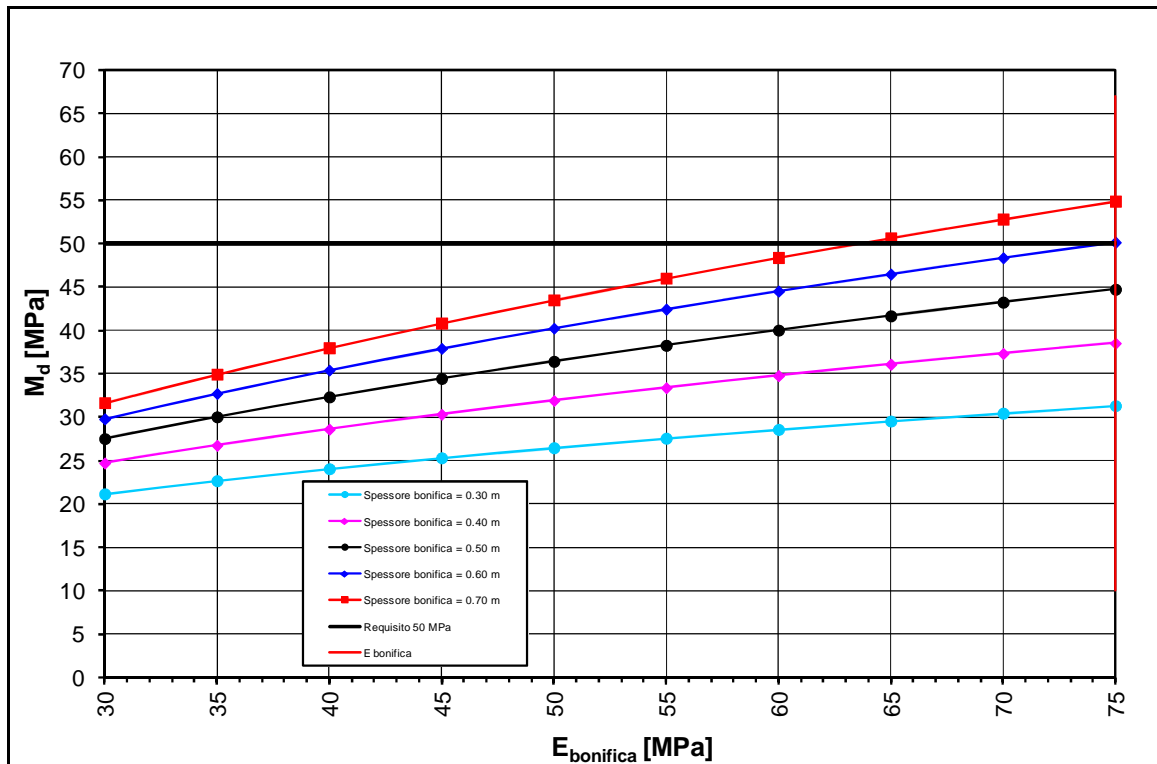
FIGURA 2-20: TRATTO 21 – DETERMINAZIONE SPESSORE DI BONIFICA.
