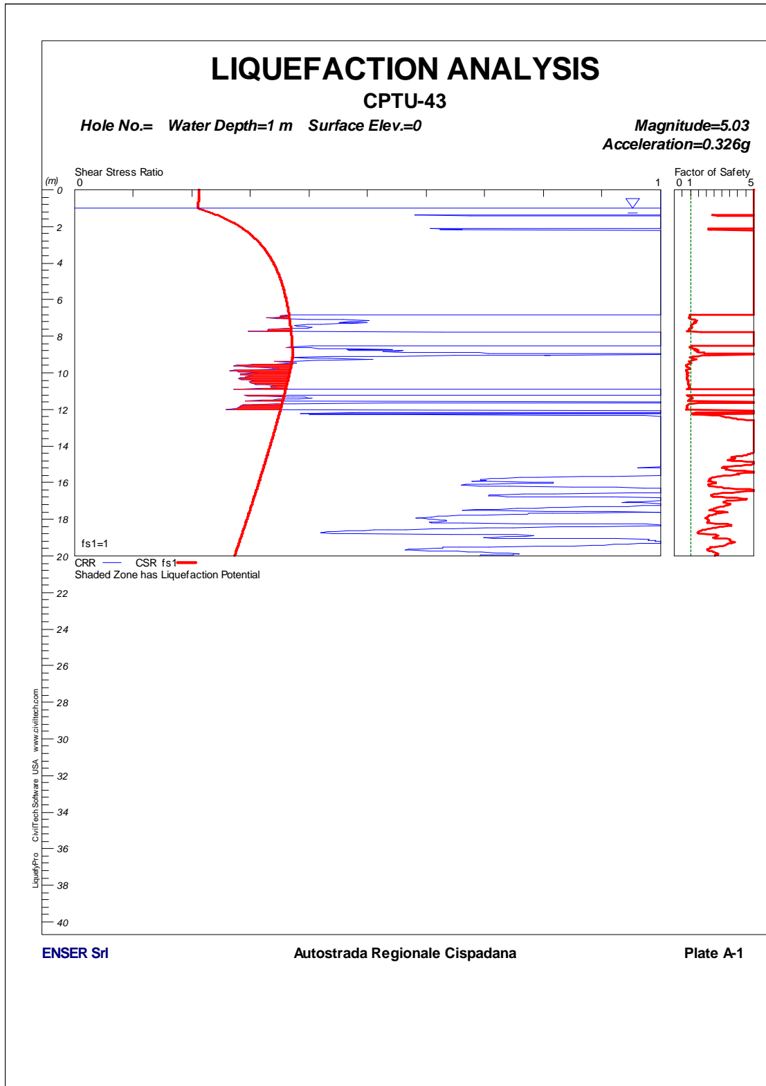
FIGURA 1-18: CPTU43 – VERIFICA A LIQUEFAZIONE.
