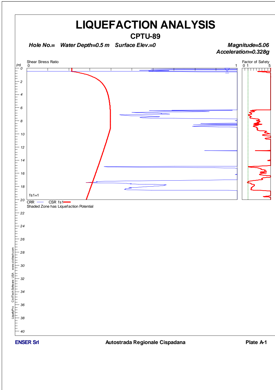
FIGURA 1-54: CPTU89 – VERIFICA A LIQUEFAZIONE.
