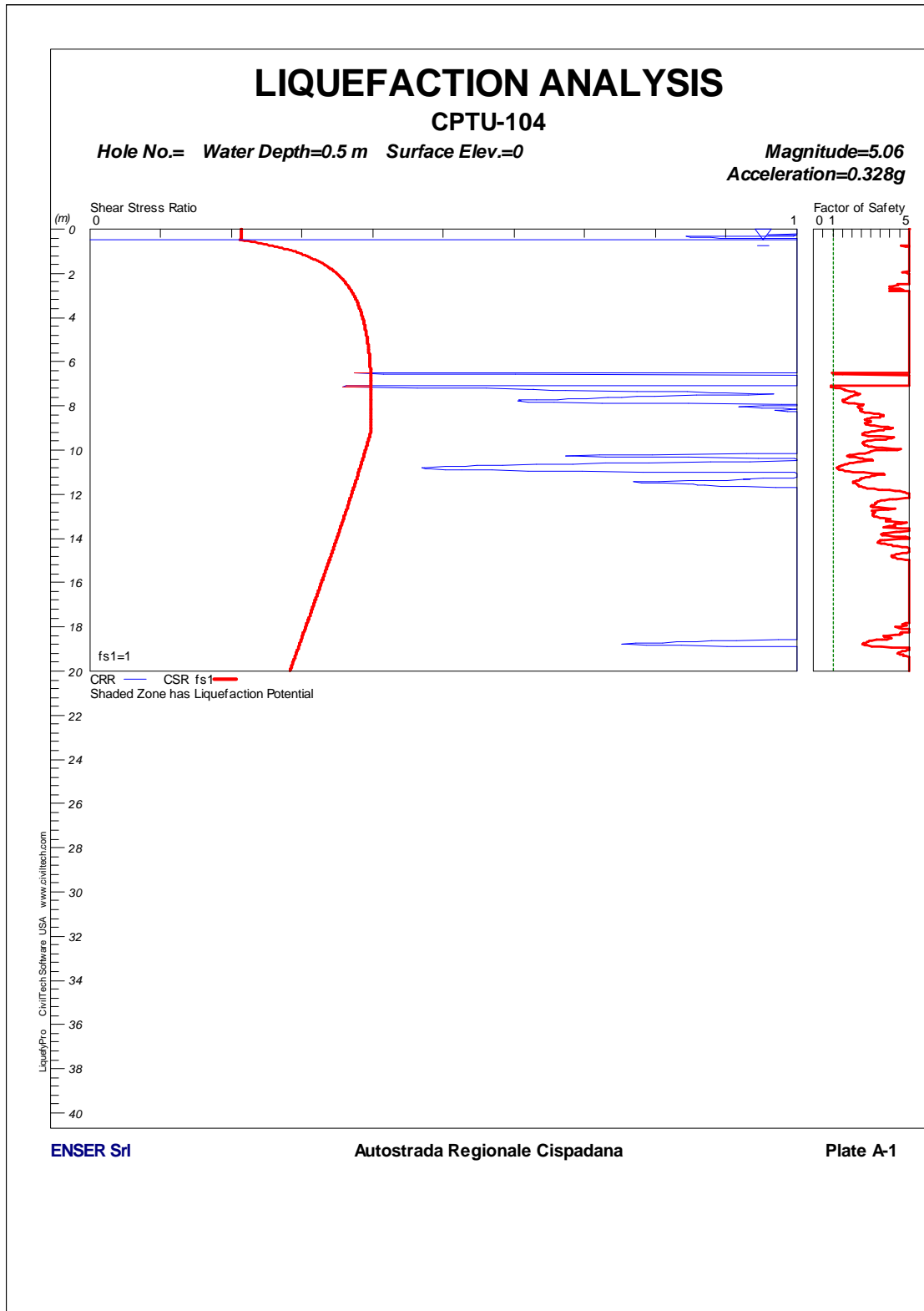
FIGURA 1-65: CPTU104 – VERIFICA A LIQUEFAZIONE.
