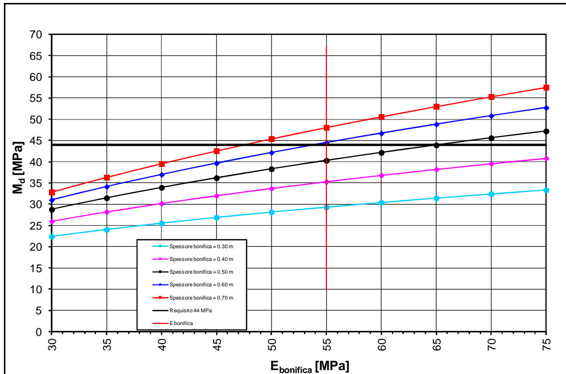
FIGURA 2-42: TRATTO 45 – DETERMINAZIONE SPESSORE DI BONIFICA.
