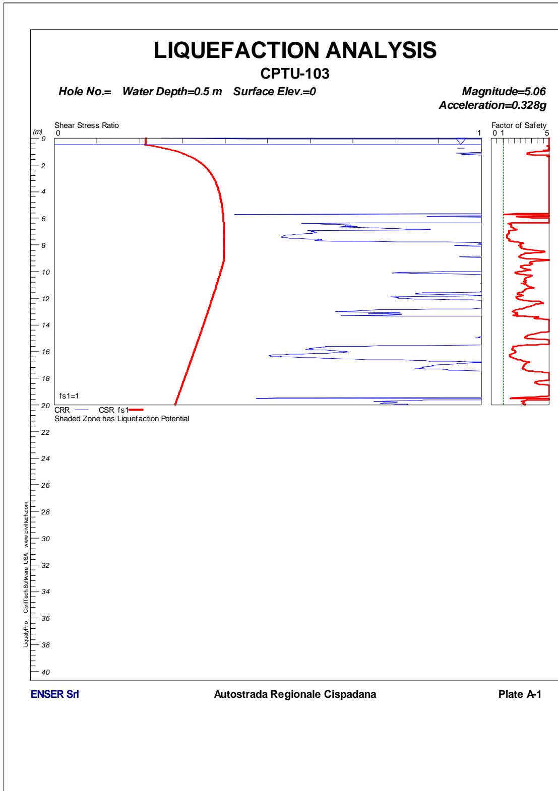
FIGURA 1-64: CPTU103 – VERIFICA A LIQUEFAZIONE.
