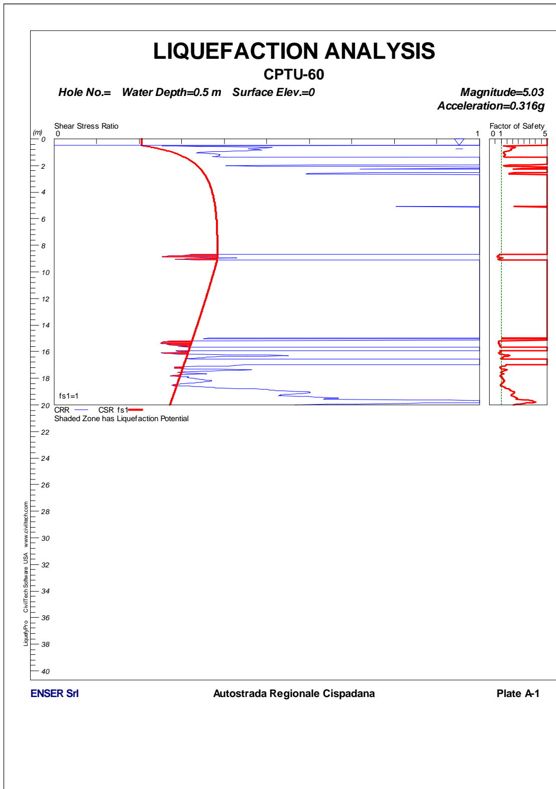
FIGURA 1-35: CPTU60 – VERIFICA A LIQUEFAZIONE.
