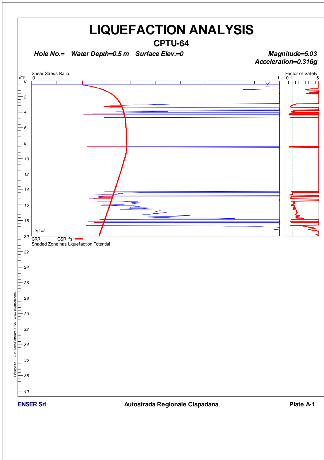
FIGURA 1-39: CPTU64 – VERIFICA A LIQUEFAZIONE.
