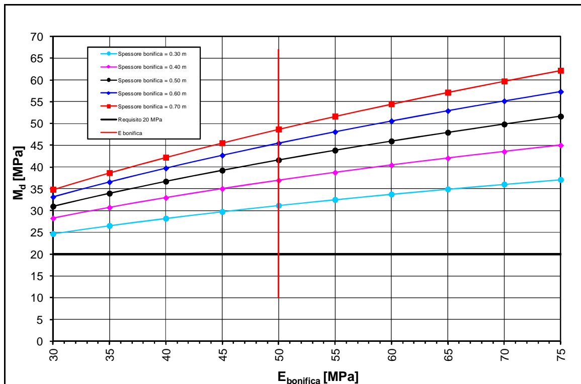
FIGURA 2-7: TRATTO 7 – DETERMINAZIONE SPESSORE DI BONIFICA.
