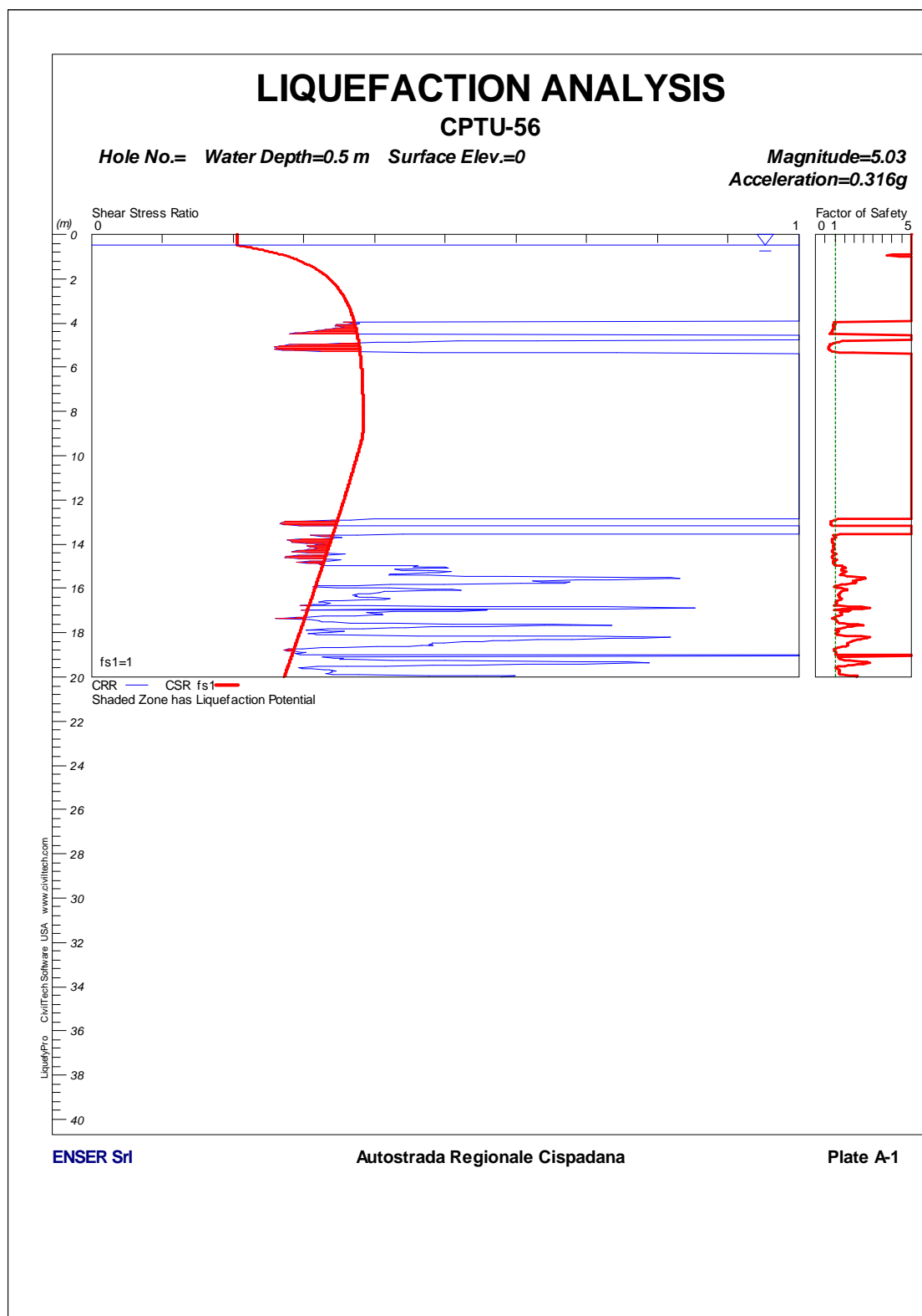
FIGURA 1-31: CPTU56 – VERIFICA A LIQUEFAZIONE.
