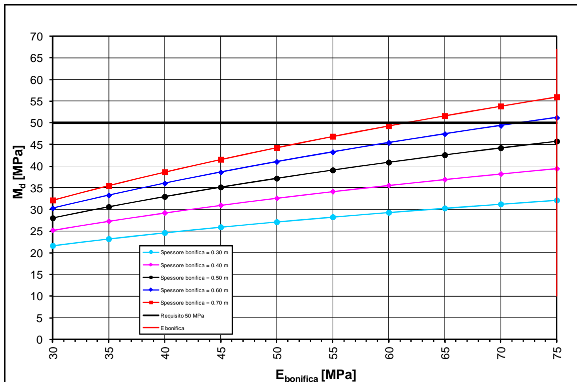
FIGURA 2-39: TRATTO 40 – DETERMINAZIONE SPESSORE DI BONIFICA.
