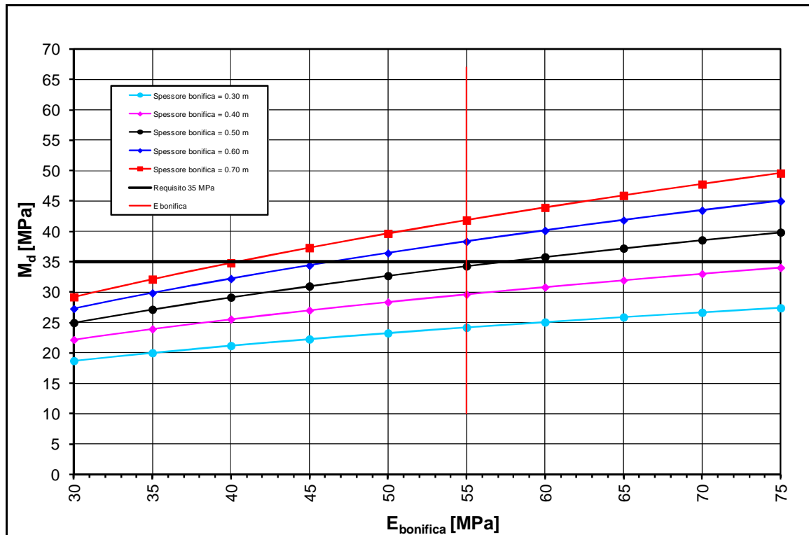
FIGURA 2-32: TRATTO 33 – DETERMINAZIONE SPESSORE DI BONIFICA.
