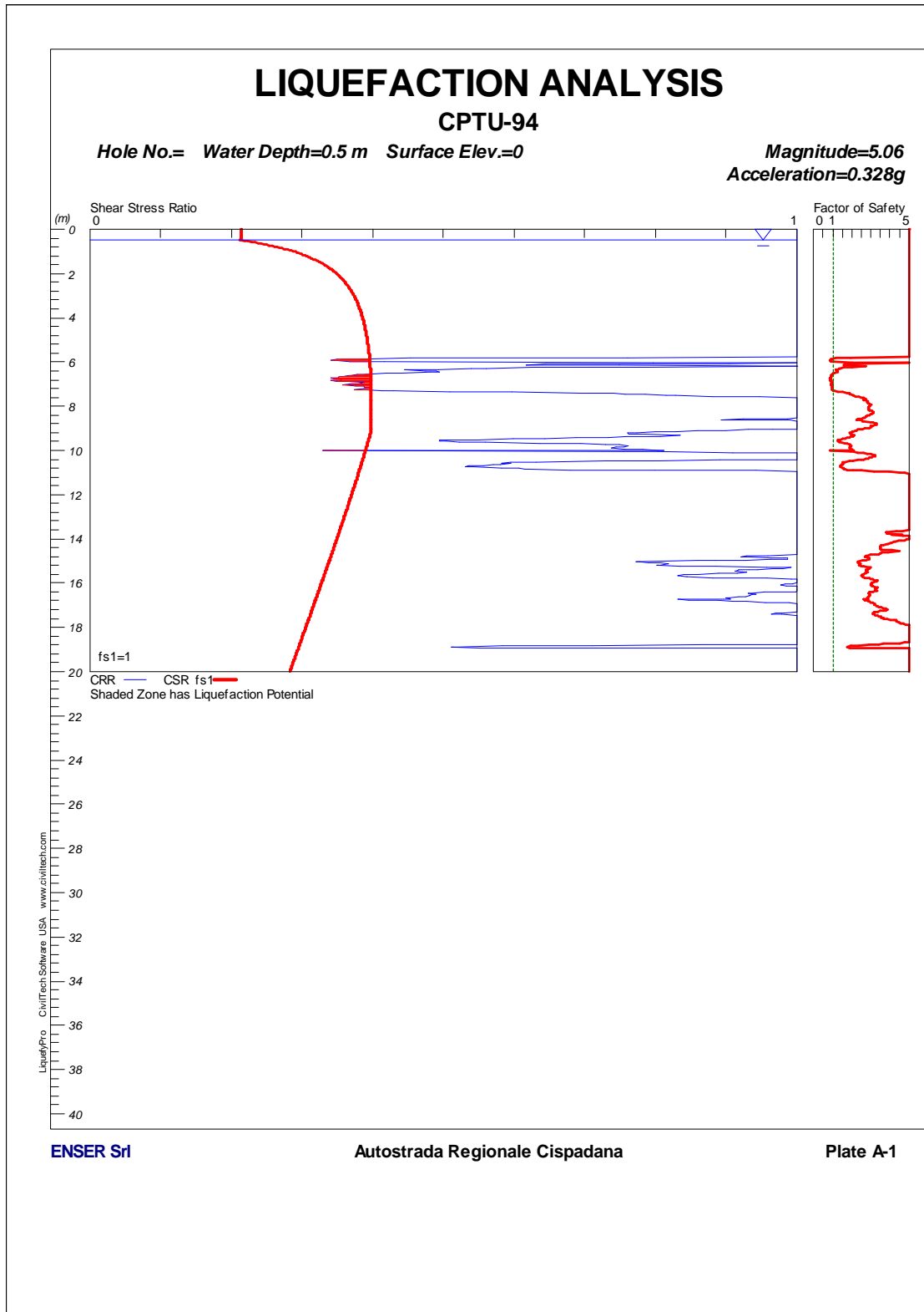
FIGURA 1-56: CPTU94 – VERIFICA A LIQUEFAZIONE.
