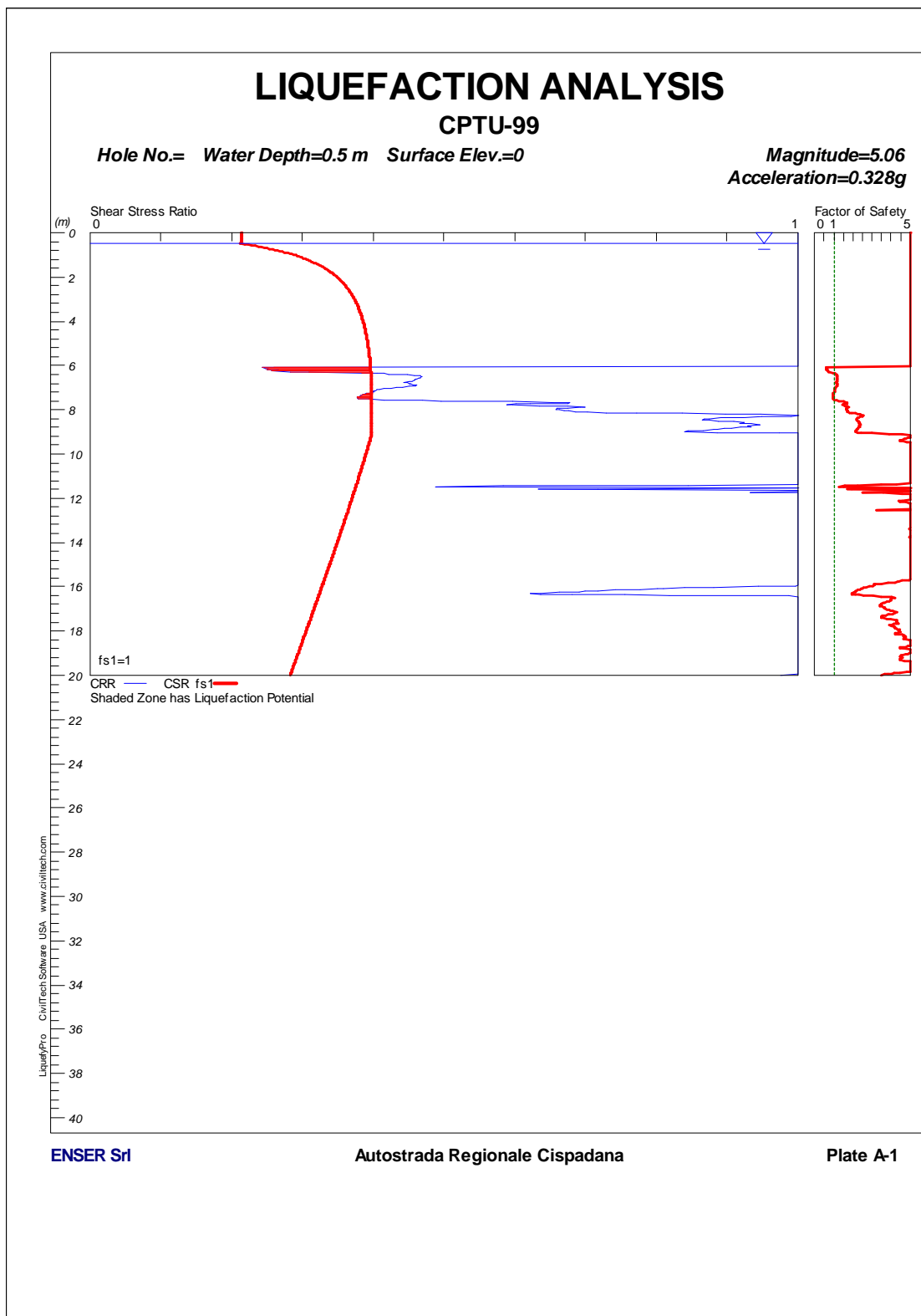
FIGURA 1-60: CPTU99 – VERIFICA A LIQUEFAZIONE.
