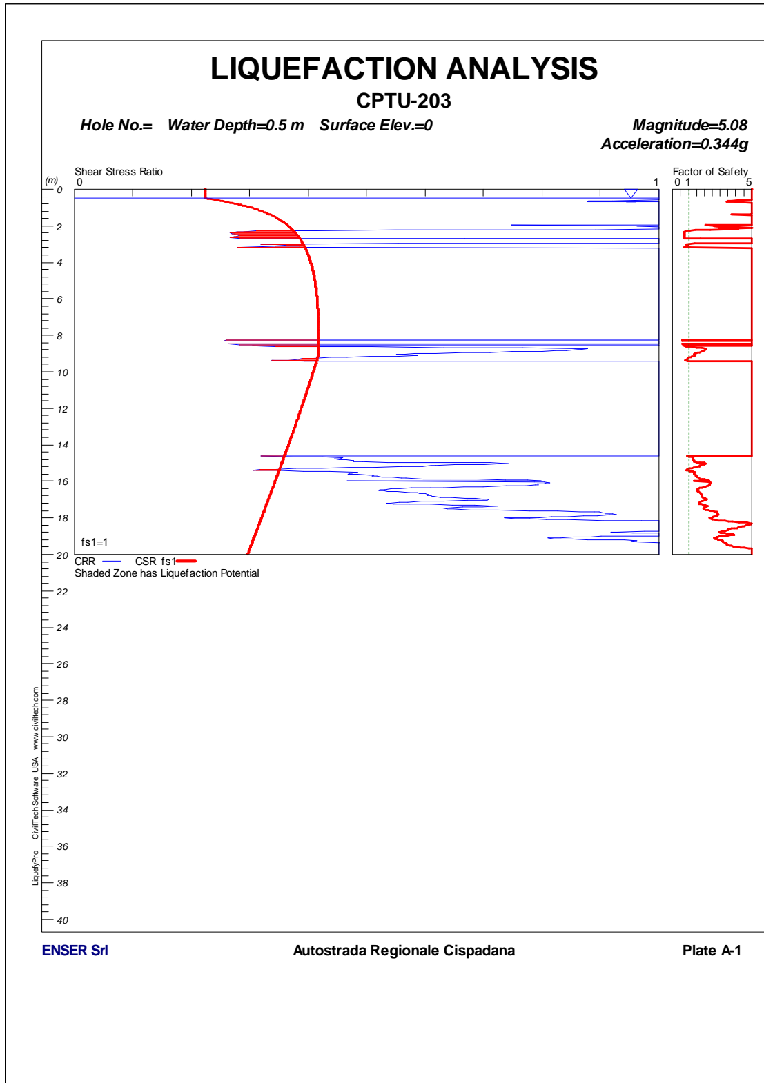
FIGURA 1-92: CPTU203 – VERIFICA A LIQUEFAZIONE.
