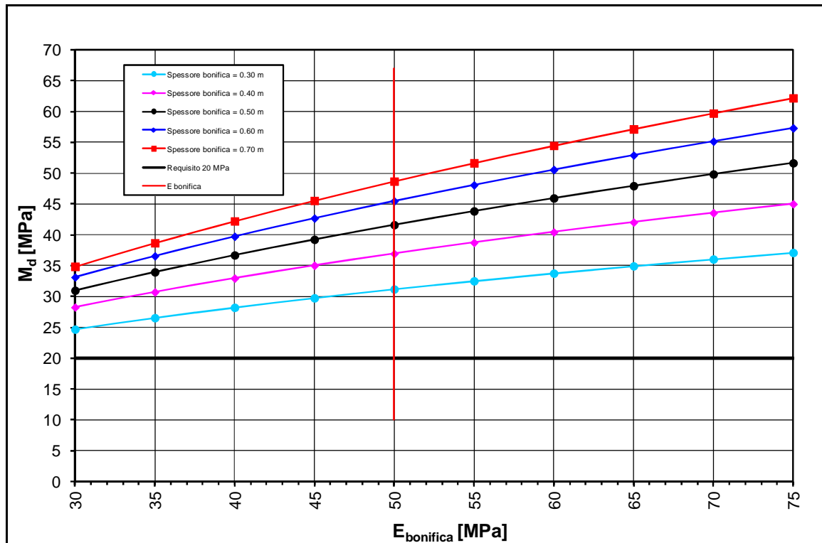
FIGURA 2-54: TRATTO 57 – DETERMINAZIONE SPESSORE DI BONIFICA.
