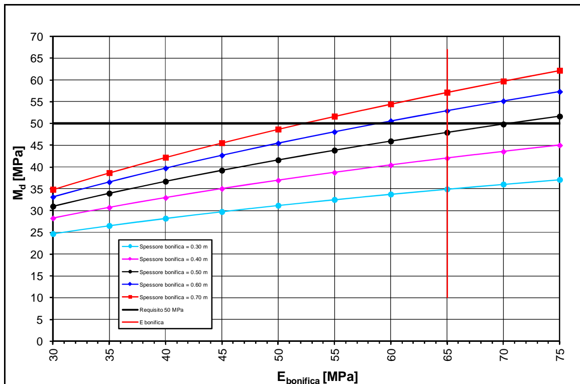
FIGURA 2-61: TRATTO 64 – DETERMINAZIONE SPESSORE DI BONIFICA.
