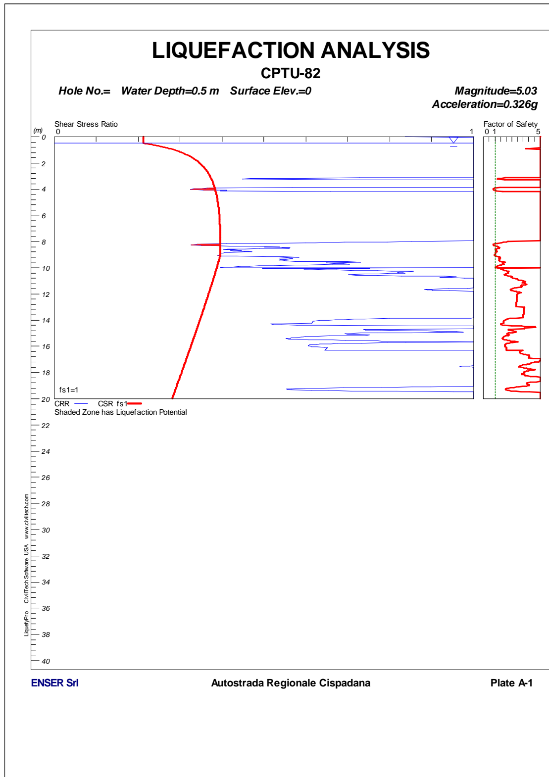
FIGURA 1-50: CPTU82 – VERIFICA A LIQUEFAZIONE.
