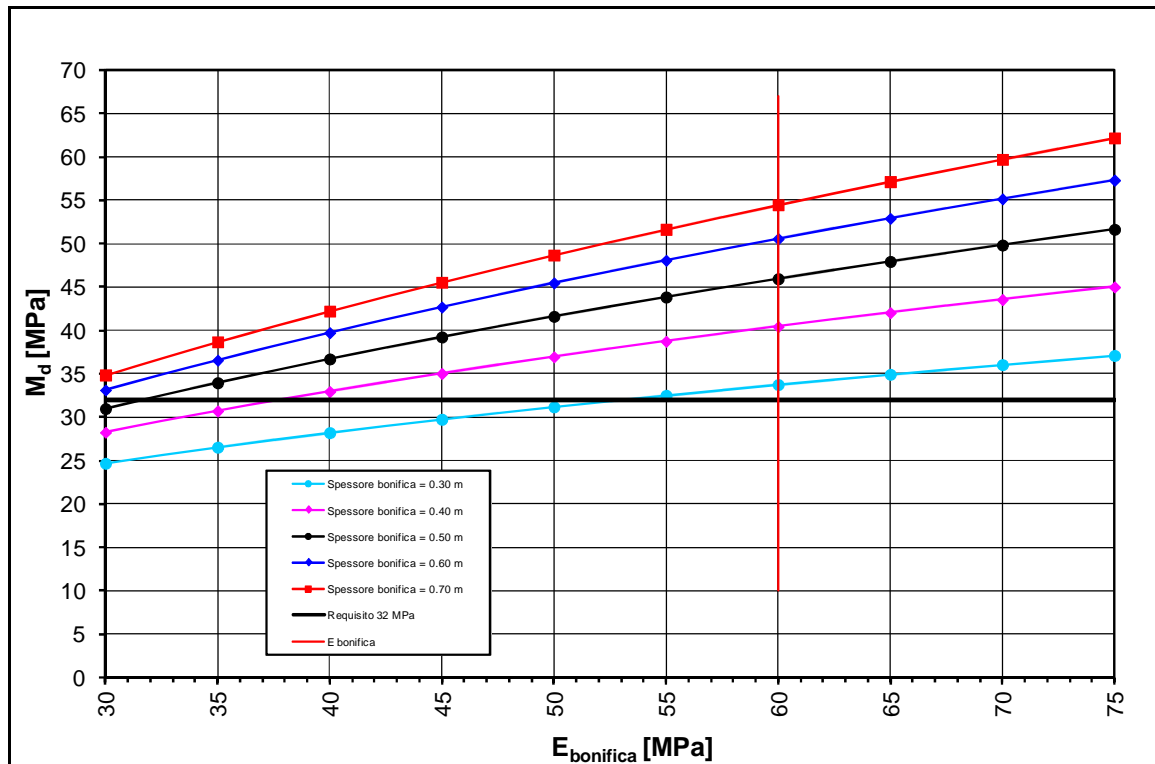
FIGURA 2-8: TRATTO 8 – DETERMINAZIONE SPESSORE DI BONIFICA.
