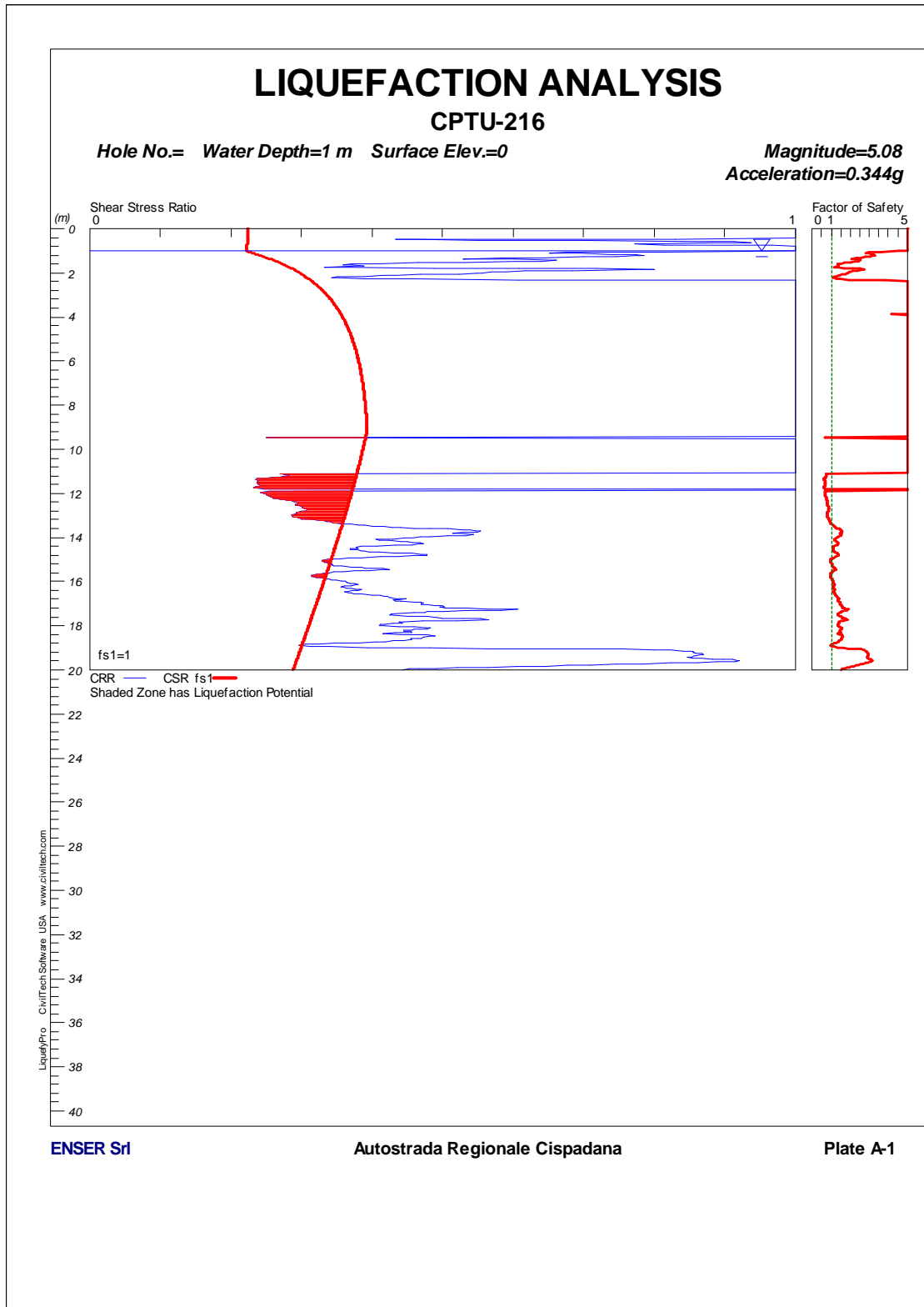
FIGURA 1-100: CPTU216 – Verifica a Liquefazione.
