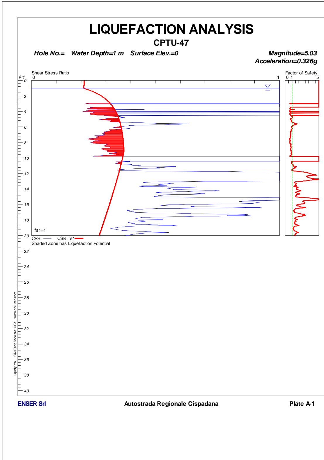
FIGURA 1-22: CPTU47 – VERIFICA A LIQUEFAZIONE.
