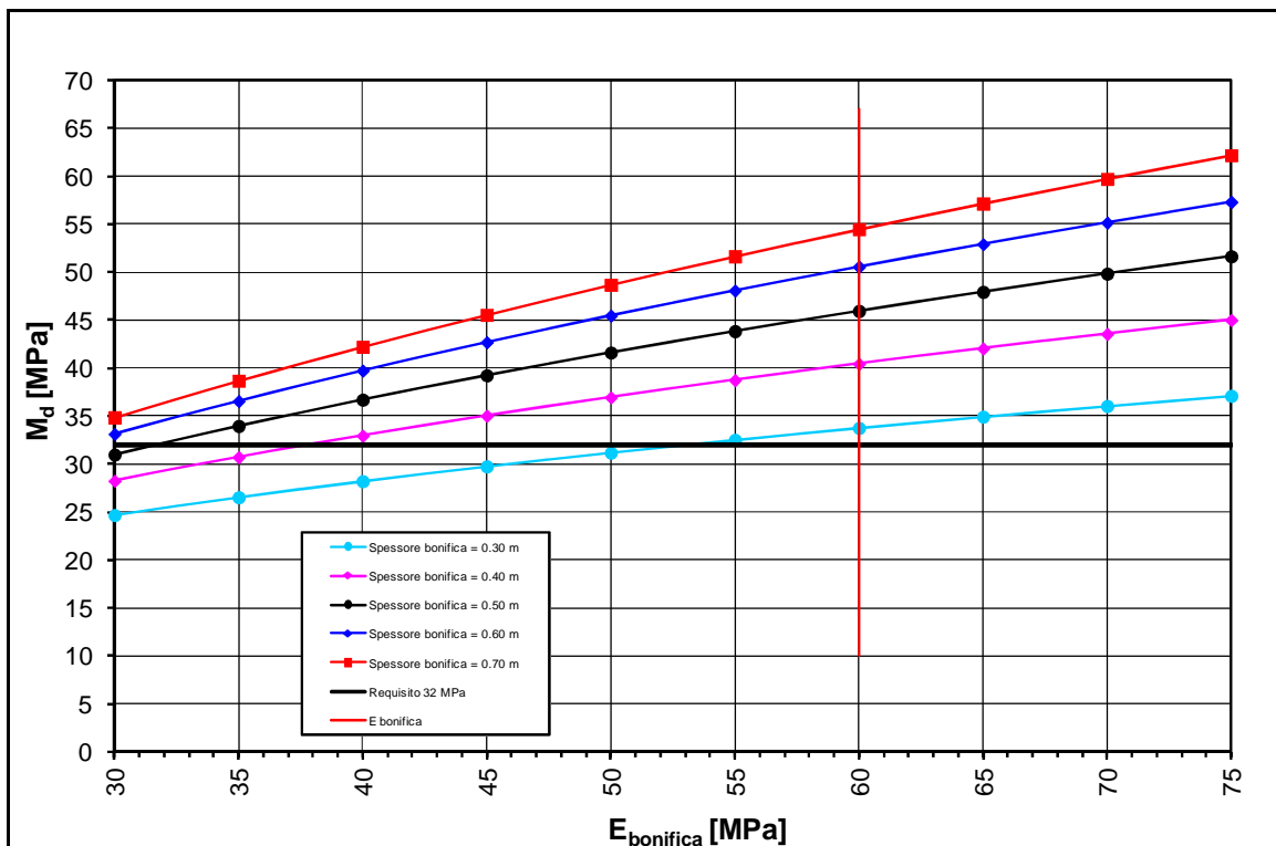
FIGURA 2-23: TRATTO 24 – DETERMINAZIONE SPESSORE DI BONIFICA.
