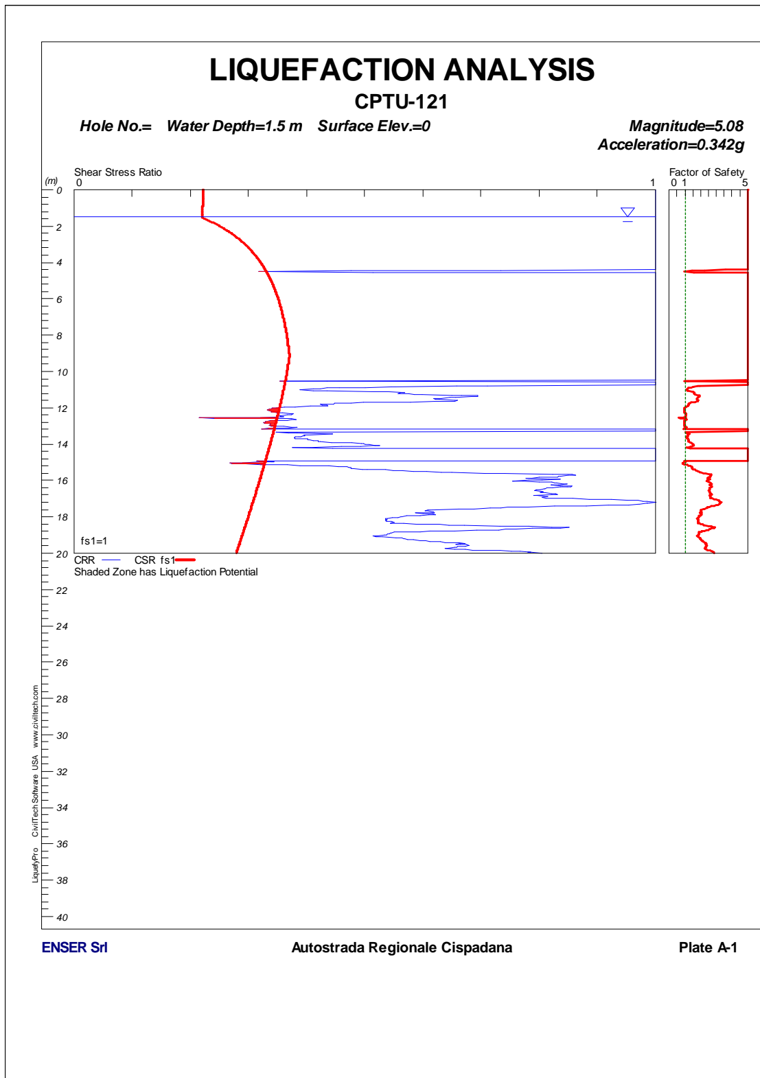
FIGURA 1-81: CPTU121 – VERIFICA A LIQUEFAZIONE.
