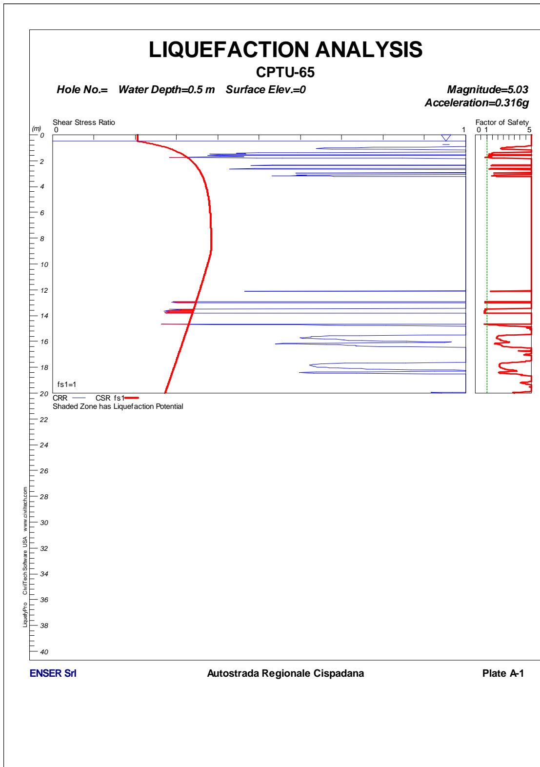
FIGURA 1-40: CPTU65 – VERIFICA A LIQUEFAZIONE.
