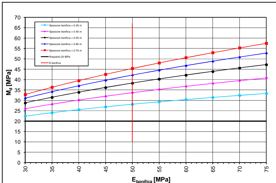
FIGURA 2-49: TRATTO 52 – DETERMINAZIONE SPESSORE DI BONIFICA.
