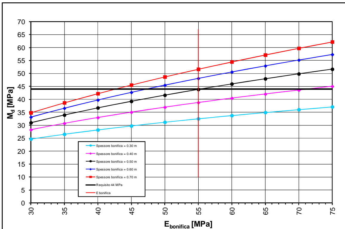
FIGURA 2-13: TRATTO 13 – DETERMINAZIONE SPESSORE DI BONIFICA.
