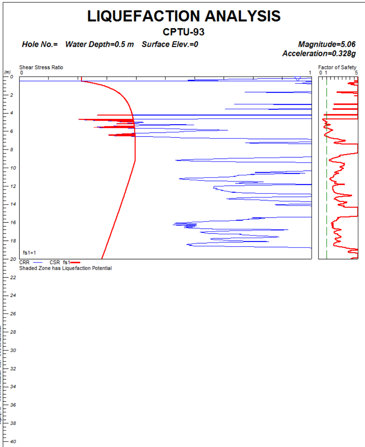
FIGURA 1-55: CPTU93 – VERIFICA A LIQUEFAZIONE.
