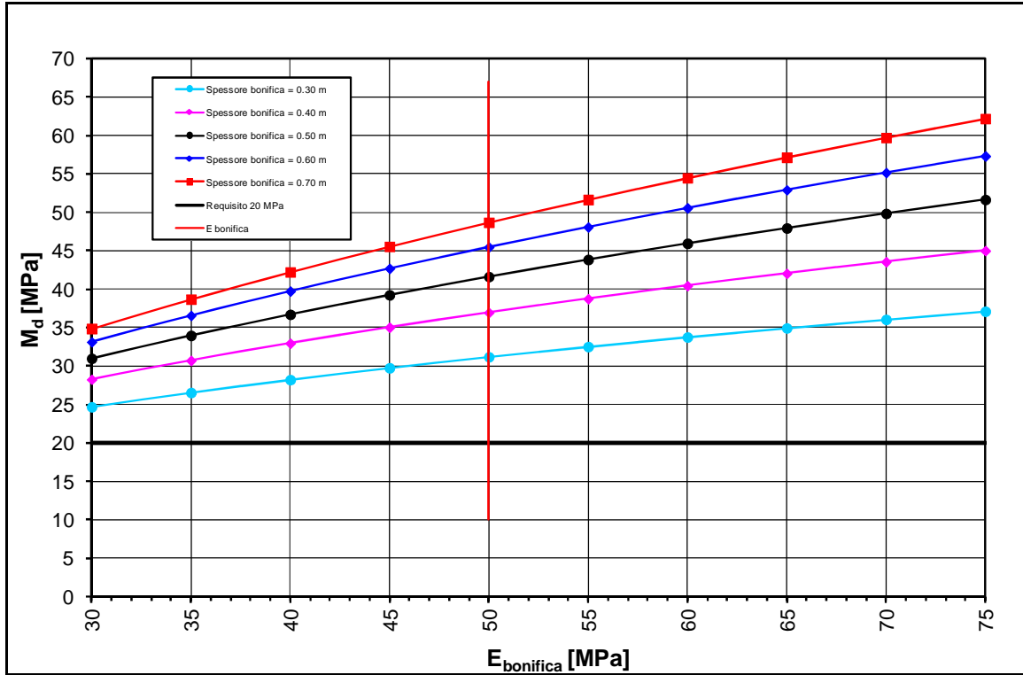
FIGURA 2-56: TRATTO 59 – DETERMINAZIONE SPESSORE DI BONIFICA.
