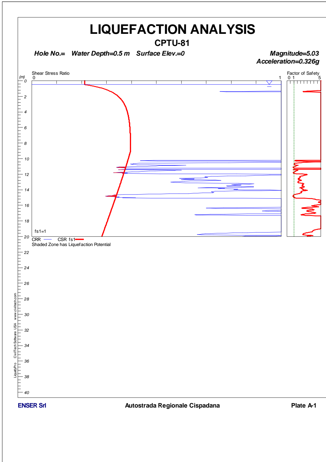
FIGURA 1-49: CPTU81 – VERIFICA A LIQUEFAZIONE.
