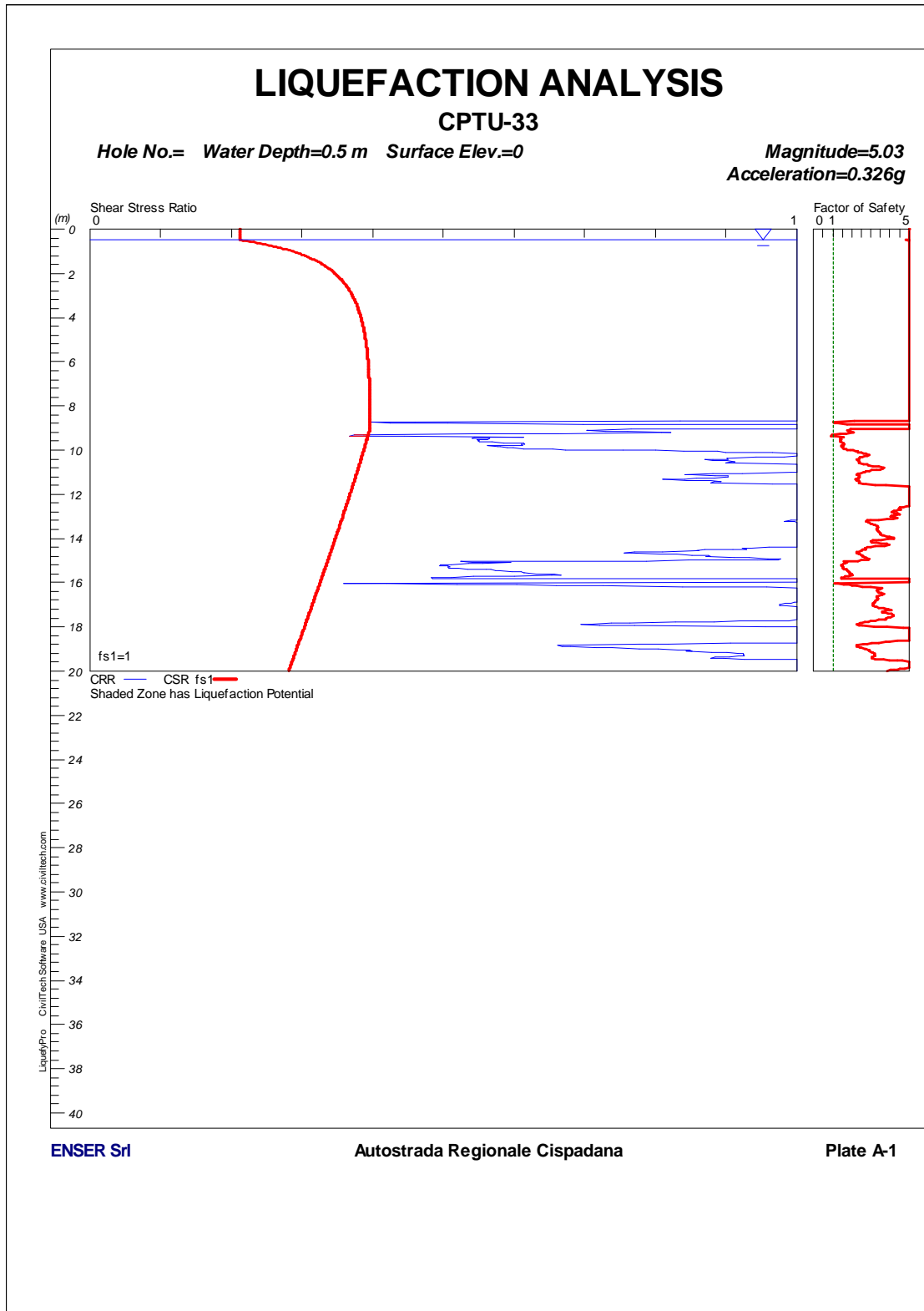
FIGURA 1-11: CPTU33 – VERIFICA A LIQUEFAZIONE.
