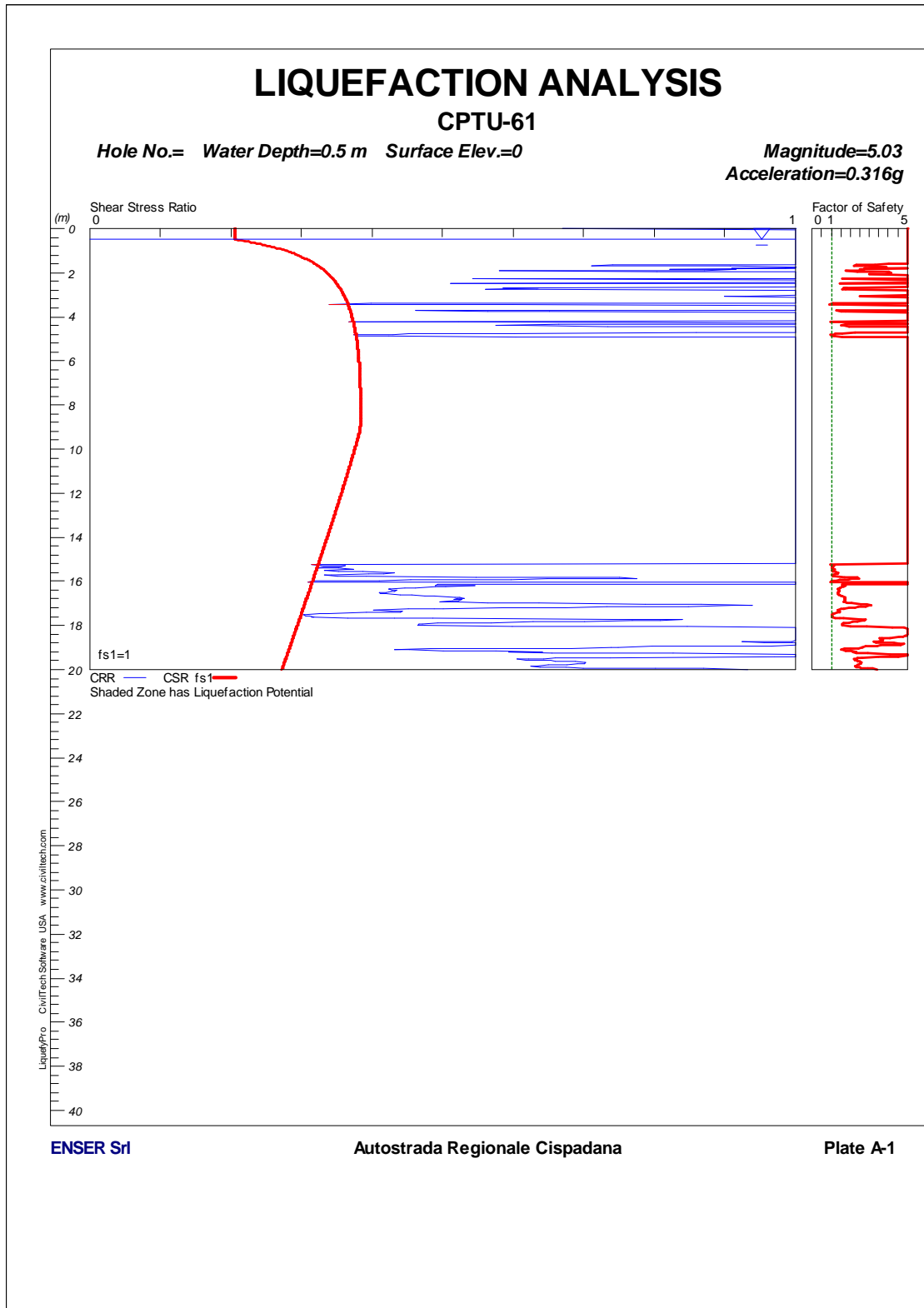
FIGURA 1-36: CPTU61 – VERIFICA A LIQUEFAZIONE.
