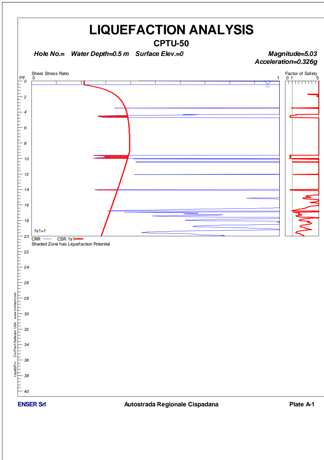
FIGURA 1-25: CPTU50 – VERIFICA A LIQUEFAZIONE.
