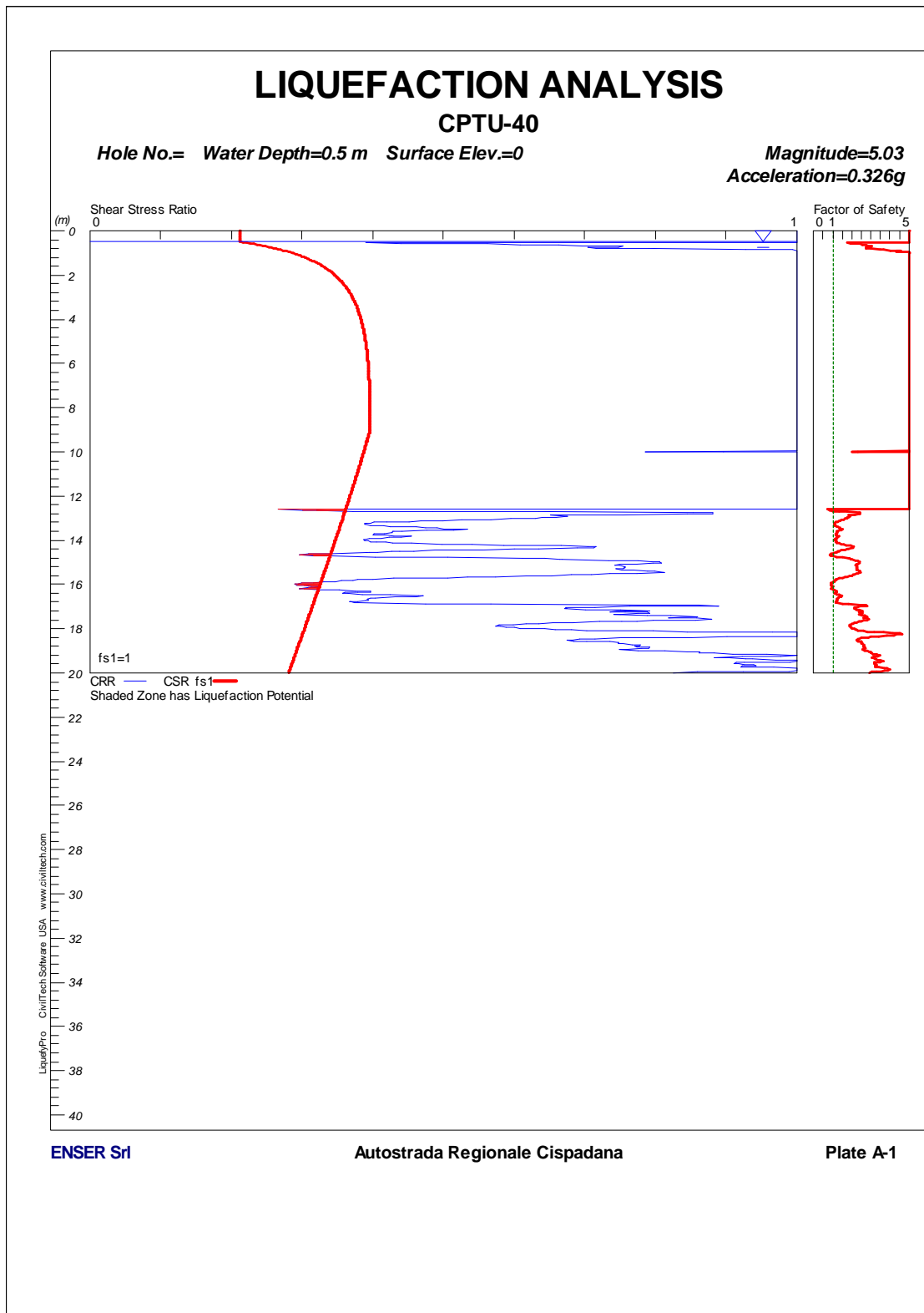
FIGURA 1-15: CPTU40 – VERIFICA A LIQUEFAZIONE.
