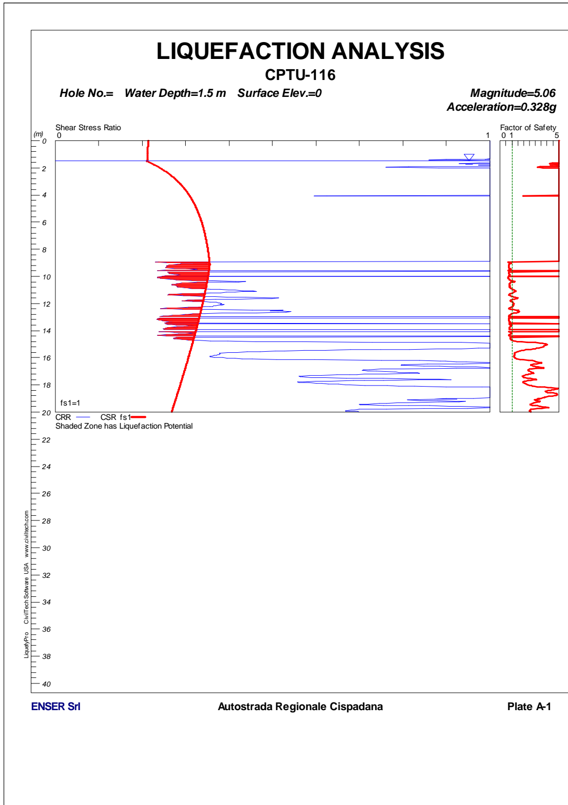
FIGURA 1-76: CPTU116 – VERIFICA A LIQUEFAZIONE.
