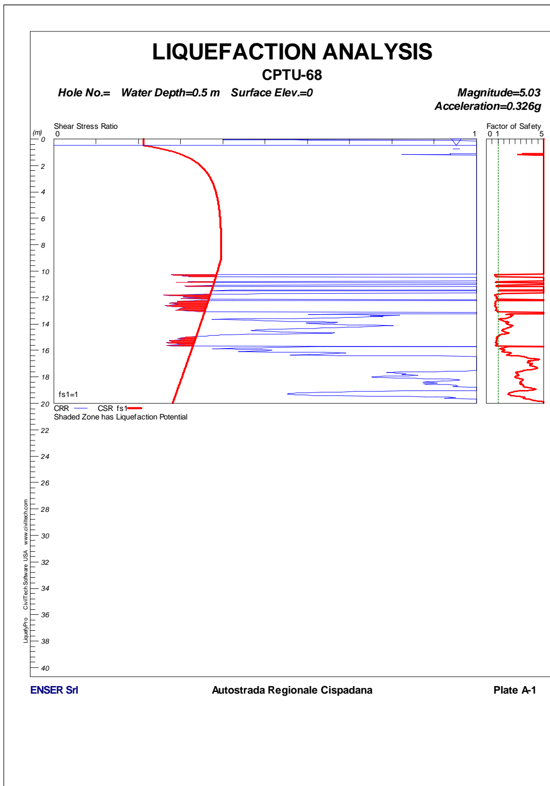
FIGURA 1-43: CPTU68 – VERIFICA A LIQUEFAZIONE.
