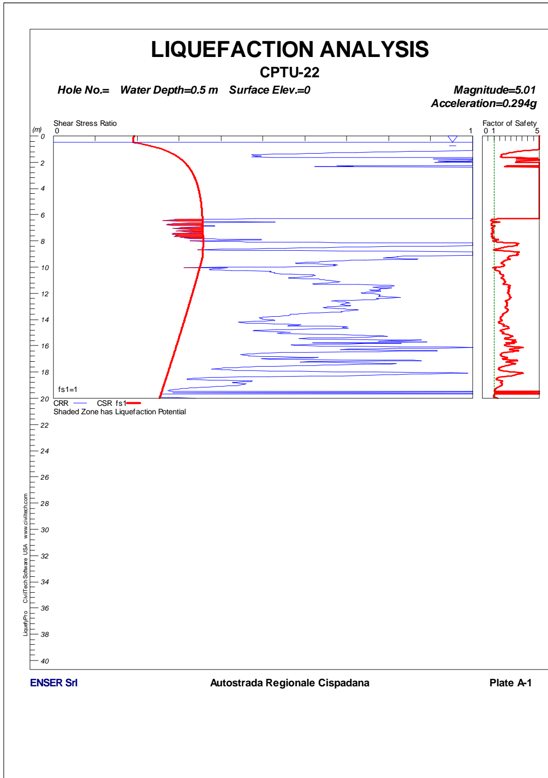
FIGURA 1-3: CPTU22 – VERIFICA A LIQUEFAZIONE.
