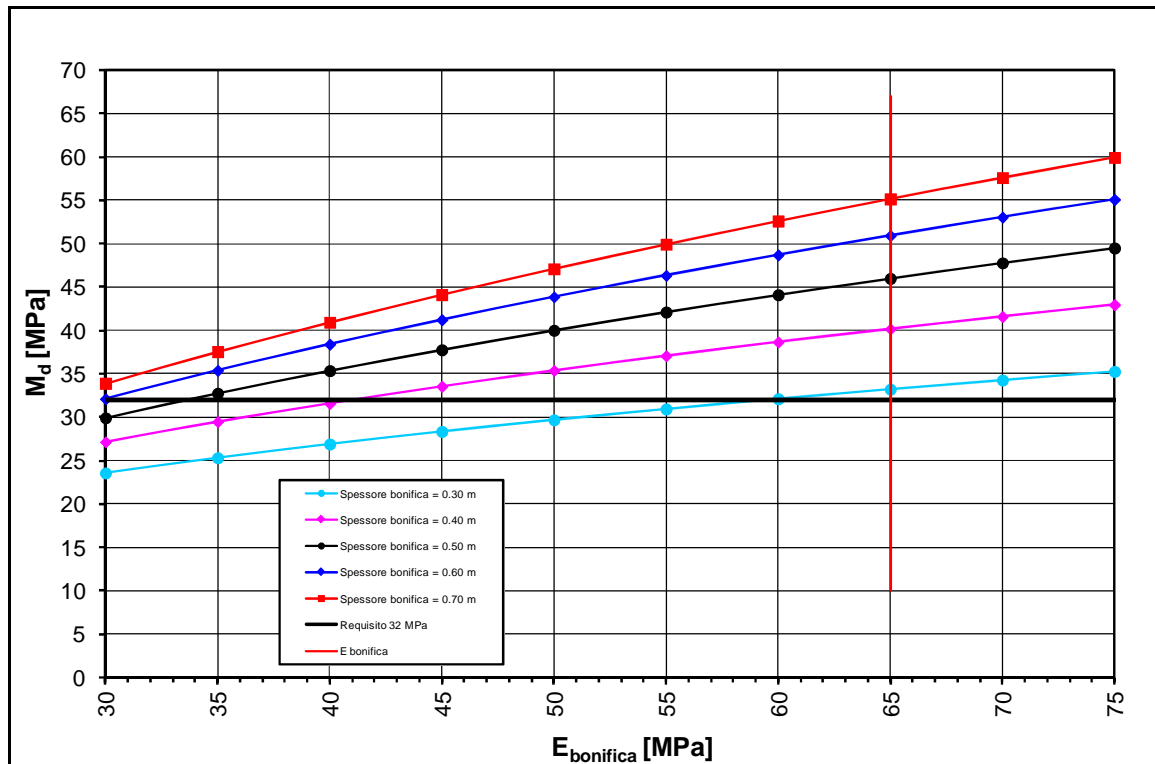
FIGURA 2-30: TRATTO 31 – DETERMINAZIONE SPESSORE DI BONIFICA.
