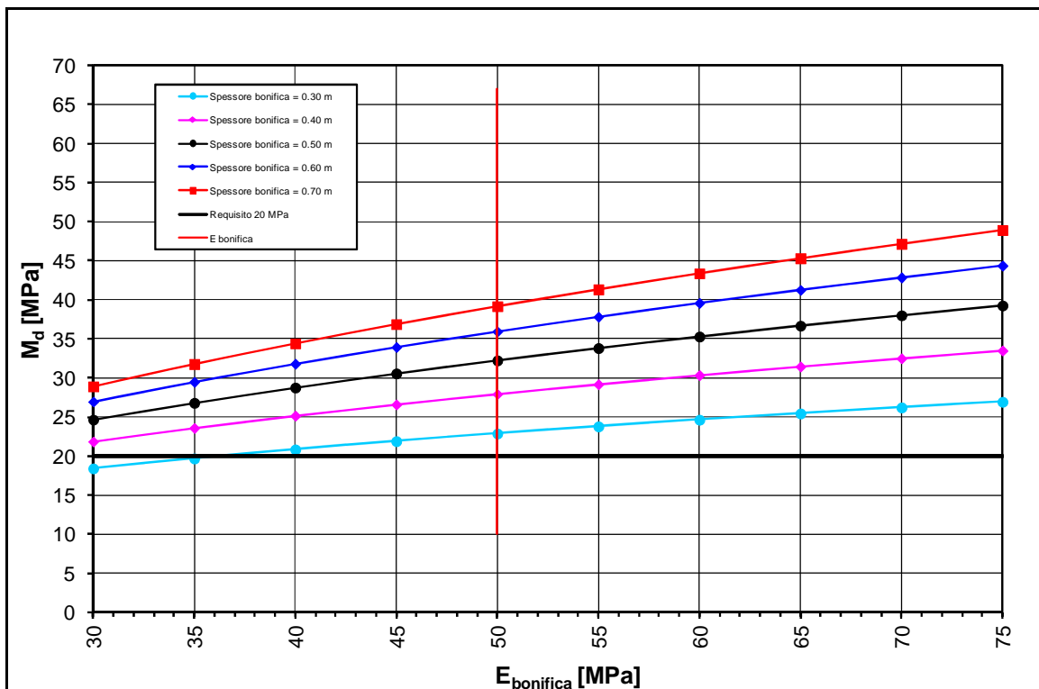
FIGURA 2-41: TRATTO 42, 43, 44 – DETERMINAZIONE SPESSORE DI BONIFICA.
