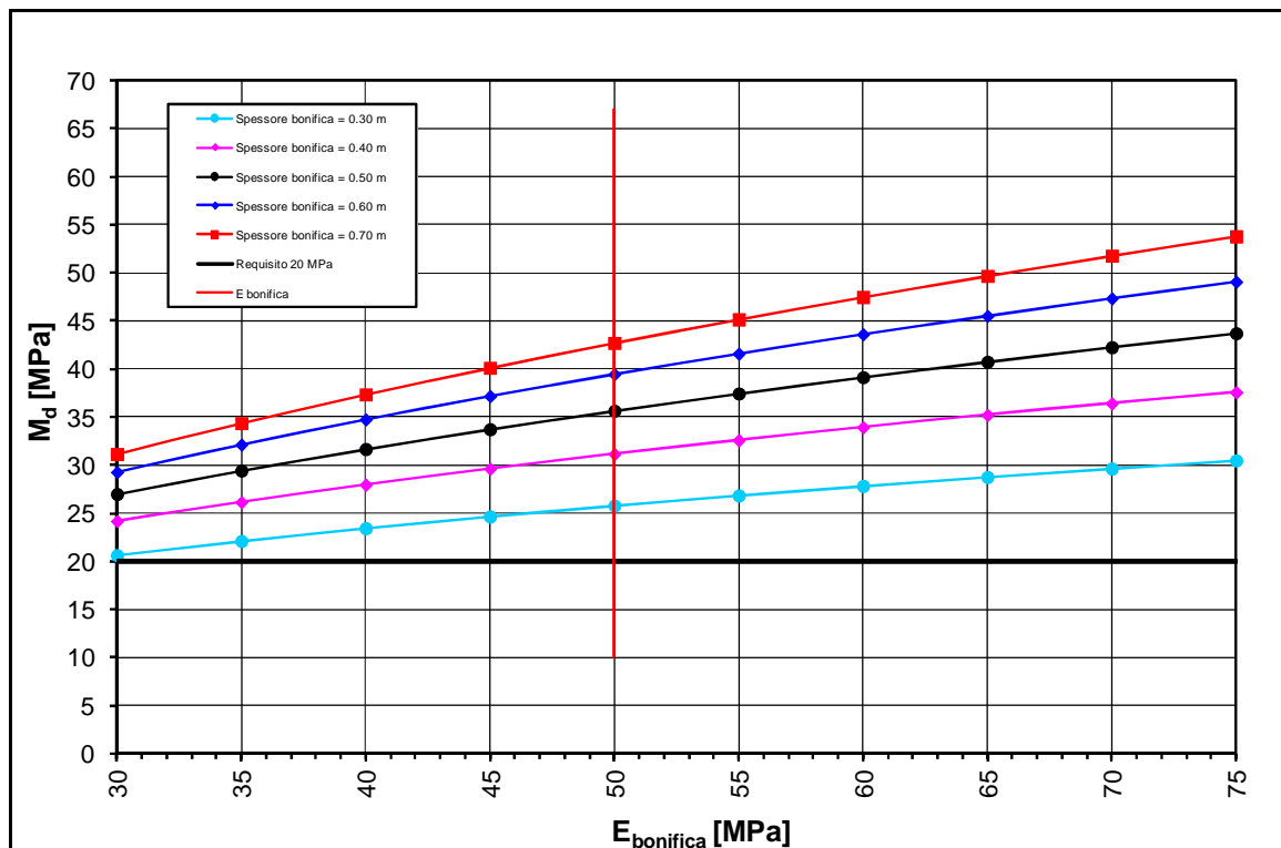
FIGURA 2-27: TRATTO 28 – DETERMINAZIONE SPESSORE DI BONIFICA.
