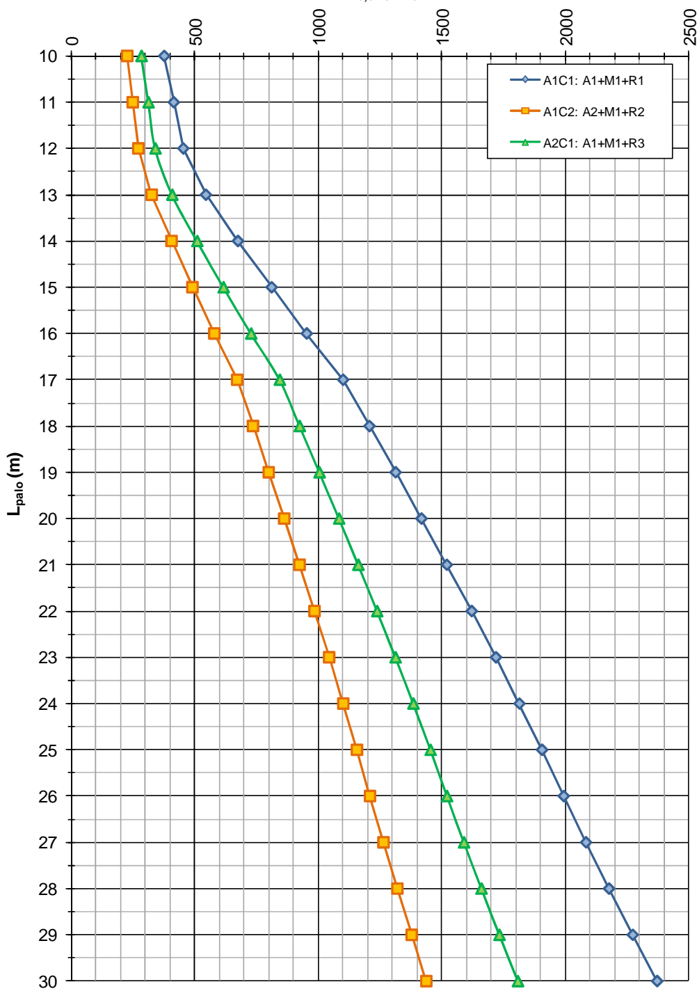
IMU02 - IMU03 - IMU04 - Interconnessione con A22 (Muri U) - ZO2 - Est NTC del 14/01/2008 Capacità portante a compressione - Pali trivellati \phi 600mm R_{c,d} (KN)
