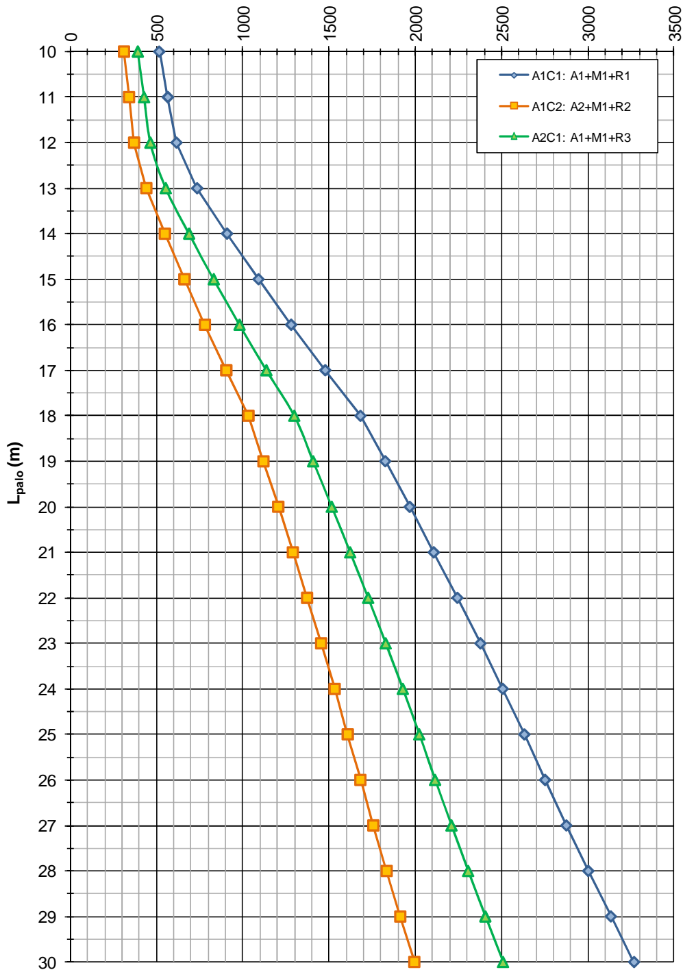
FIGURA 6-11: CAPACITÀ PORTANTE A COMPRESSIONE – PALI TRIVELLATI \phi 800 (IMU05)
