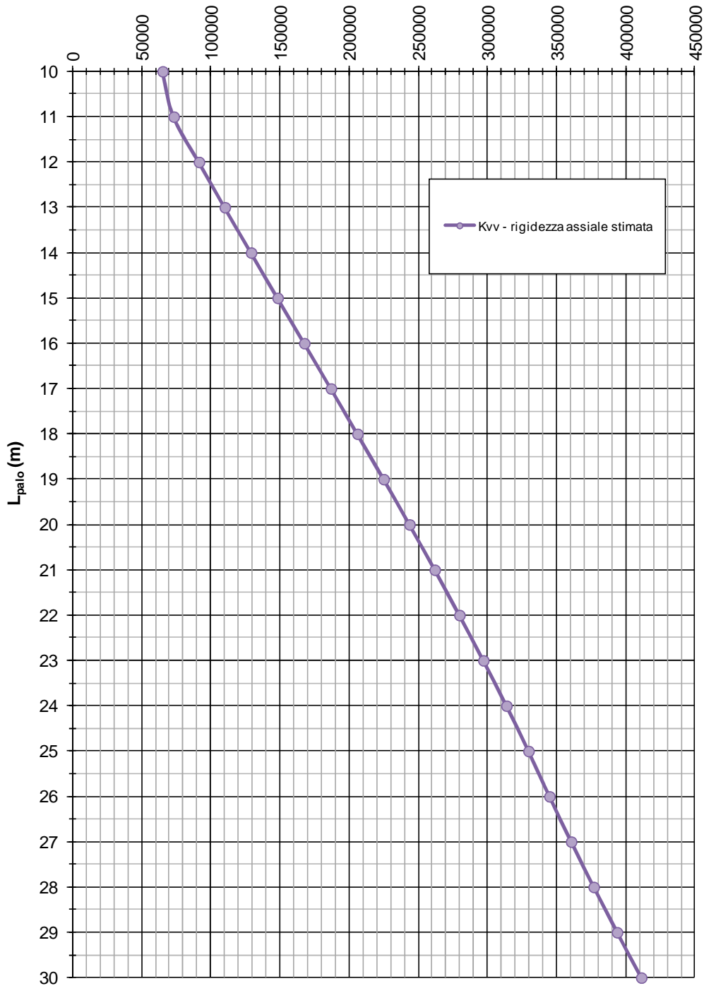
IMU02 - IMU03 - IMU04 - Interconnessione con A22 (Muri U) - ZO2 - Ovest NTC del 14/01/2008 Rigidezza assiale - Pali trivellati \phi 800mm K_{VV} (KN/m)
