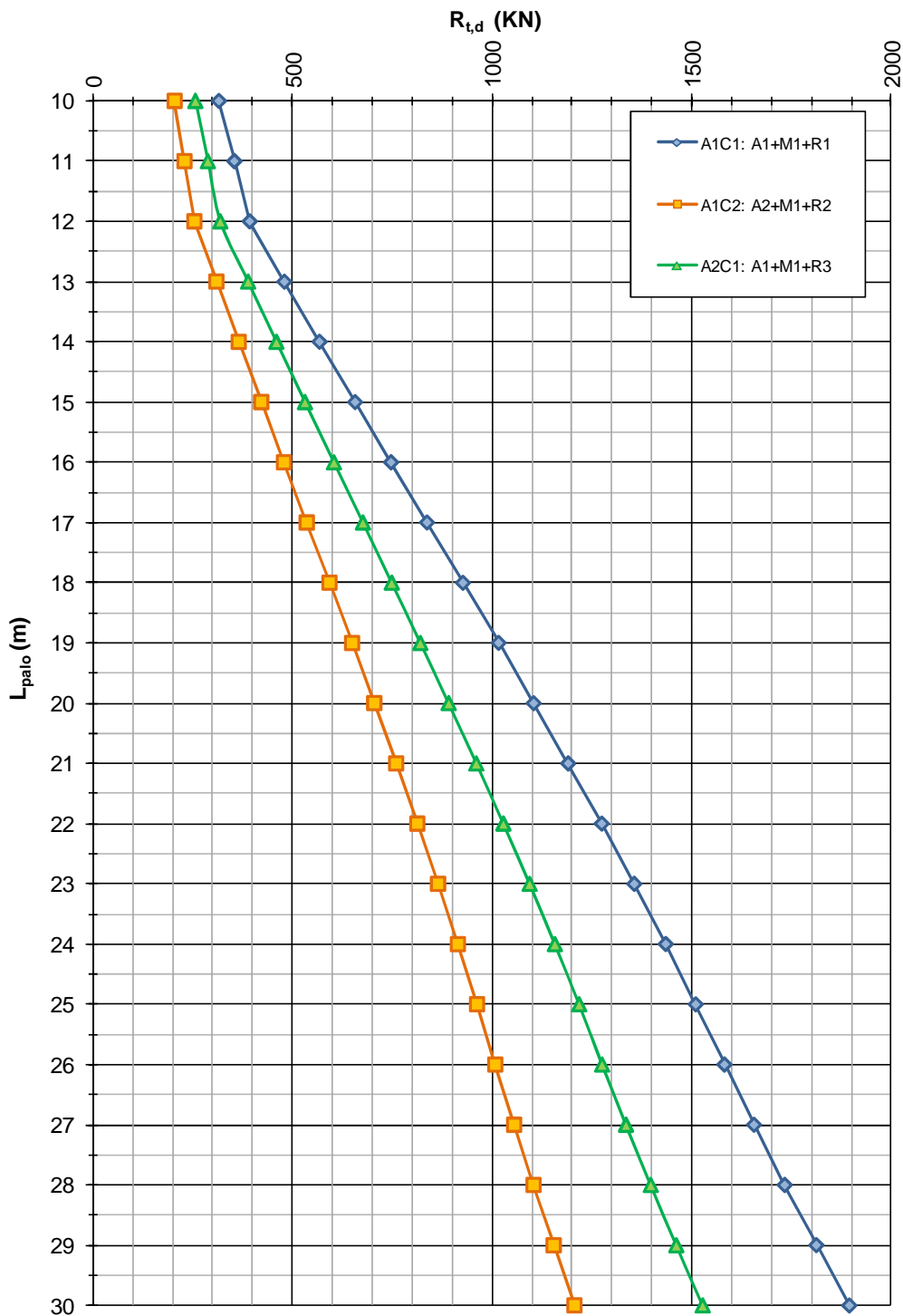
FIGURA 6-10: CAPACITÀ PORTANTE A TRAZIONE – PALI TRIVELLATI \phi 600 (IMU05)
