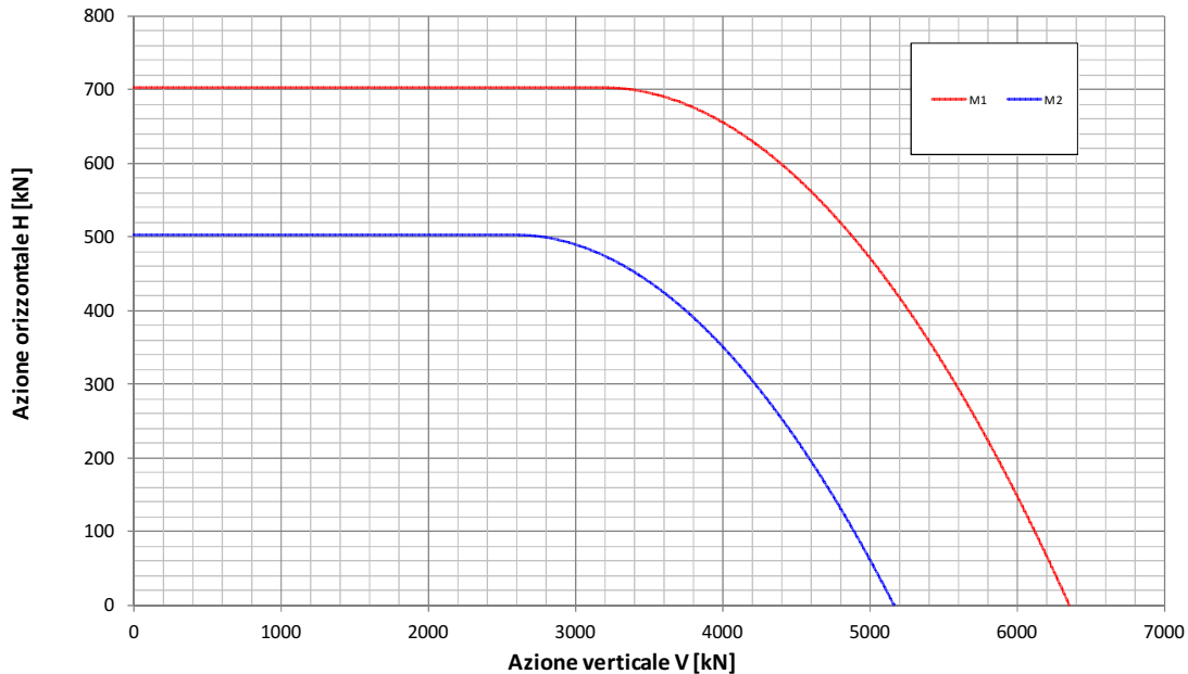
Fondazione B=17.60m - Approfondimento D=6.70m Condizione Statica Non Drenata Dominio di interazione nel piano V-H ( Gourvenec, 2007 )
