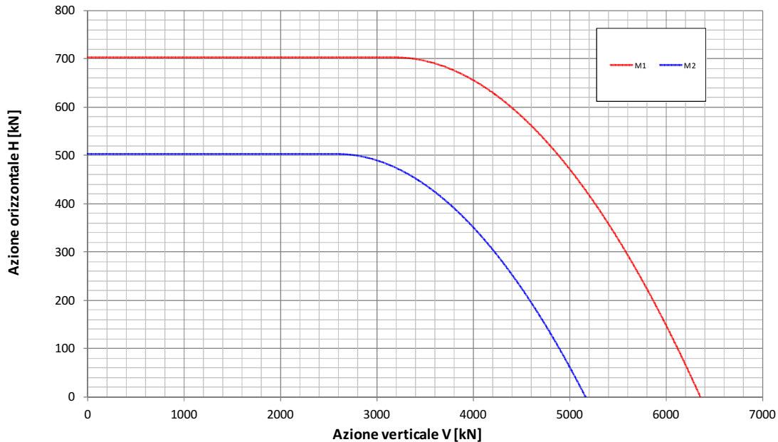
Fondazione B=17.60m - Approfondimento D=6.70m Condizione Sismica Non Drenata Dominio di interazione nel piano V-H ( Gourvenec, 2007 )
