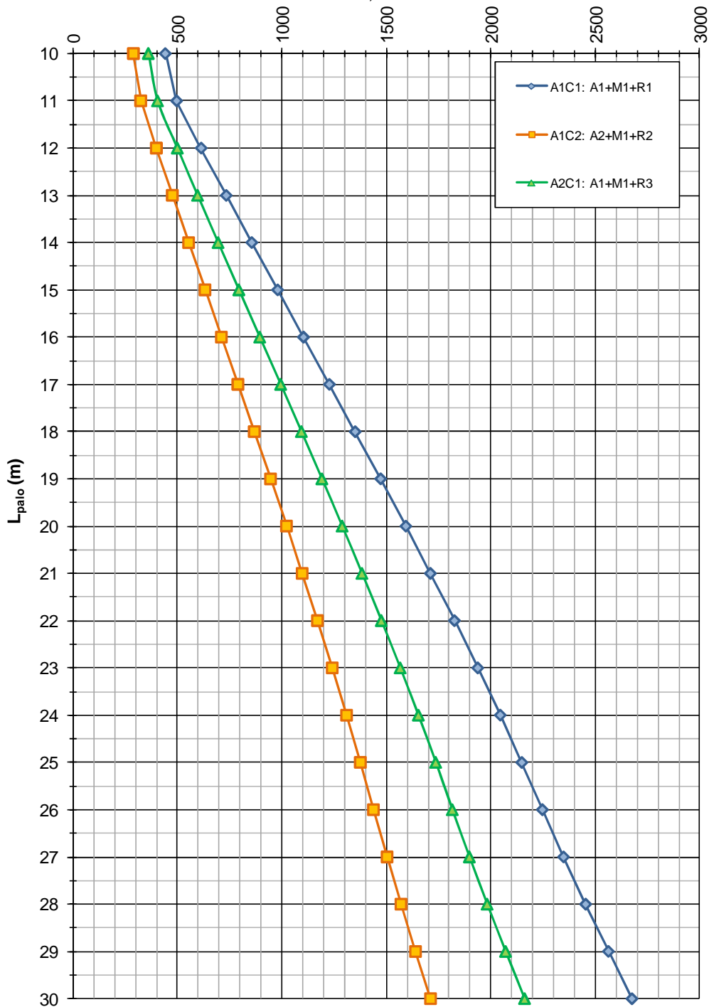
IMU02 - IMU03 - IMU04 - Interconnessione con A22 (Muri U) - ZO2 - Ovest NTC del 14/01/2008 Capacità portante a trazione - Pali trivellati \phi 800mm R_{t,d} (KN)
