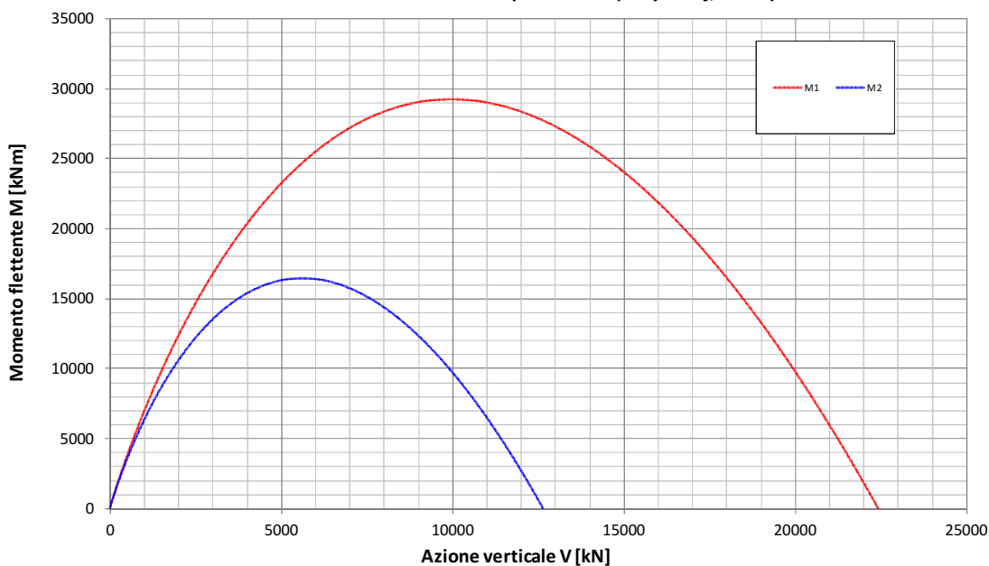
Fondazione B=17.60m - Approfondimento D=6.70m Condizione Statica Drenata Dominio di interazione nel piano V-M ( Meyerhof, 1953 )
