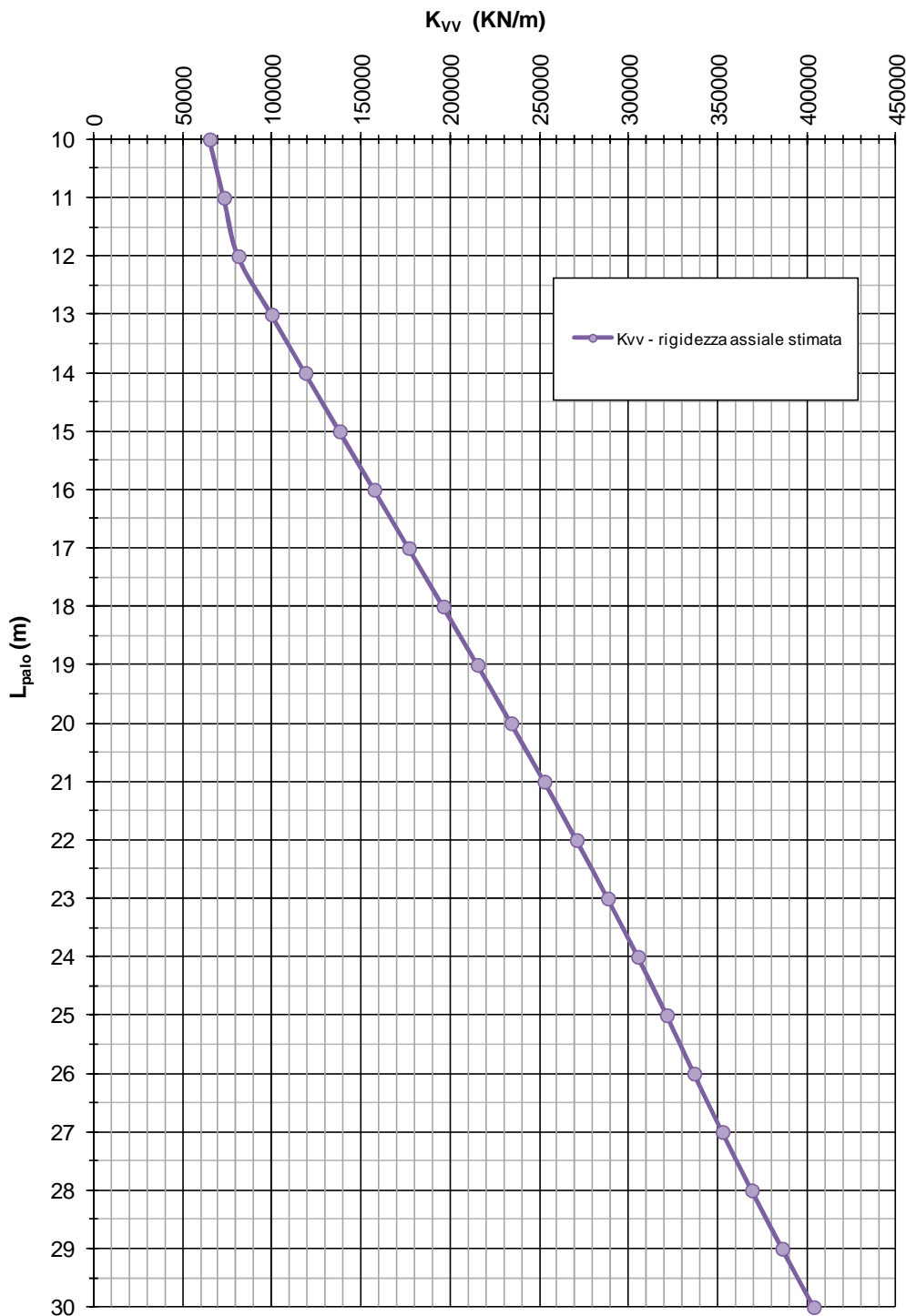
FIGURA 8-7: RIGIDEZZA VERTICALE – PALI TRIVELLATI \phi 800 (IMU05)
