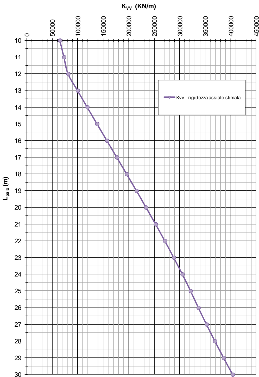
FIGURA 8-5: RIGIDEZZA VERTICALE – PALI TRIVELLATI \phi 800 (IMU02, IMU03, IMU04 – LATO EST)
