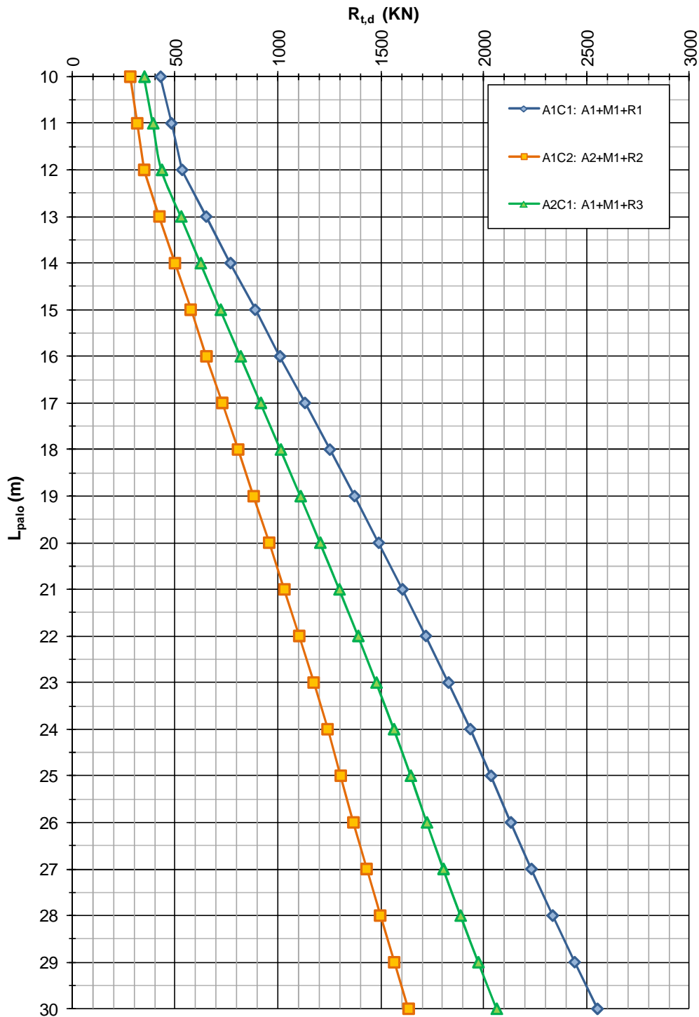
FIGURA 6-12: CAPACITÀ PORTANTE A TRAZIONE – PALI TRIVELLATI \phi 800 (IMU05)
