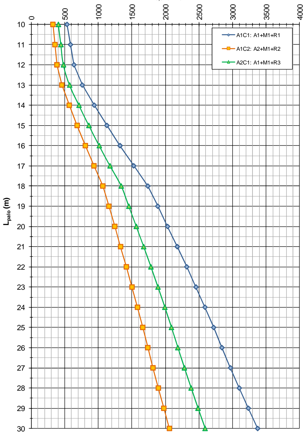
IMU02 - IMU03 - IMU04 - Interconnessione con A22 (Muri U) - ZO2 - Est NTC del 14/01/2008 Capacità portante a compressione - Pali trivellati \phi 800mm R_{c,d} (KN)
