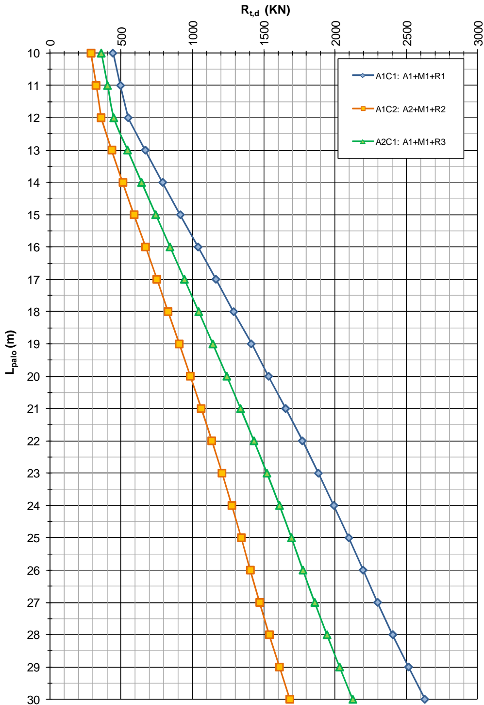
IMU02 - IMU03 - IMU04 - Interconnessione con A22 (Muri U) - ZO2 - Est NTC del 14/01/2008 Capacità portante a trazione - Pali trivellati \phi 800mm
