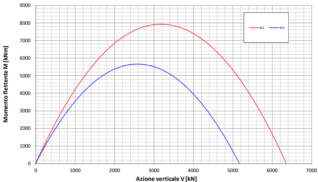
Fondazione B=17.60m - Approfondimento D=6.70m Condizione Sismica Non Drenata Dominio di interazione nel piano V-M ( Gourvenec, 2007 )
