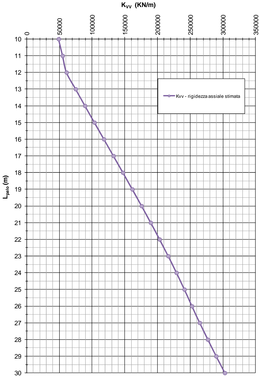
FIGURA 8-6: RIGIDEZZA VERTICALE – PALI TRIVELLATI \phi 600 (IMU05)
