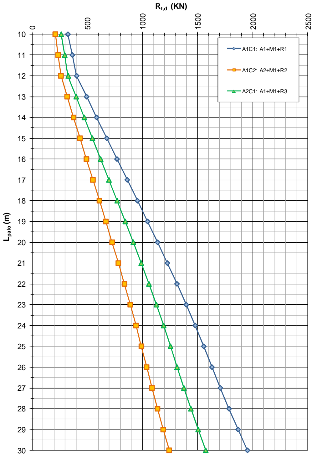
IMU02 - IMU03 - IMU04 - Interconnessione con A22 (Muri U) - ZO2 - Est NTC del 14/01/2008 Capacità portante a trazione - Pali trivellati \phi 600mm
