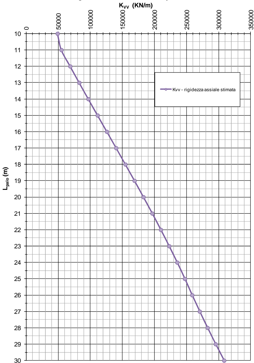
FIGURA 8-2: RIGIDEZZA VERTICALE – PALI TRIVELLATI \phi 600 (IMU02, IMU03, IMU04 – LATO OVEST)
