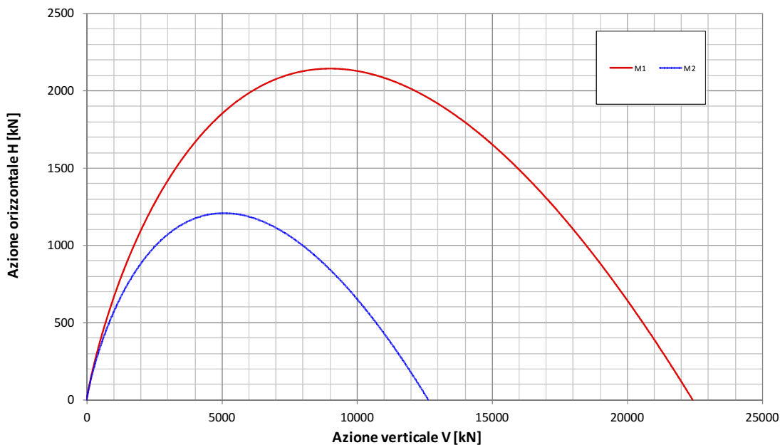
Fondazione B=17.60m - Approfondimento D=6.70m Condizione Statica Drenata Dominio di interazione nel piano V-H ( Brinch Hansen, 1970 )
