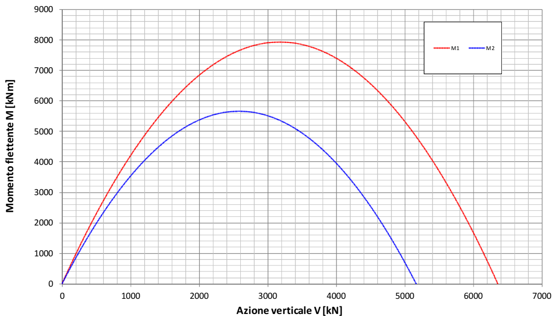
Fondazione B=17.60m - Approfondimento D=6.70m Condizione Statica Non Drenata Dominio di interazione nel piano V-M ( Gourvenec, 2007 )
