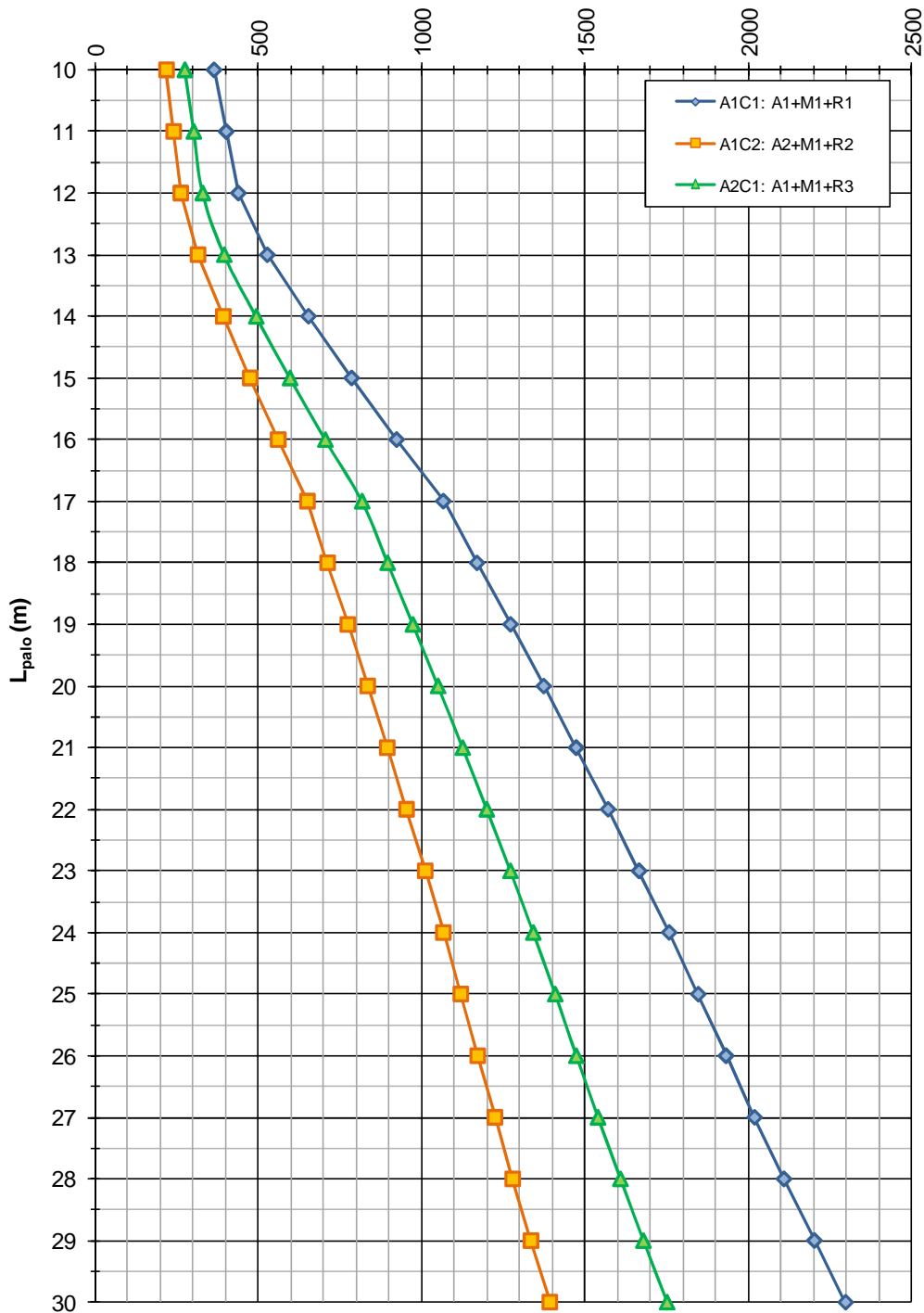
FIGURA 6-9: CAPACITÀ PORTANTE A COMPRESSIONE – PALI TRIVELLATI \phi 600 (IMU05)
