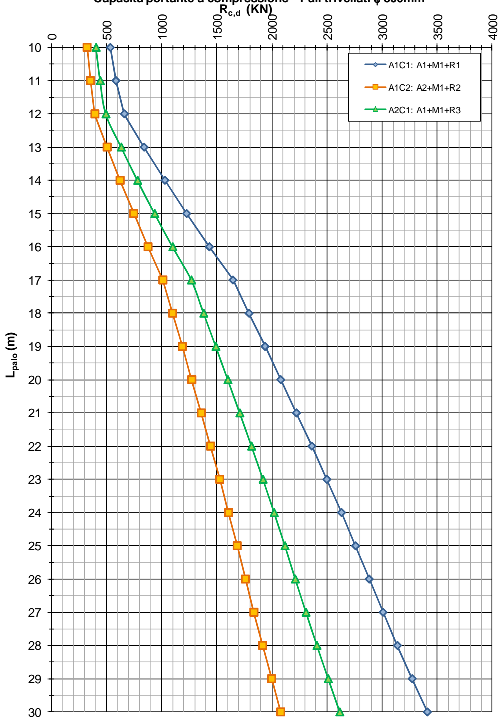
FIGURA 6-3: CAPACITÀ PORTANTE A COMPRESSIONE – PALI TRIVELLATI \phi 800 (IMU02, IMU03, IMU04 – LATO OVEST)
