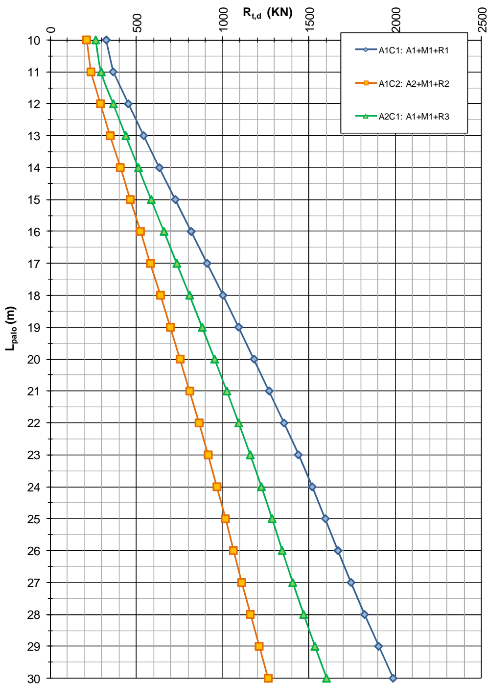
FIGURA 6-2: CAPACITÀ PORTANTE A TRAZIONE – PALI TRIVELLATI \phi 600 (IMU02, IMU03, IMU04 – LATO OVEST)
