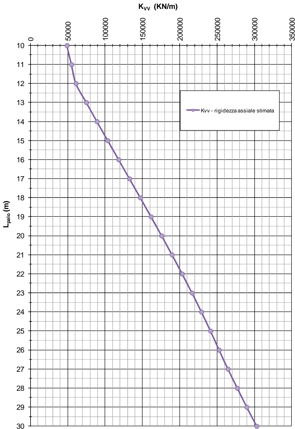
IMU02 - IMU03 - IMU04 - Interconnessione con A22 (Muri U) - ZO2 - Est NTC del 14/01/2008 Rigidezza assiale - Pali trivellati \phi 600mm
