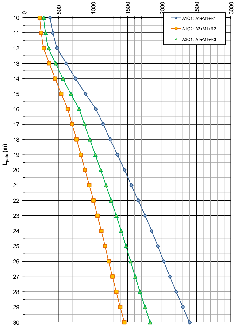
IMU02 - IMU03 - IMU04 - Interconnessione con A22 (Muri U) - ZO2 - Ovest NTC del 14/01/2008 Capacità portante a compressione - Pali trivellati \phi 600mm R_{c,d} (KN)
