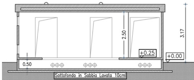
SEZIONE A-A
