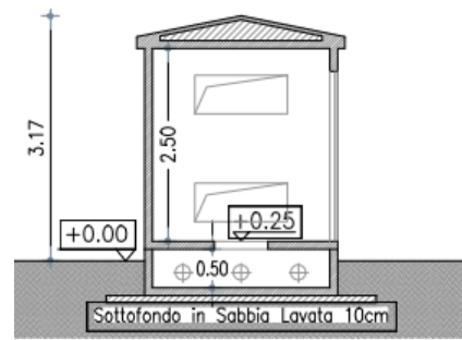
SEZIONE B-B
